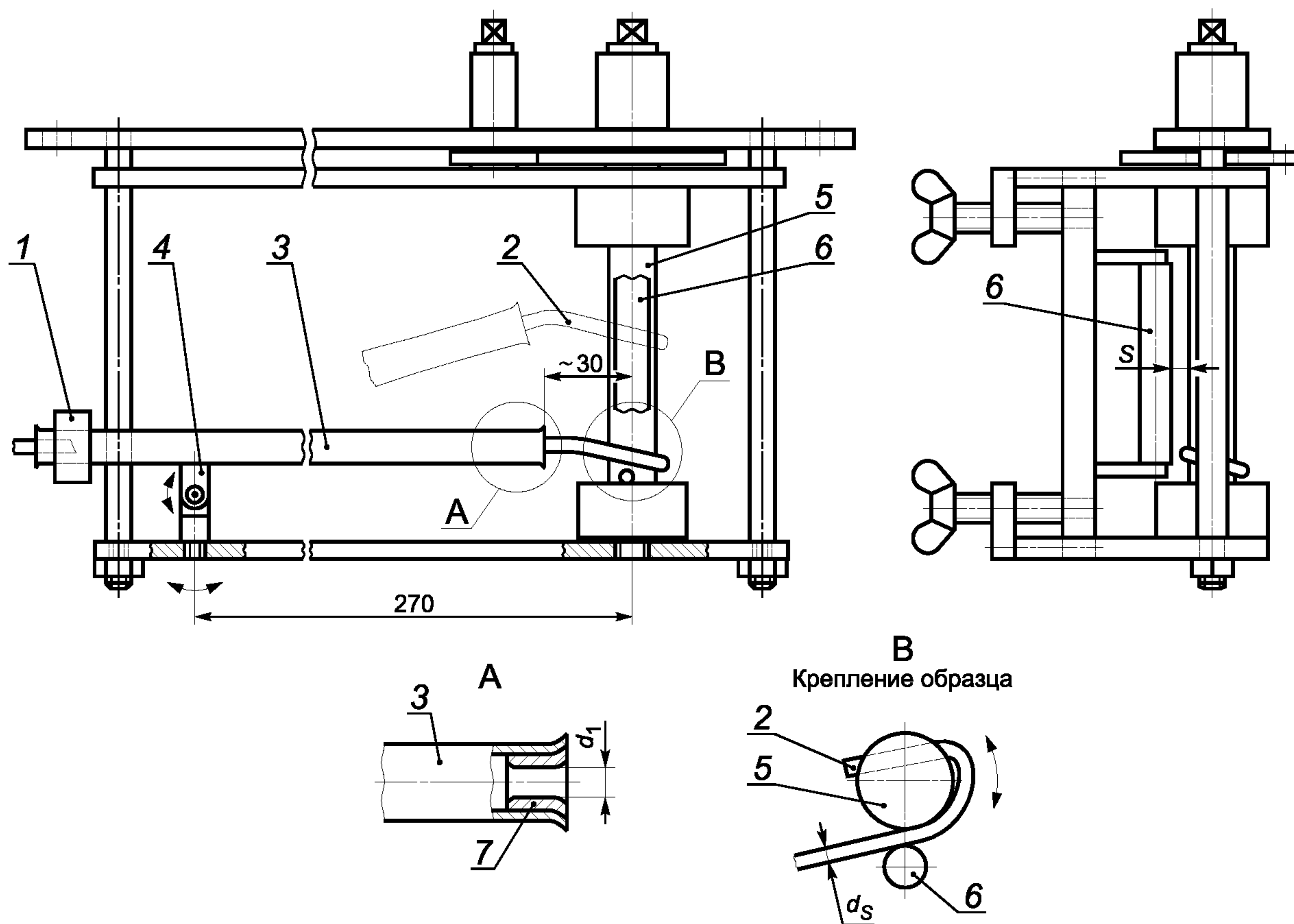
Вид спереди
