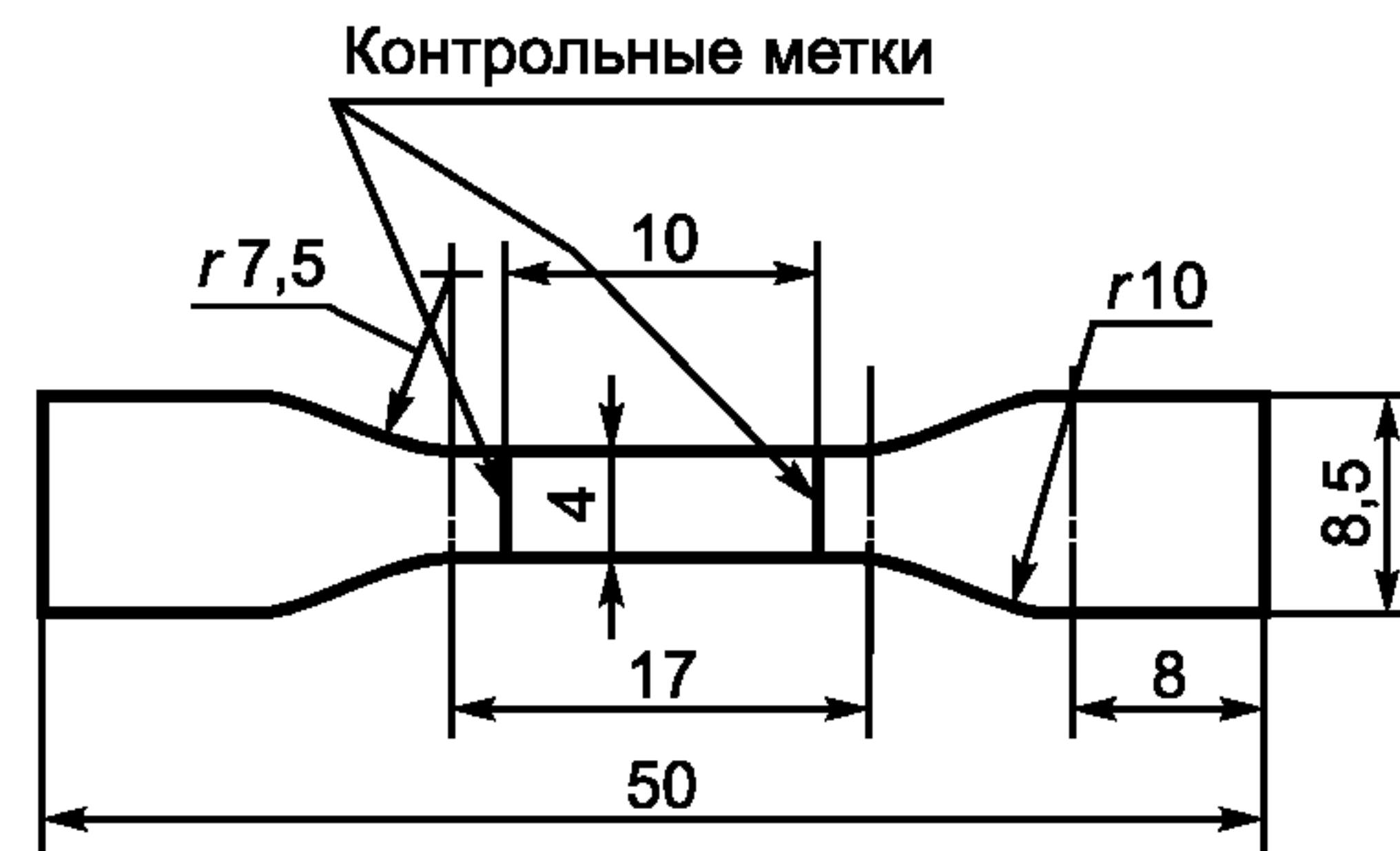
Рисунок 4 — Образец в форме двусторонней лопатки небольшого размера
