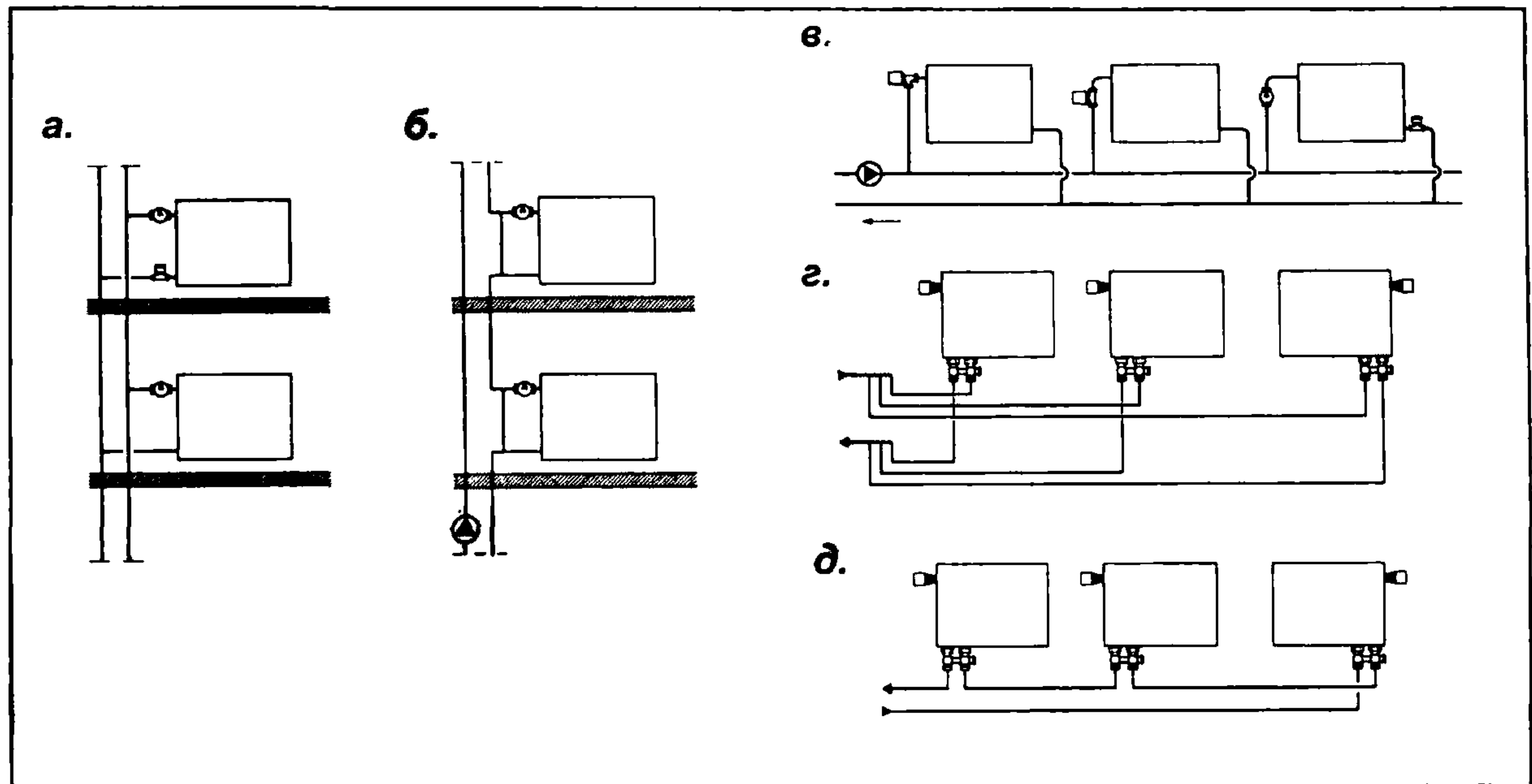
Рис. 2.1. Схемы систем водяного отопления с радиаторами «Kermi»: вертикальные двухтрубная (а) и однетрубная (б) с радиаторами «Profil-Kompakt»; горизонтальная двухтрубная (в) с радиаторами «Profil-Kompakt»; горизонтальные двухтрубная (г) и однетрубная (д) с радиаторами «Profil-Ventil»
