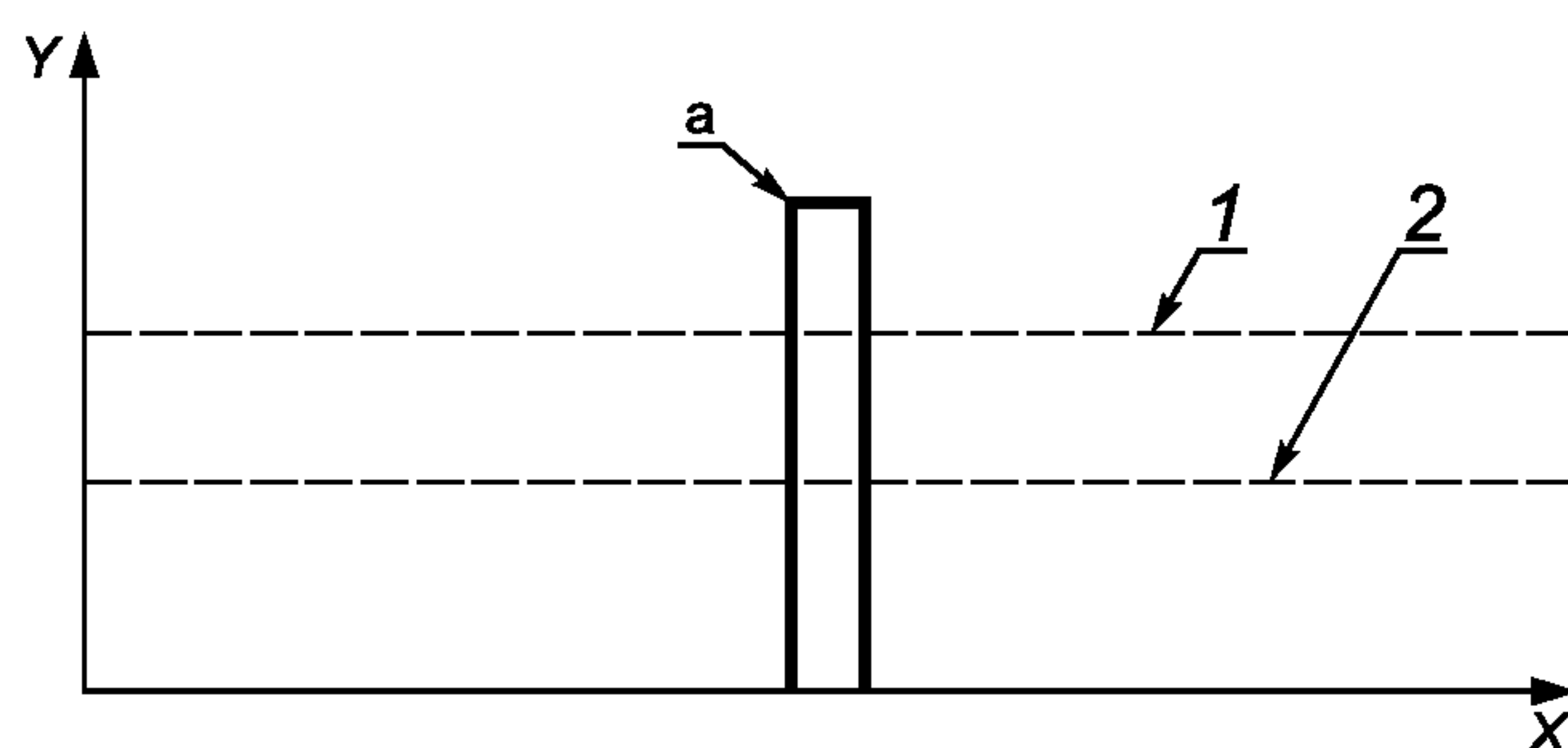
Рисунок 1 — «Плохой» сигнал датчика фазы
