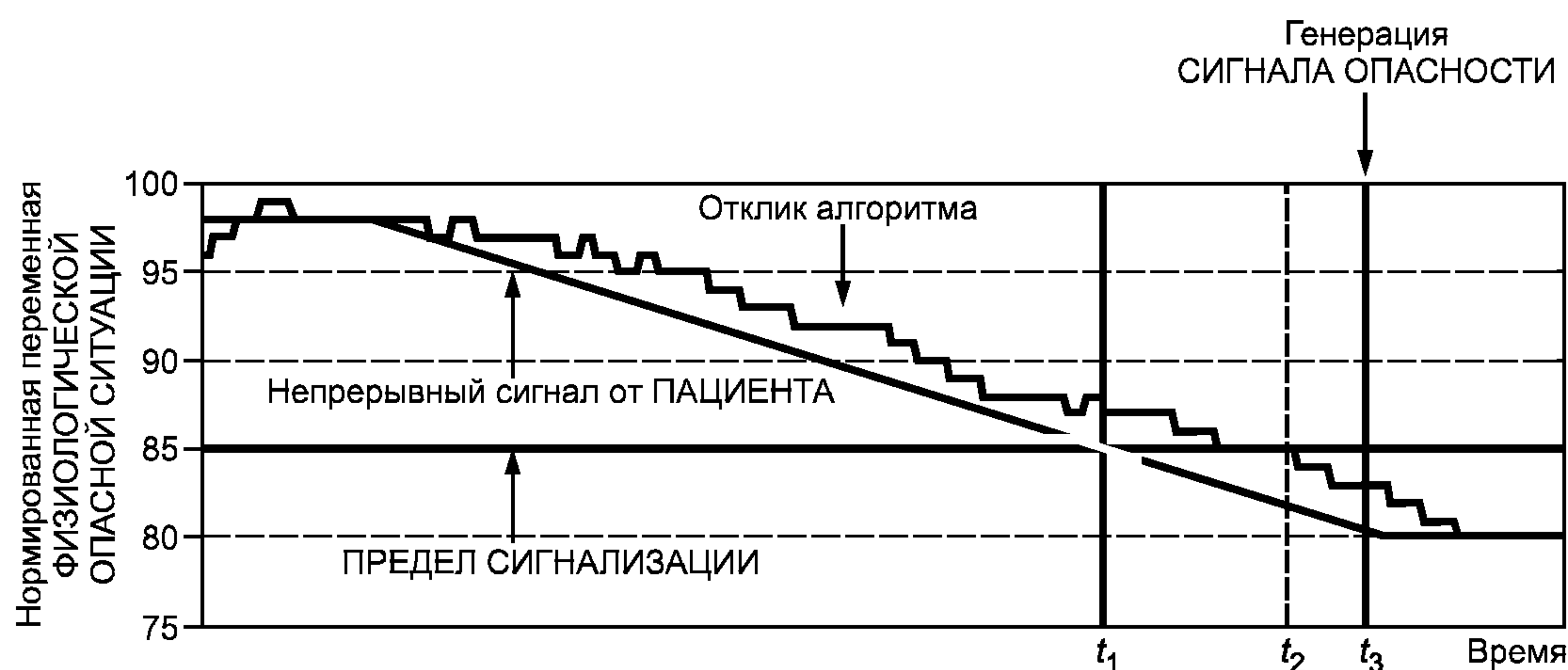
Рисунок ААА.1 — Графическое изображение элементов задержки СИСТЕМЫ СИГНАЛИЗАЦИИ
