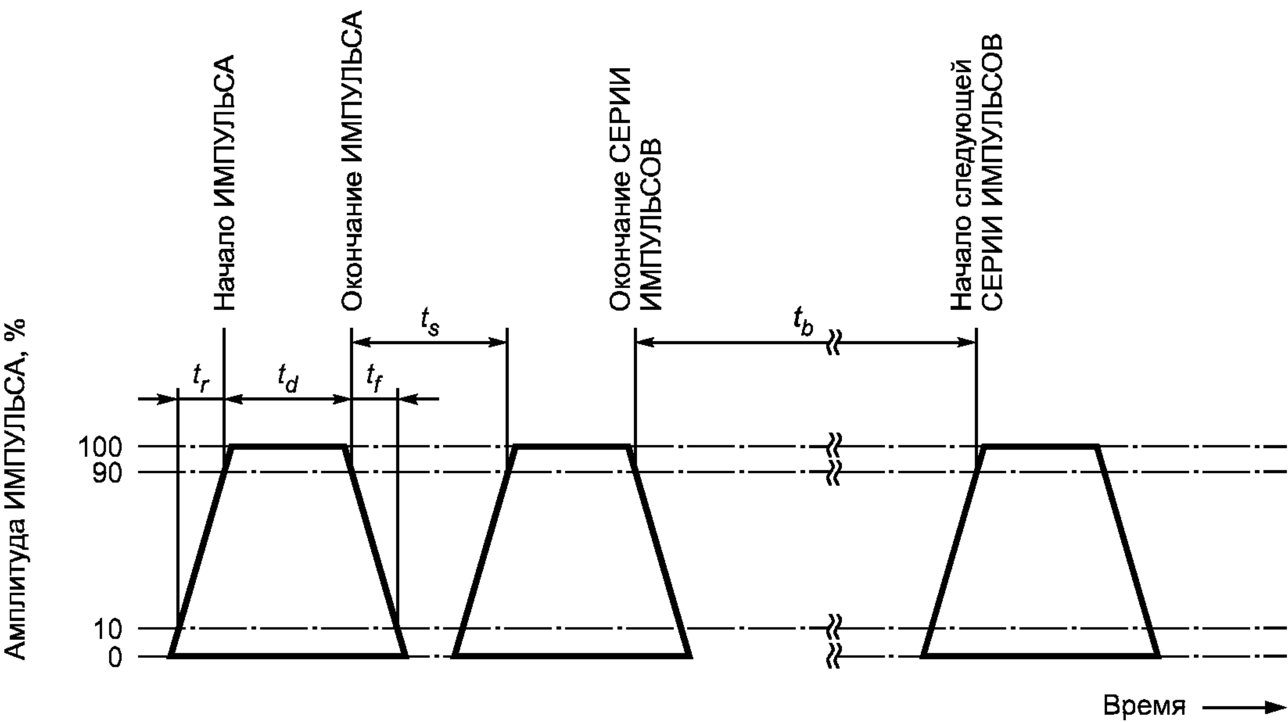
Рисунок 201 — Пояснение временных характеристик звуковых СИГНАЛОВ ОПАСНОСТИ
