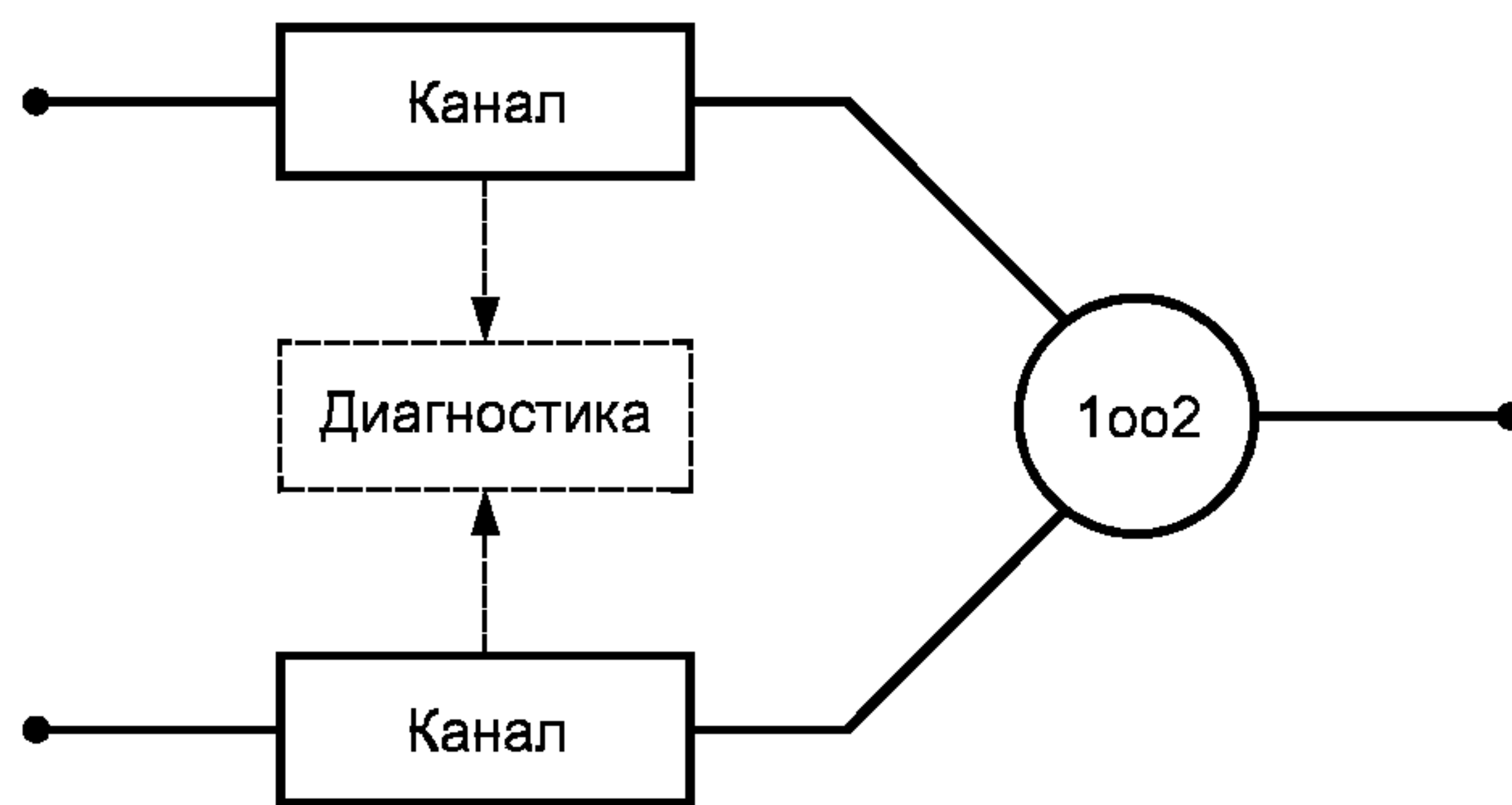
Рисунок В.5 — Структурная схема архитектуры 1oo2
