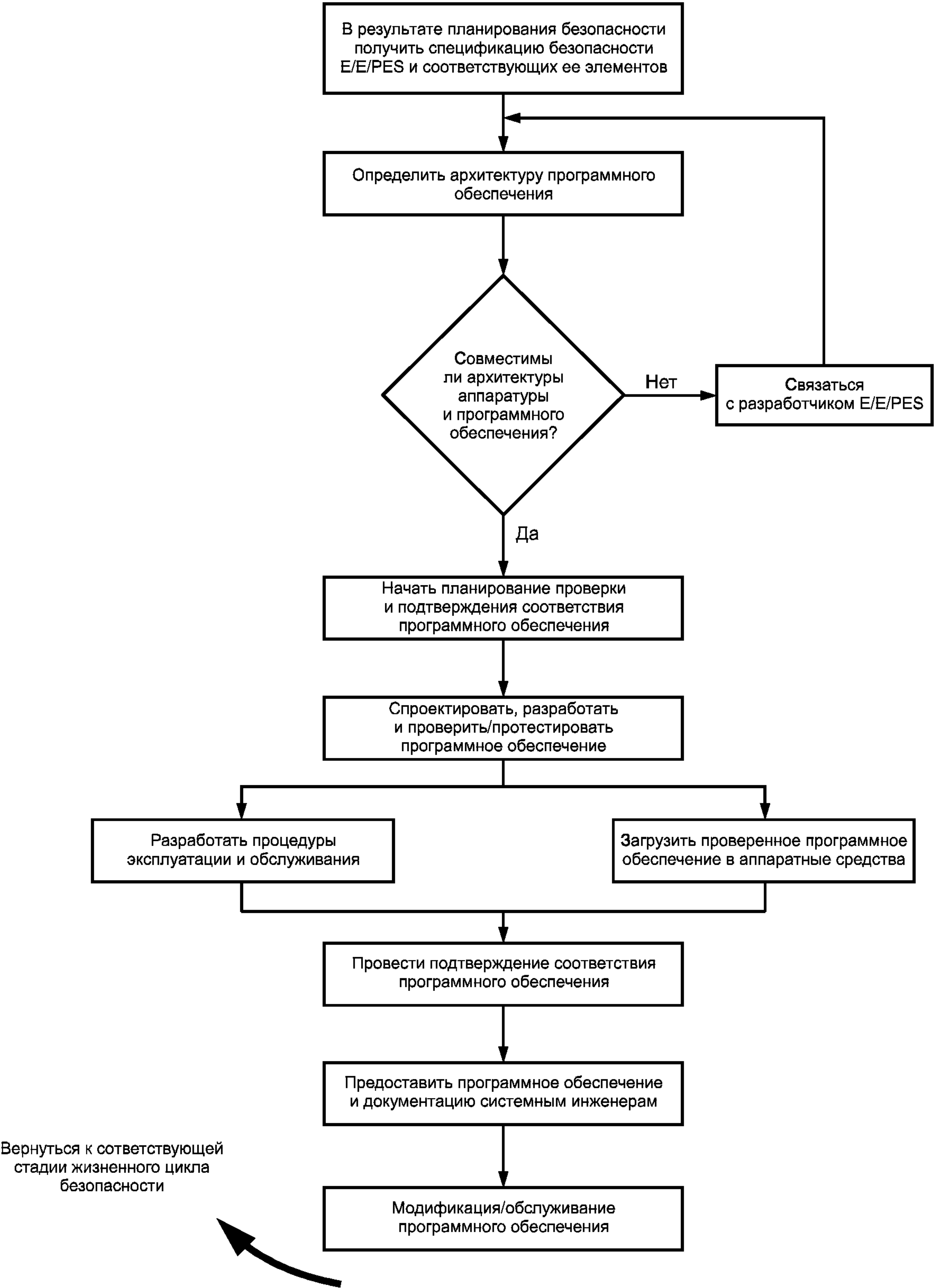
Рисунок А.3 — Функциональные этапы применения МЭК 61508-3
