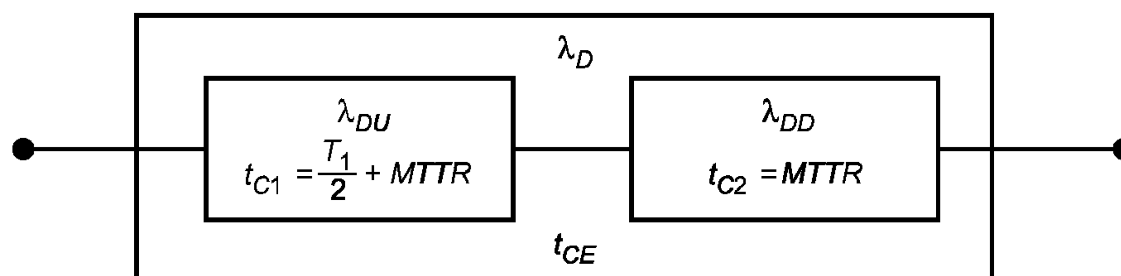
Рисунок В.4 — Схема расчета надежности архитектуры 1oo1
