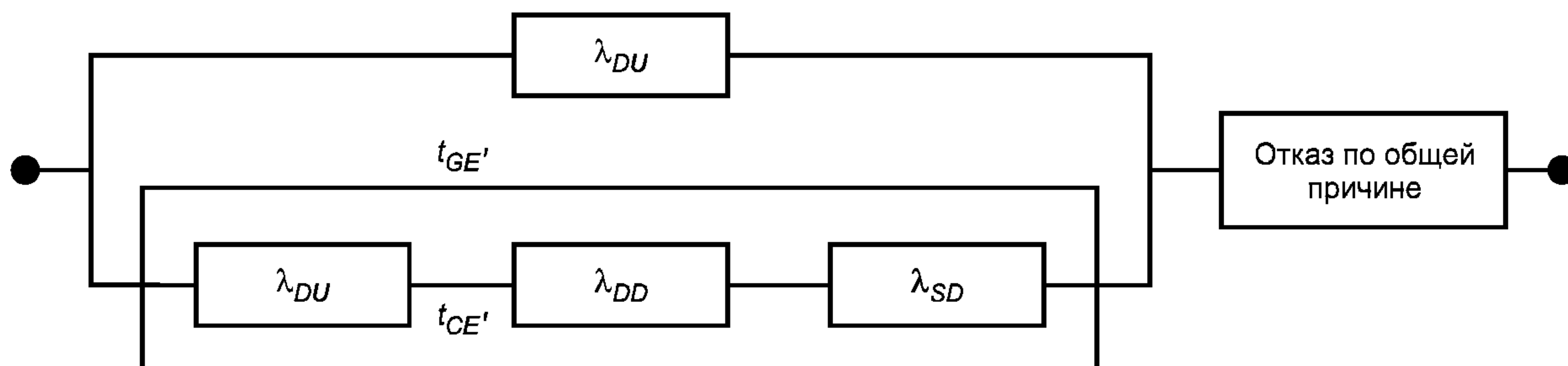
Рисунок В.10 — Схема расчета надежности архитектуры 1oo2D
