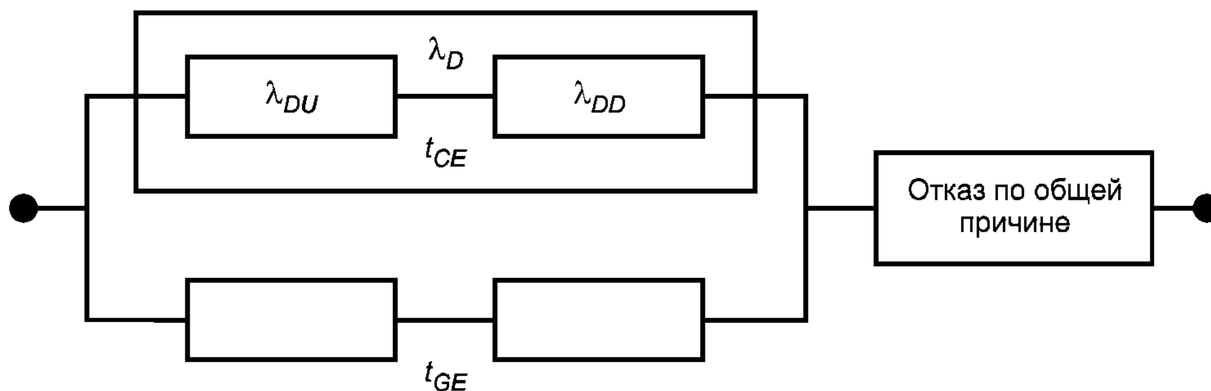
Рисунок В.6 — Схема расчета надежности архитектуры 1oo2
