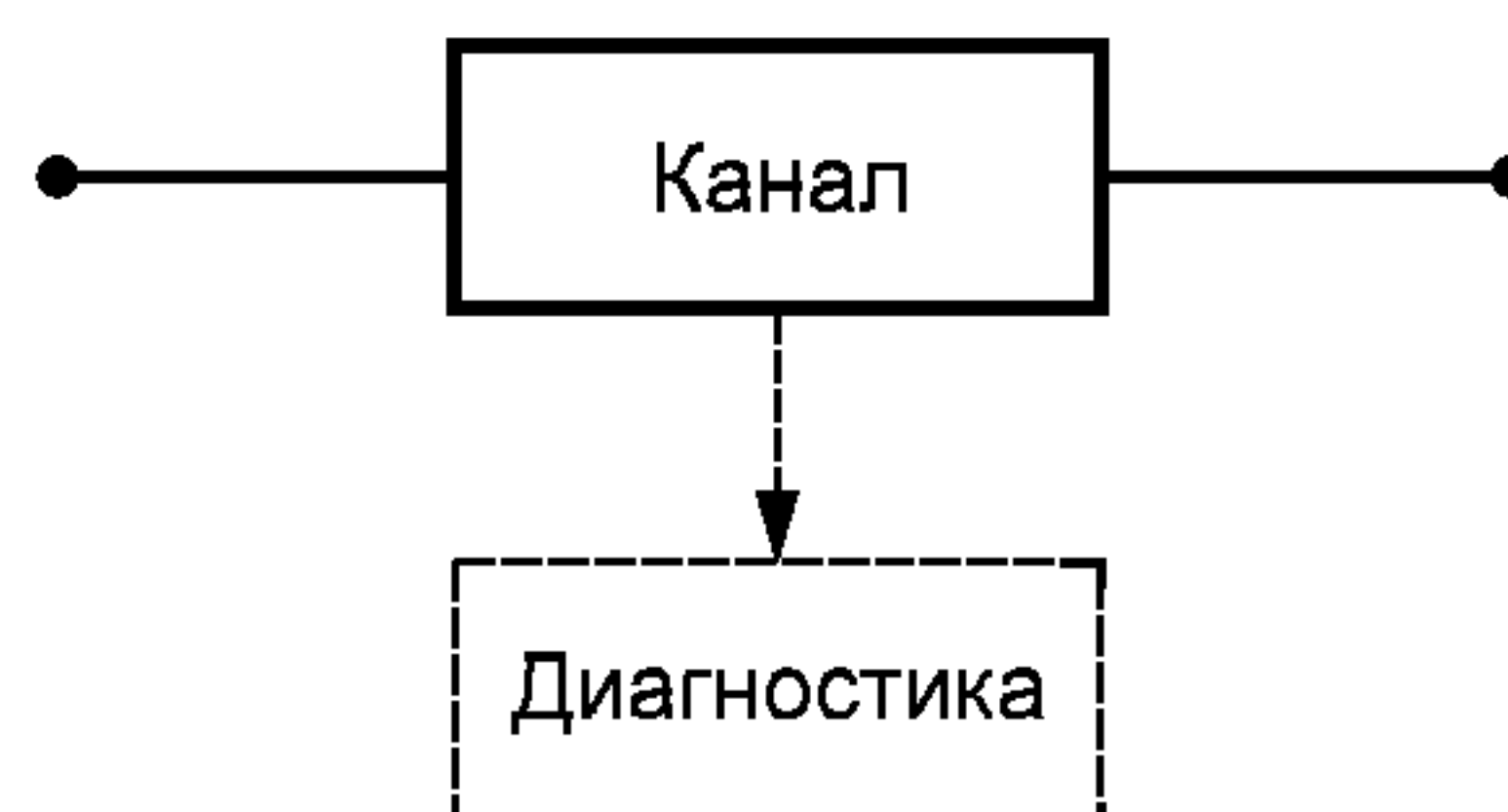
Рисунок В.3 — Структурная схема архитектуры 1oo1
