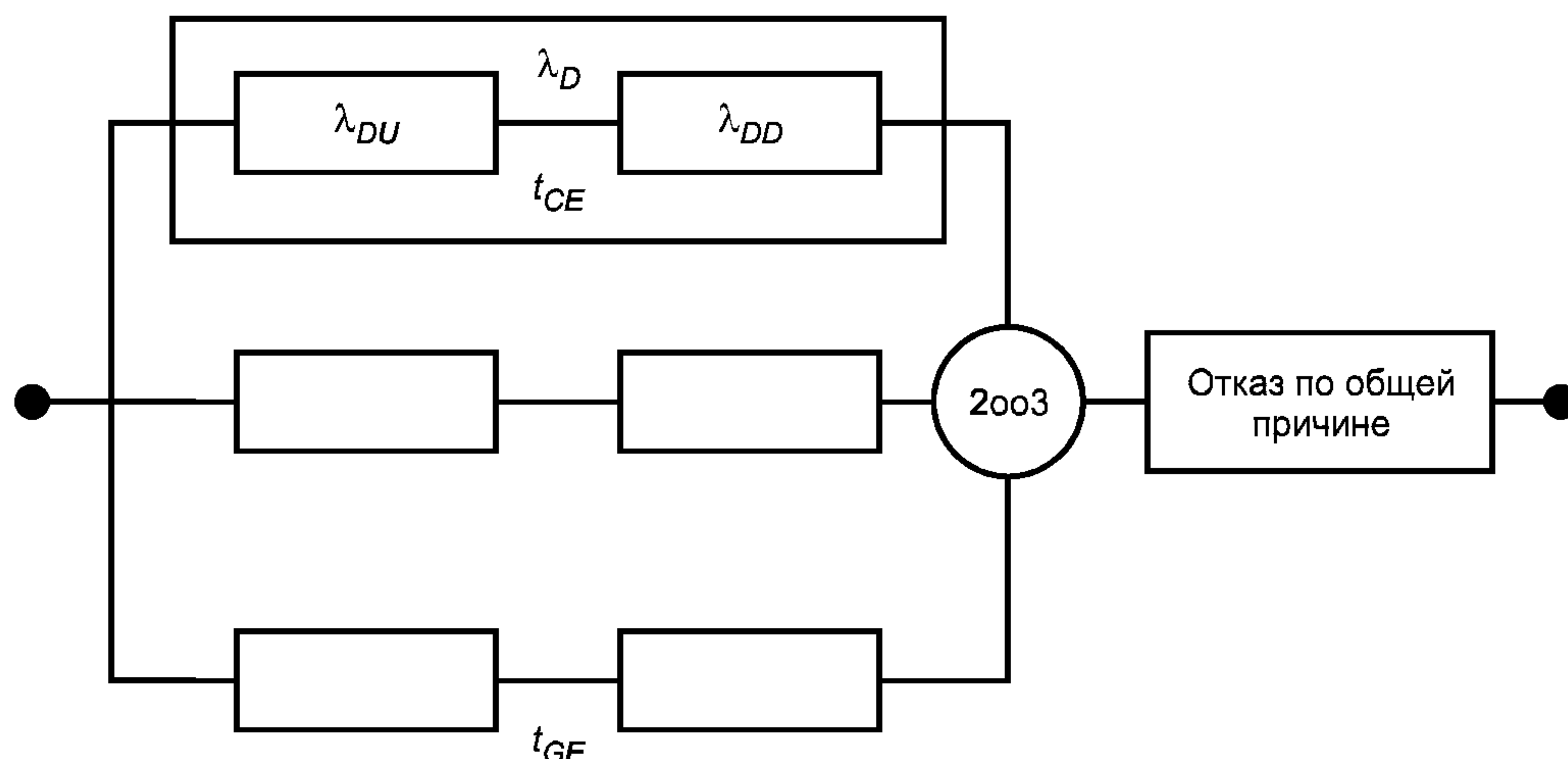
Рисунок В.12 — Схема расчета надежности архитектуры 2oo3
