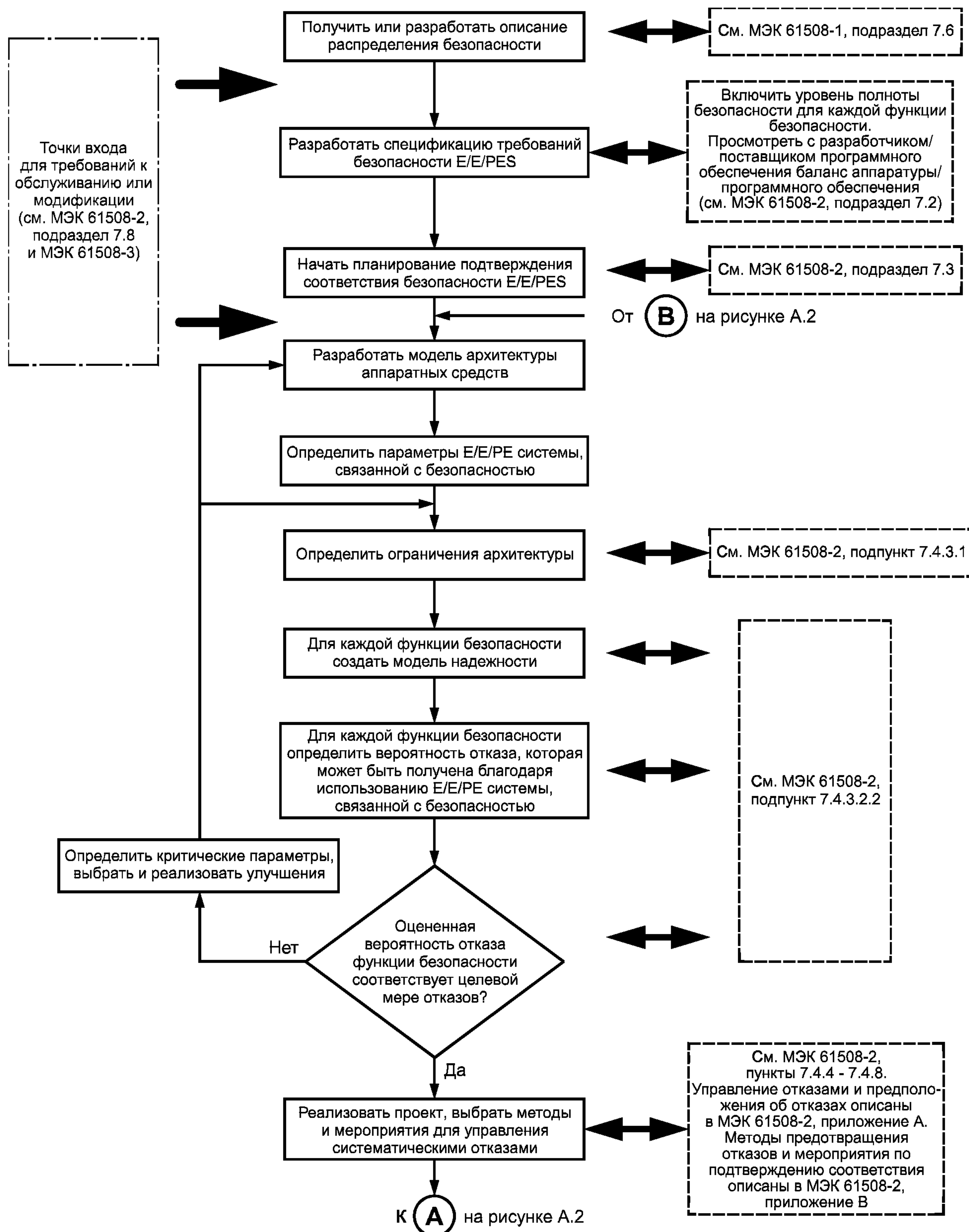
Рисунок А.1 — Функциональные этапы применения МЭК 61508-2
