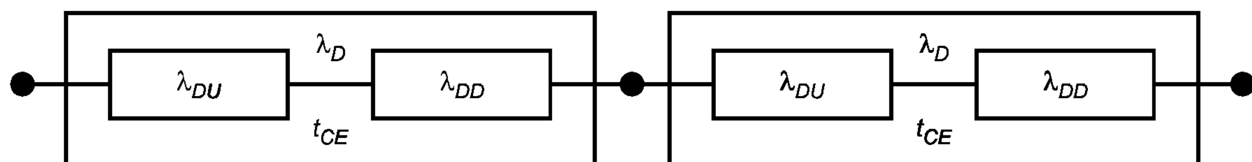
Рисунок В.8 — Схема расчета надежности архитектуры 2oo2
