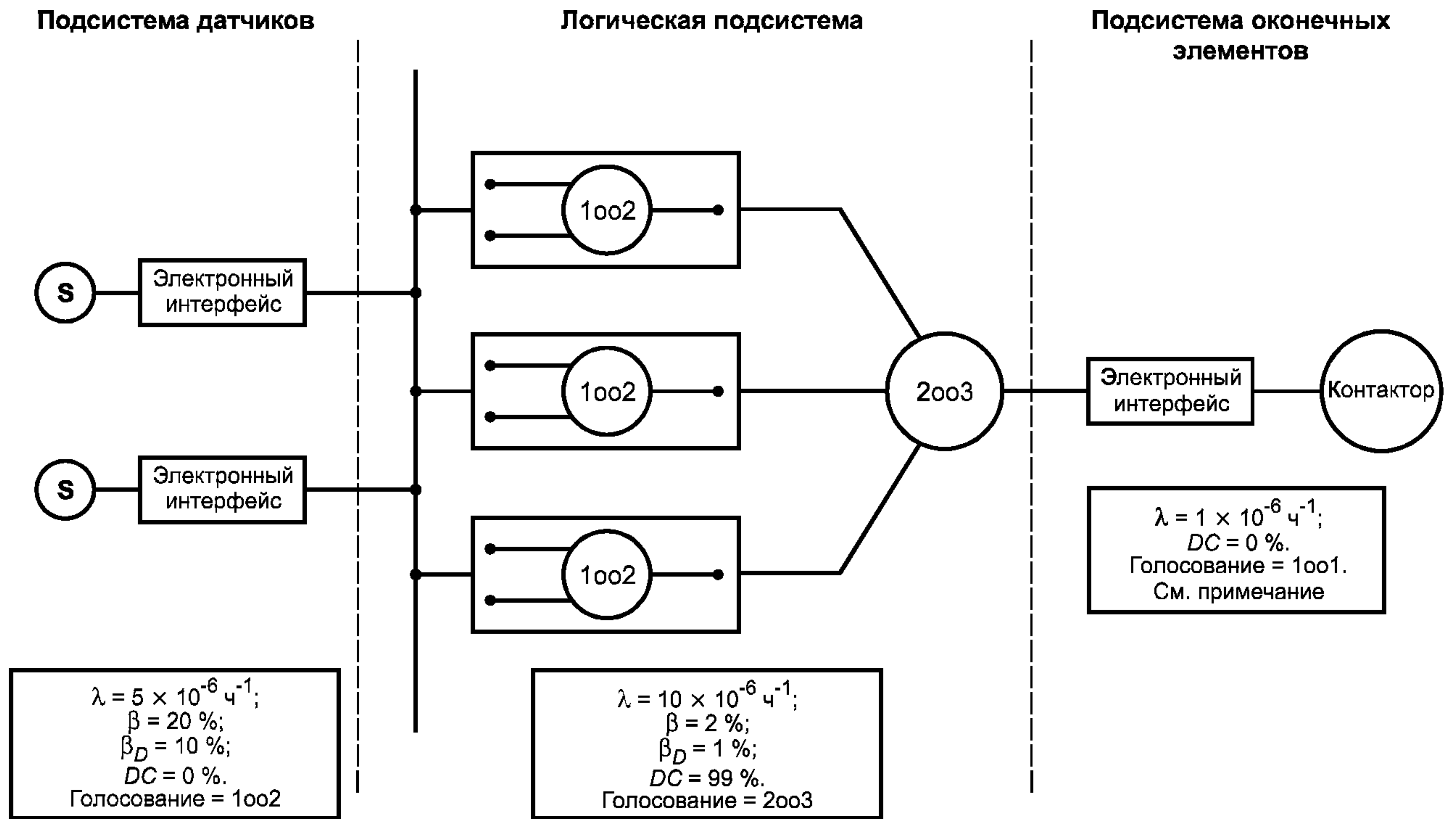
Рисунок В.14 — Архитектура системы рассматриваемого примера для режима высокой интенсивности запросов или непрерывного режима
