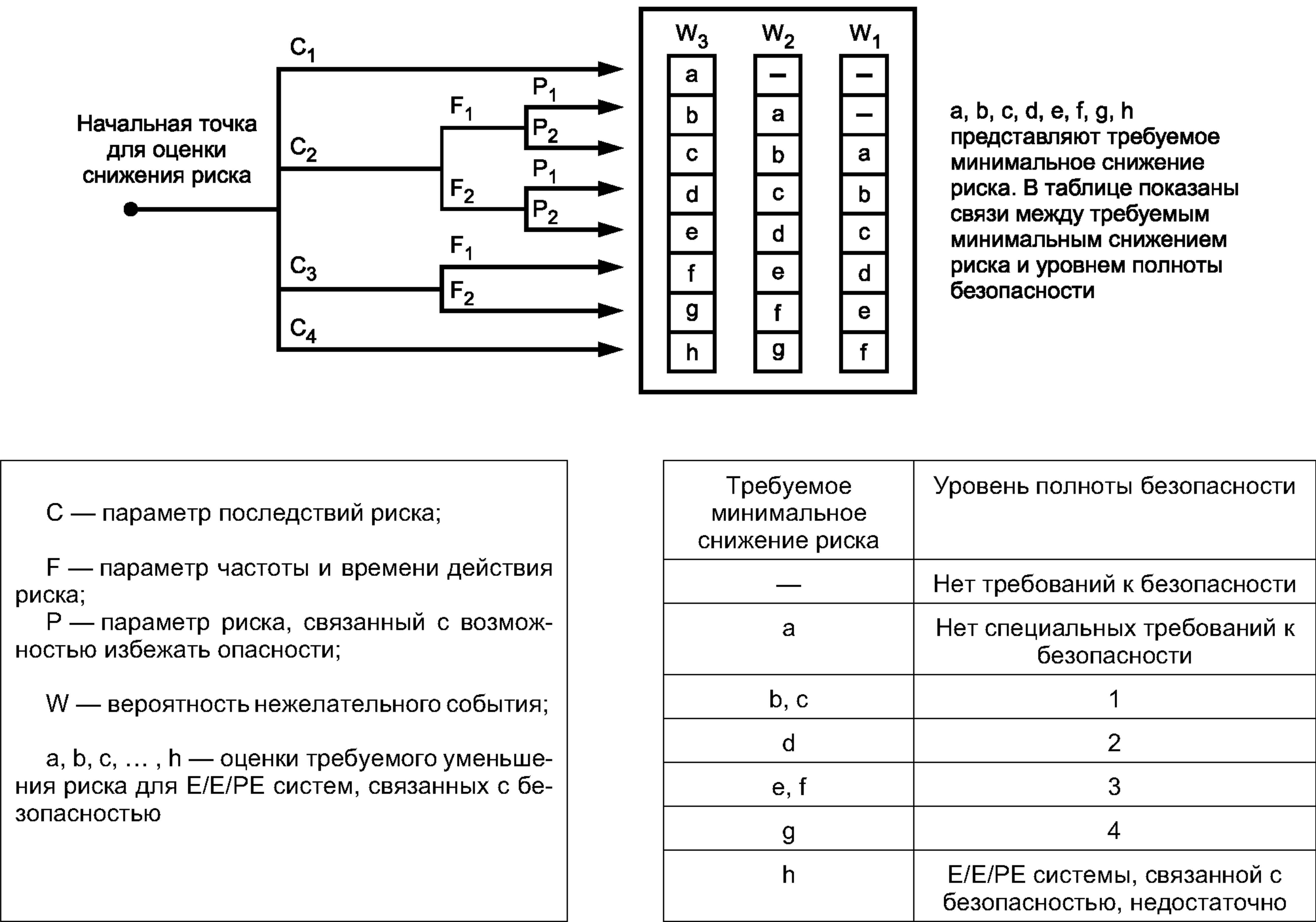
Рисунок D.2 — Граф риска: пример (показывает только общие принципы)
