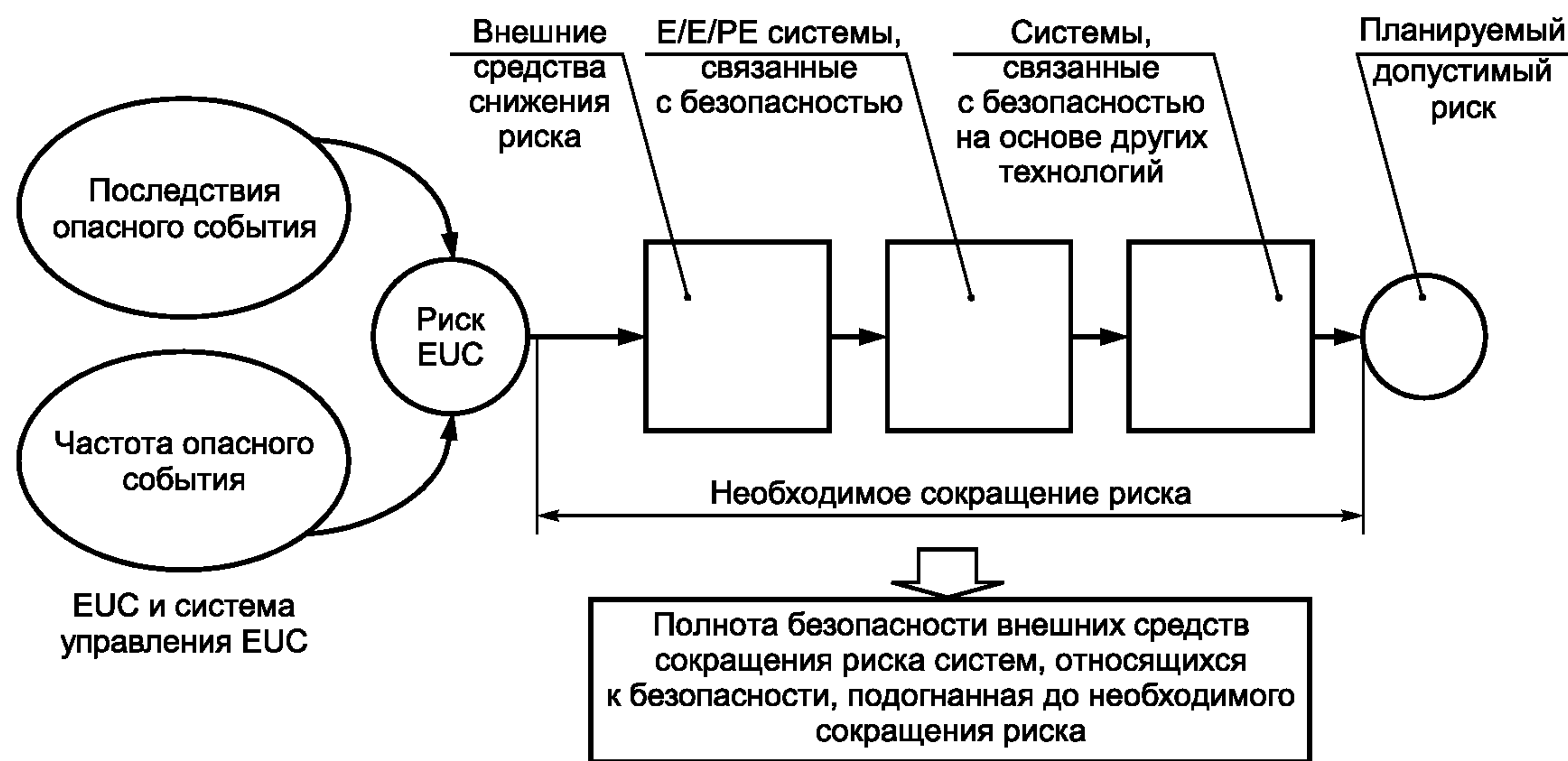
Рисунок А.2 — Понятия риска и полноты безопасности
