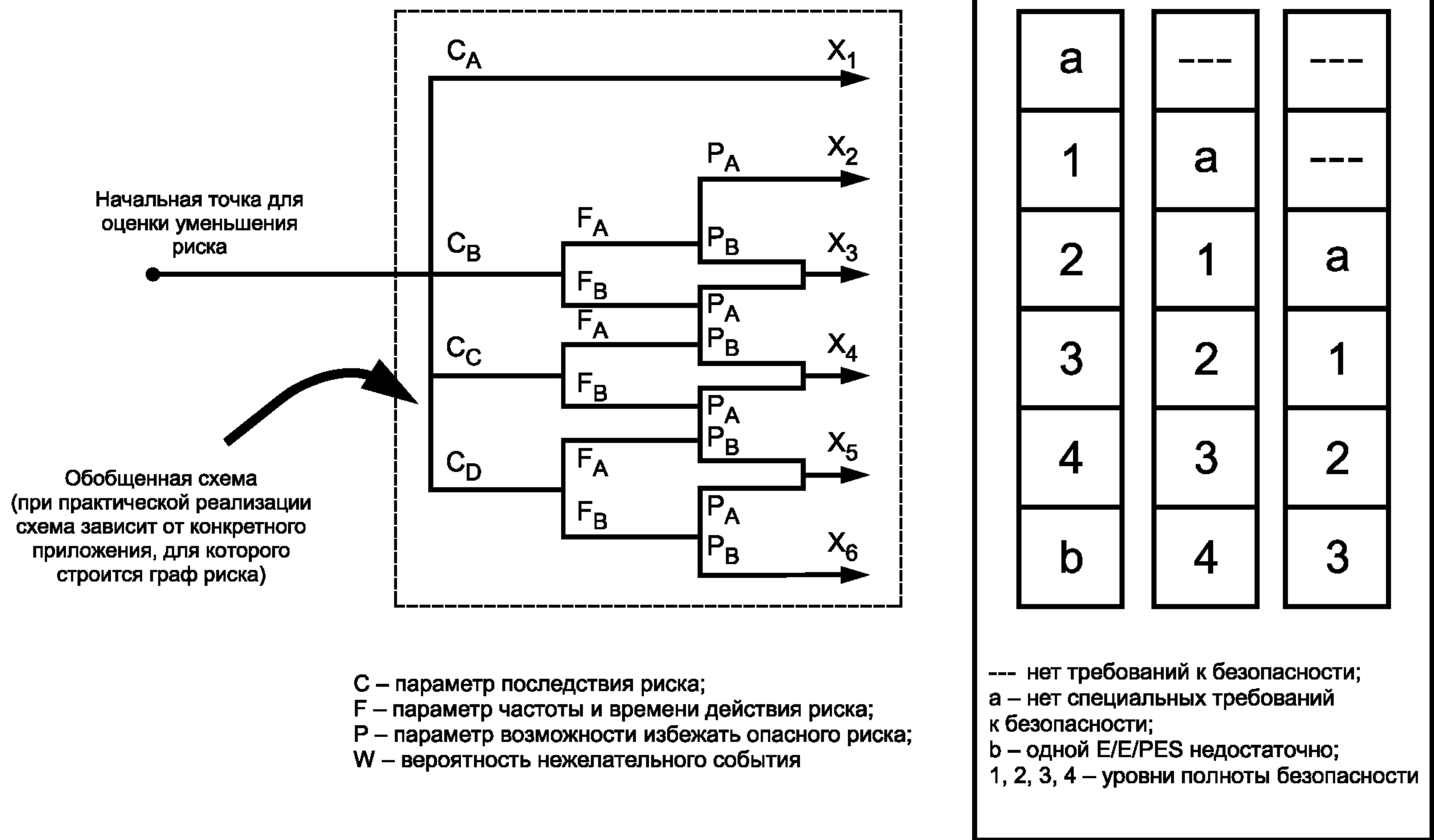
Рисунок D.1 — Граф риска: общая схема
