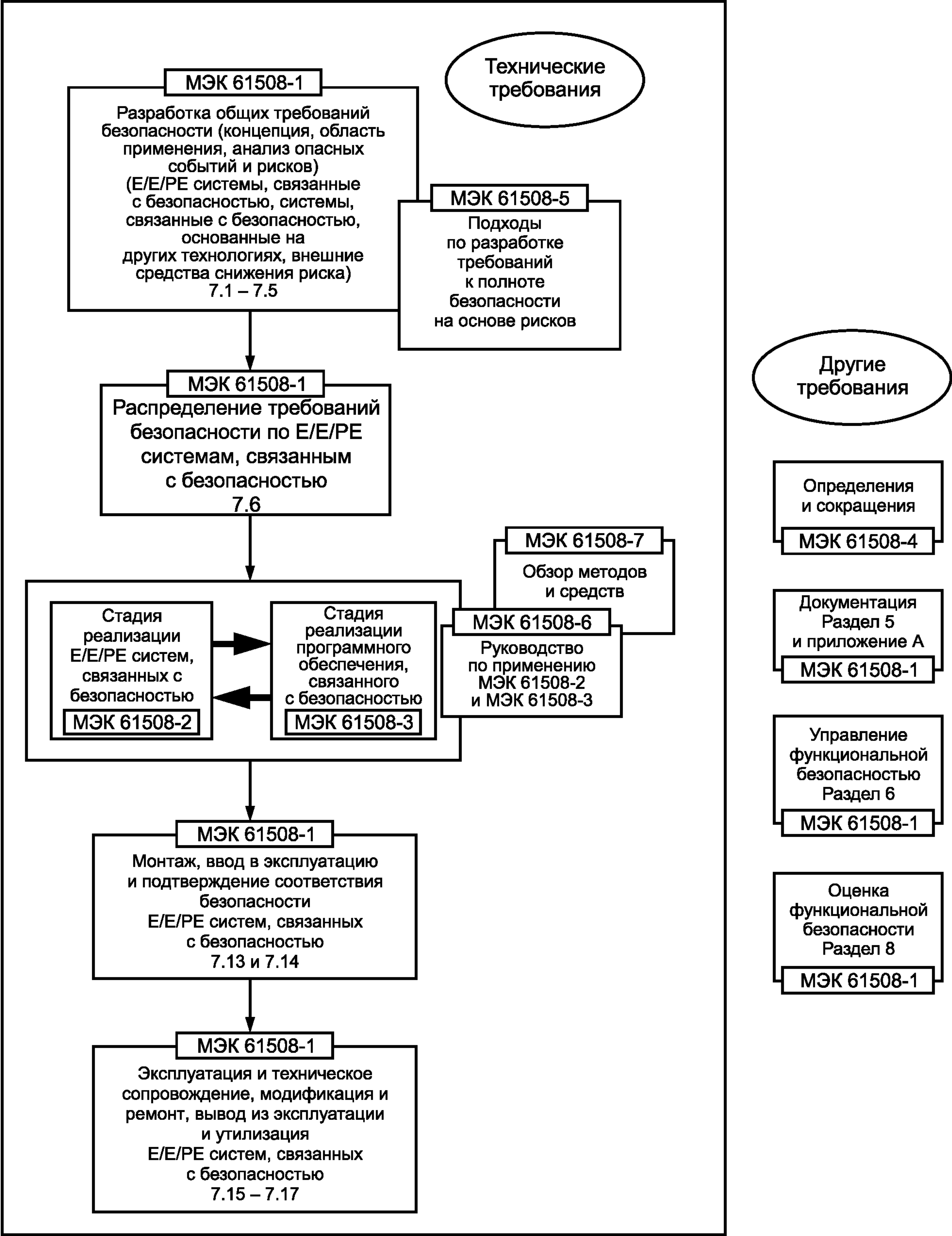
Рисунок 1 — Общая структура настоящего стандарта
