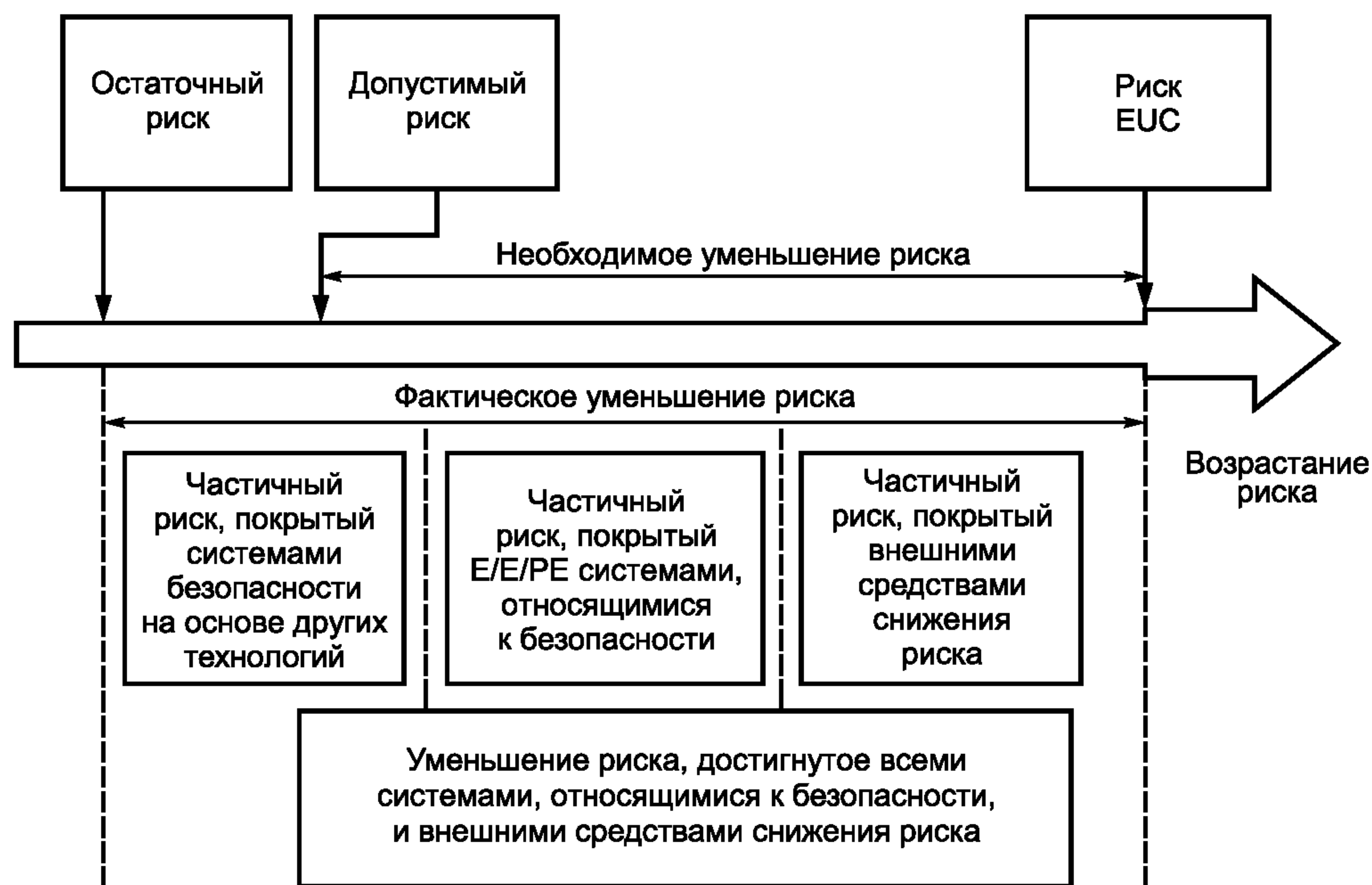
Рисунок А.1 — Уменьшение риска: основные понятия
