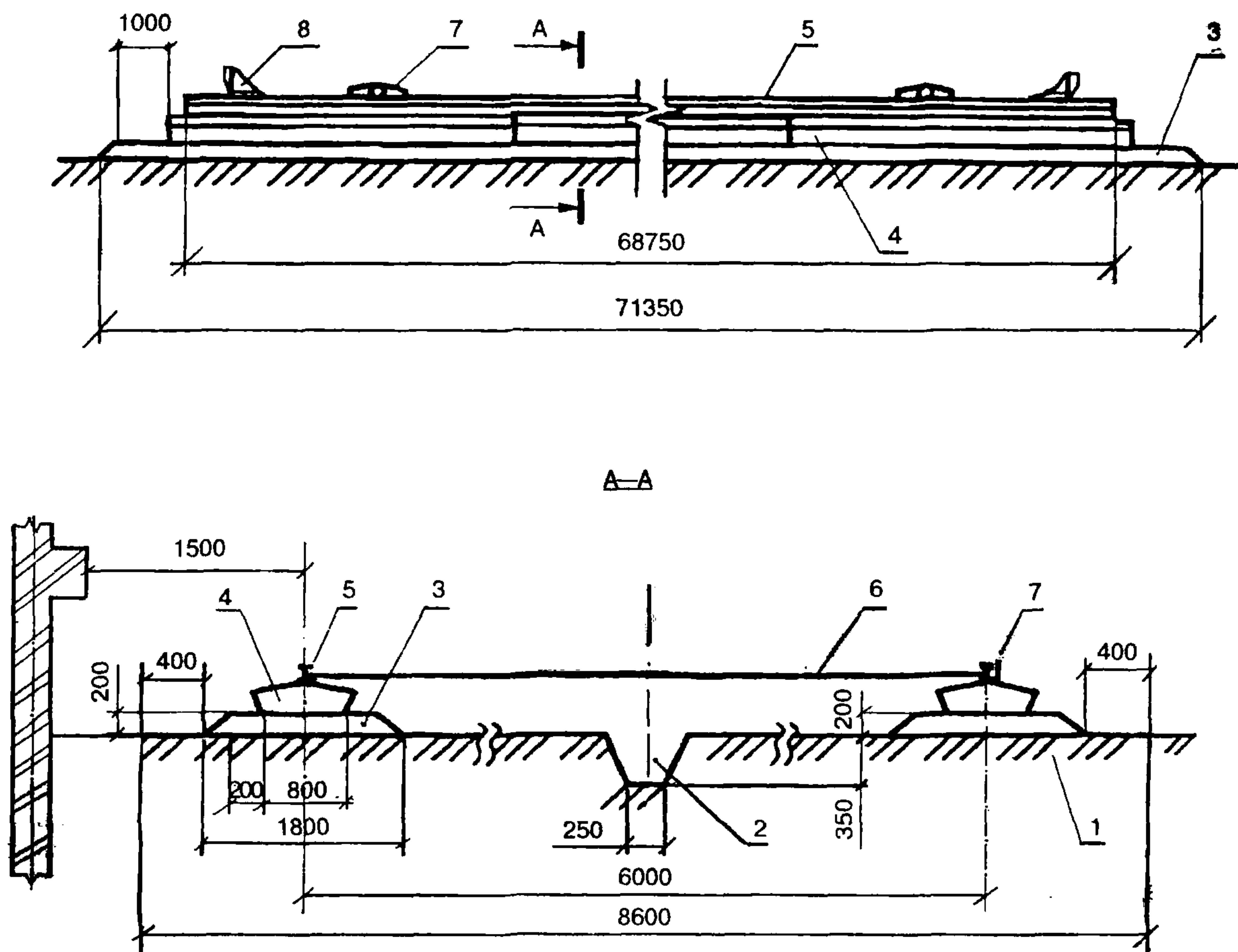
Рисунок 1 — Рельсовый путь башенного крана
