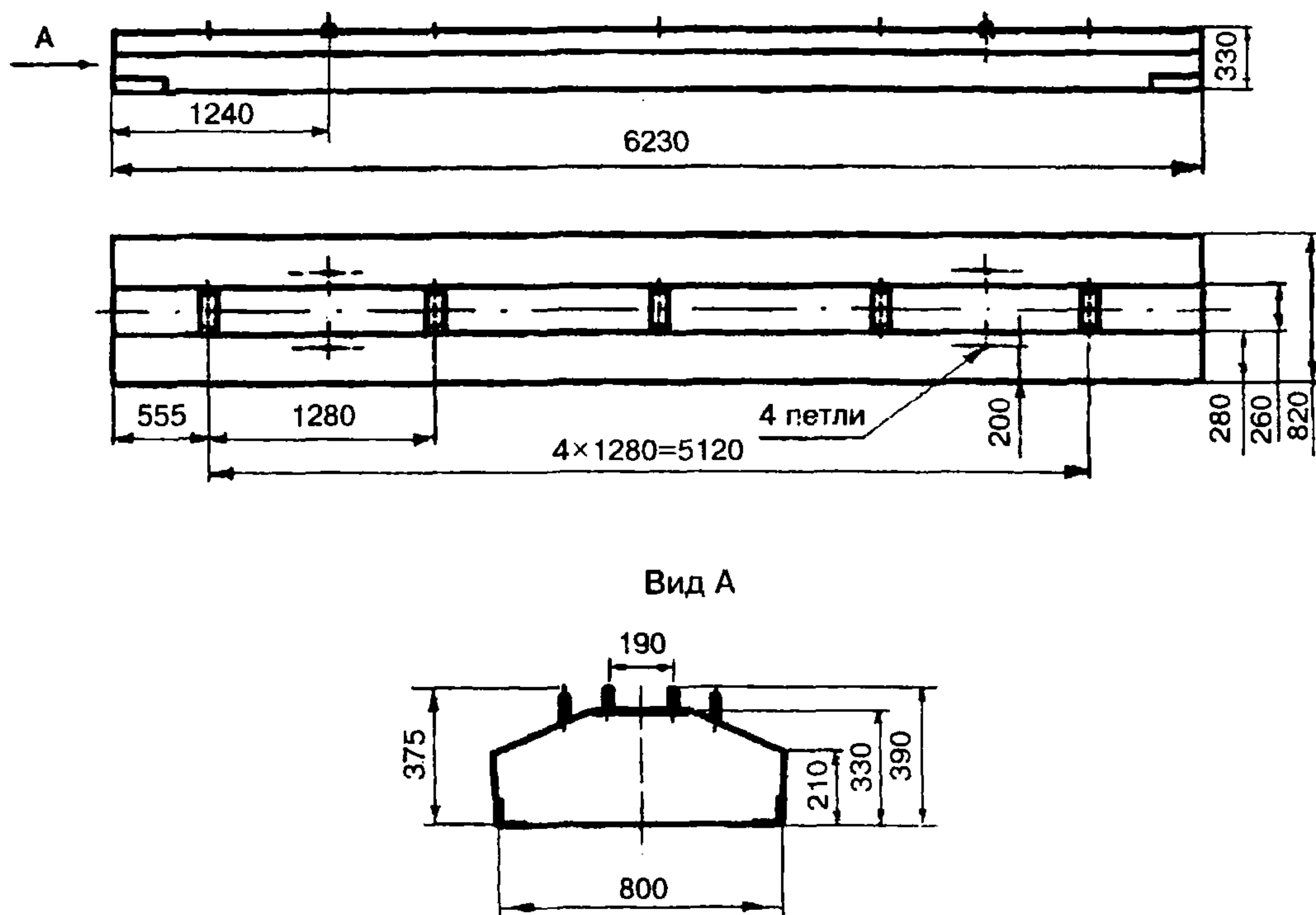
Рисунок 2 — Железобетонная балка БРП-62.8.3
