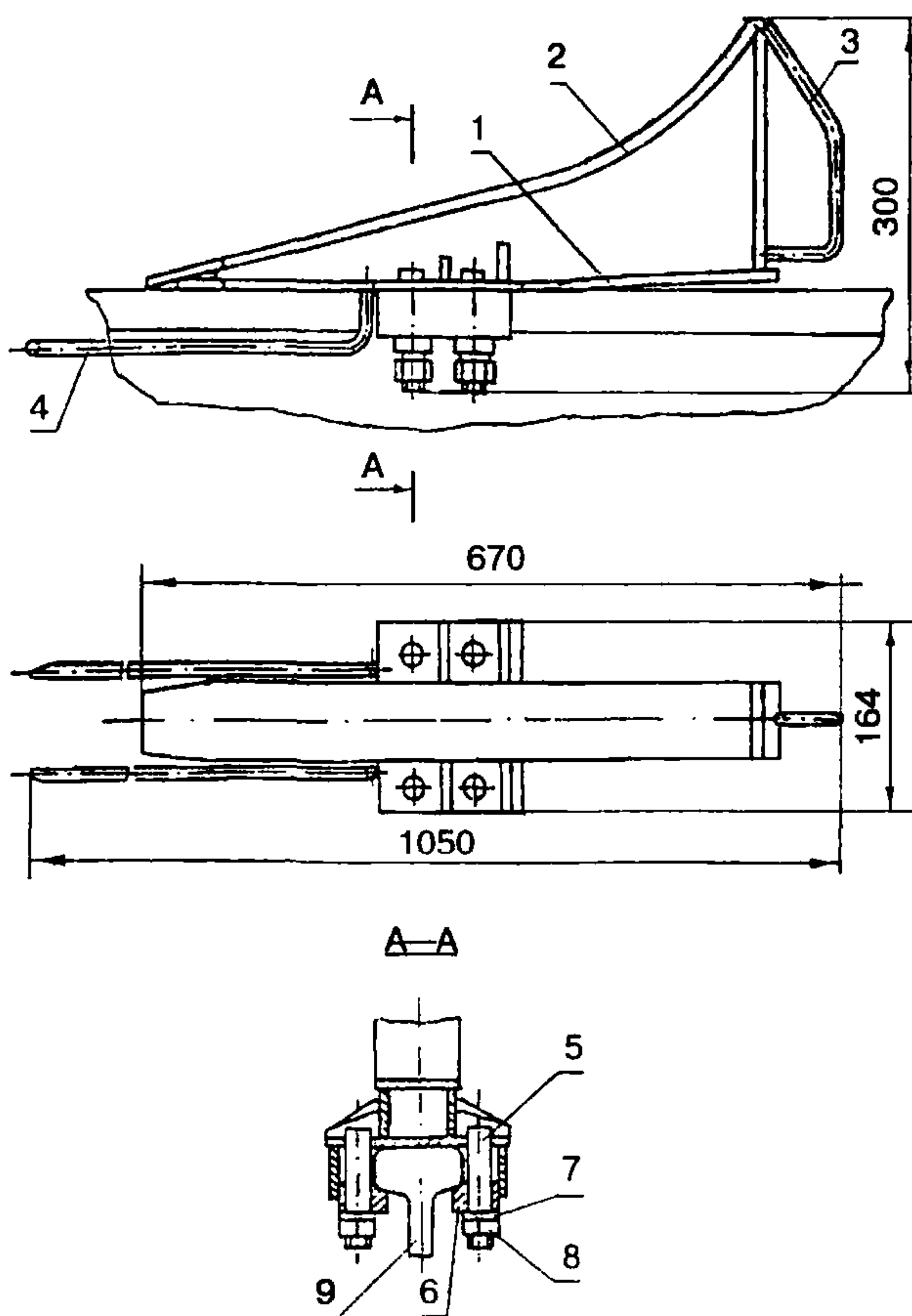
Рисунок 5 — Крепление тупикового упора к рельсу
