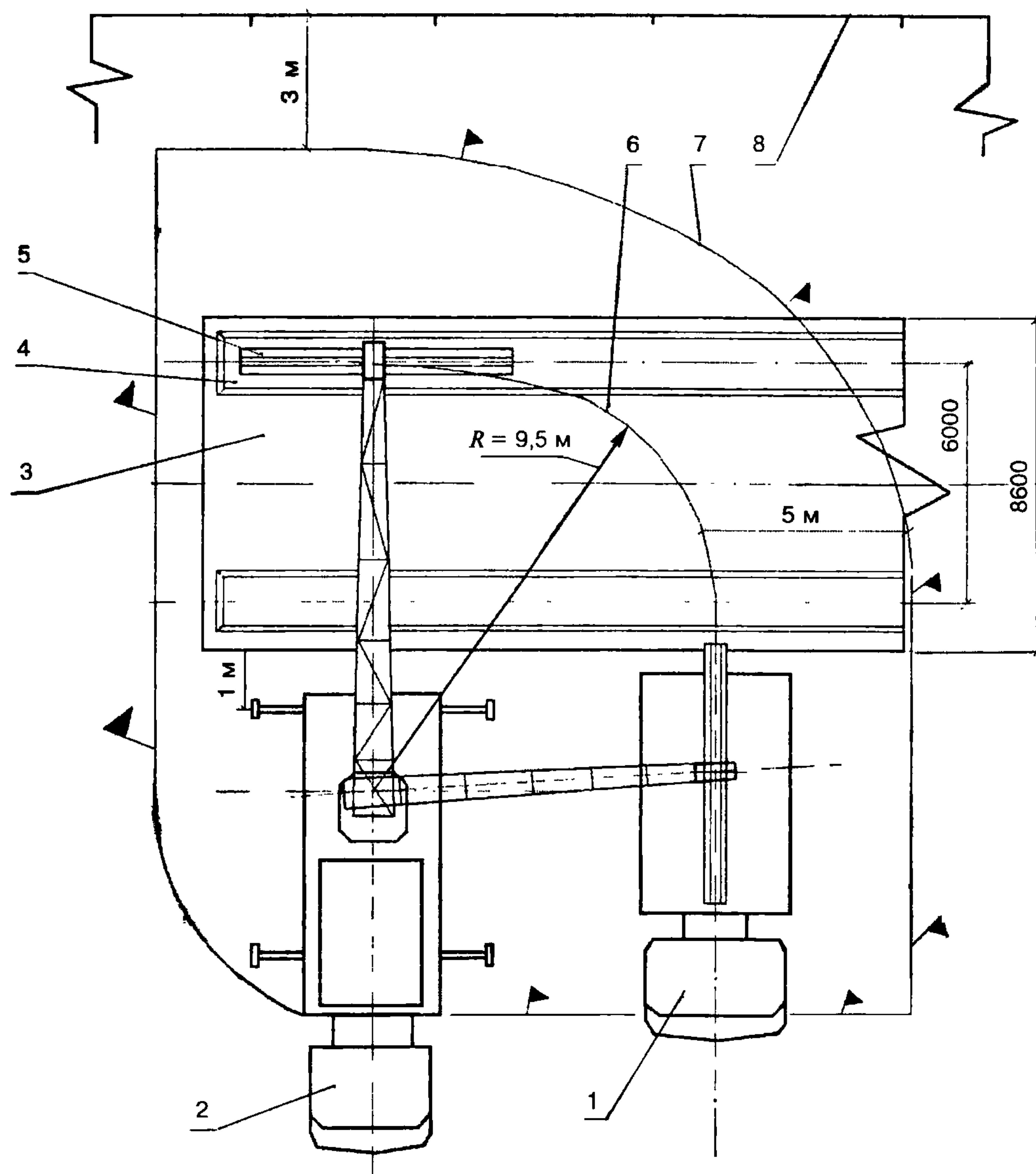
Рисунок 3 — Организация участка работ
