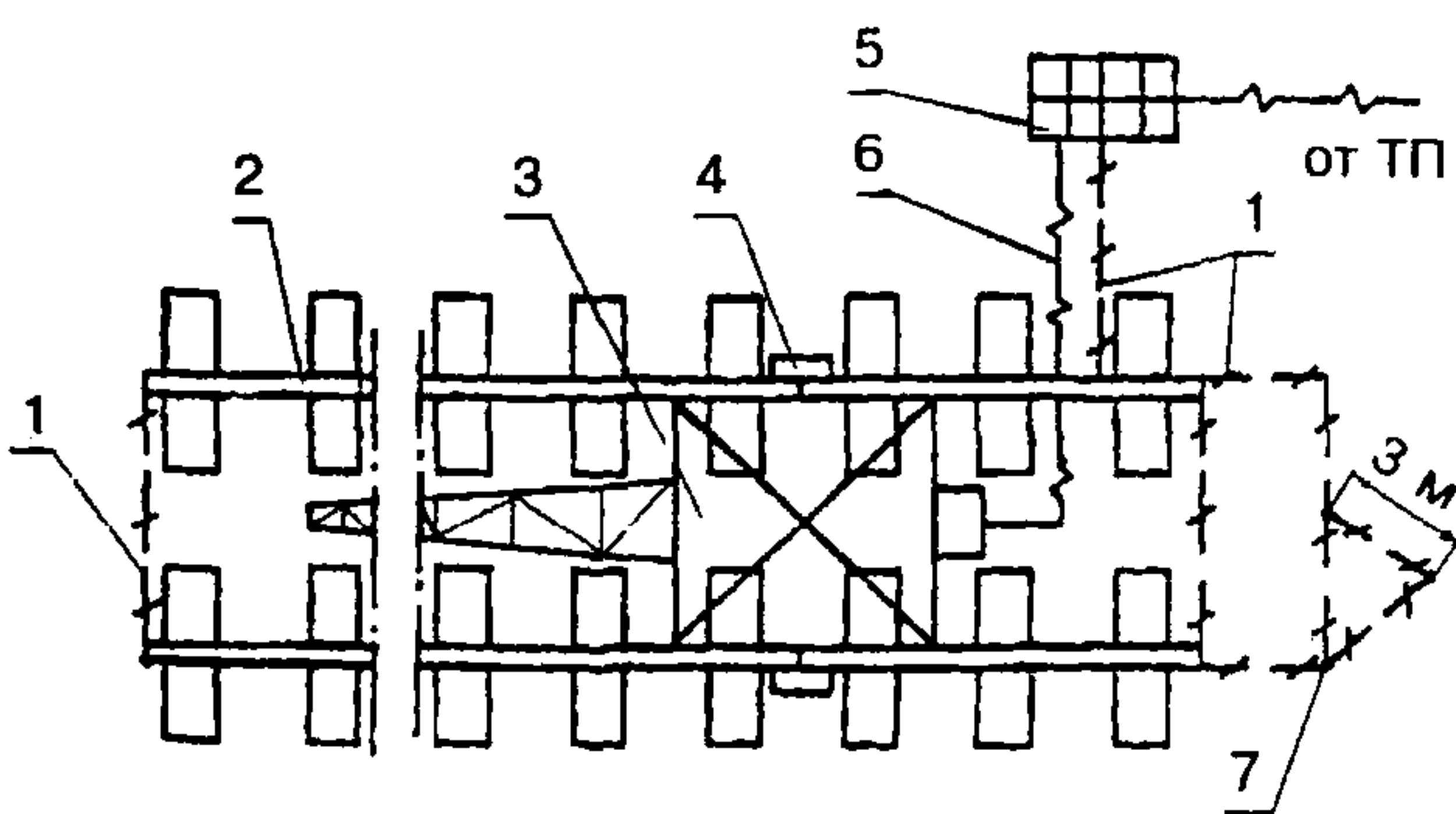
Рисунок 6 — Устройство заземления рельсового пути
