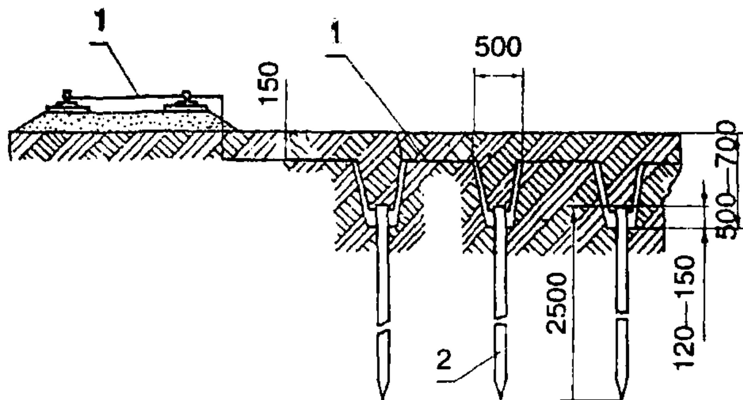
Рисунок 7 — Соединение заземлителей
