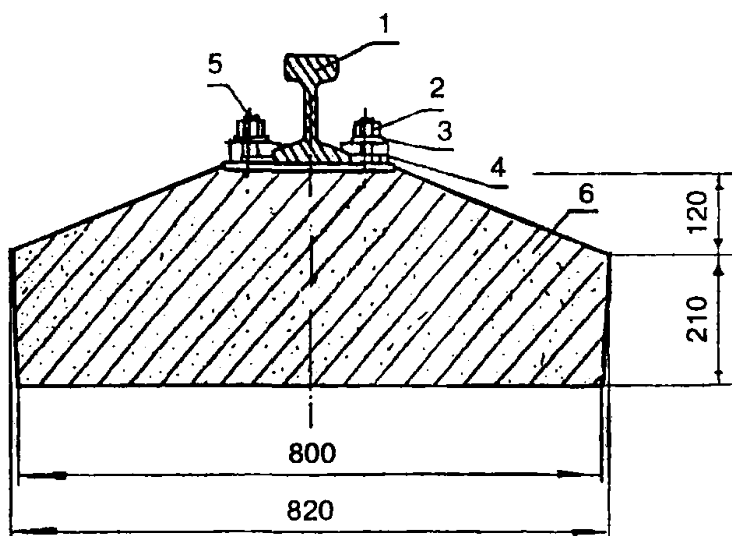
Рисунок 4 — Крепление рельса к балке
