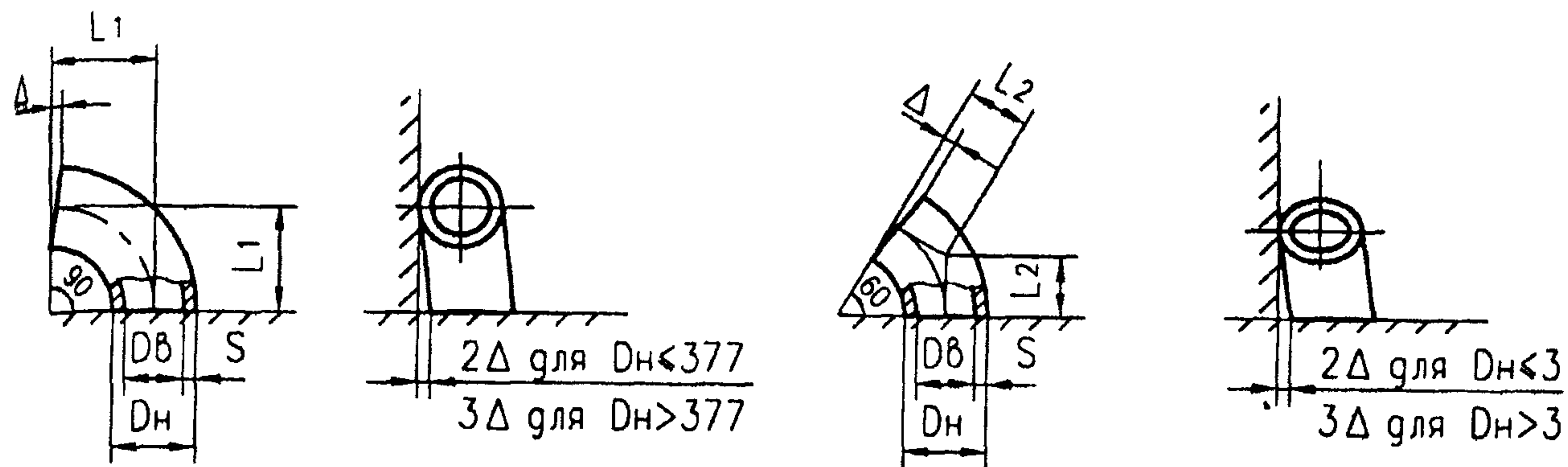
Отвод 45°
