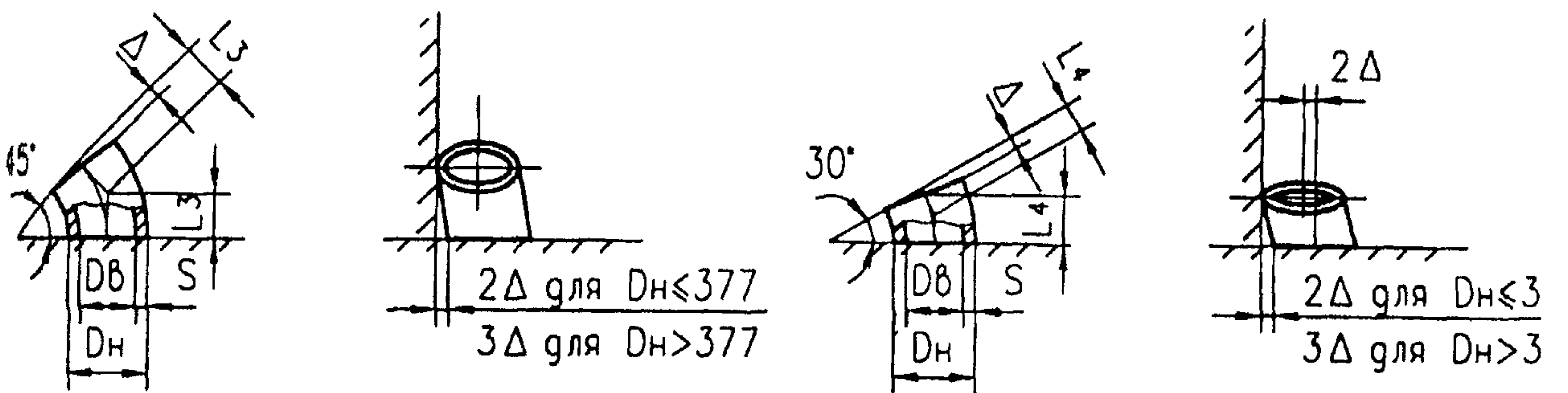
Отвод 30°
