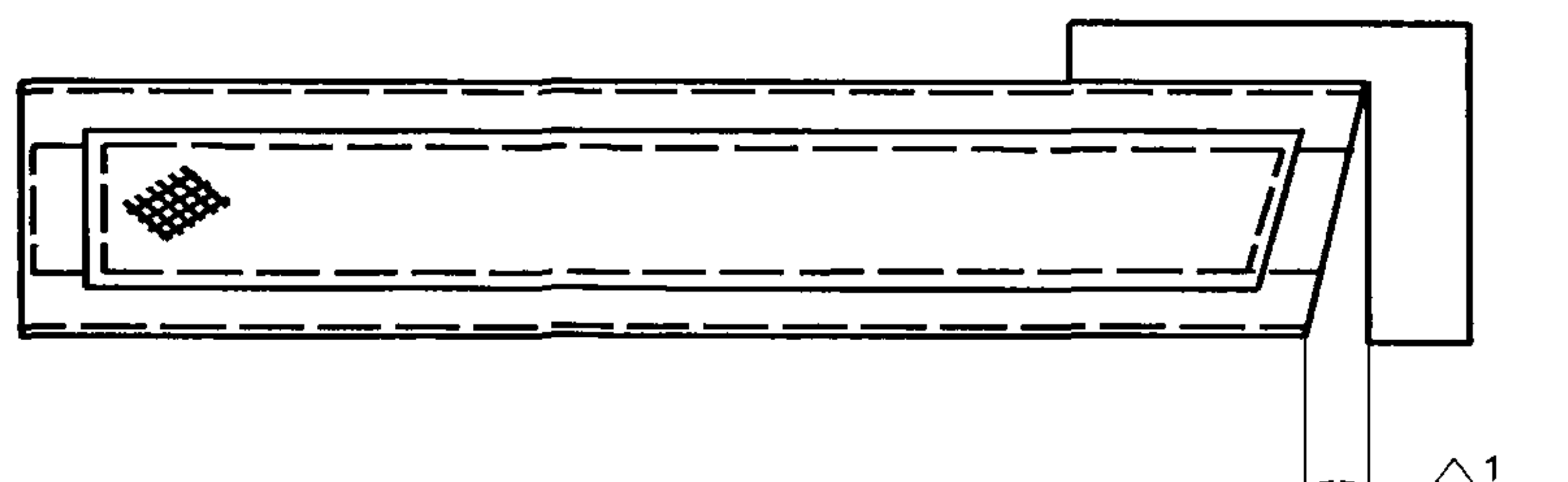
Рисунок 7 Отклонение от перпендикулярности торца рамы, площадки (помоста) относительно боковой поверхности
