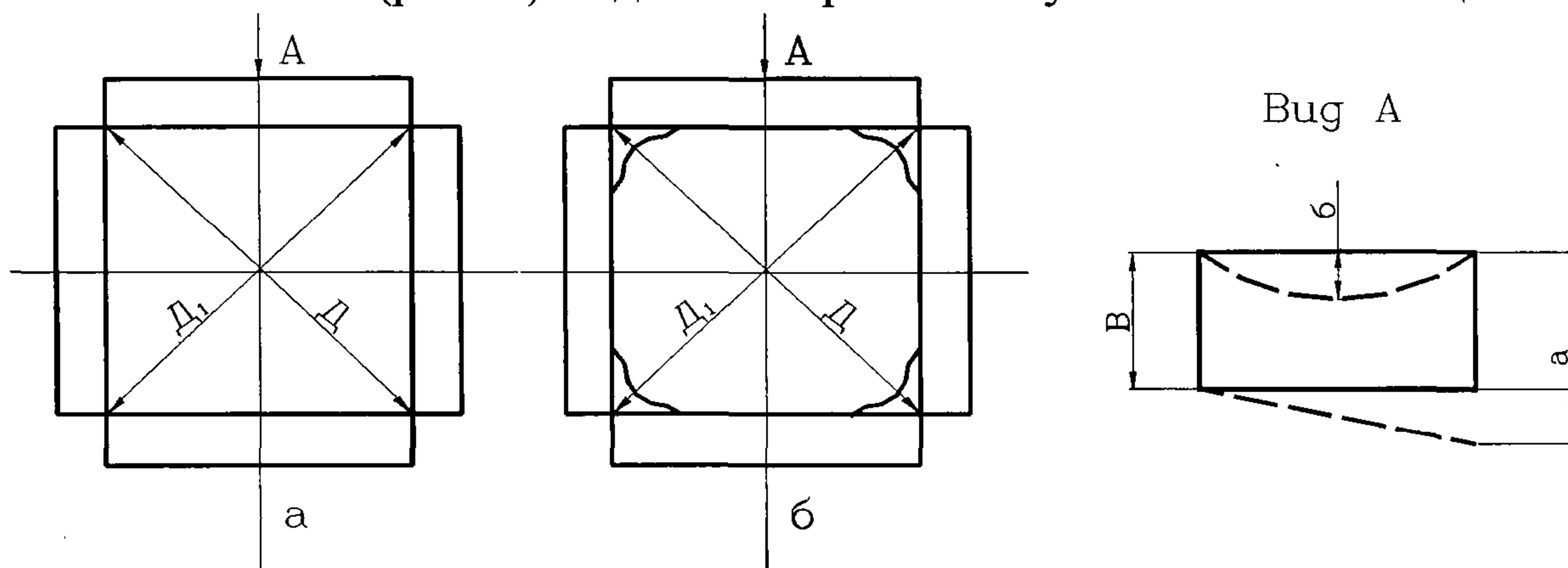
Рисунок 11 Отклонения размеров конструкций коробчатого сечения
