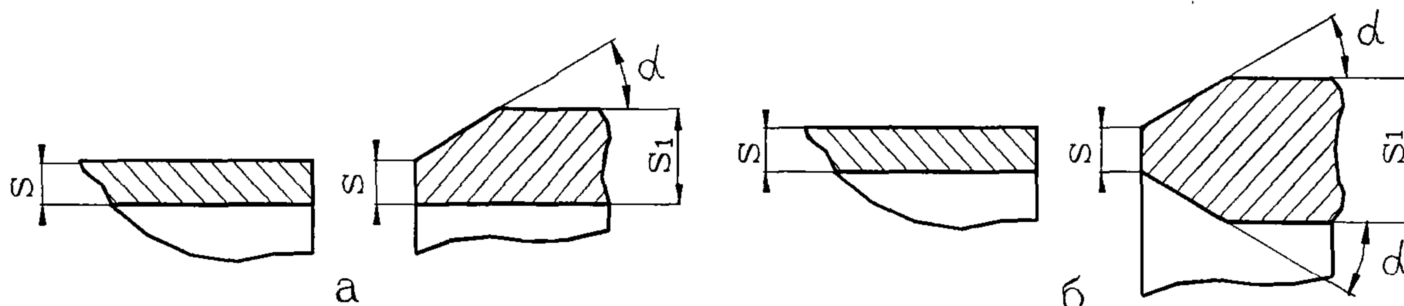
Рисунок 14 Стыковка элементов разной толщины
