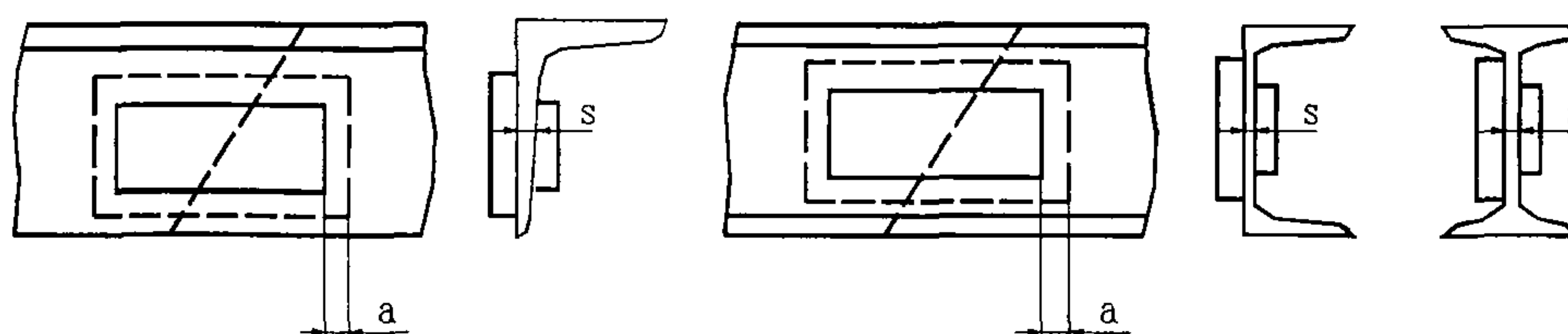
Рисунок 13 Расстояние между сварными швами в противоположных планках
