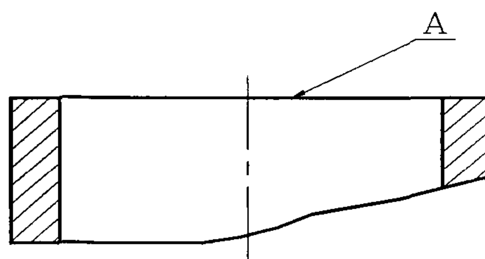
Рисунок 10 Отклонение от перпендикулярности торца А
