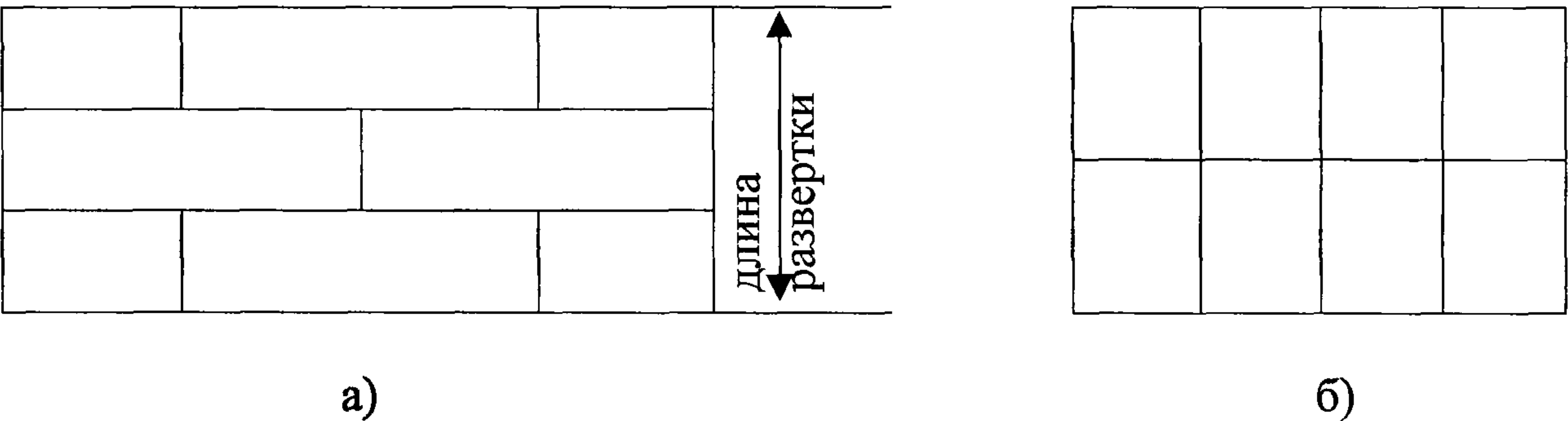
Рисунок 9. Развертка обечаек
