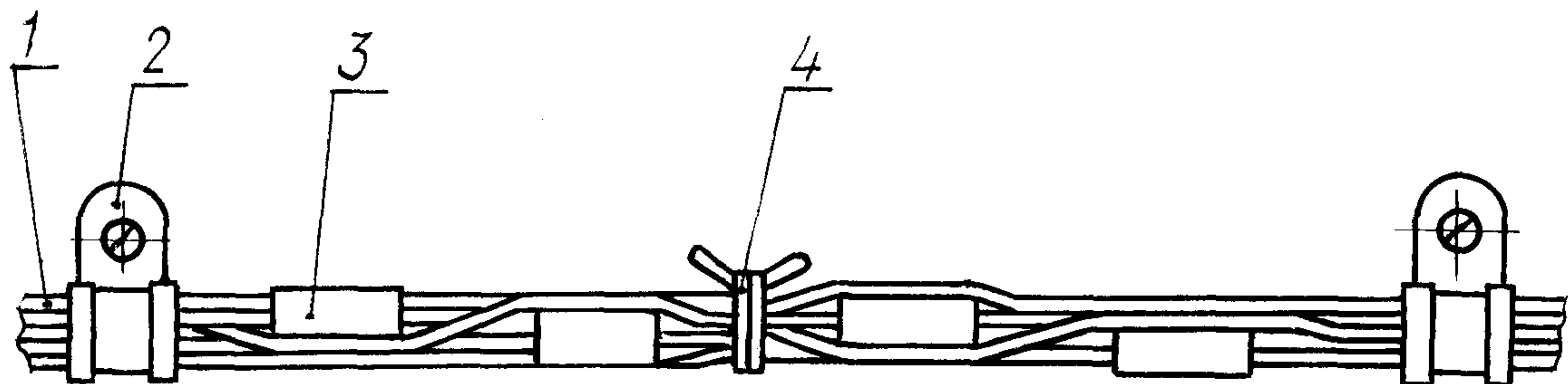
1 - жгут; 2 - хомут; 3 - муфта сращивания; 4 - бандаж
