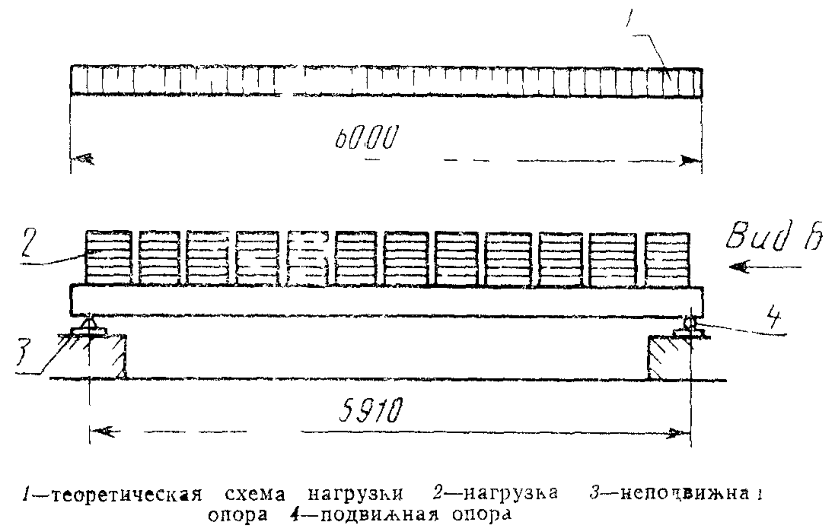
Схема испытания плит
