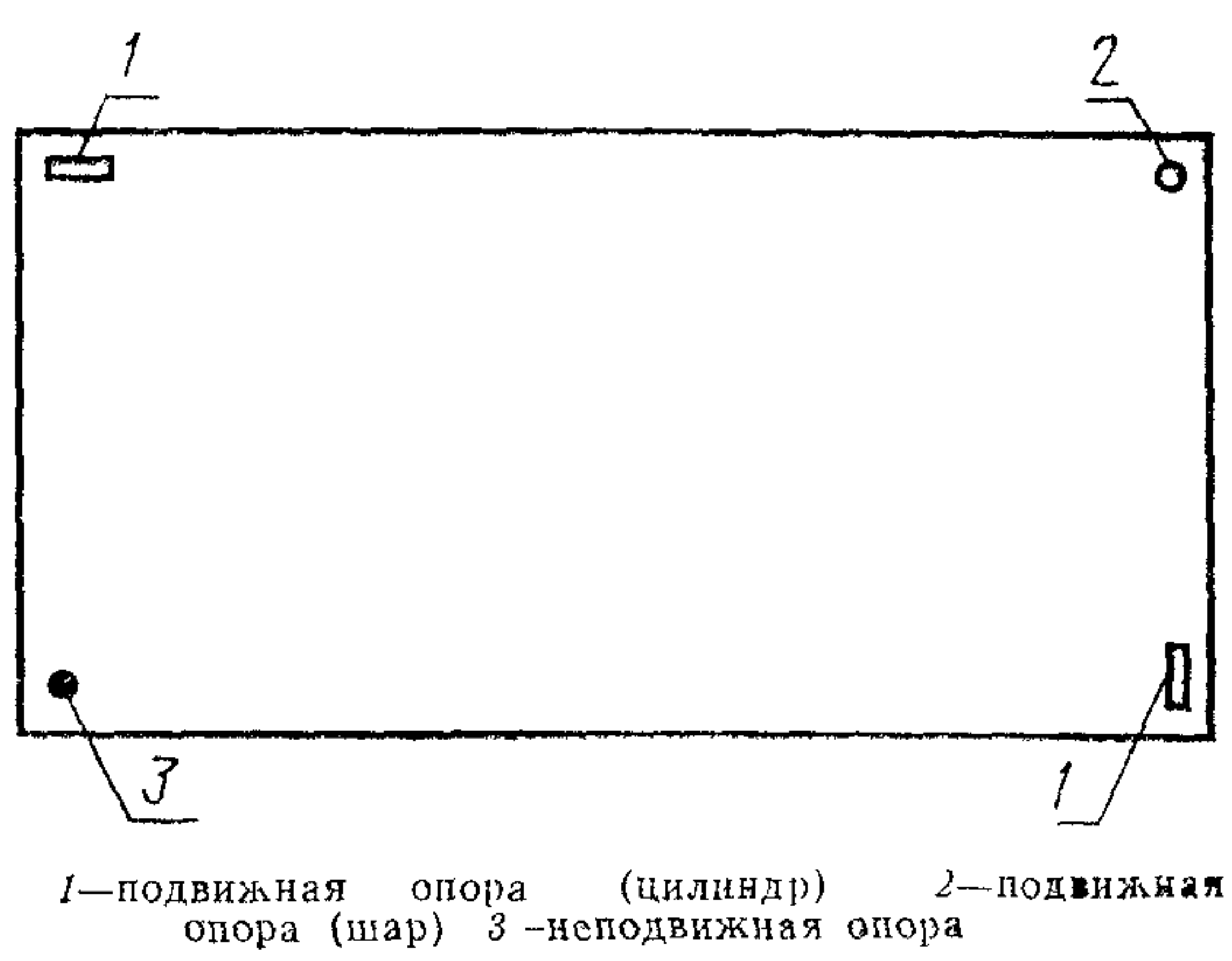
Схема перемещения продольных ребер плиты при загрузении
