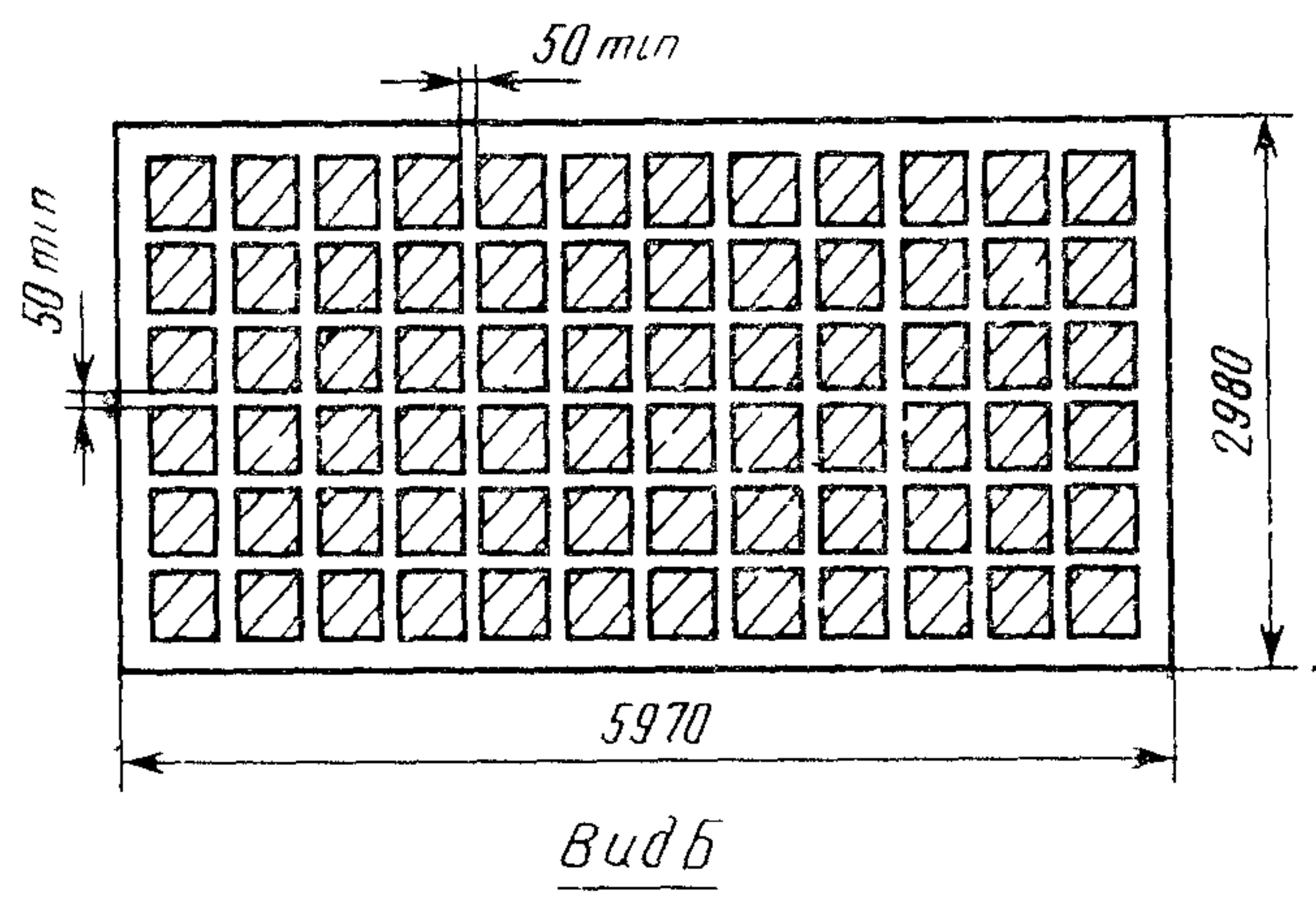
Расположение нагрузки на плите в плане
