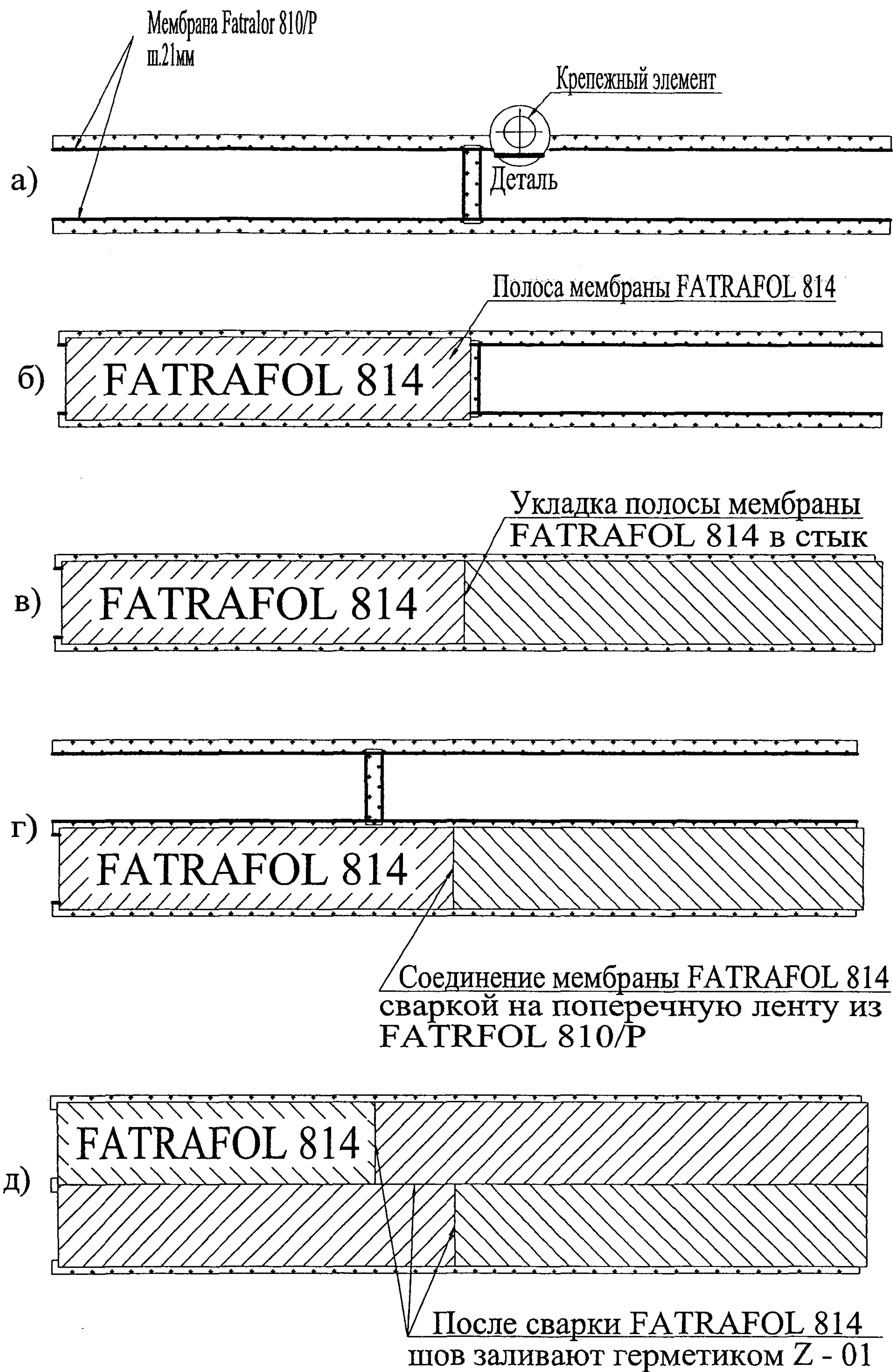
Рис. 4. Укладка мембраны Fatrafol 814
