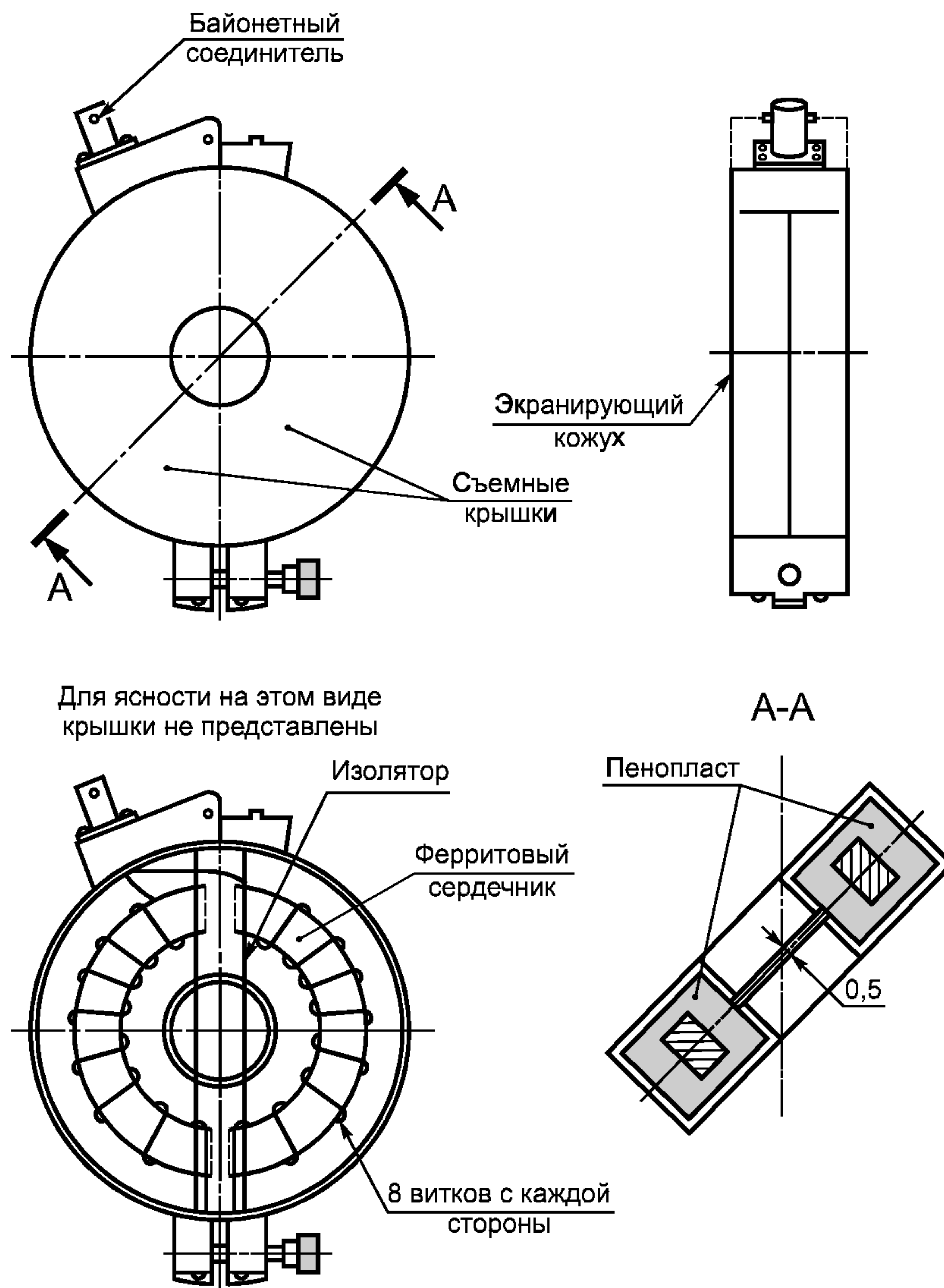
Рисунок Б.1 — Типовая конфигурация пробника тока
