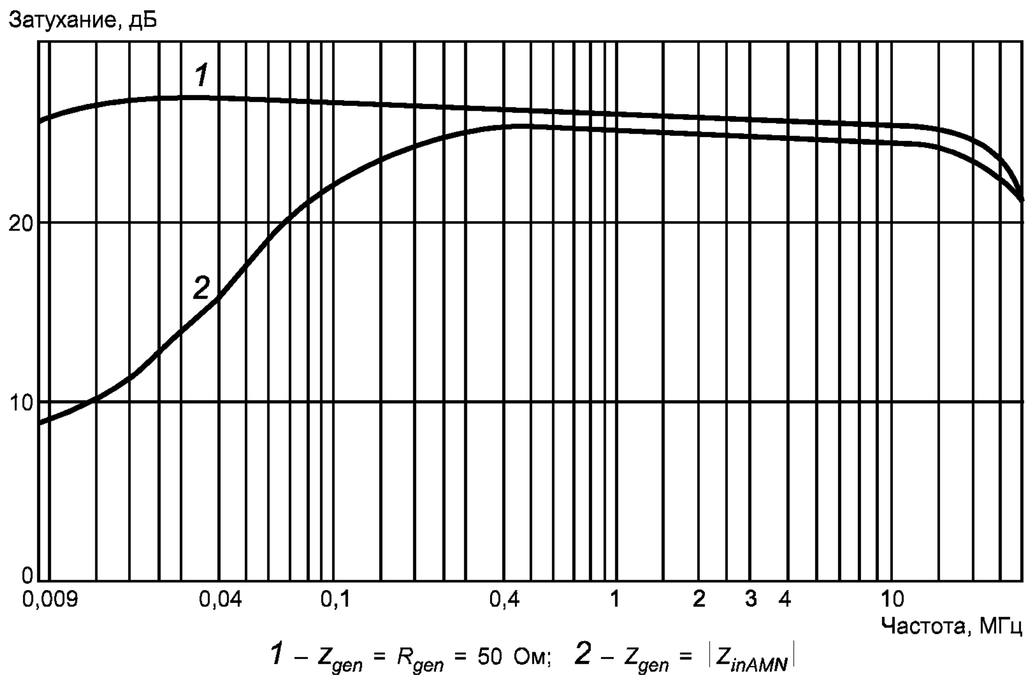
Рисунок А.5 — Затухание фильтра эквивалента сети питания
