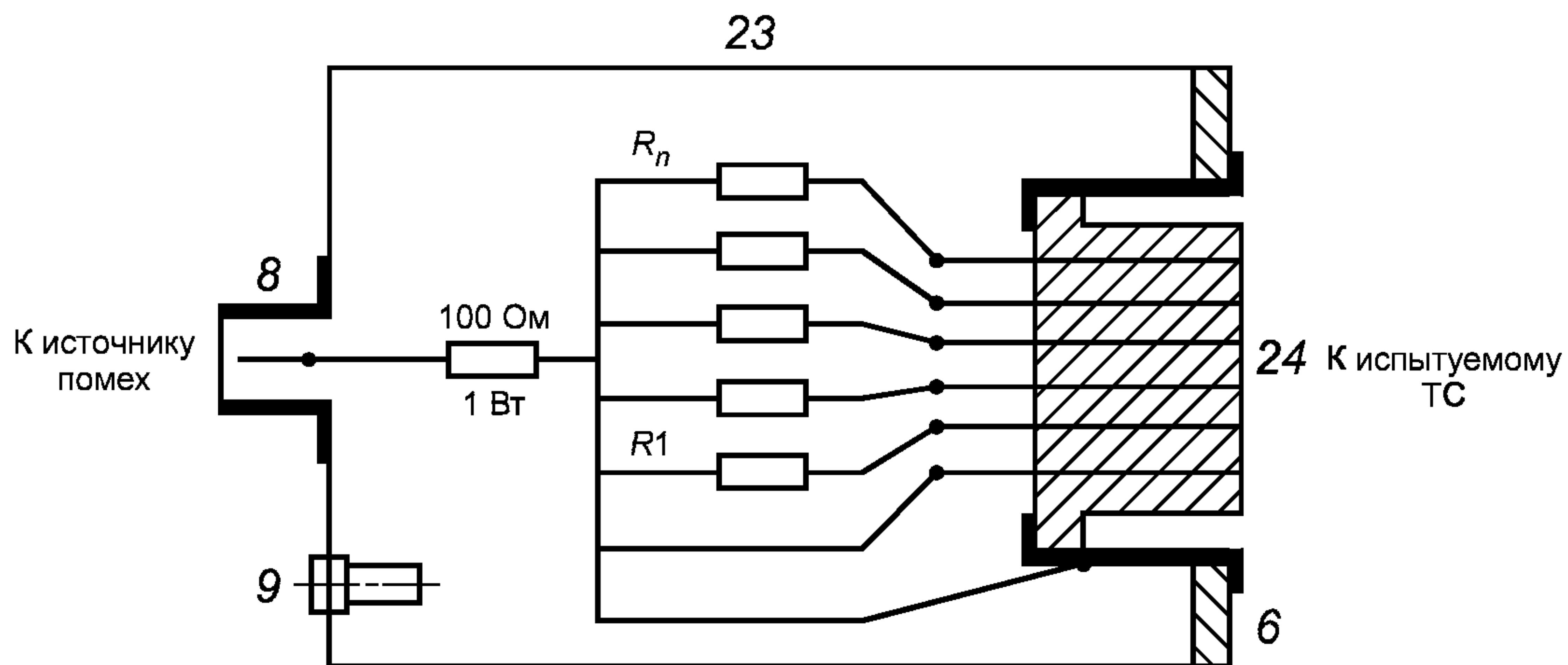
6, 8, 9 — см. устройство связи типа А; 23 — металлический корпус 100 × 55 × 55 мм; 24 — многштырьковый разъем; R_1 — R_n — согласованные нагрузочные сопротивления
