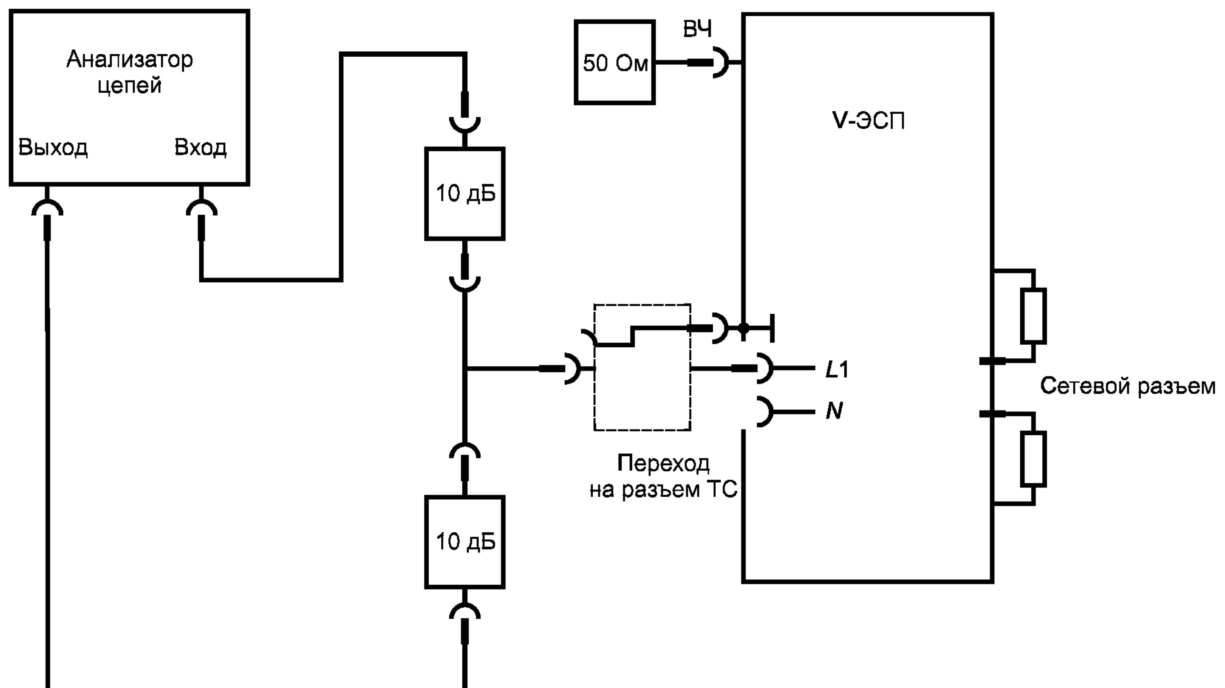
а) Калибровка выходного напряжения анализатора цепей
