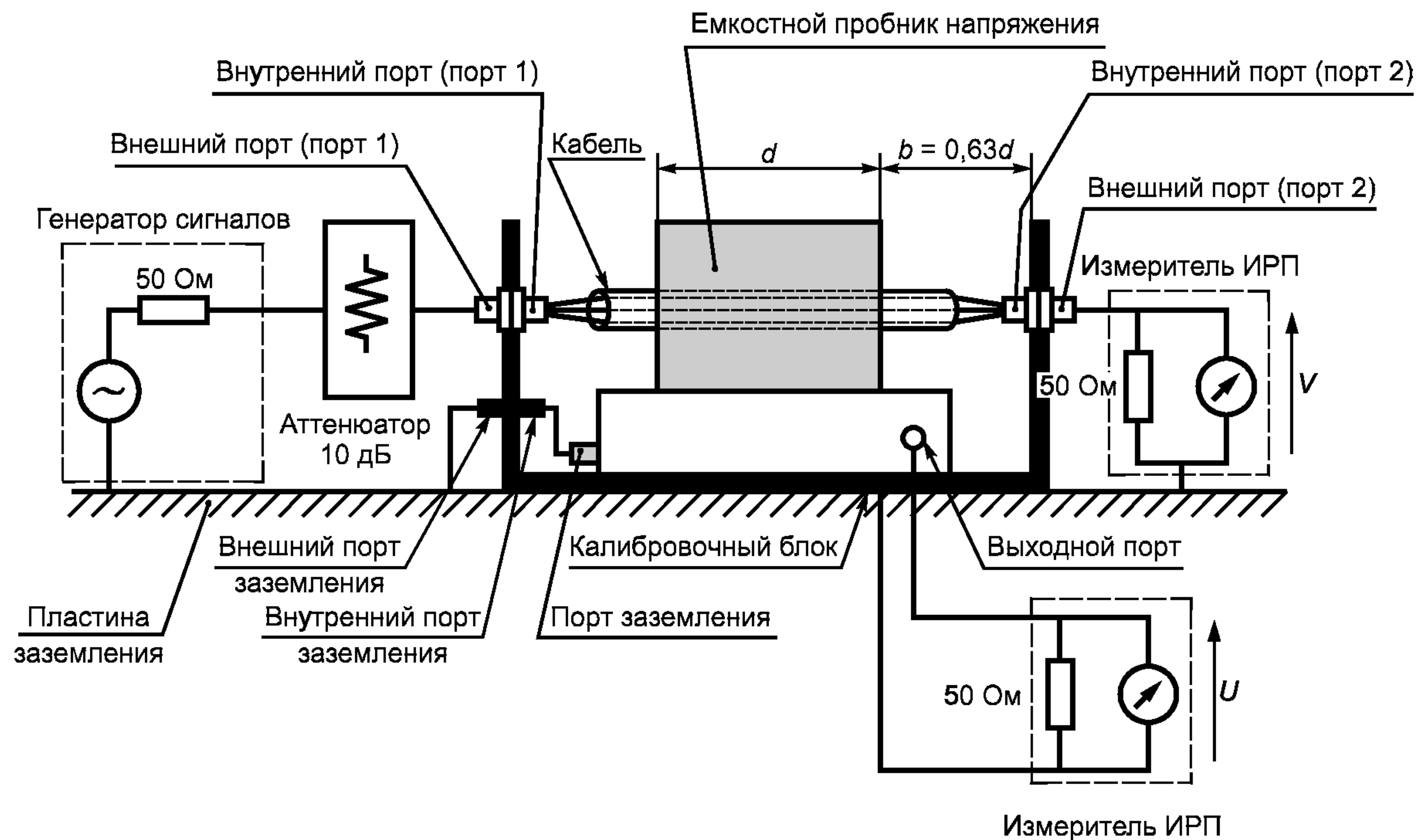
Рисунок Ж.3 — Испытательная установка для измерения частотной зависимости коэффициента калибровки
