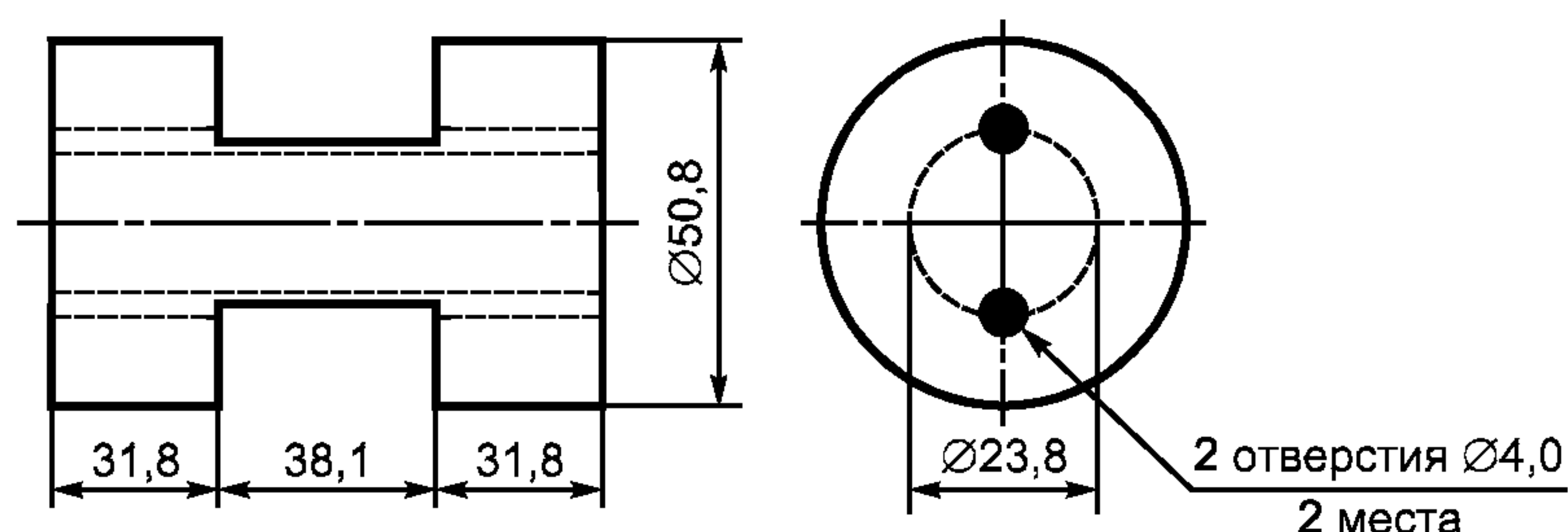
Рисунок Б.5 — Конструкция дополнительного экрана
