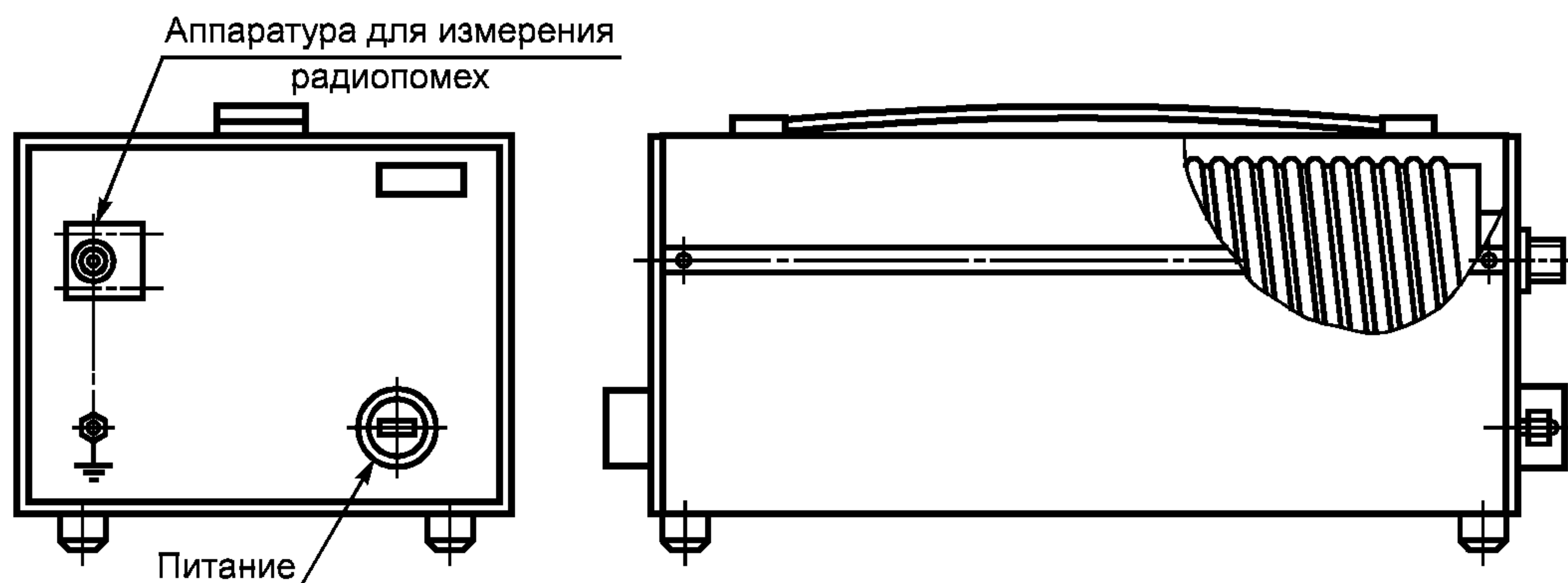
Рисунок А.4 — Общий вид эквивалента сети питания
