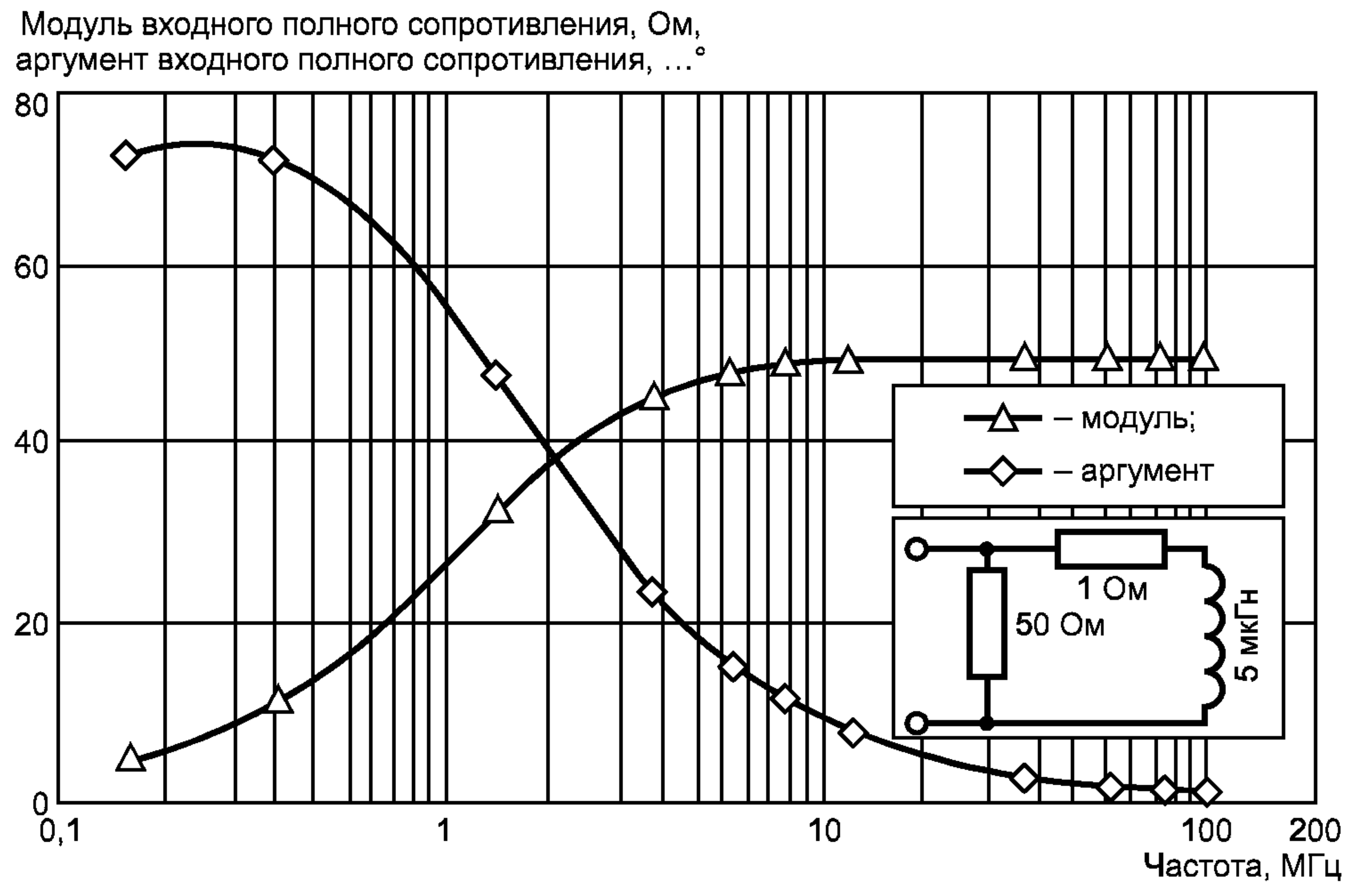
Рисунок 2 — Значение модуля и аргумента входного полного сопротивления V-образного эквивалента сети питания в соответствии с 4.4 (для полос частот В и С — по ГОСТ Р 51318.16.1.1) (от 0,15 до 108 МГц)
