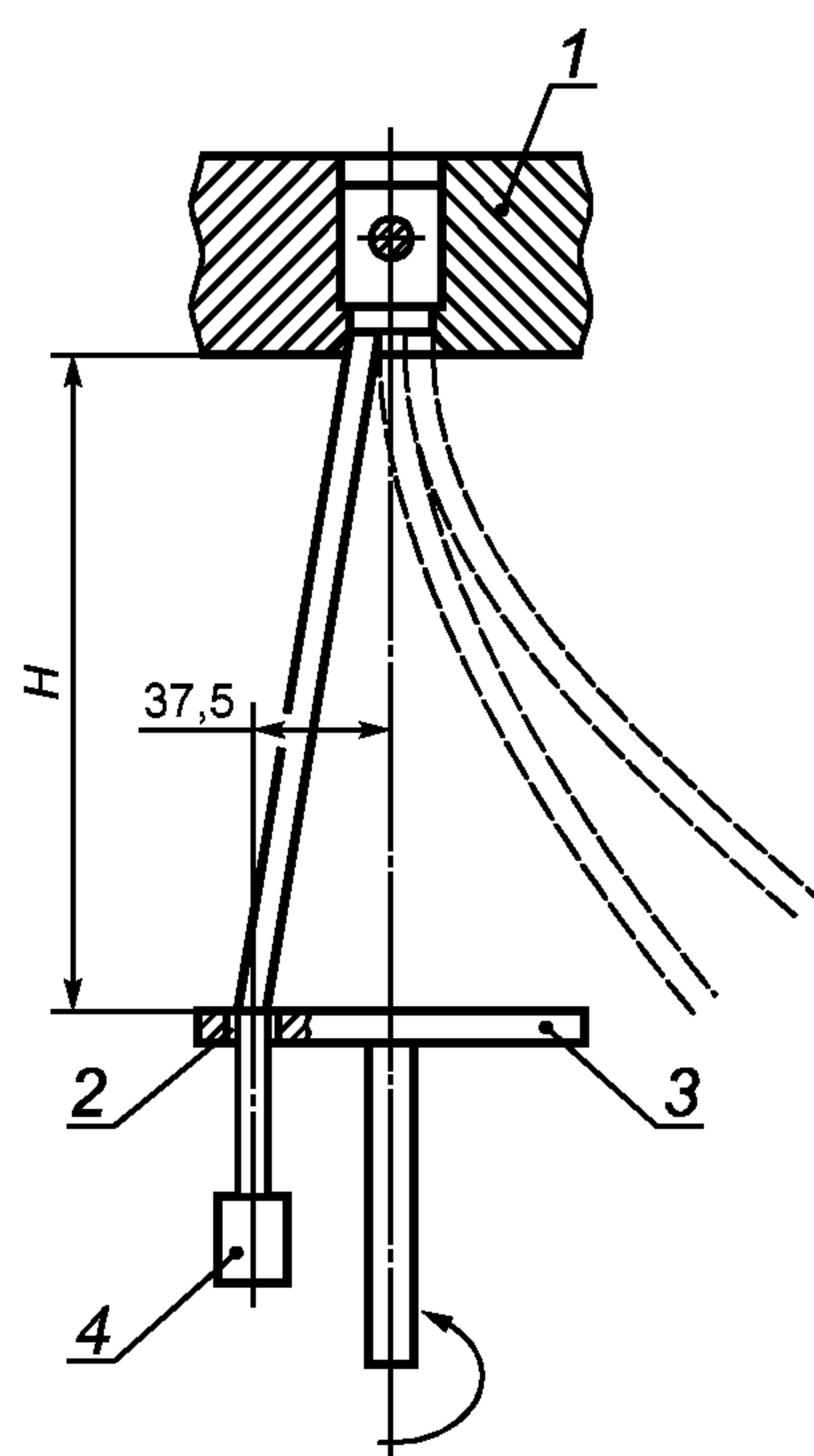
1 — узел фиксации; 2 — гильза; 3 — диск; 4 — груз
