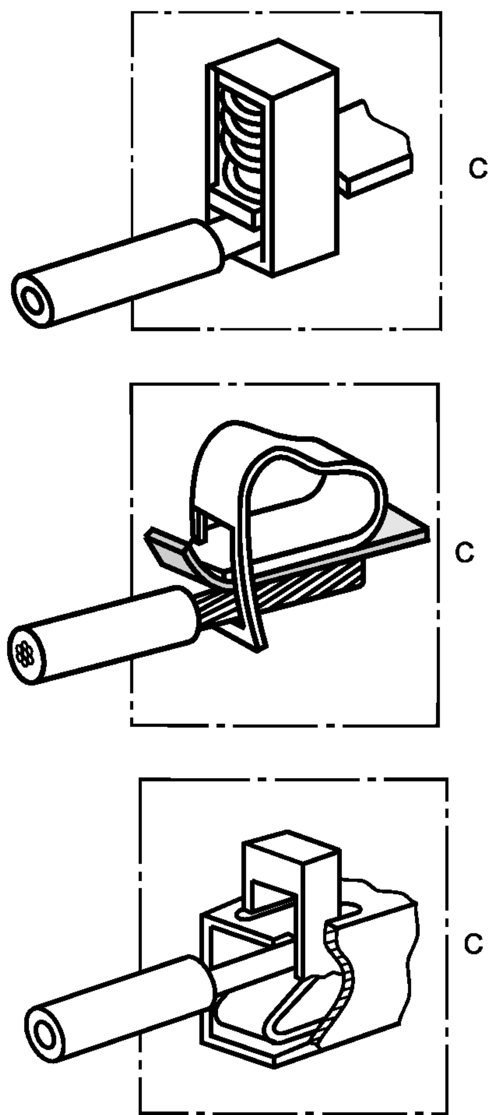
Рисунок D.7 — Безрезьбовые выводы
