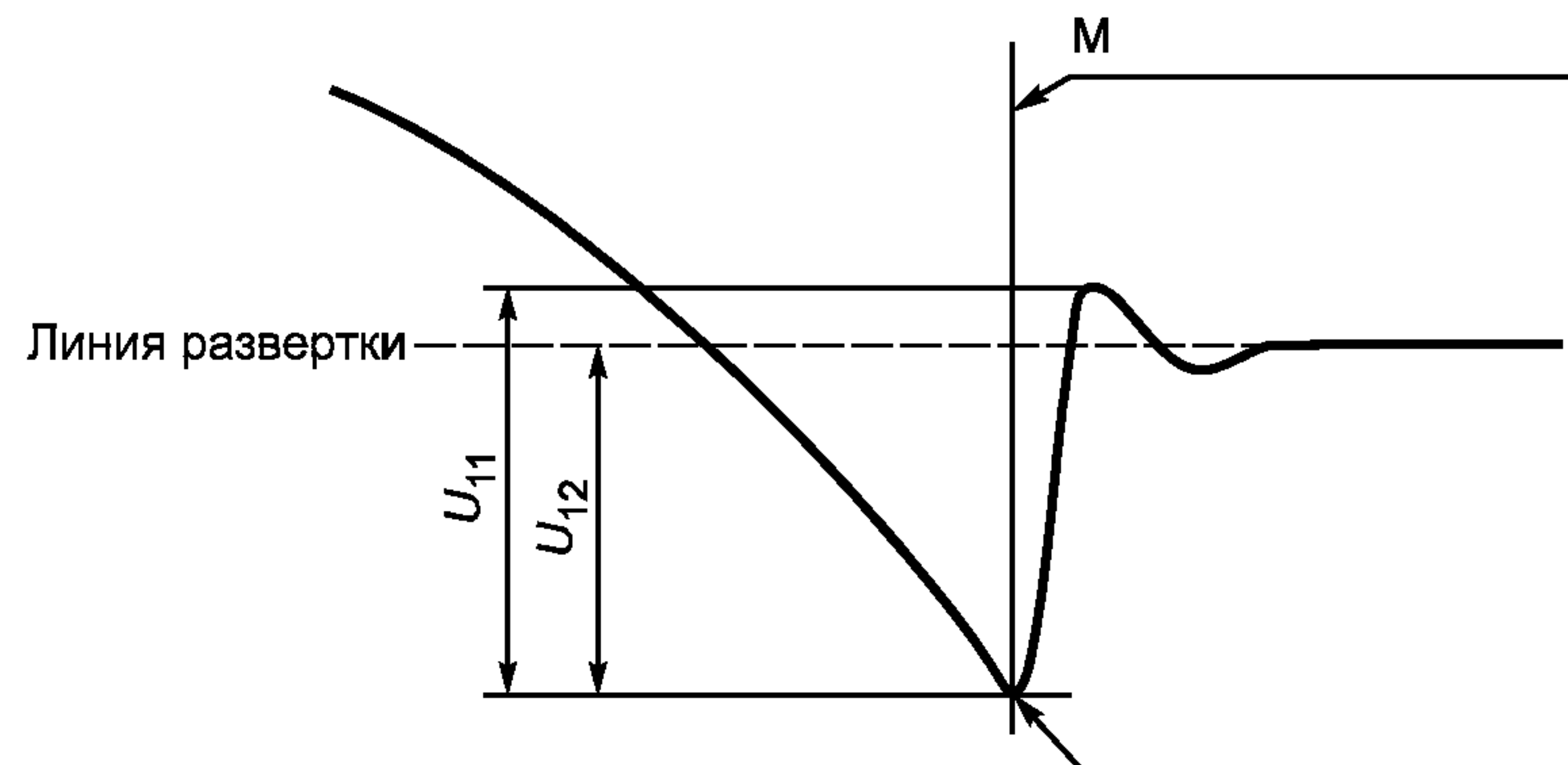
Рисунок Е.1 — Определение фактического значения коэффициента \gamma
