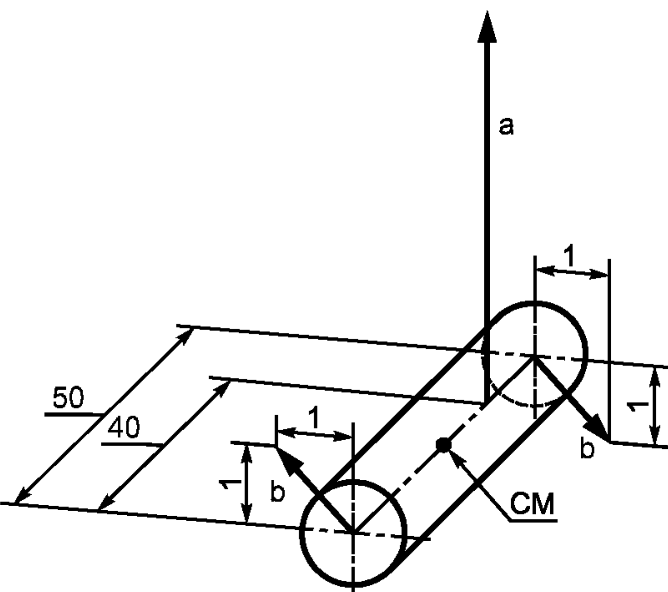
а) Главный вектор дисбалансов с парой косо-симметричных дисбалансов в торцовых плоскостях ротора
