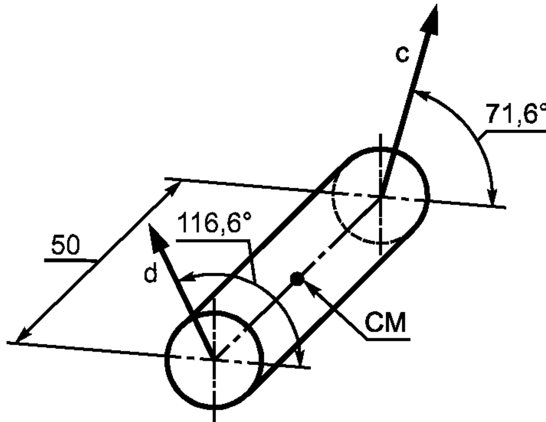
д) Векторы дисбалансов в торцовых плоскостях ротора
