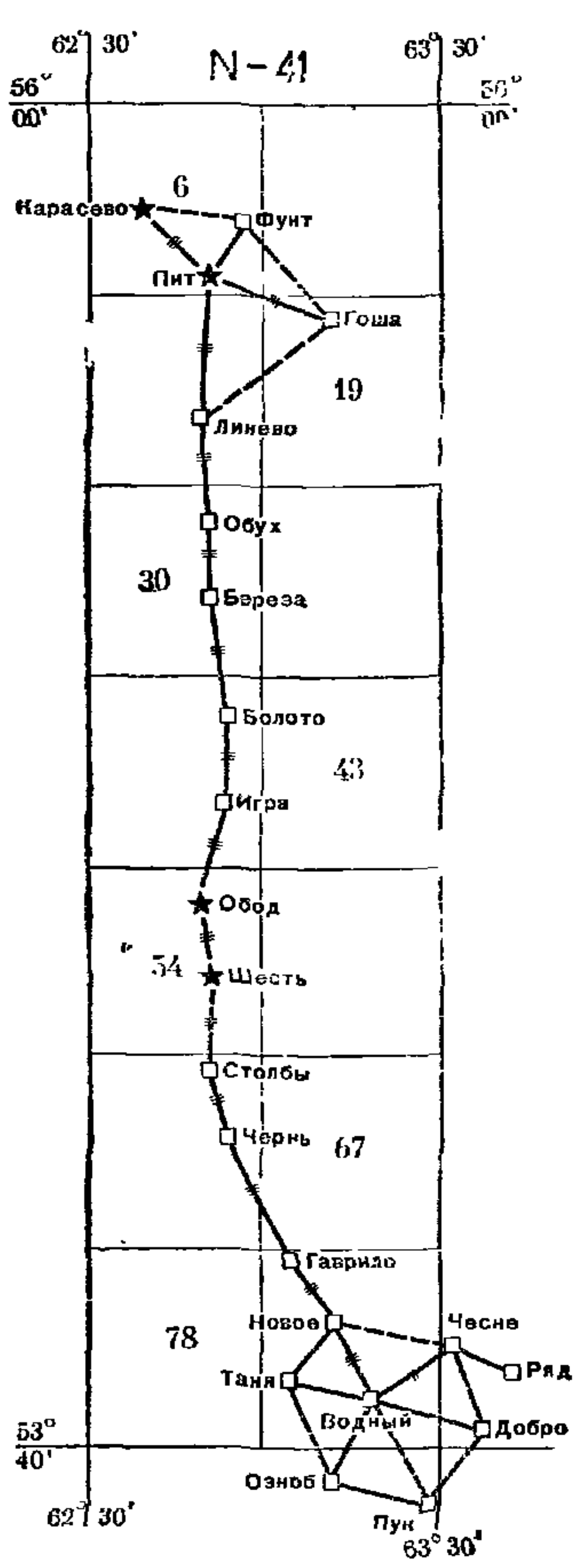
Схема звена полигонометрии 1 класса Карасево — водный
