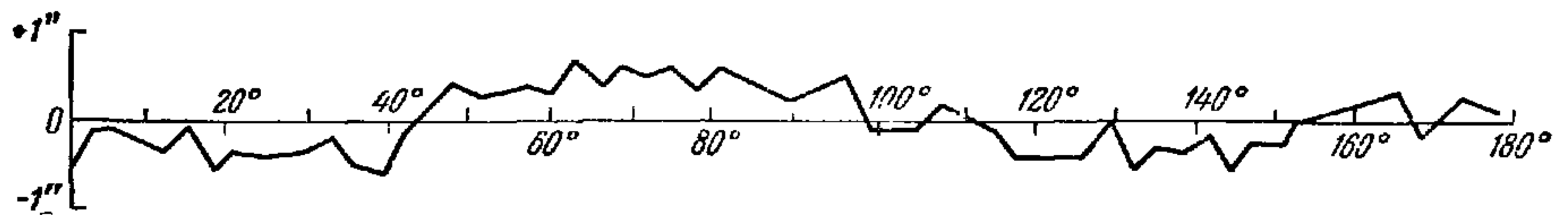
График ошибок диаметров круга триангуляционного теодолита ТТ2"/6" № 8542
