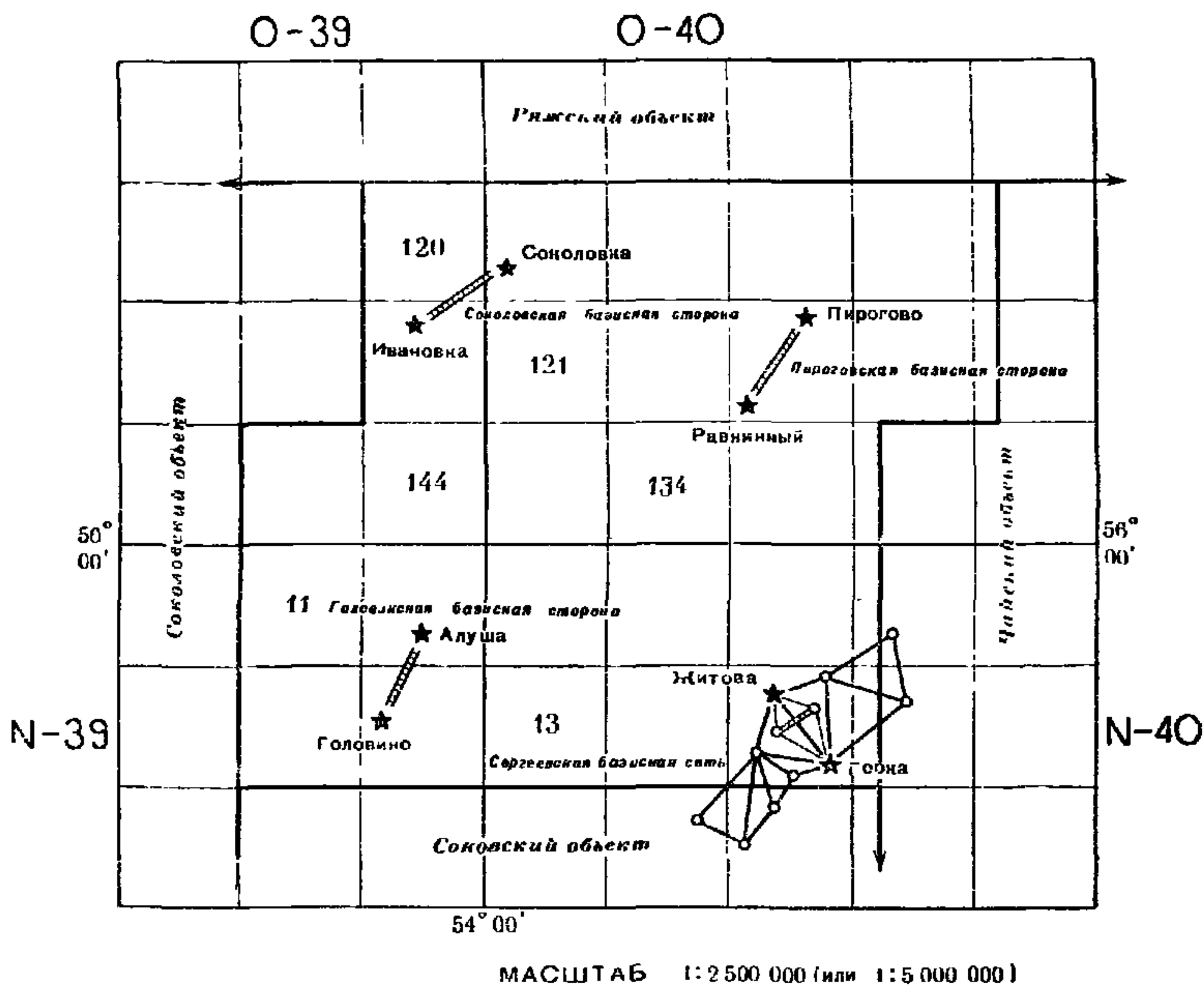
Схема исходной основы Кумской сплошной сети триангуляции 1 класса
