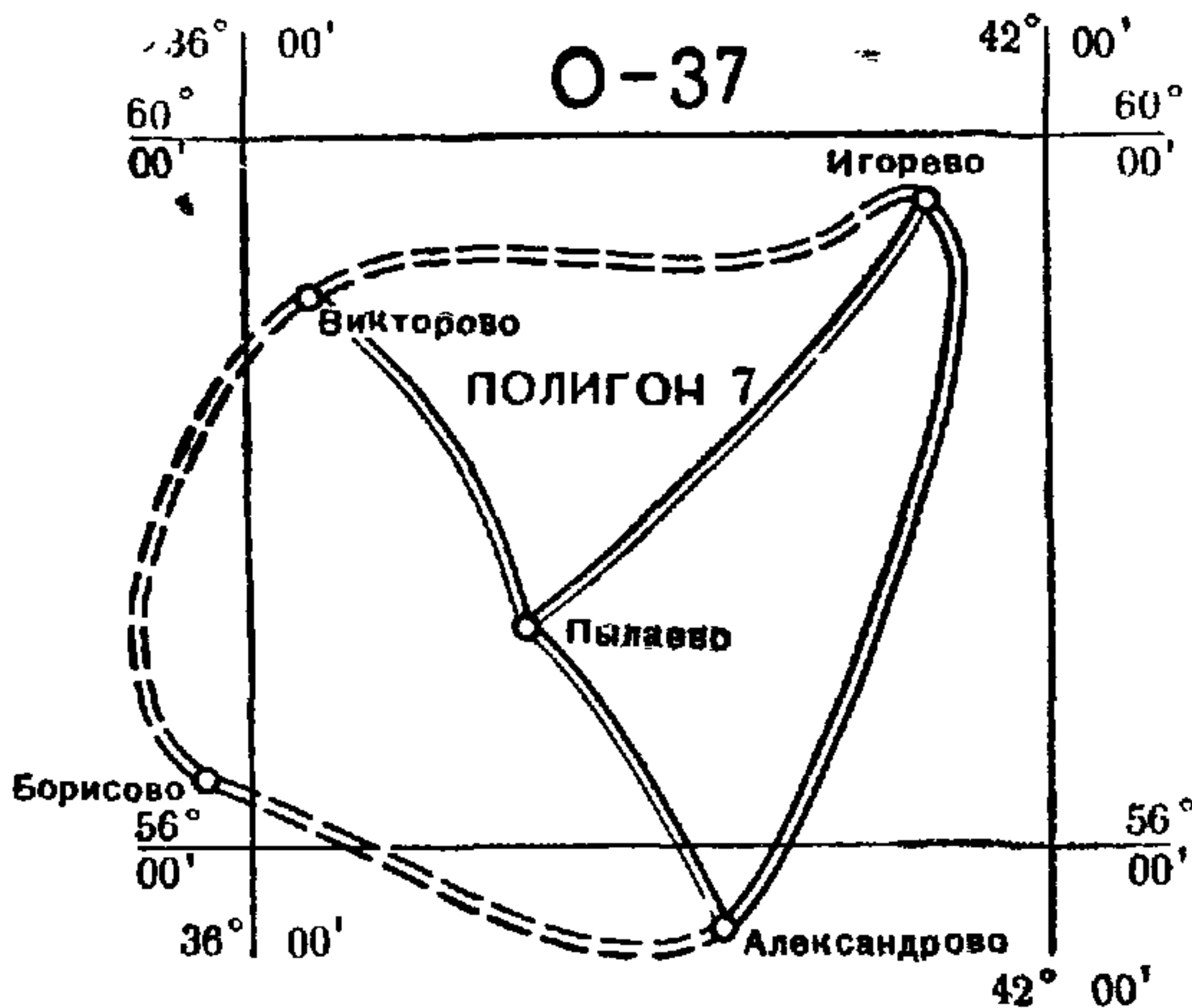
Схема нивелирования I класса Игорево—Александрово
