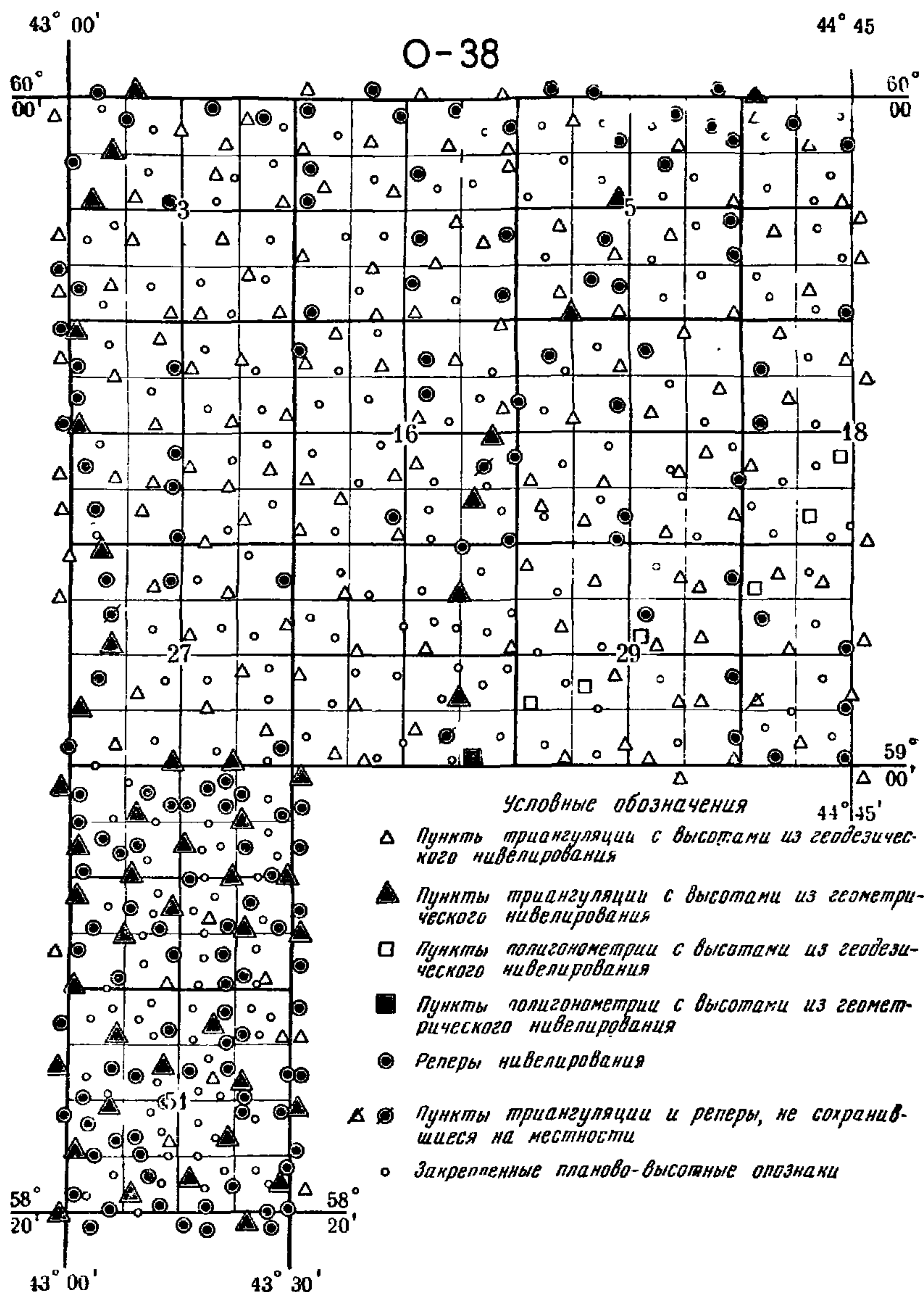
Схема плановой и высотной геодезической основы на Орловском объекте
