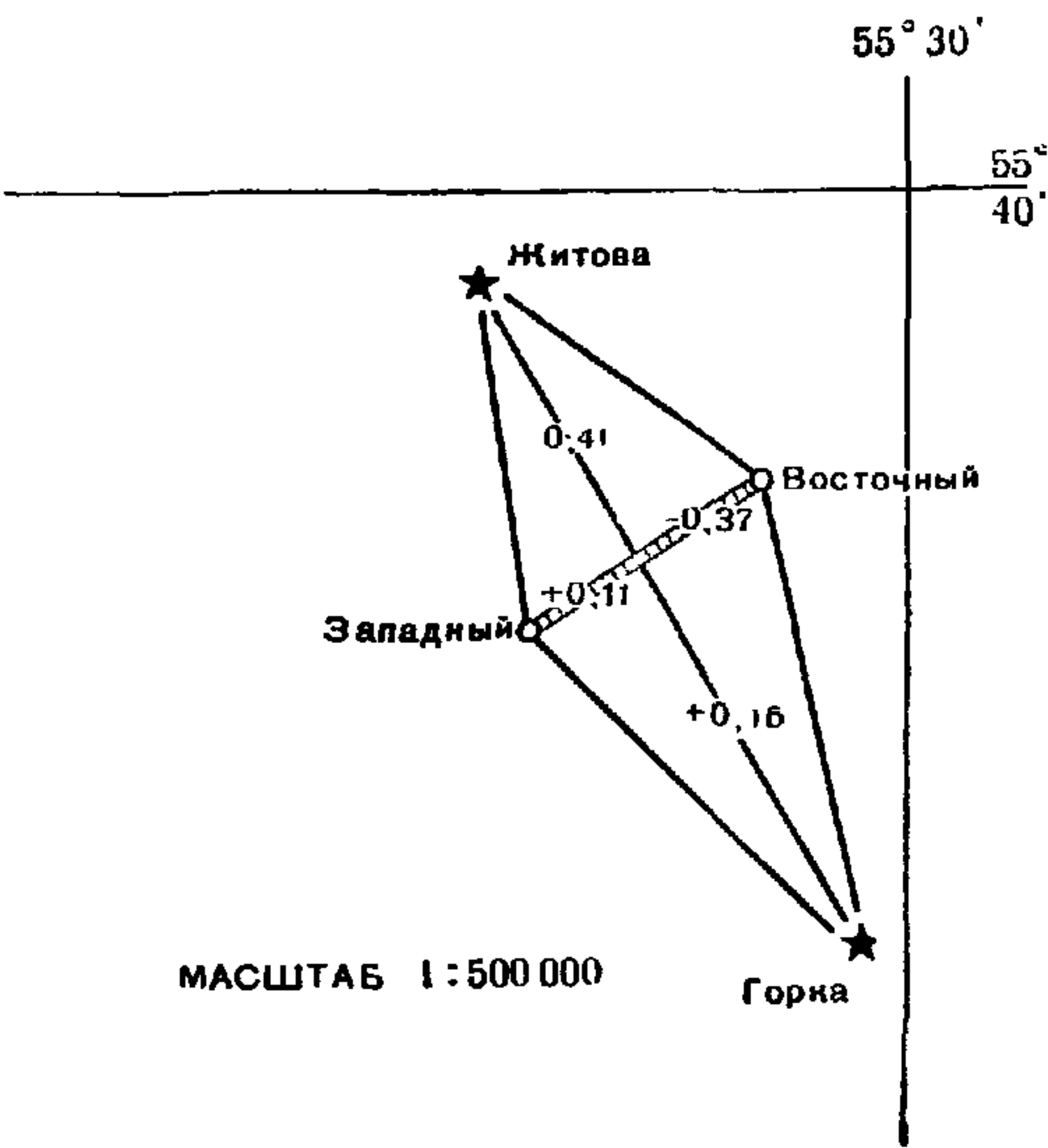
Схема Сергеевской базисной сети
