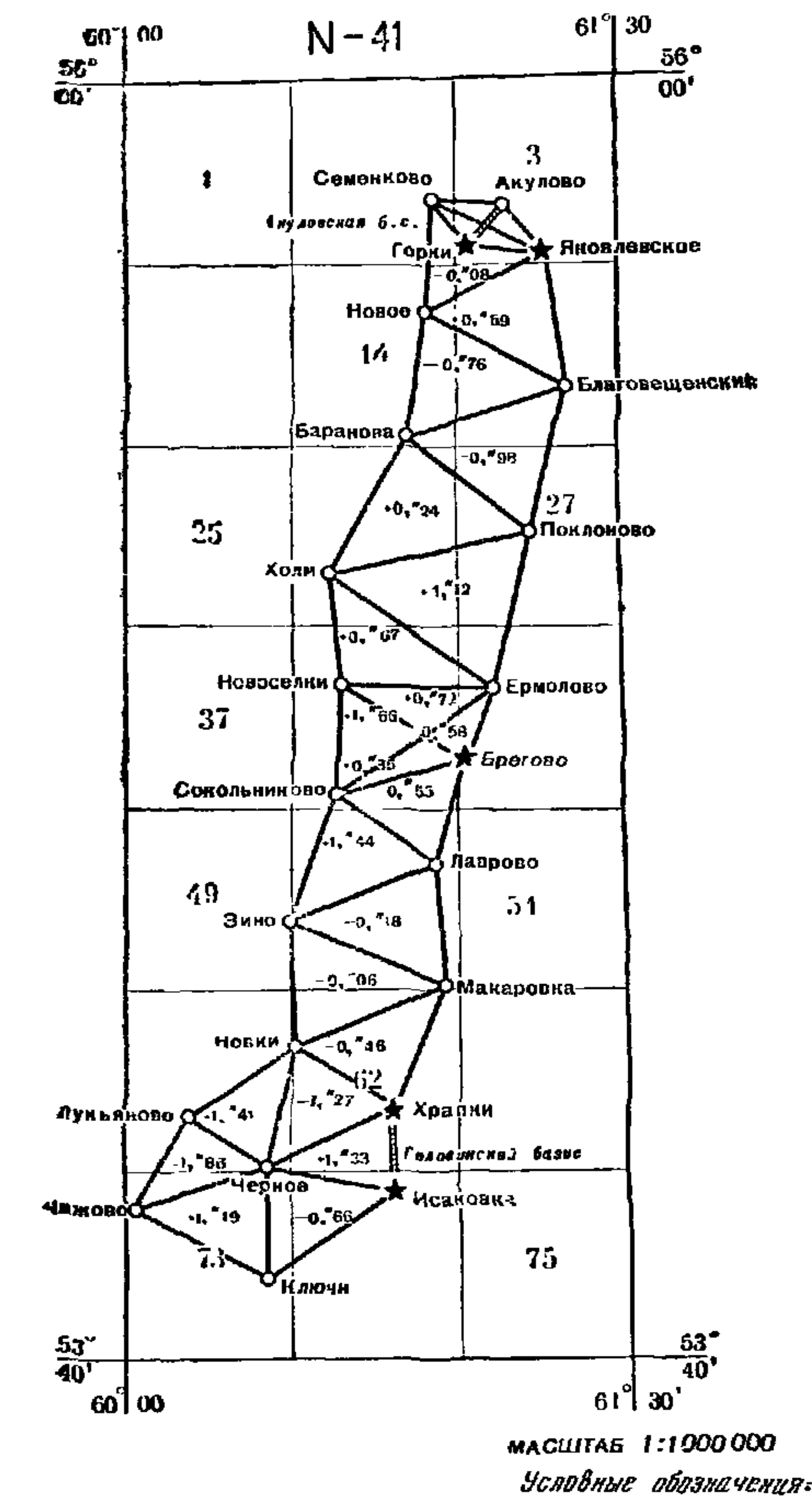
Схема звена триангуляции 1 класса Акулово — Головино
