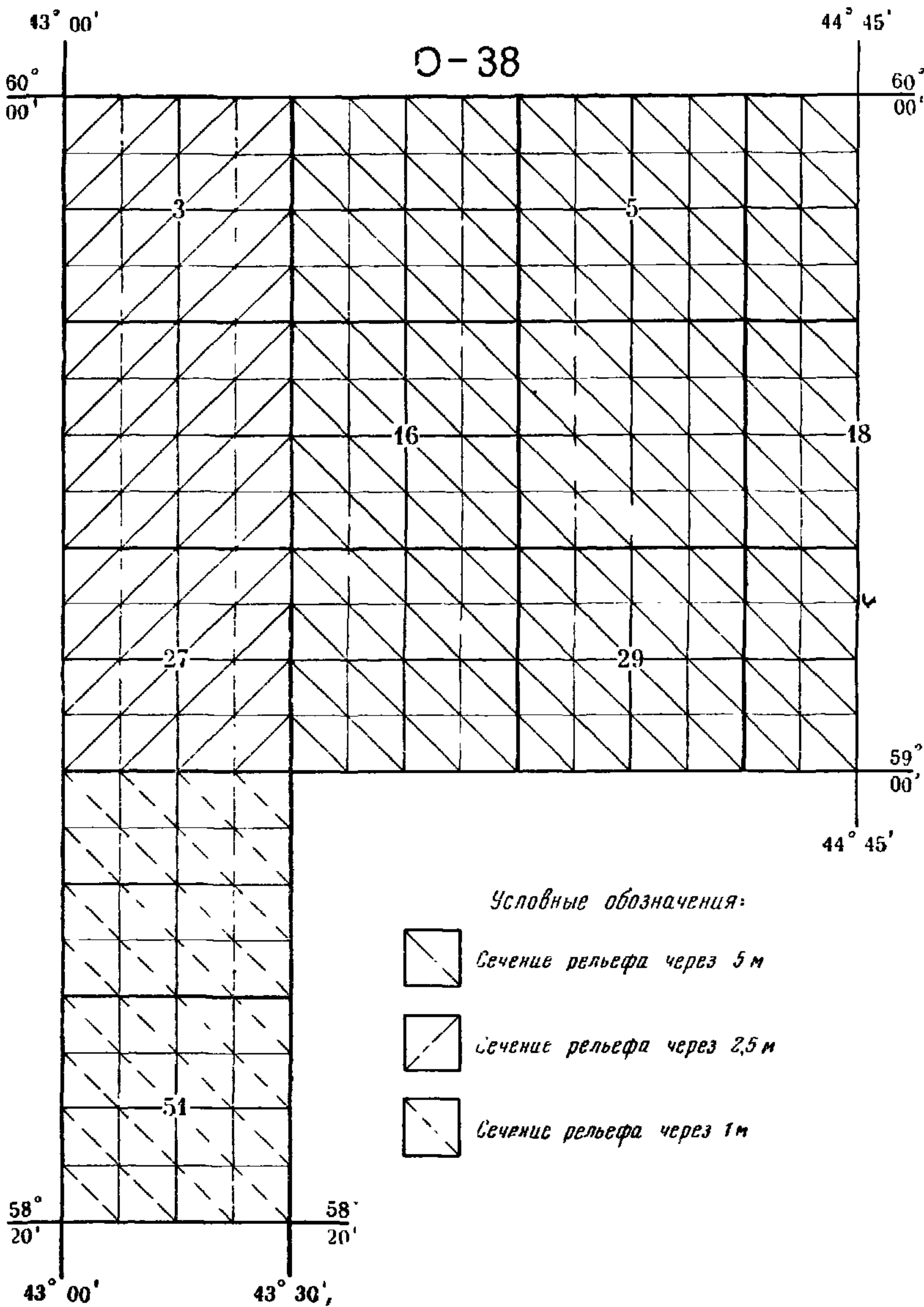
Схема сечений рельефа на Орловском объекте
