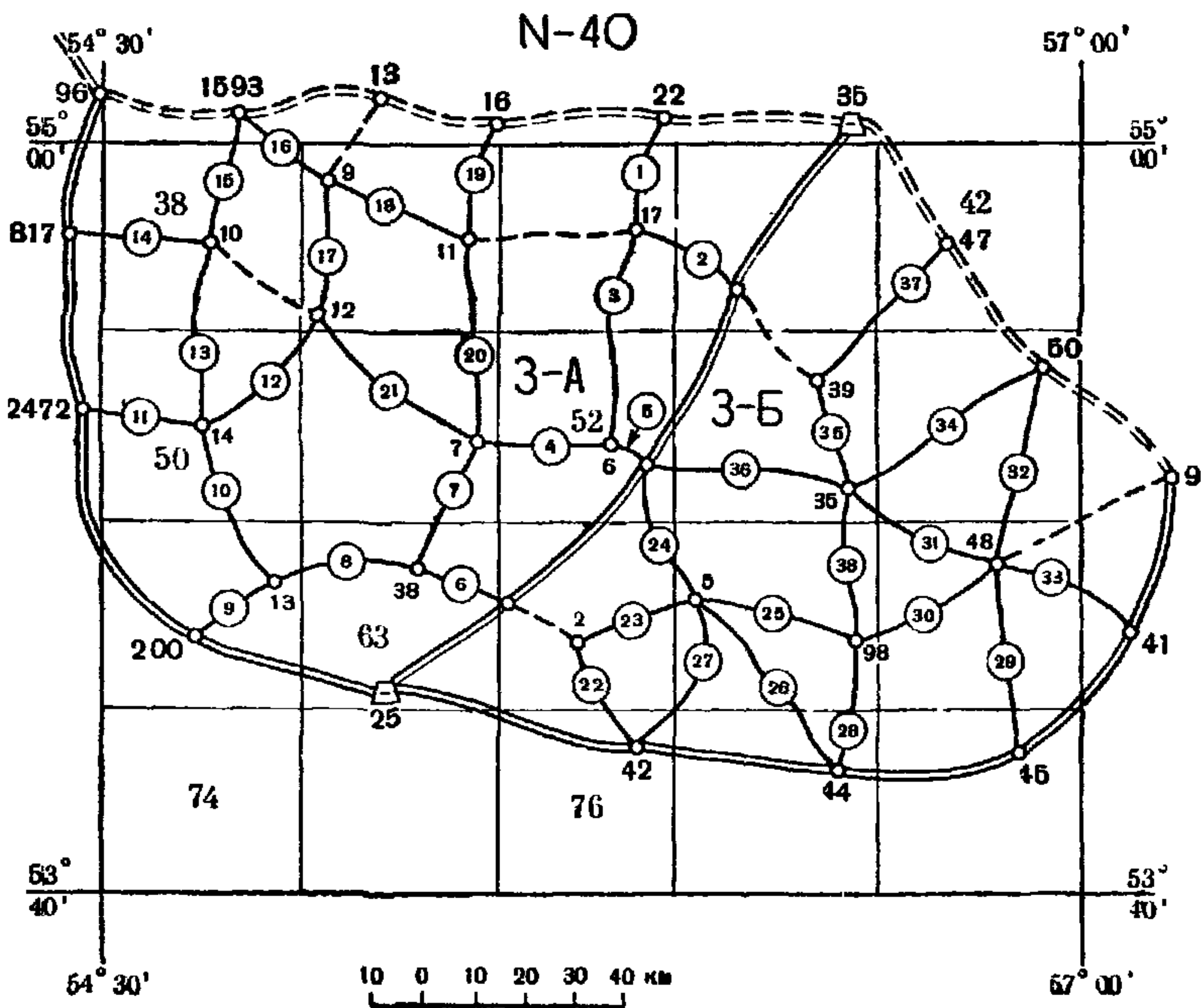
Схема полигонов сети нивелирования II и III классов
