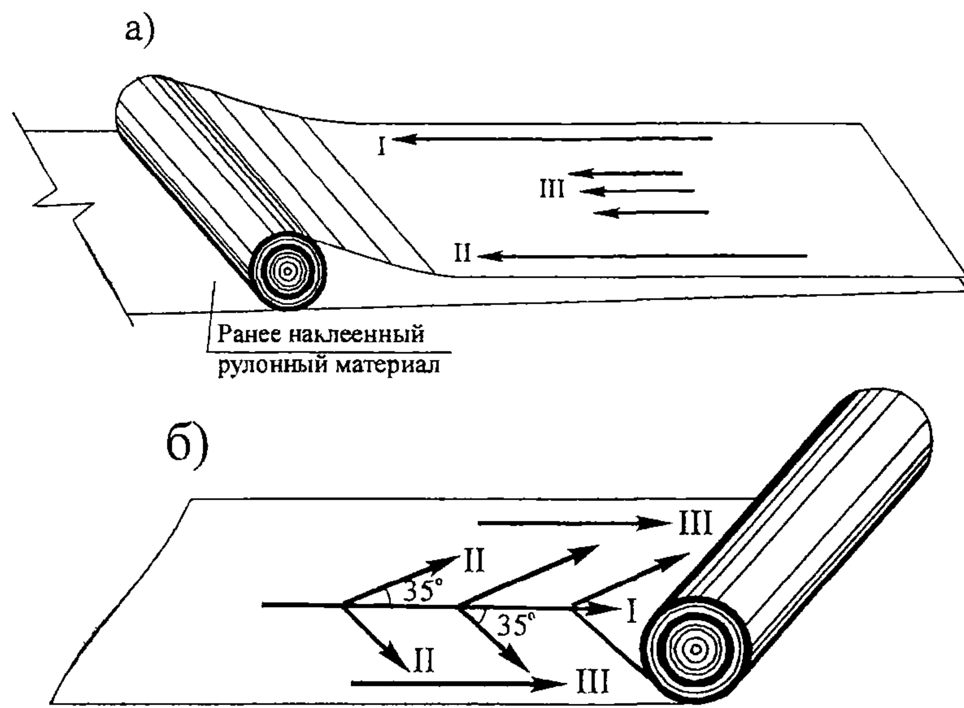
а) Нанесение мастики I-III – очередность нанесения мастики б) Прижатие рулонного материала I-III последовательность работы шпателя
