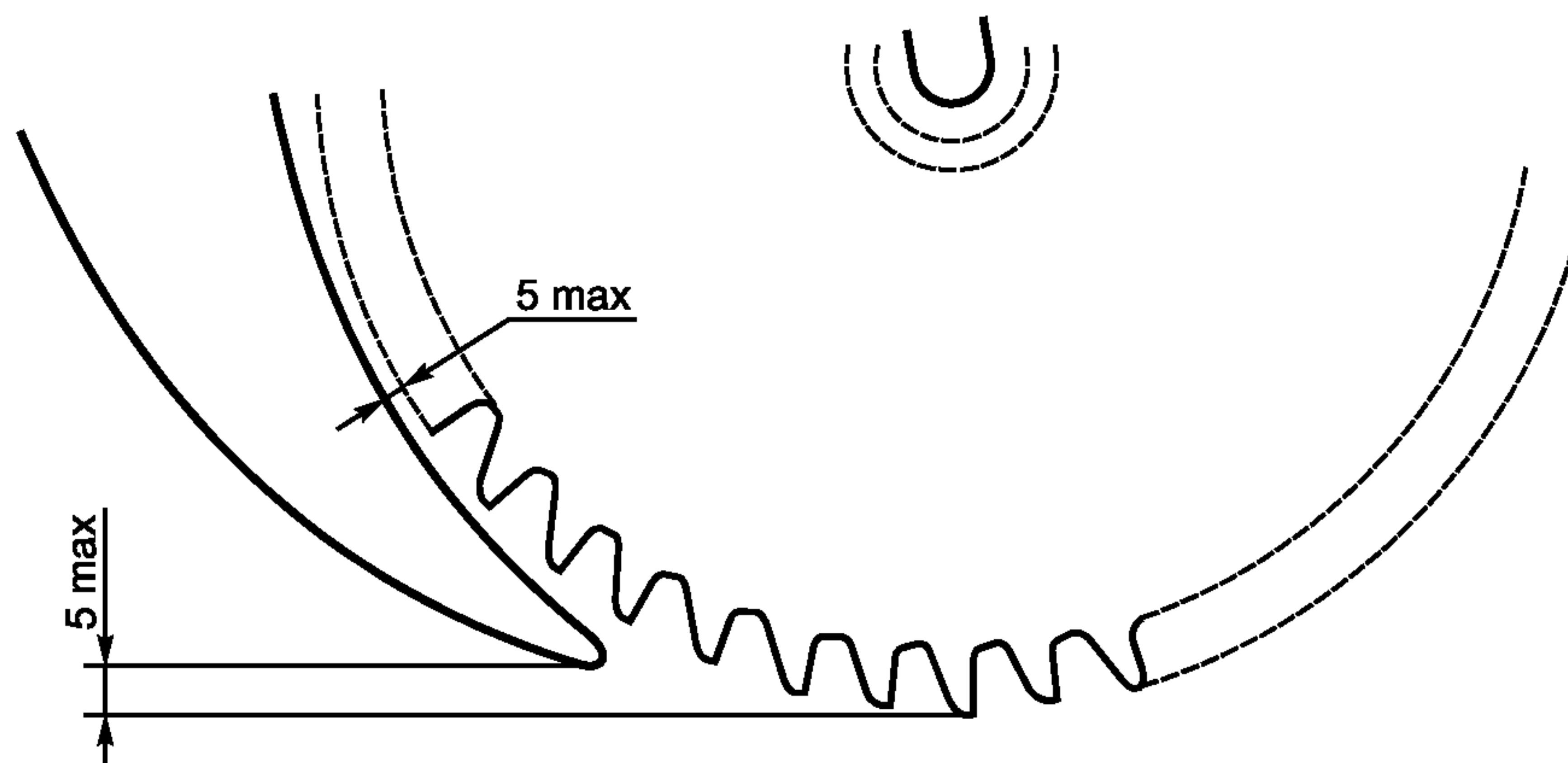
Рисунок АА.102 — Регулирование расклинивающего ножа
