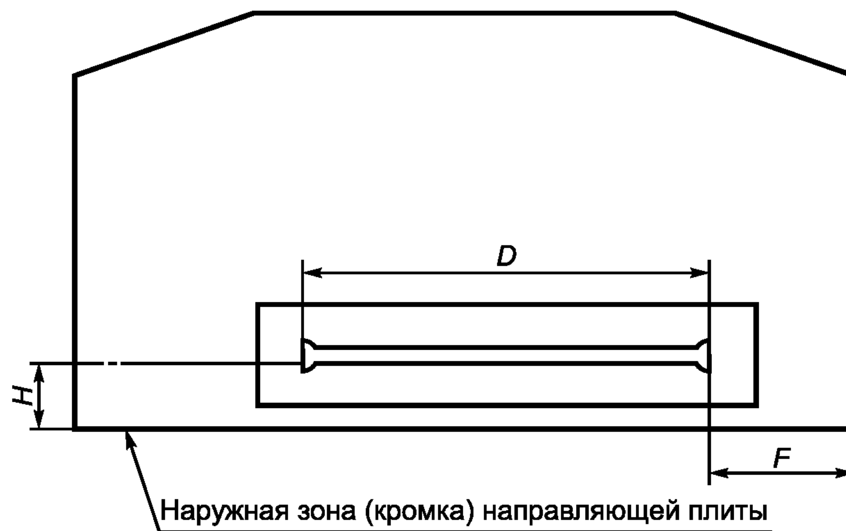
Рисунок 113 — Основные размеры направляющей плиты
