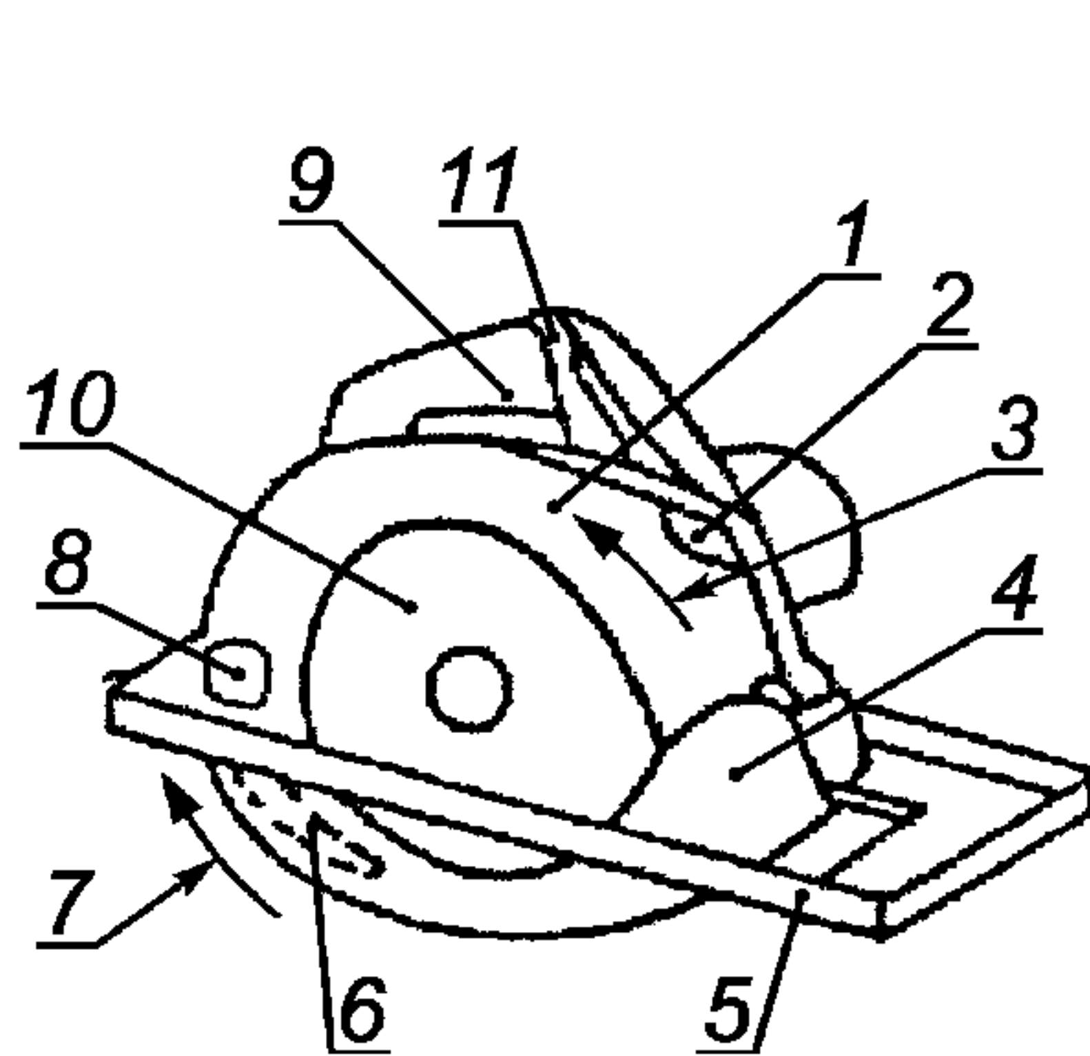
Рисунок 103 — Дисковая пила с защитным кожухом тянущегося типа
