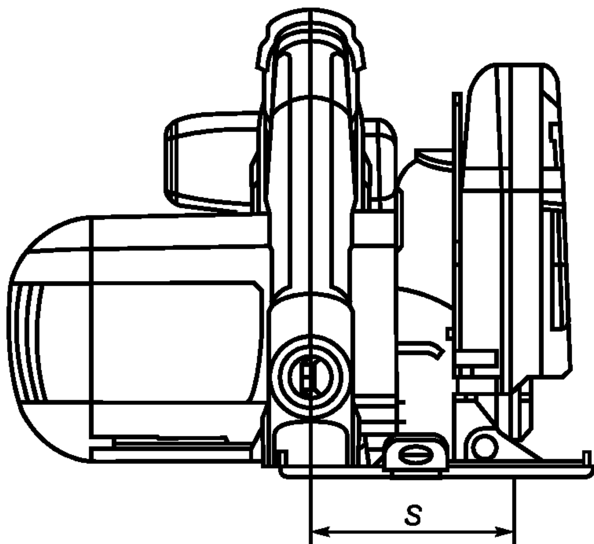
Рисунок 108с — Размер S
