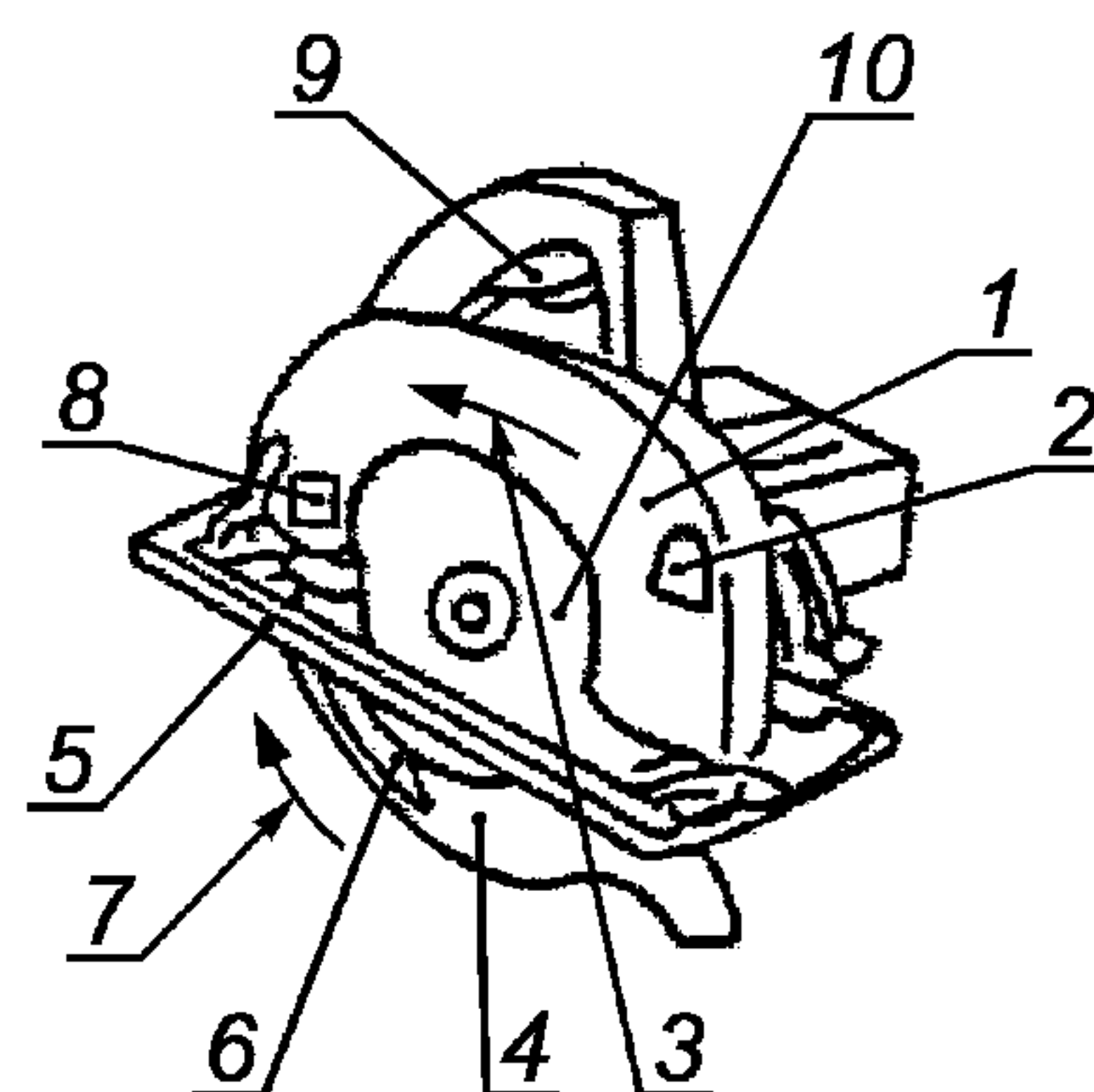
Рисунок 102 — Дисковая пила с внутренним качающимся защитным кожухом
