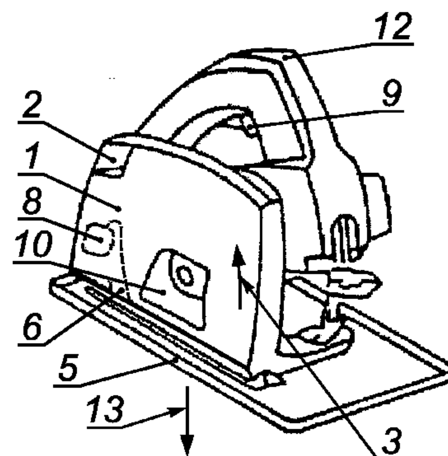
Рисунок 104 — Дисковая пила погружного типа
