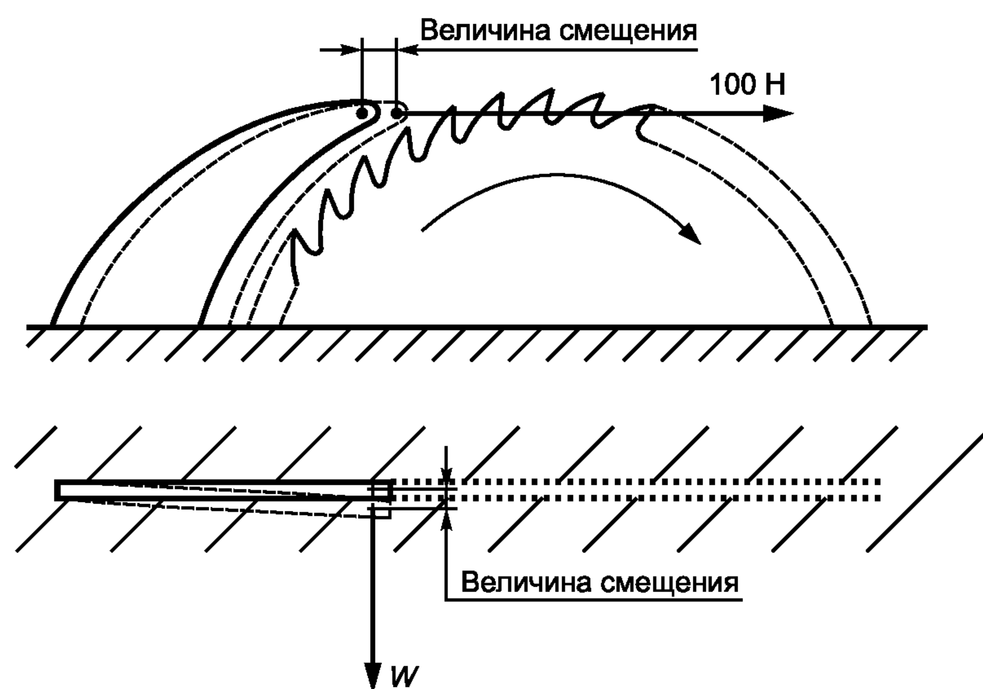
Рисунок АА.101 — Испытание расклинивающего ножа на устойчивость
