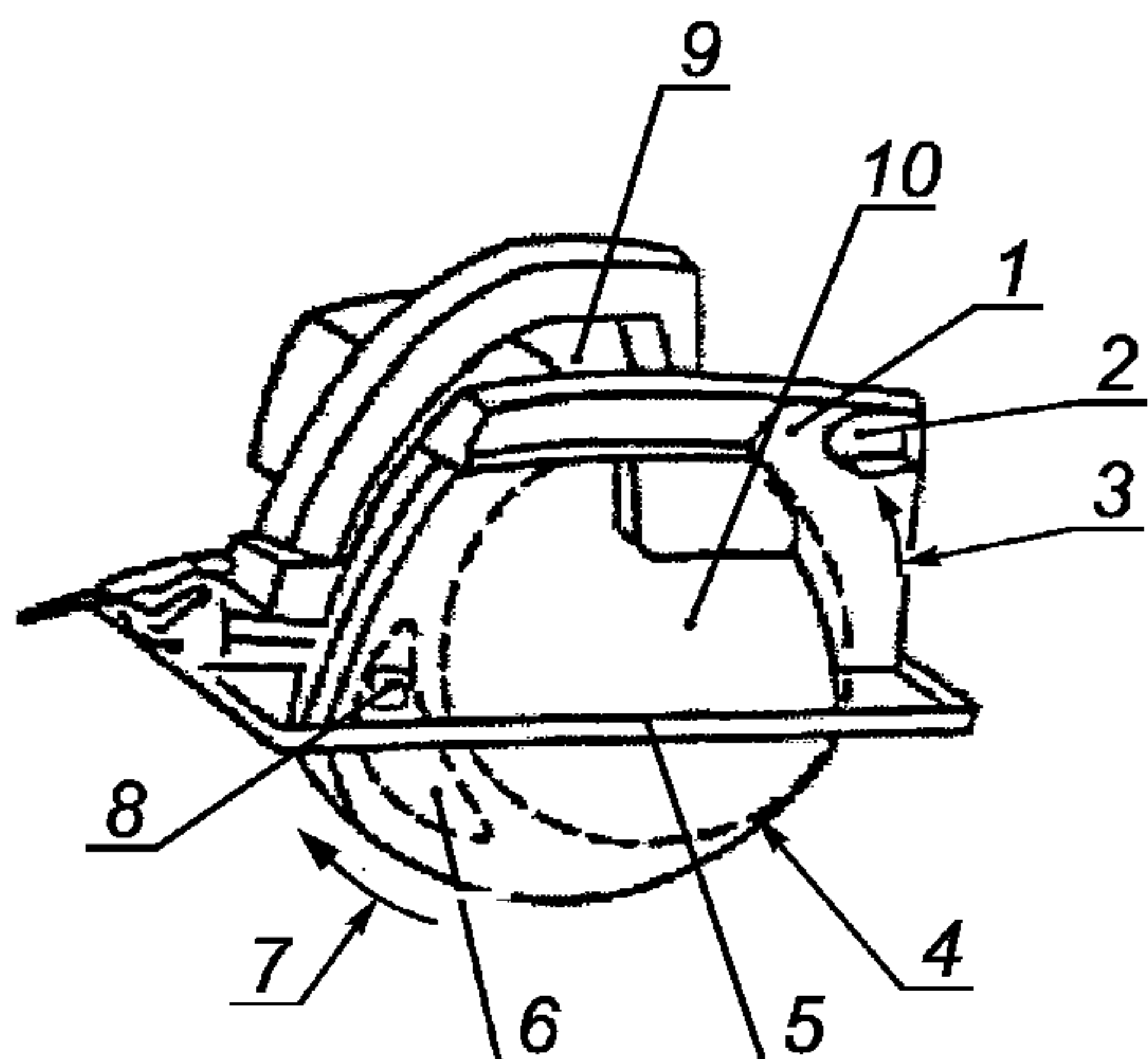
Рисунок 101 — Дисковая пила с наружным качающимся защитным кожухом
