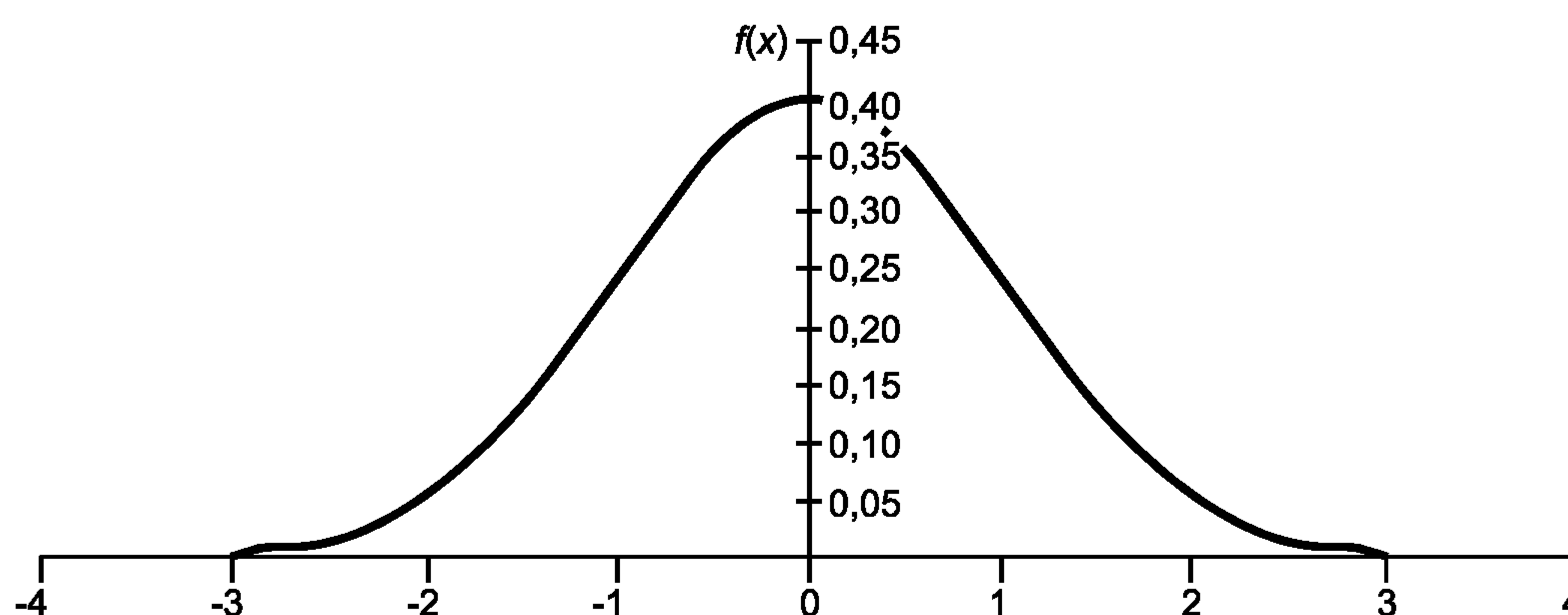
Рисунок Б.3 — Функция плотности нормального распределения
