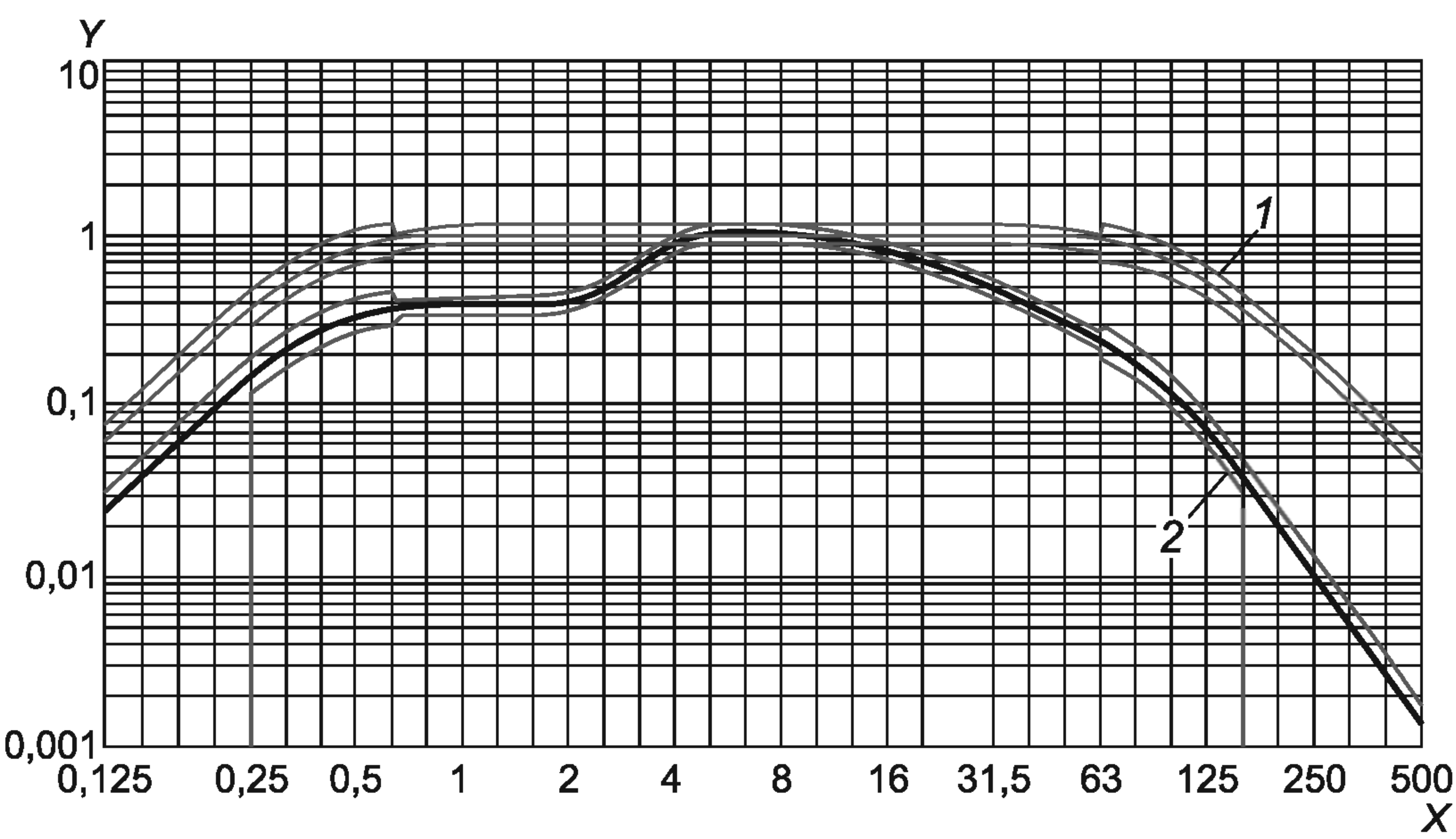
X — частота, Гц; Y — весовой коэффициент; 1 — полосовой фильтр; 2 — функция частотной коррекции
