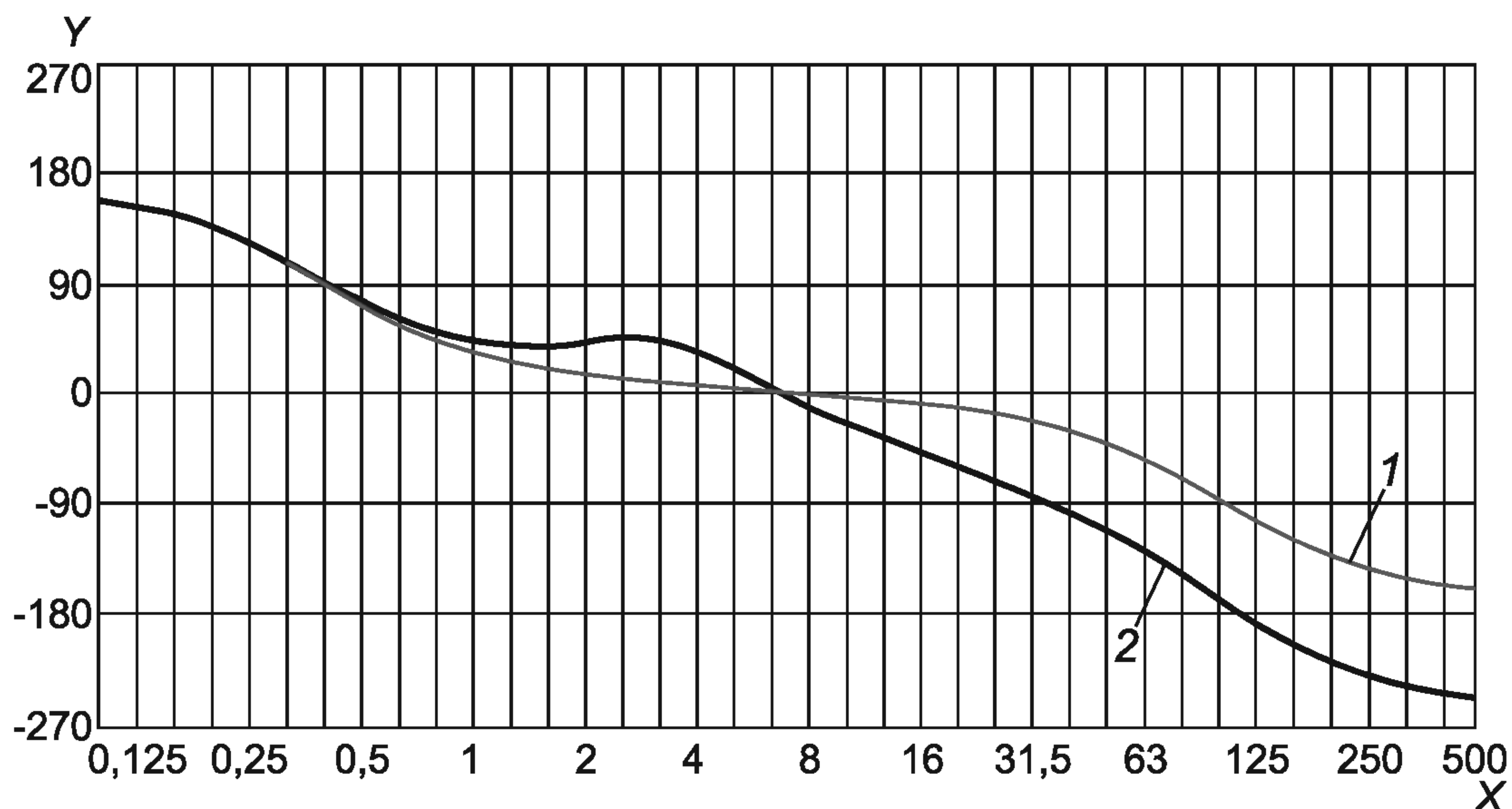
Рисунок В.2 — Фаза функции частотной коррекции W_b
