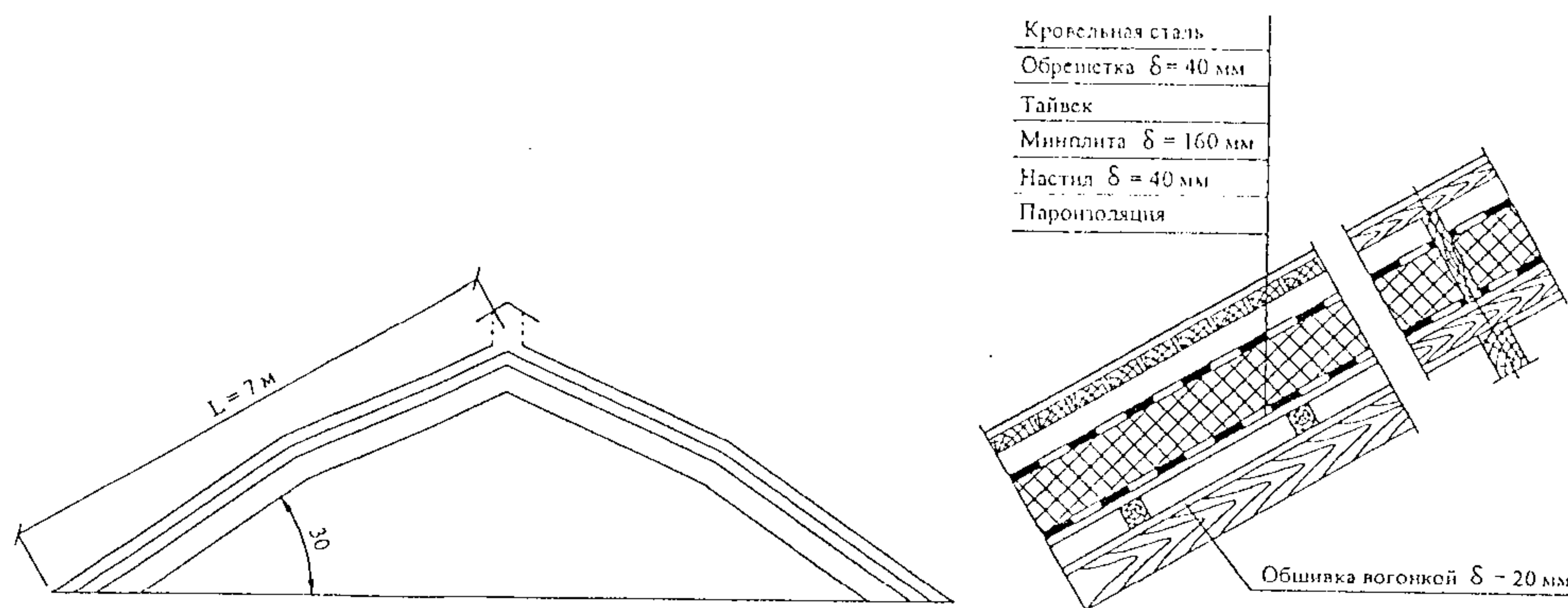
Конструктивное решение покрытия мансарды
