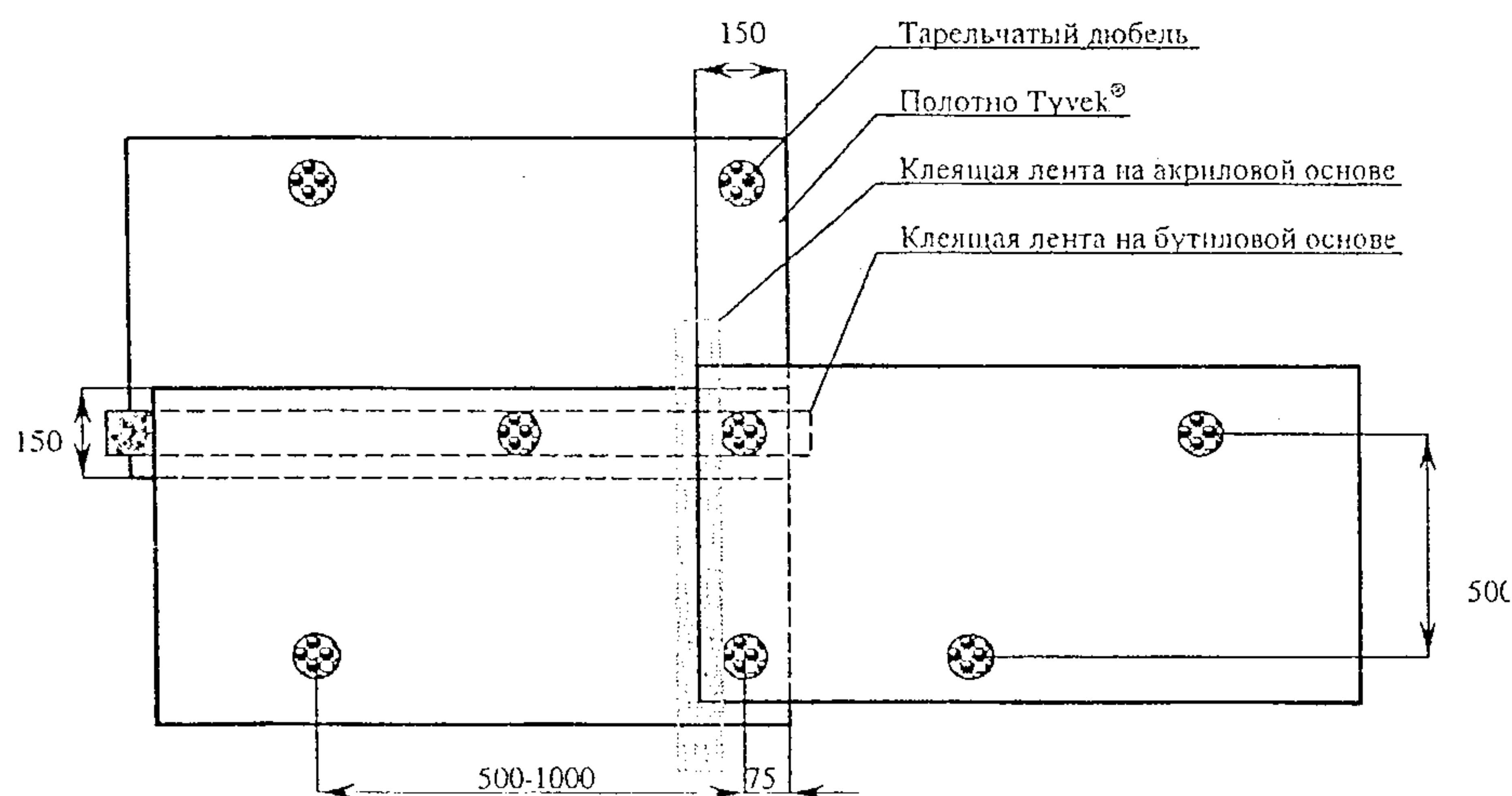
СХЕМА ЗАКРЕПЛЕНИЯ МАТЕРИАЛА «ТАЙВЕК»
