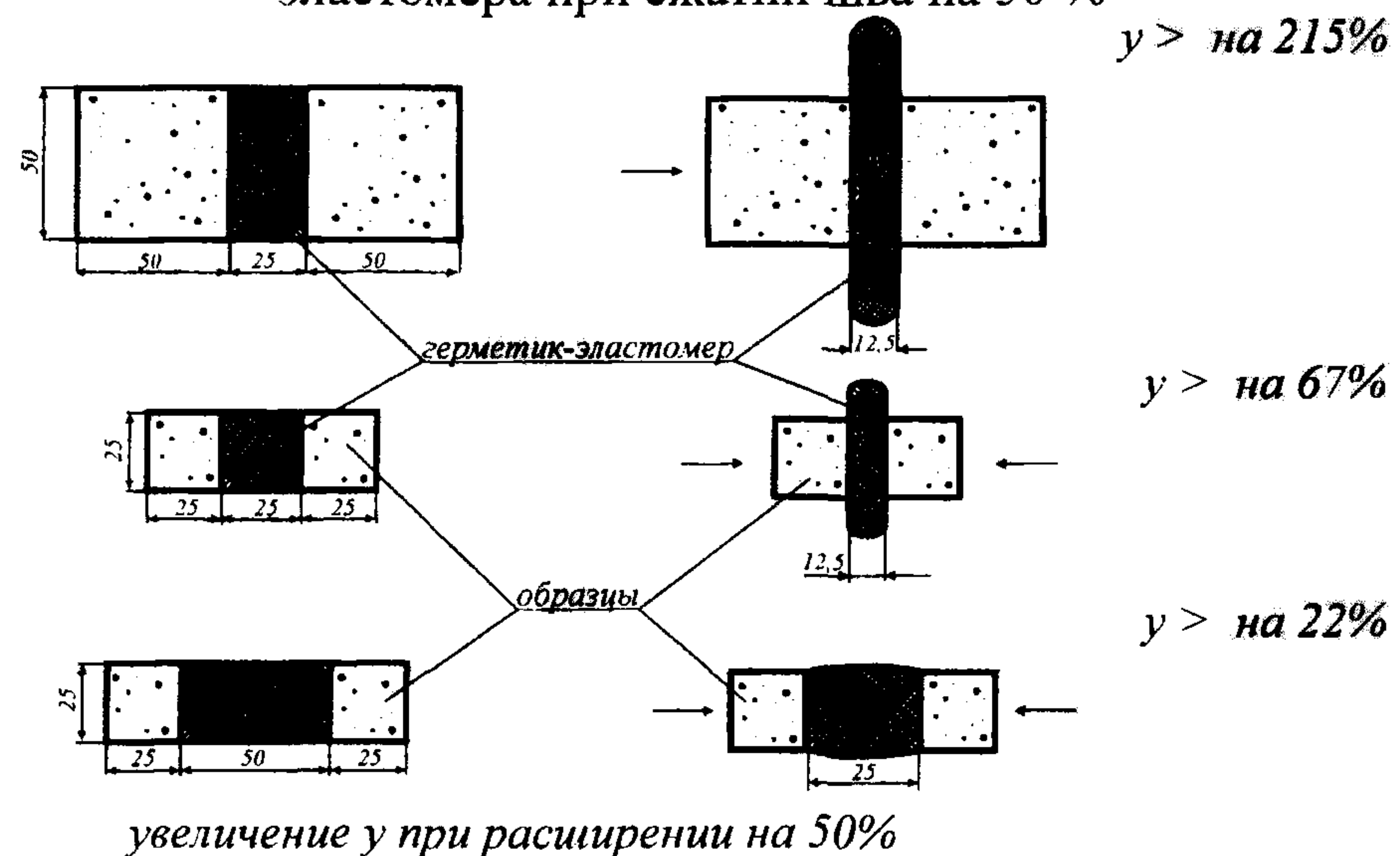
Рис. 1.2. Деформации герметиков при различных соотношениях толщины герметика ( h ) к ширине ( b_w ).
