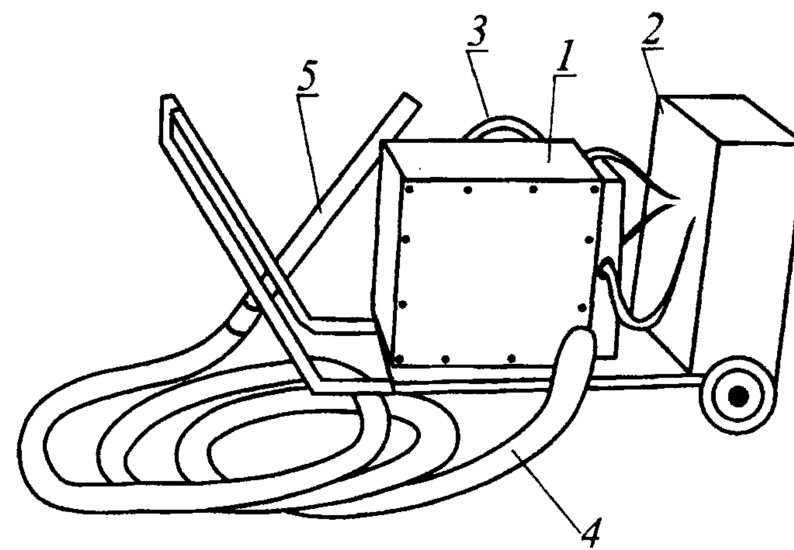
Рис. 6.4. Схема механизма СКБ Мосстроя для сушки стыков:
