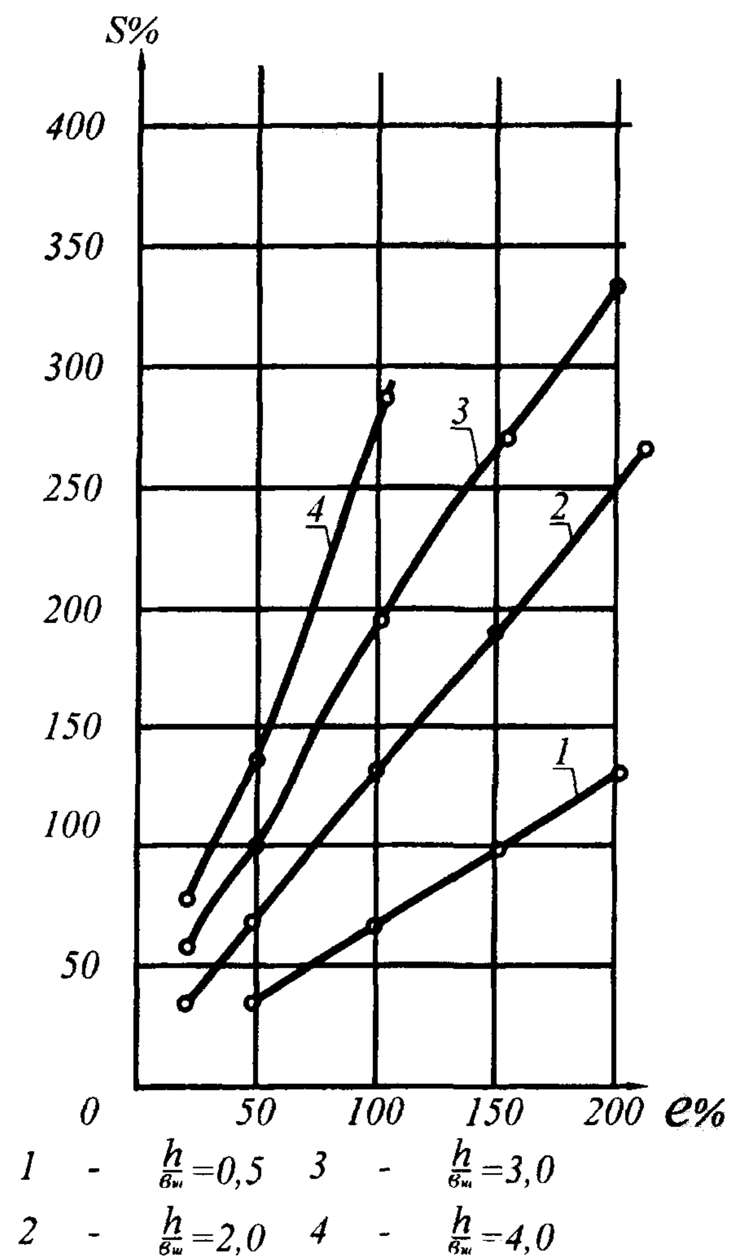
Рис. 1.2. Деформации герметиков при различных соотношениях толщины герметика ( h ) к ширине ( b_w ).
