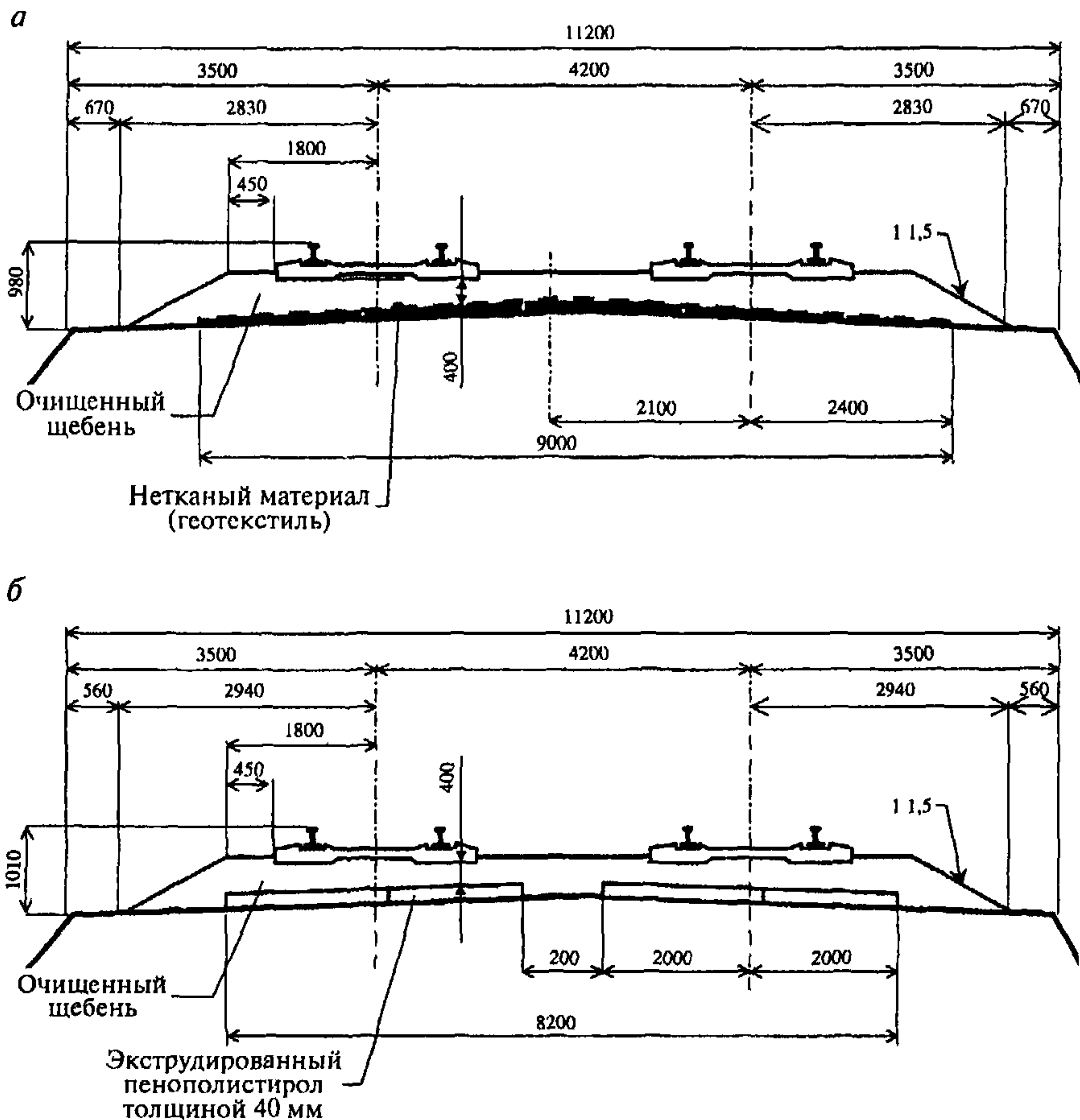
Рис. 3.2. Варианты покрытия из геотекстиля (а) и пенополистирольных плит (б) для ширины междупутья 4200 мм
