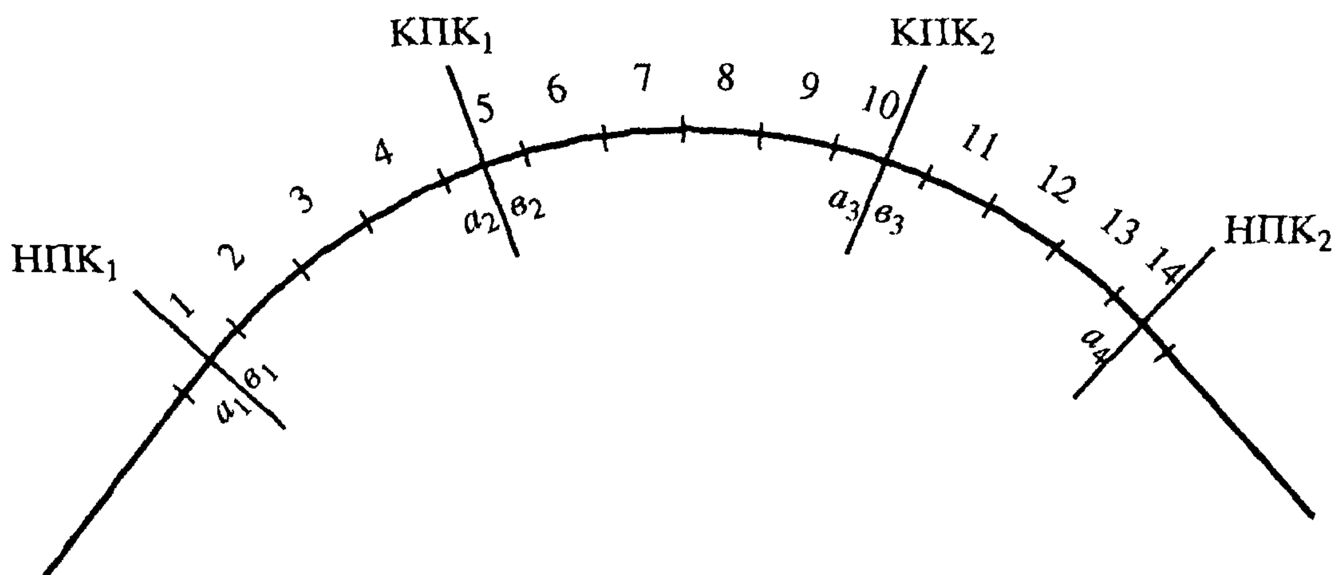
Рис. 3.1. Схема укладки укороченных рельсов в кривой
