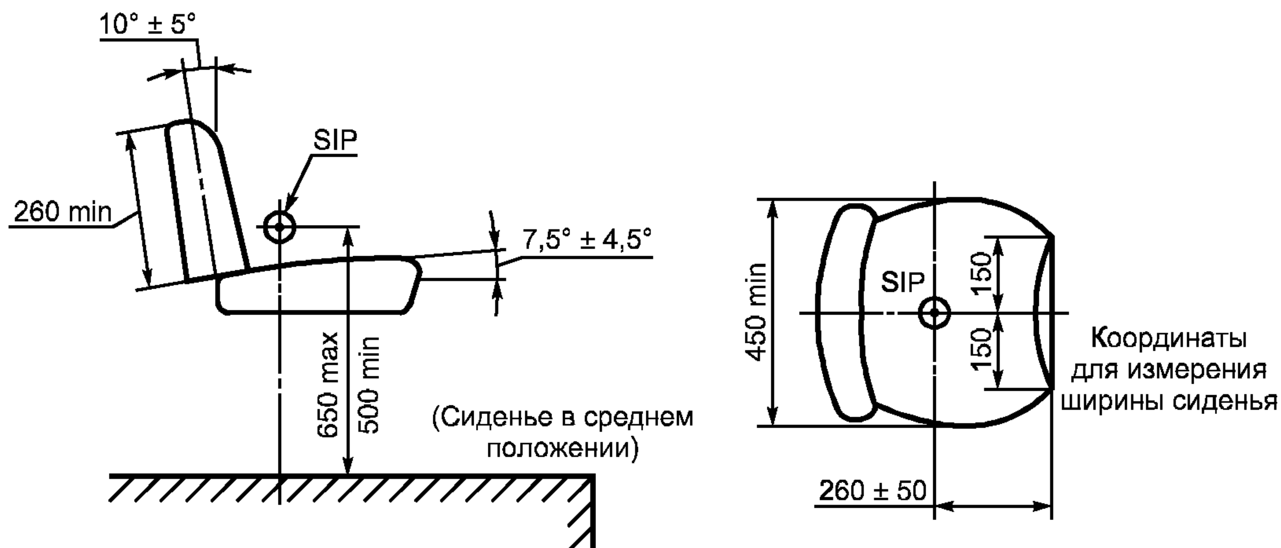
Рисунок 2 — Размеры сиденья
