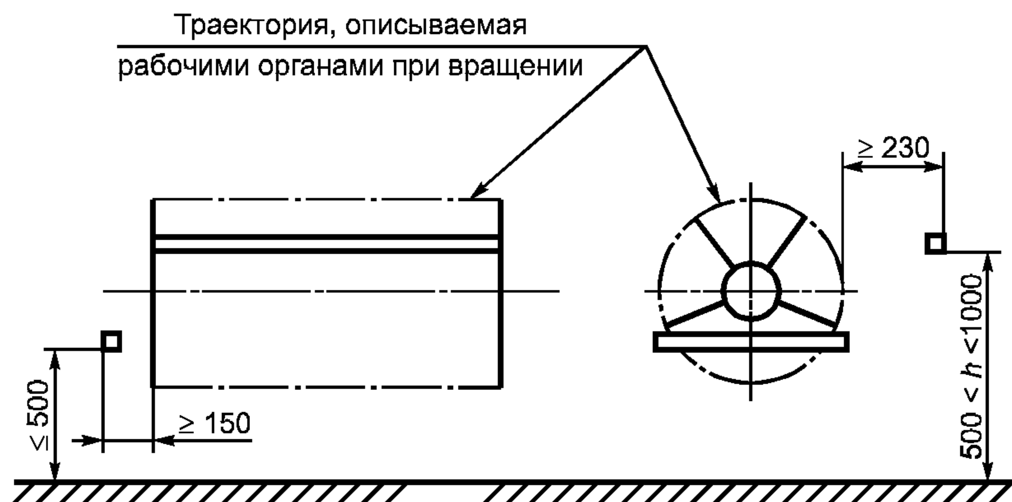
Рисунок 11 — Вращающееся подающее устройство
