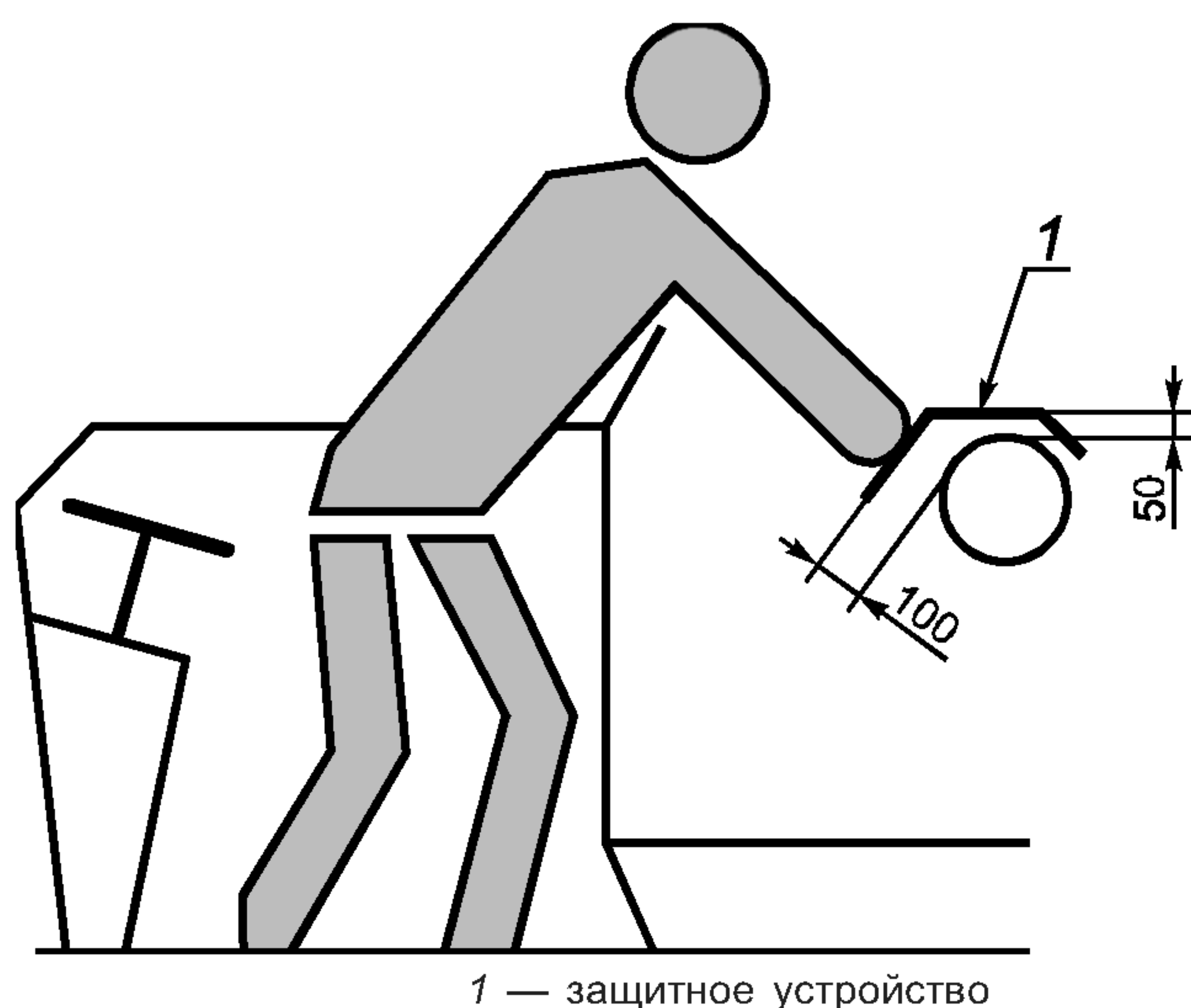
Рисунок 8 — Доступ к распределительному шнеку
