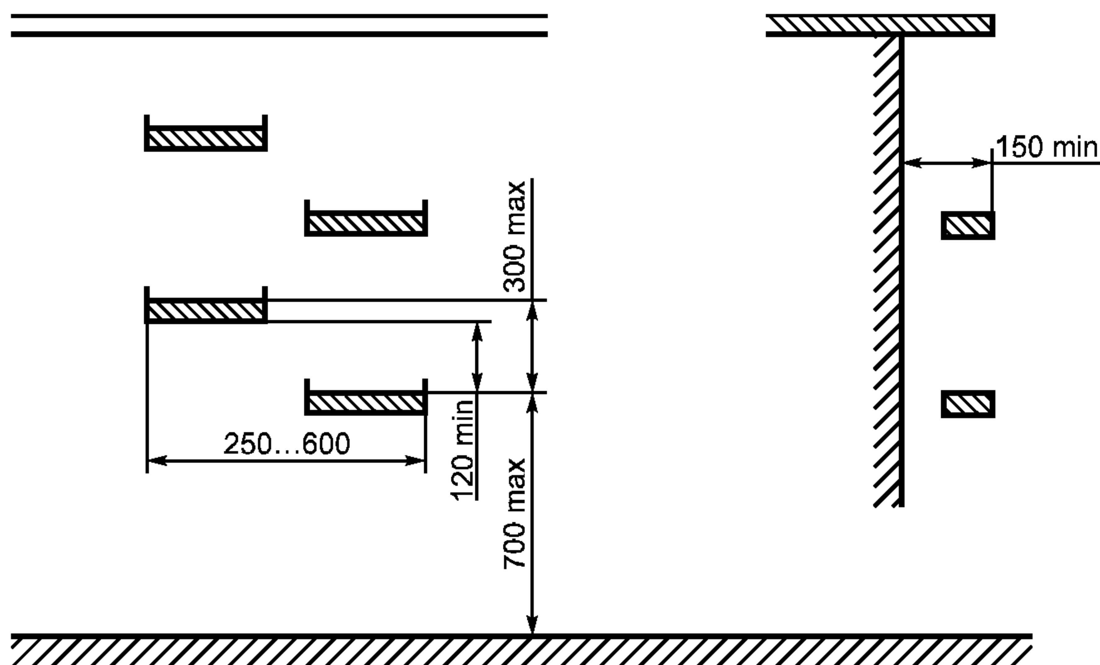
Рисунок 7 — Другие средства доступа и места обслуживания
