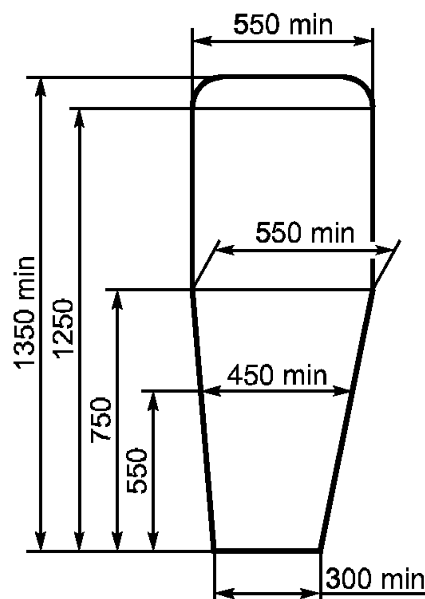
Рисунок 5 — Основные размеры дверного проема
