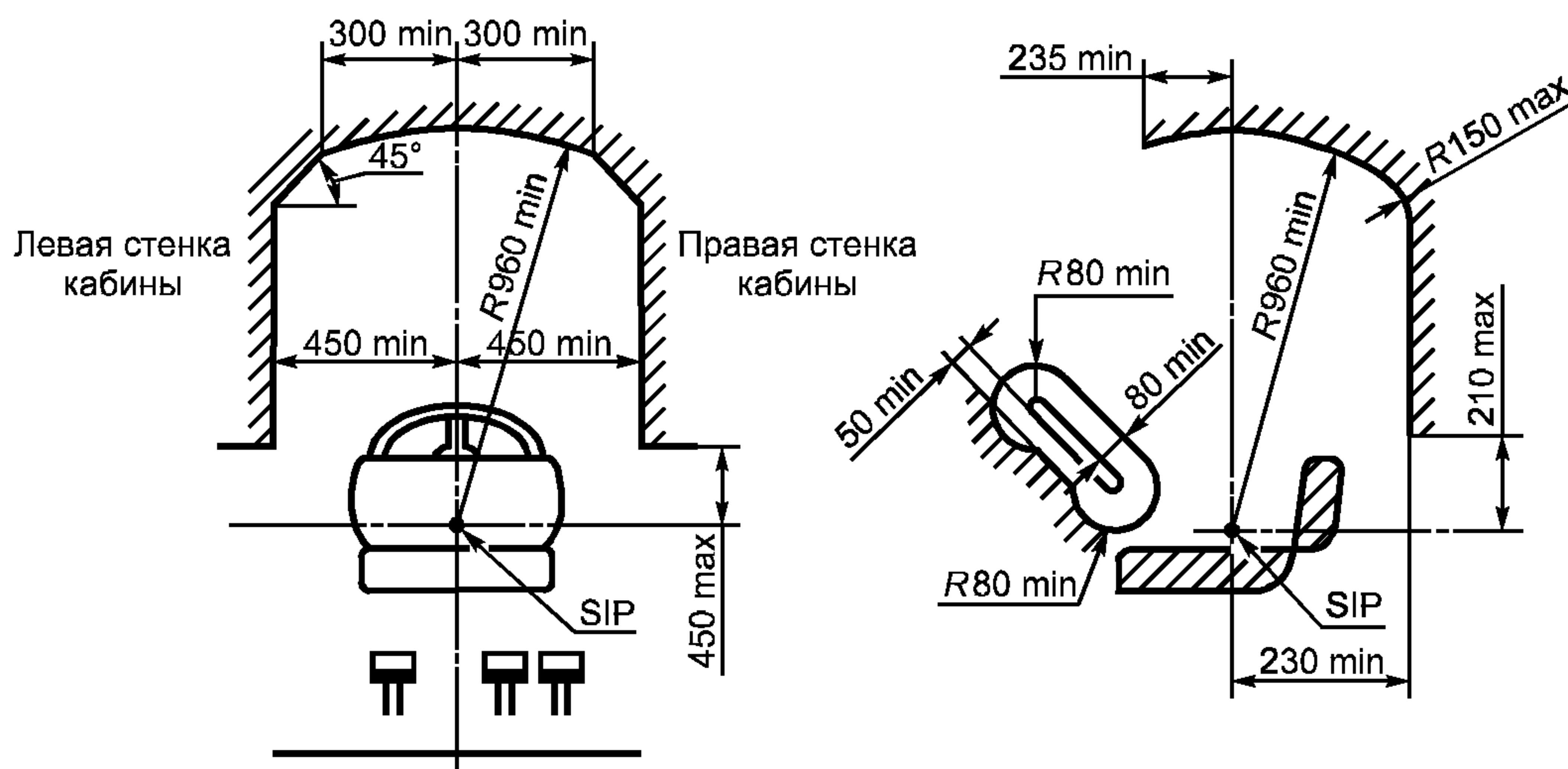
Рисунок 6 — Размеры внутреннего рабочего пространства
