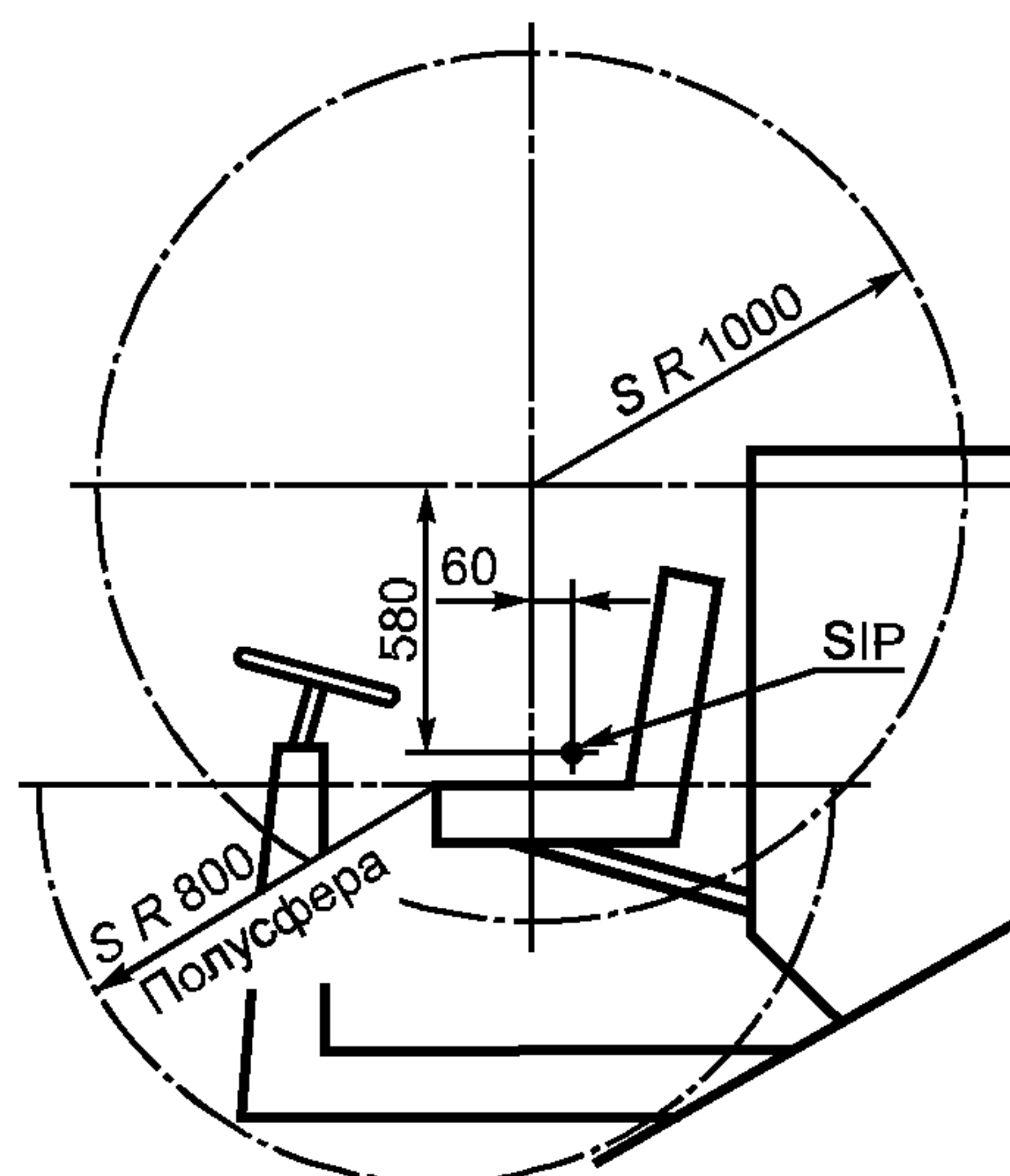
Рисунок 3 — Зоны досягаемости рук и ног
