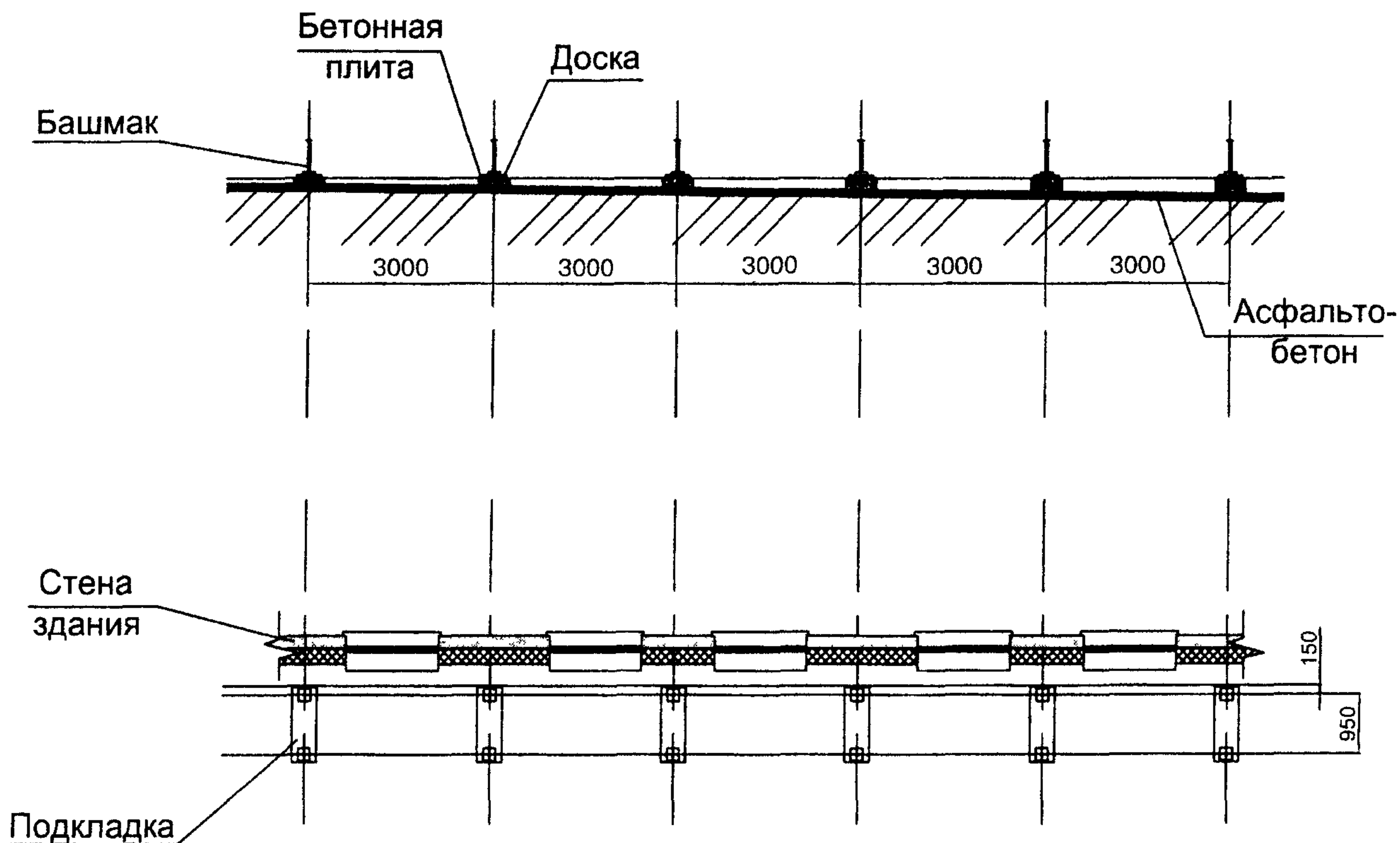
Рис. 3. Установка башмаков
