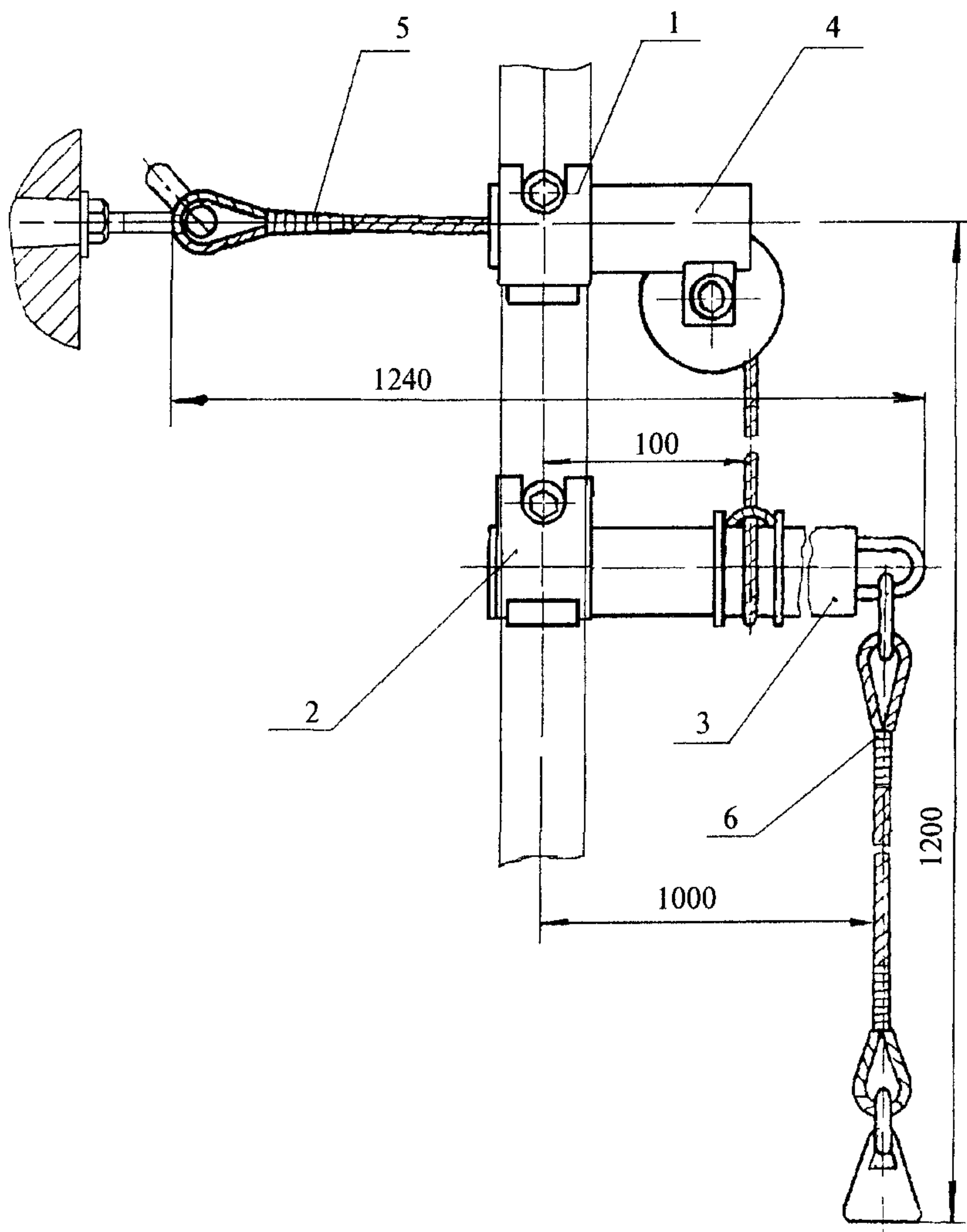
Приспособление для контроля заклинивания пробок
