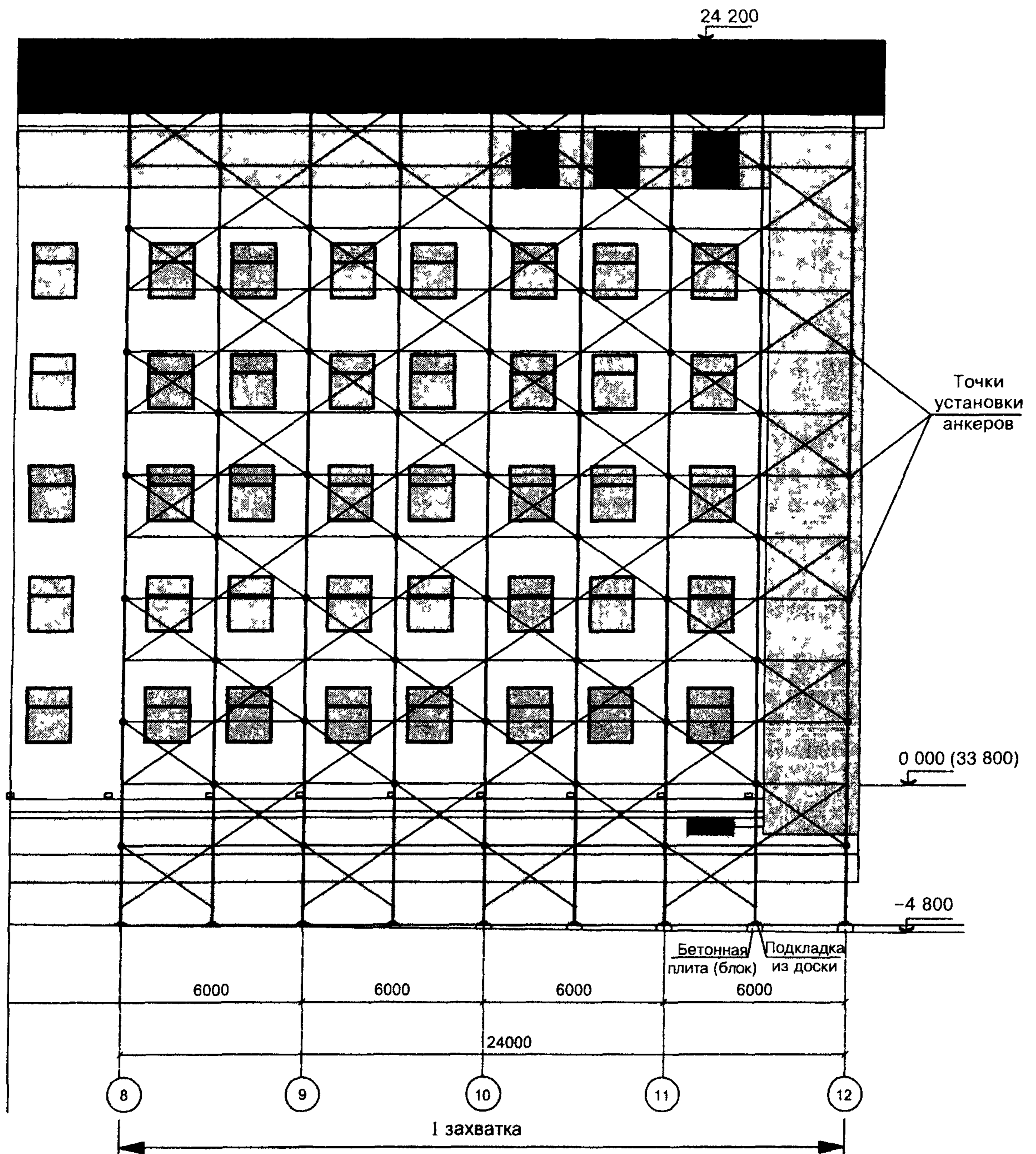
Рис. 2. Расположение лесов на первой захватке
