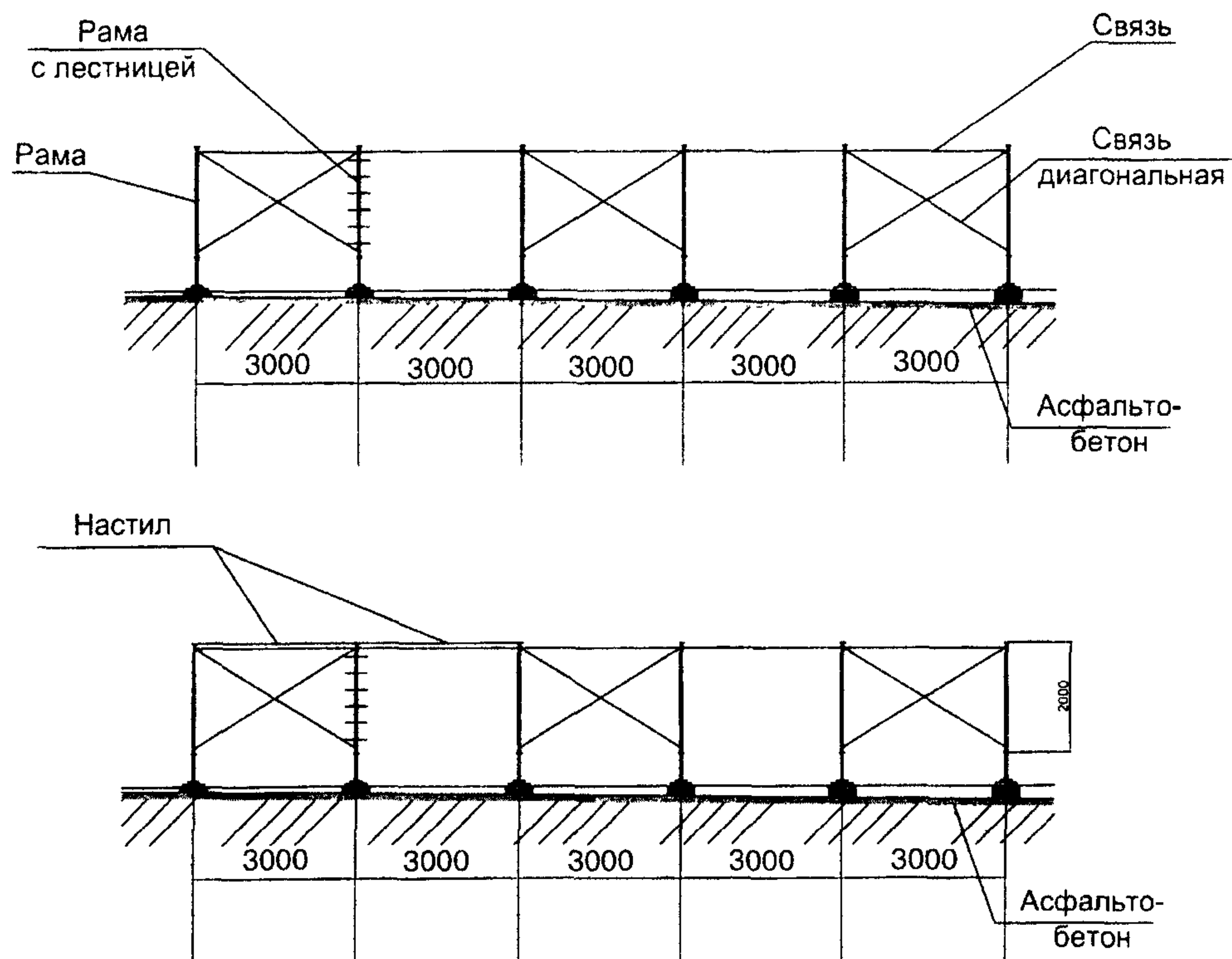
Рис. 4. Сборка первого яруса лесов
