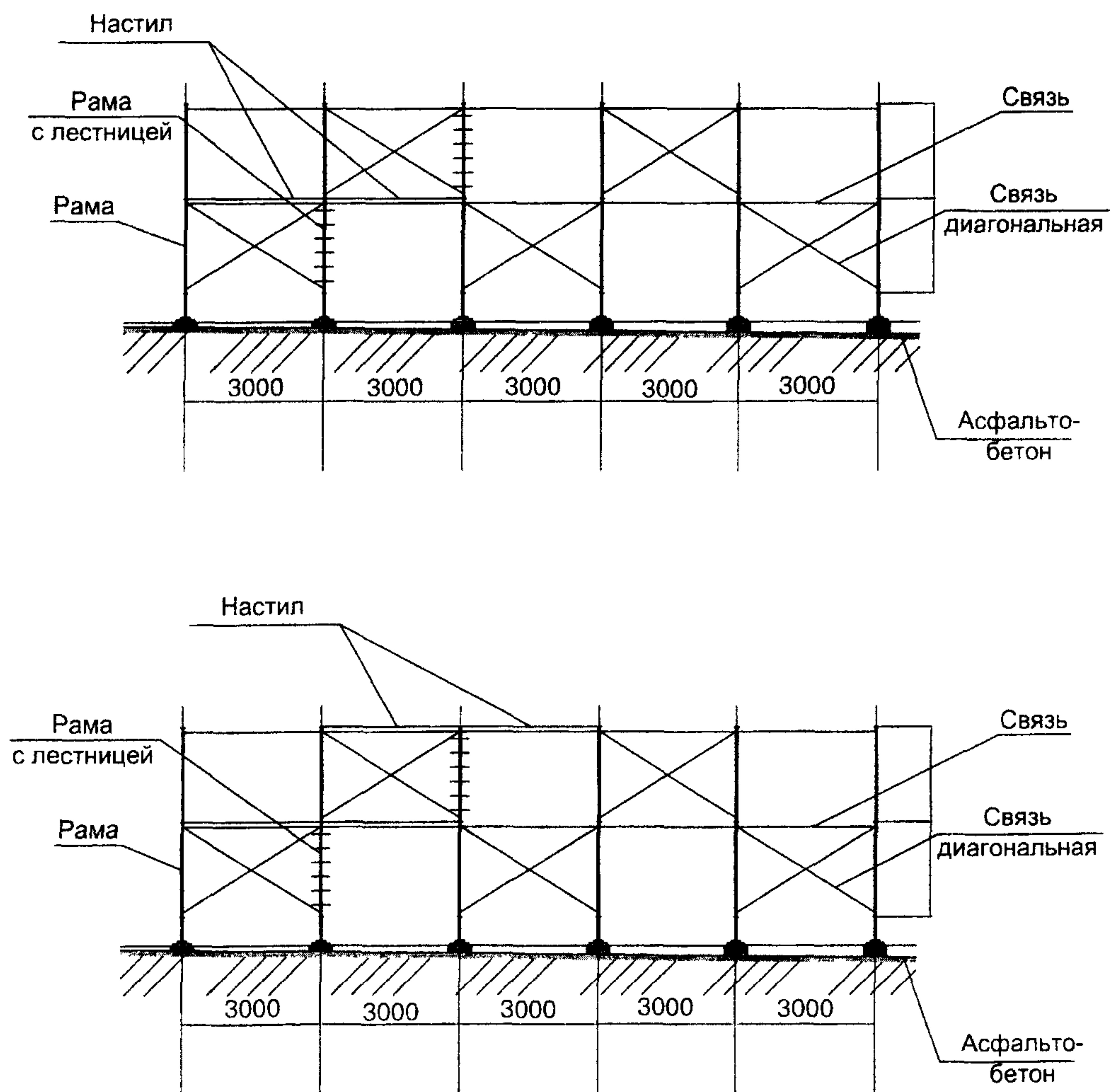
Рис. 5. Сборка второго яруса лесов
