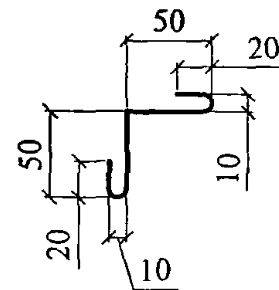
НАЩЕЛЬНИК Н4
