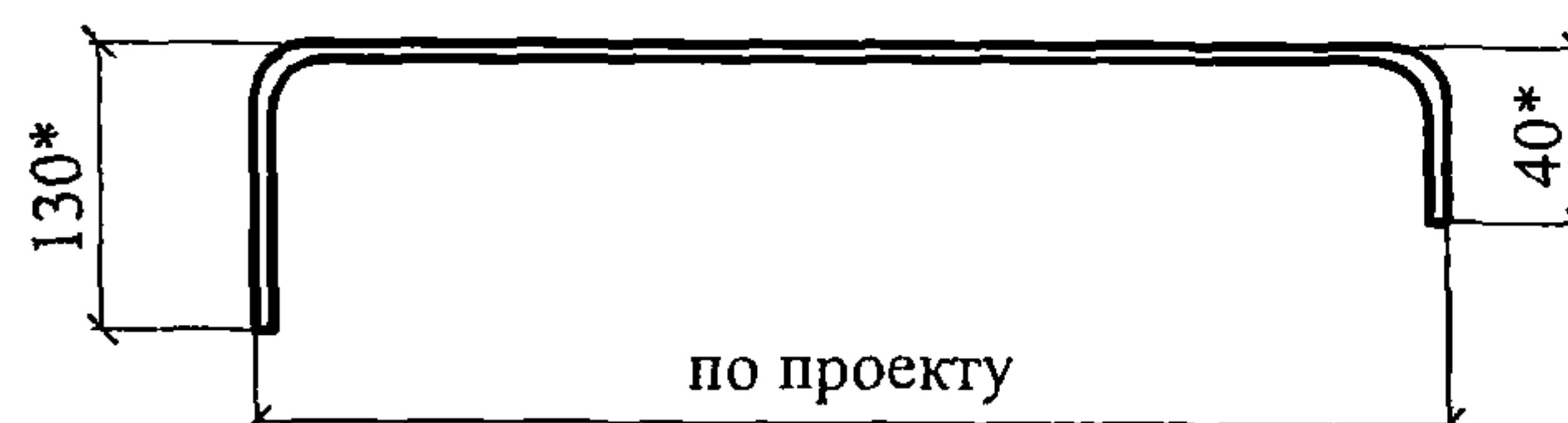
КОСТЫЛЬ К4
