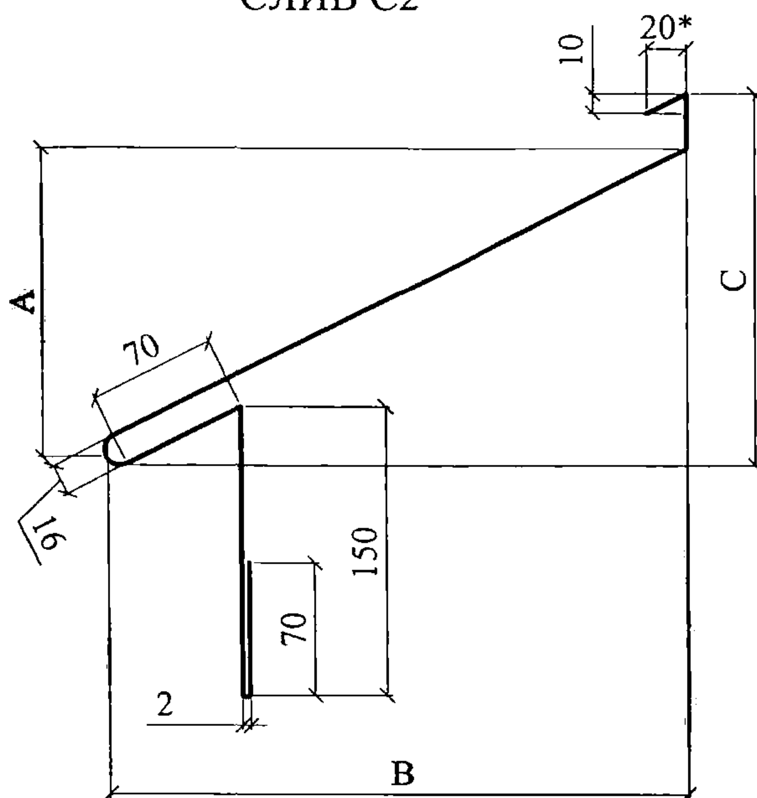
СЛИВ С2
