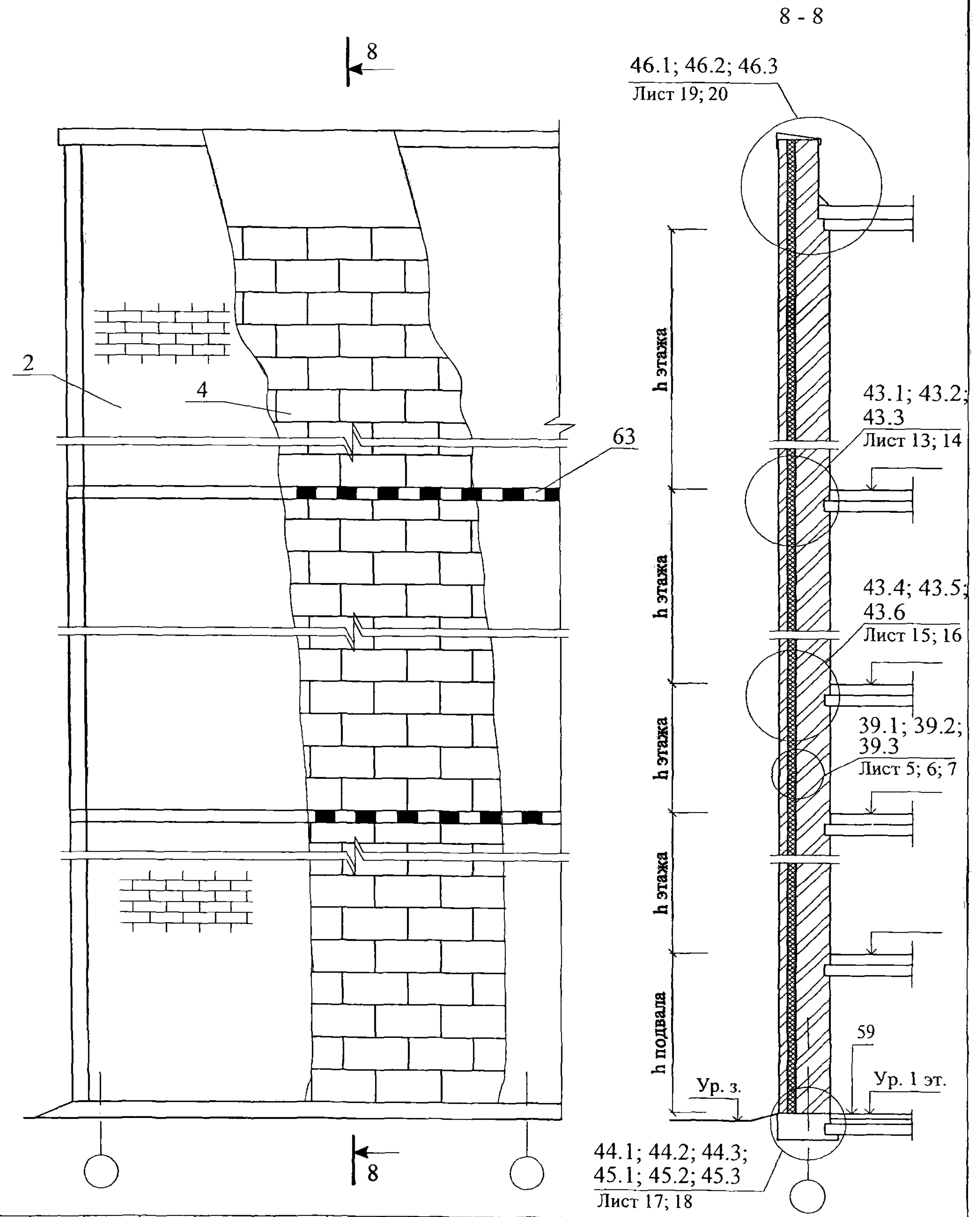
СХЕМА № 7. Расположение плит утеплителя, защитно-декоративной кладки, несущей балки-пояса
