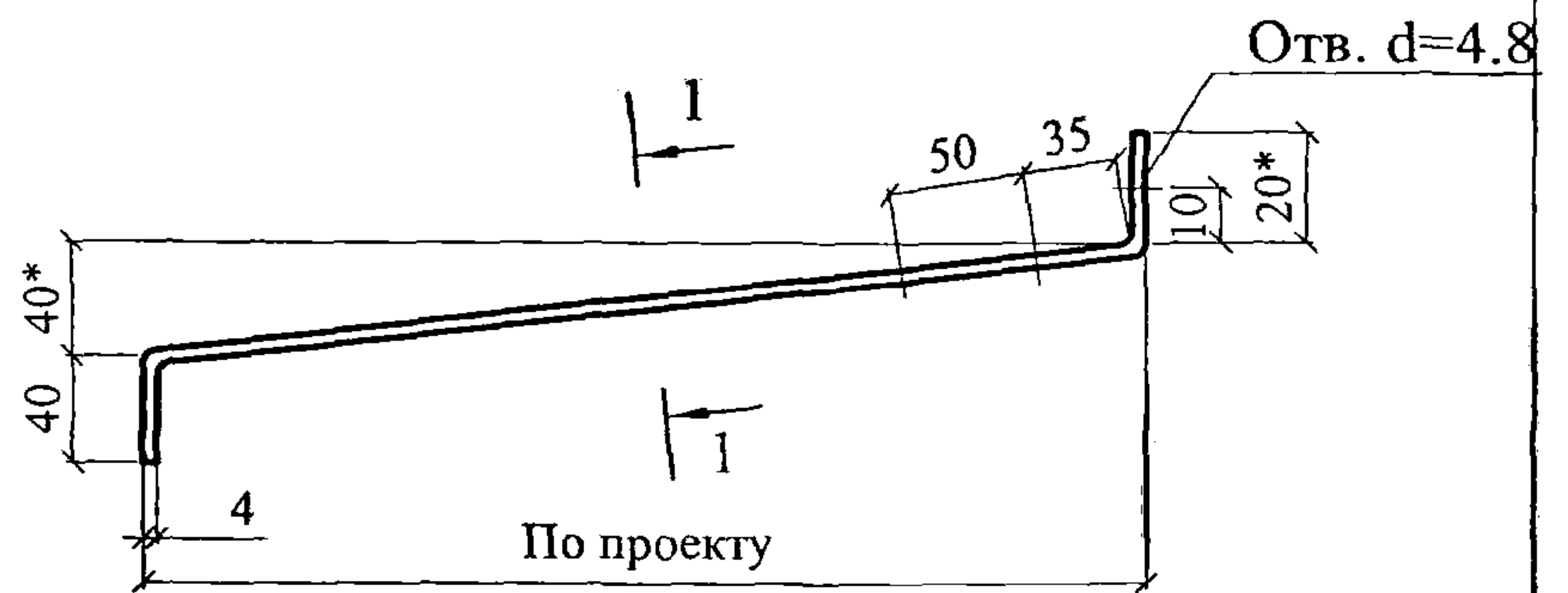
КОСТЫЛЬ К2
