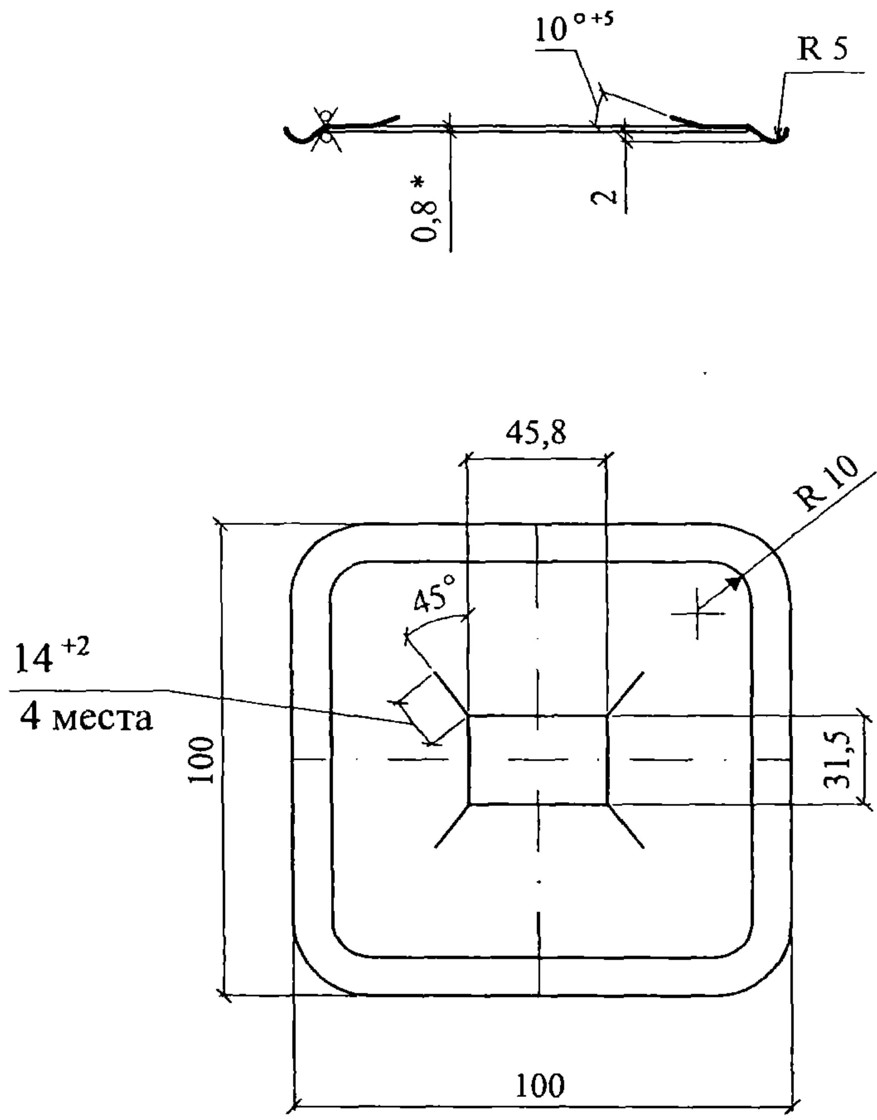
ПРИЖИМНАЯ ПЛАНКА
