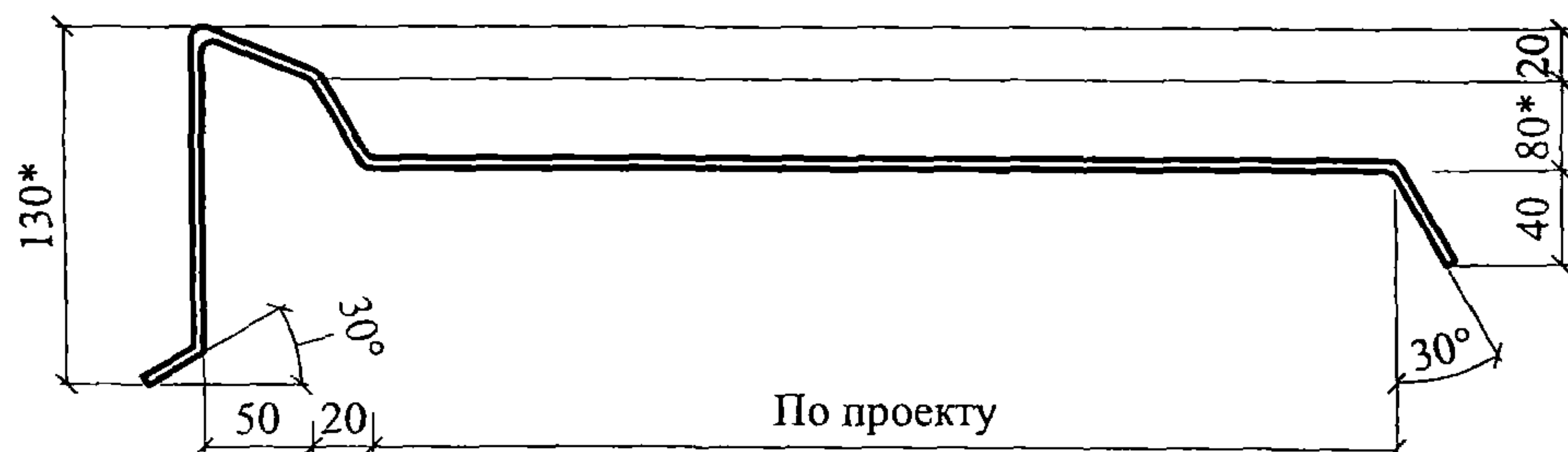
КОСТЫЛЬ К3
