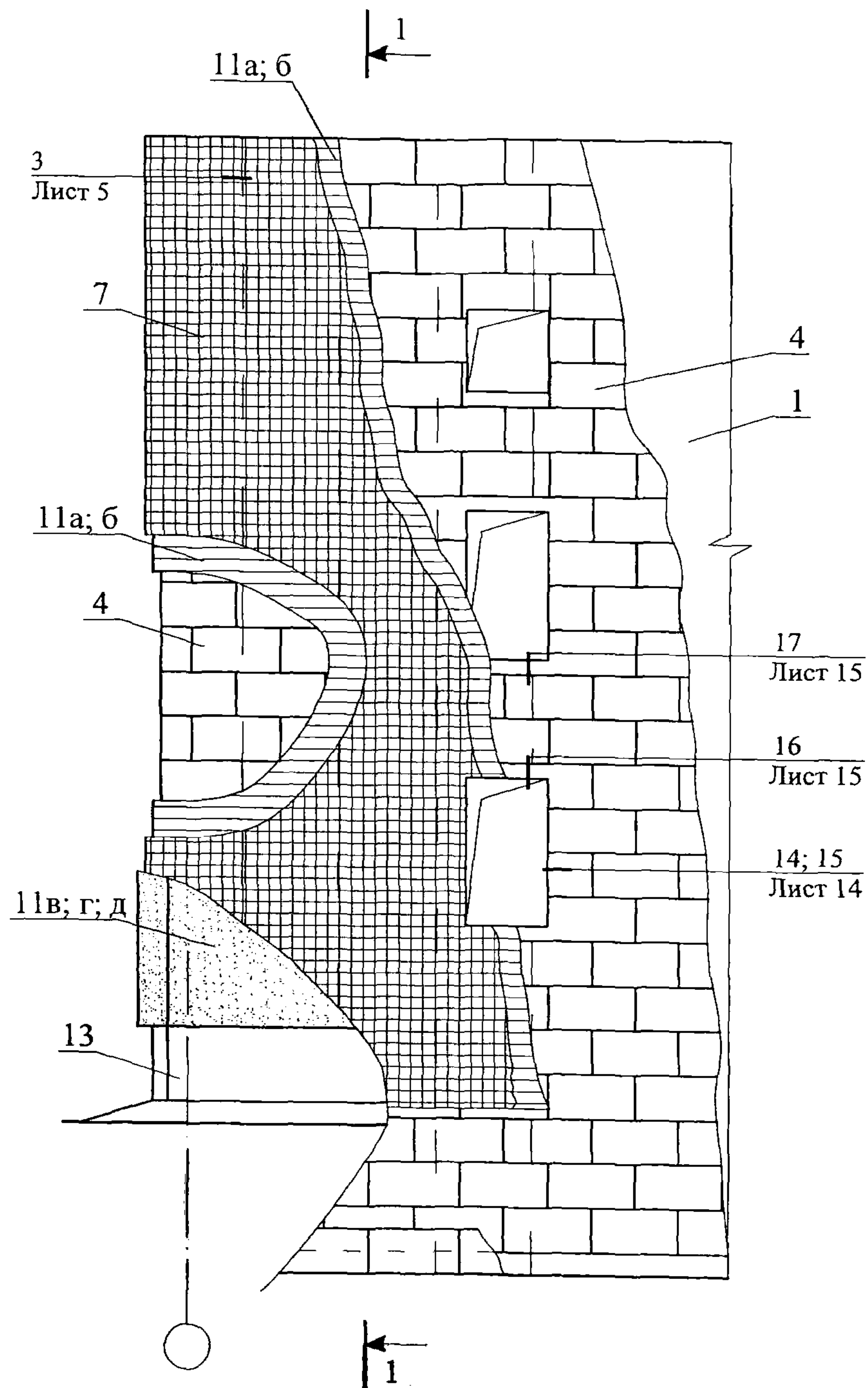
СХЕМА № 1. Расположение плит утеплителя, сетки и штукатурки
