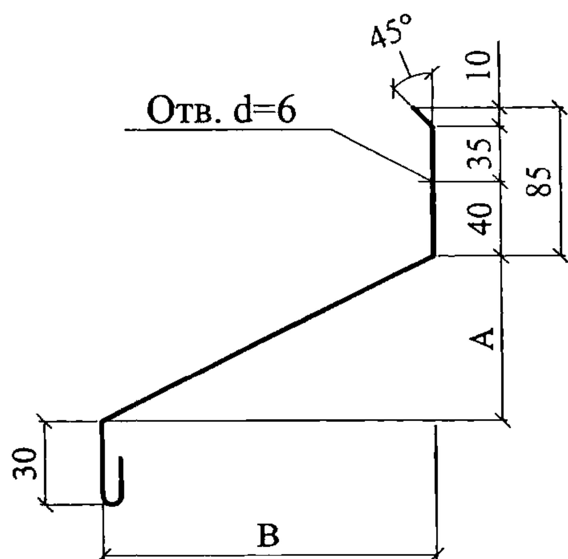
СЛИВ С3
