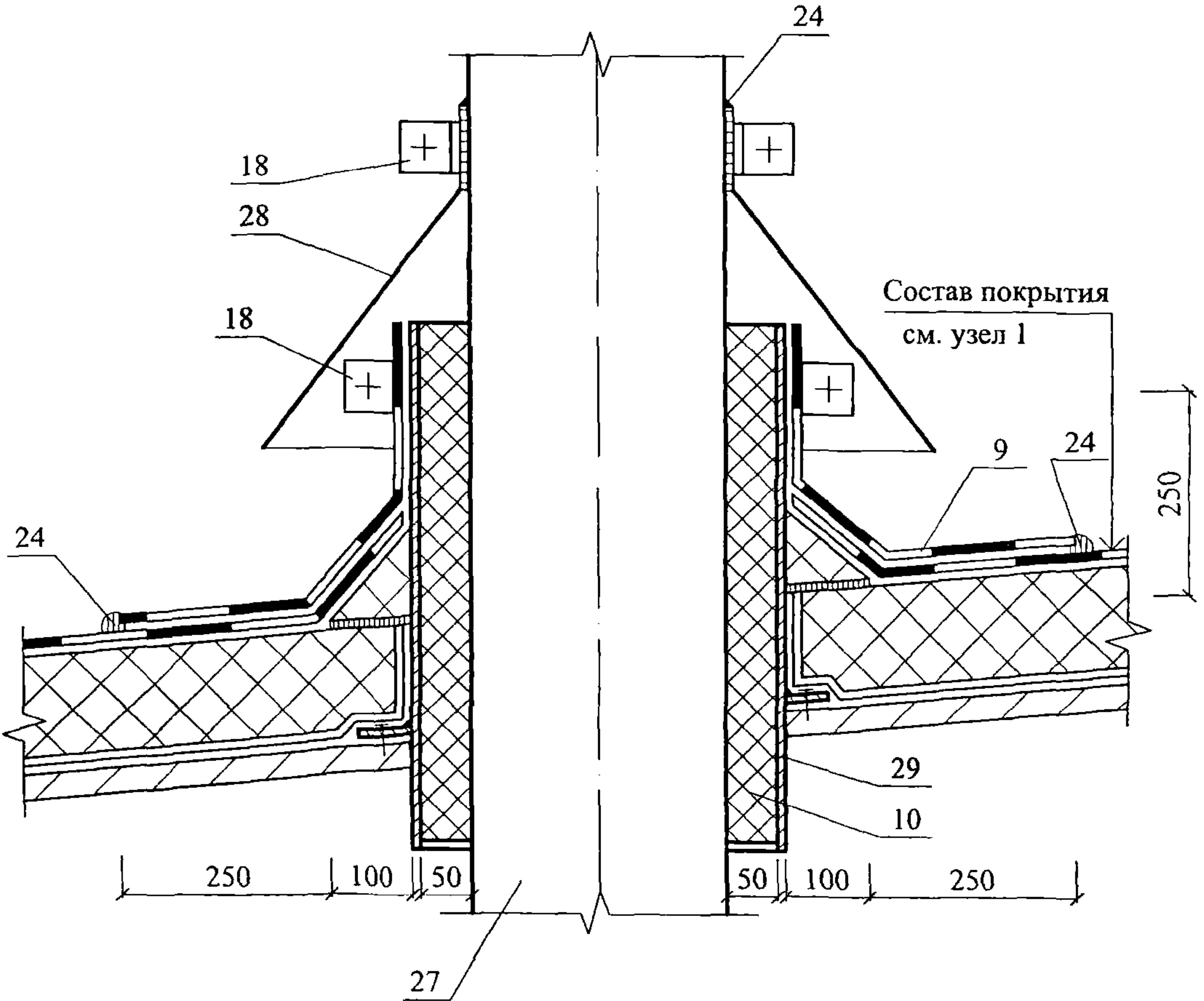
Пропуск трубы через покрытие
