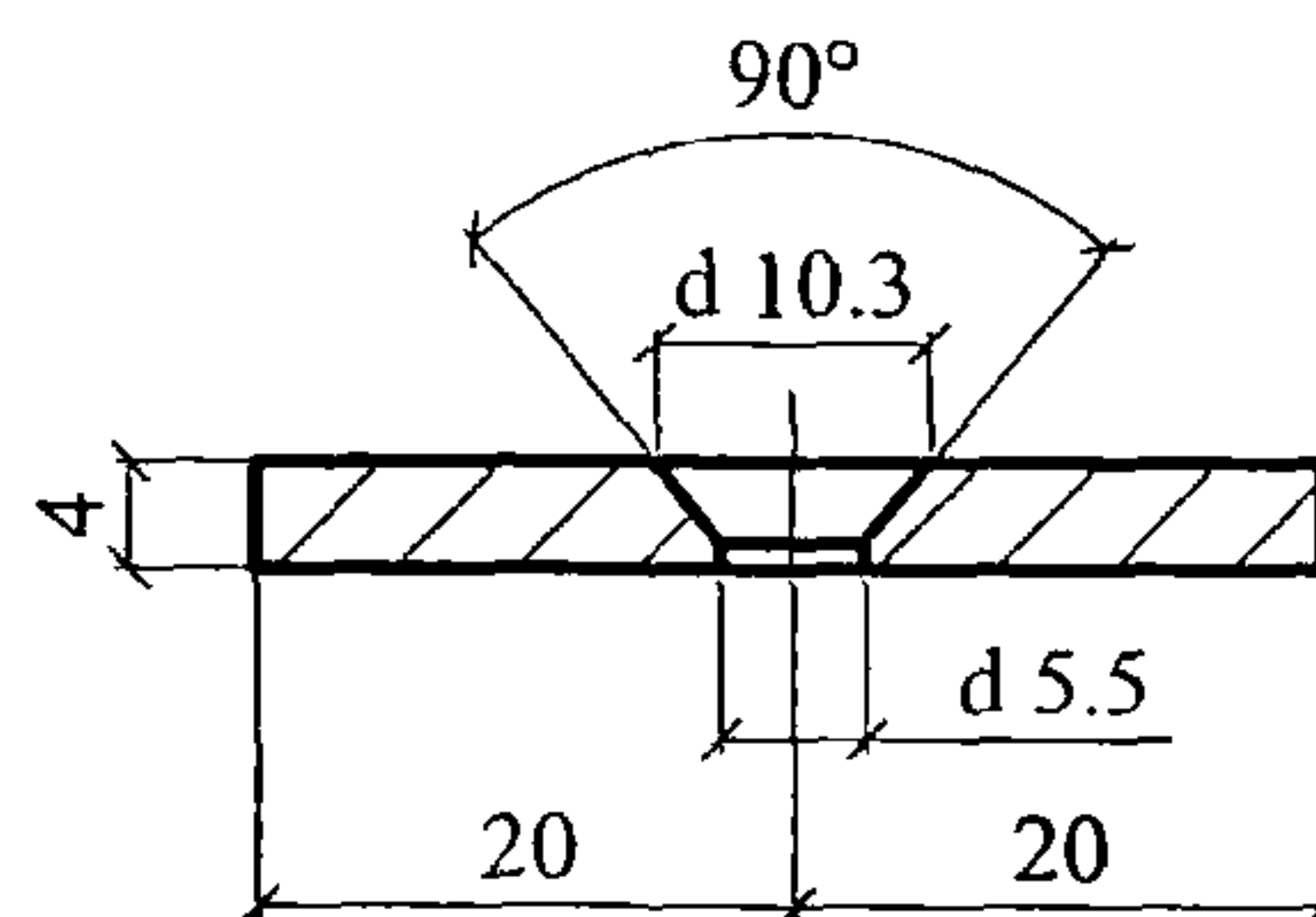
КОСТЫЛЬ К3
