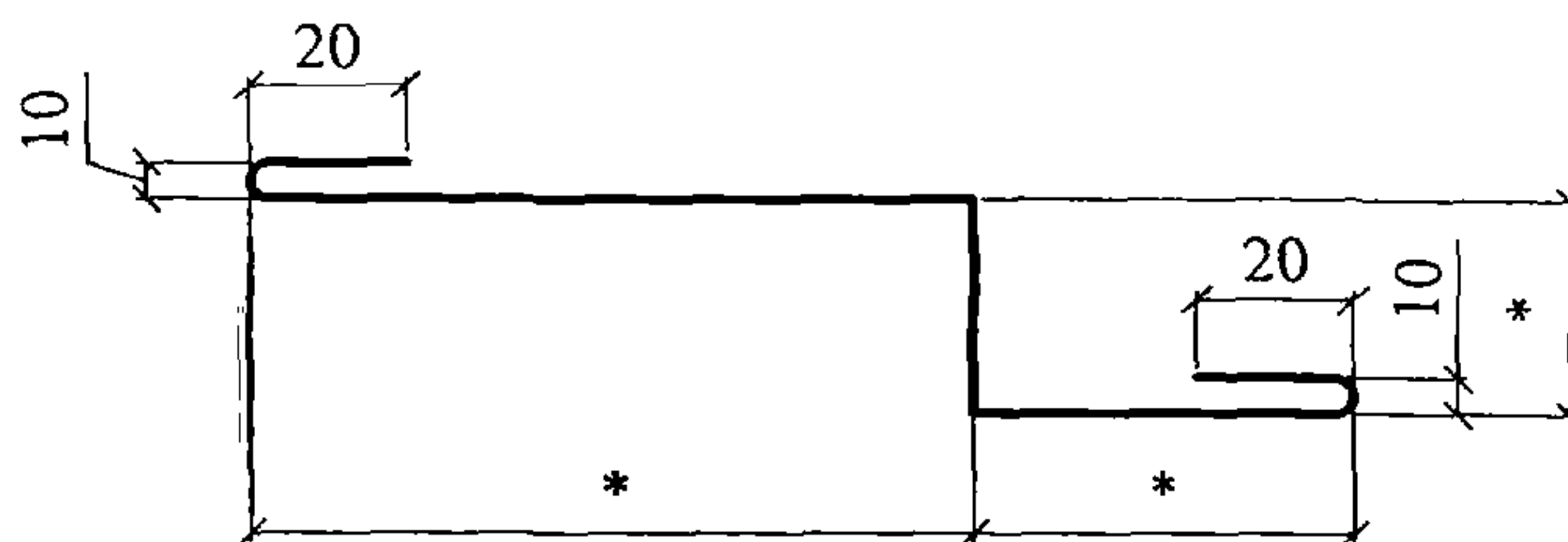
НАЩЕЛЬНИК Н3
