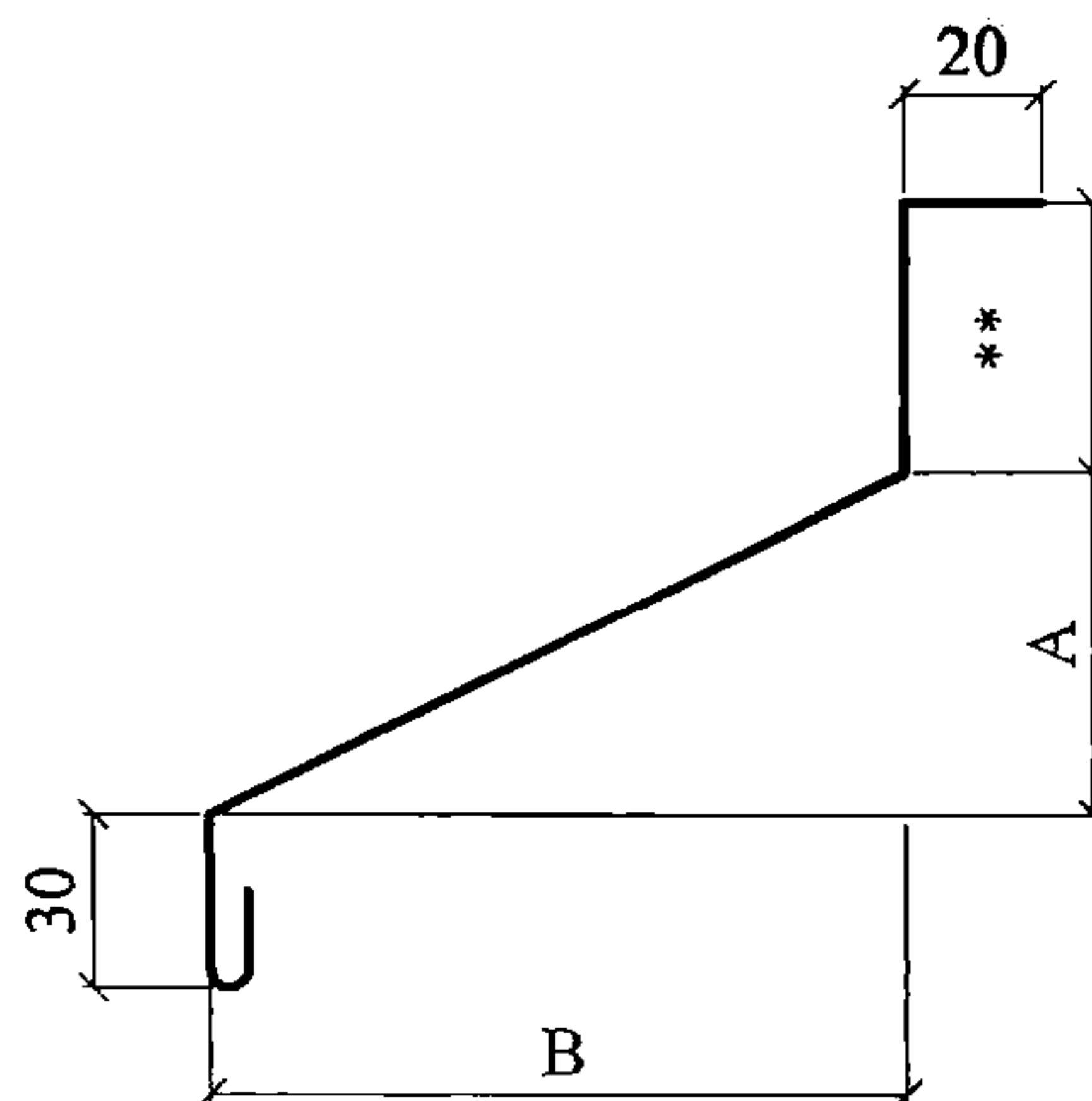
СЛИВ С5
