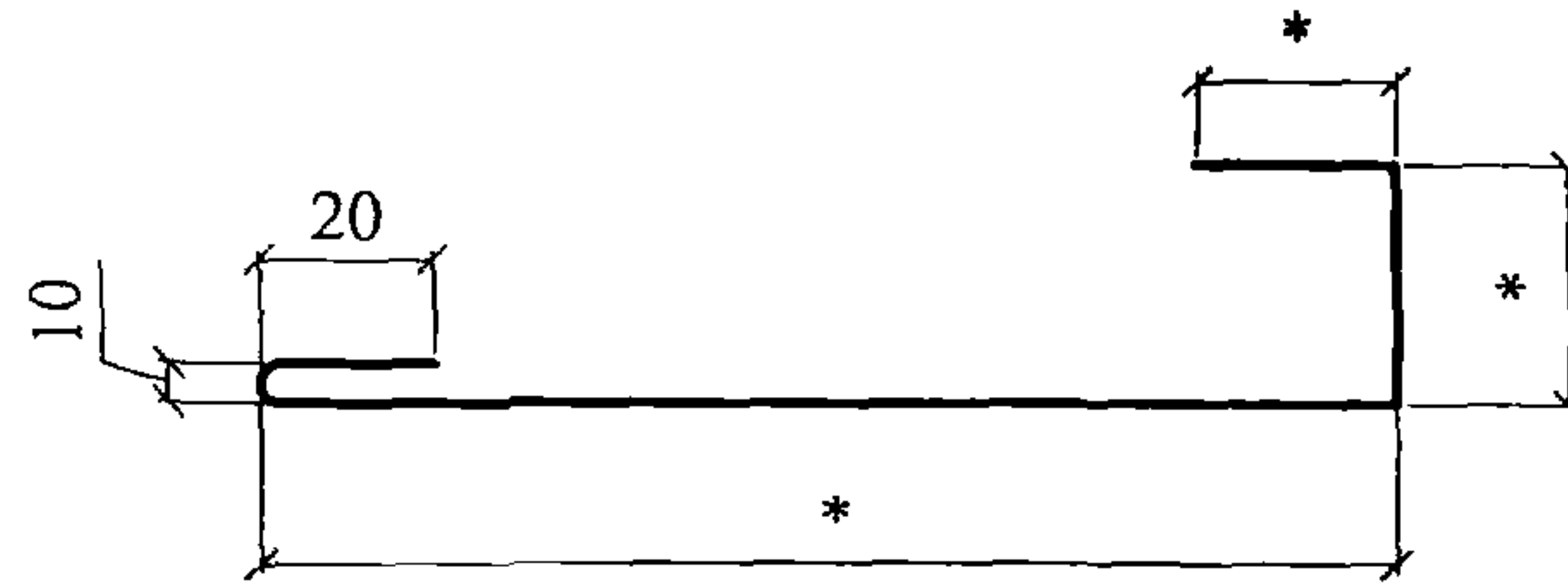
НАЩЕЛЬНИК Н2
