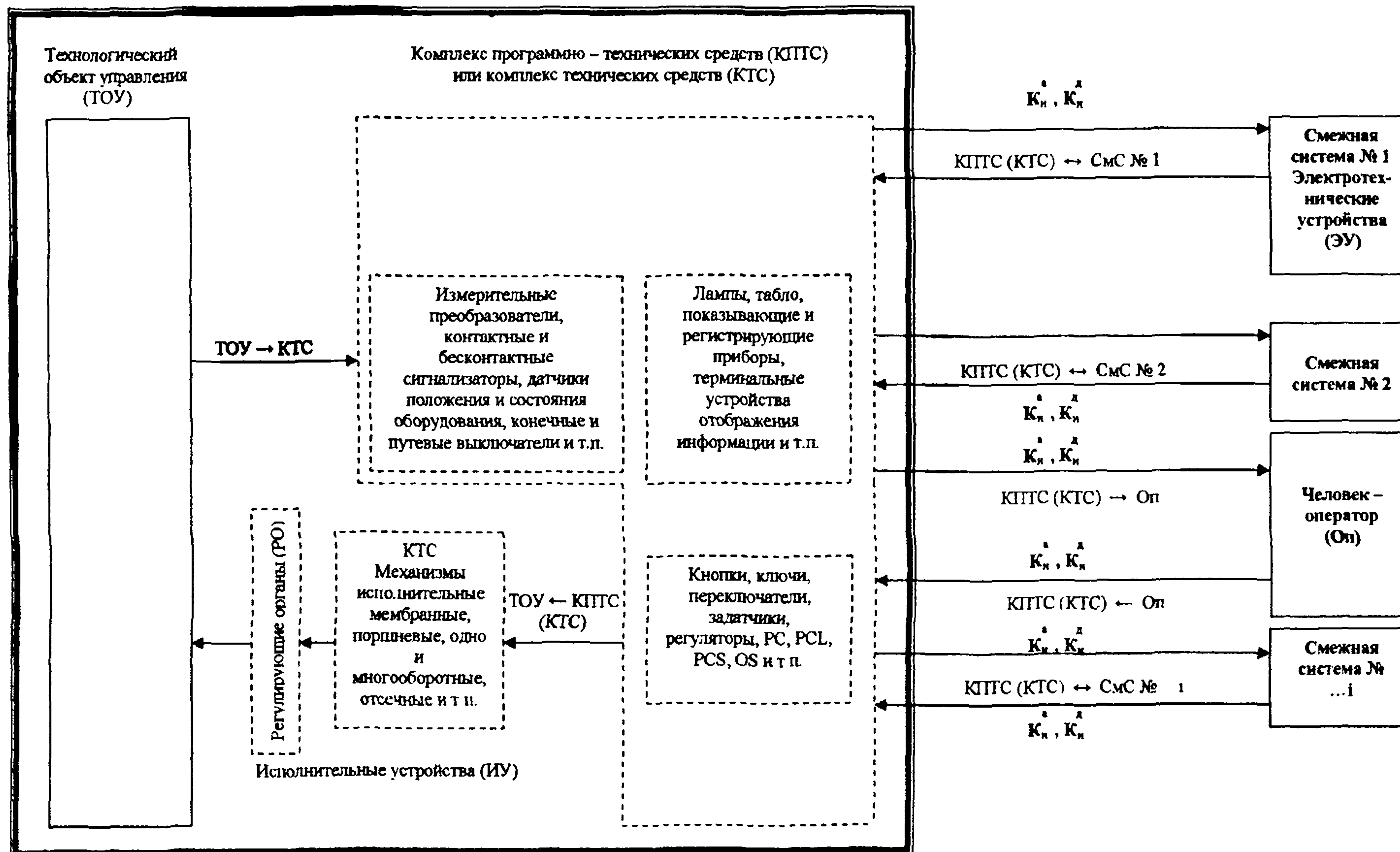
Схема автоматизированного технологического комплекса (АТК)
