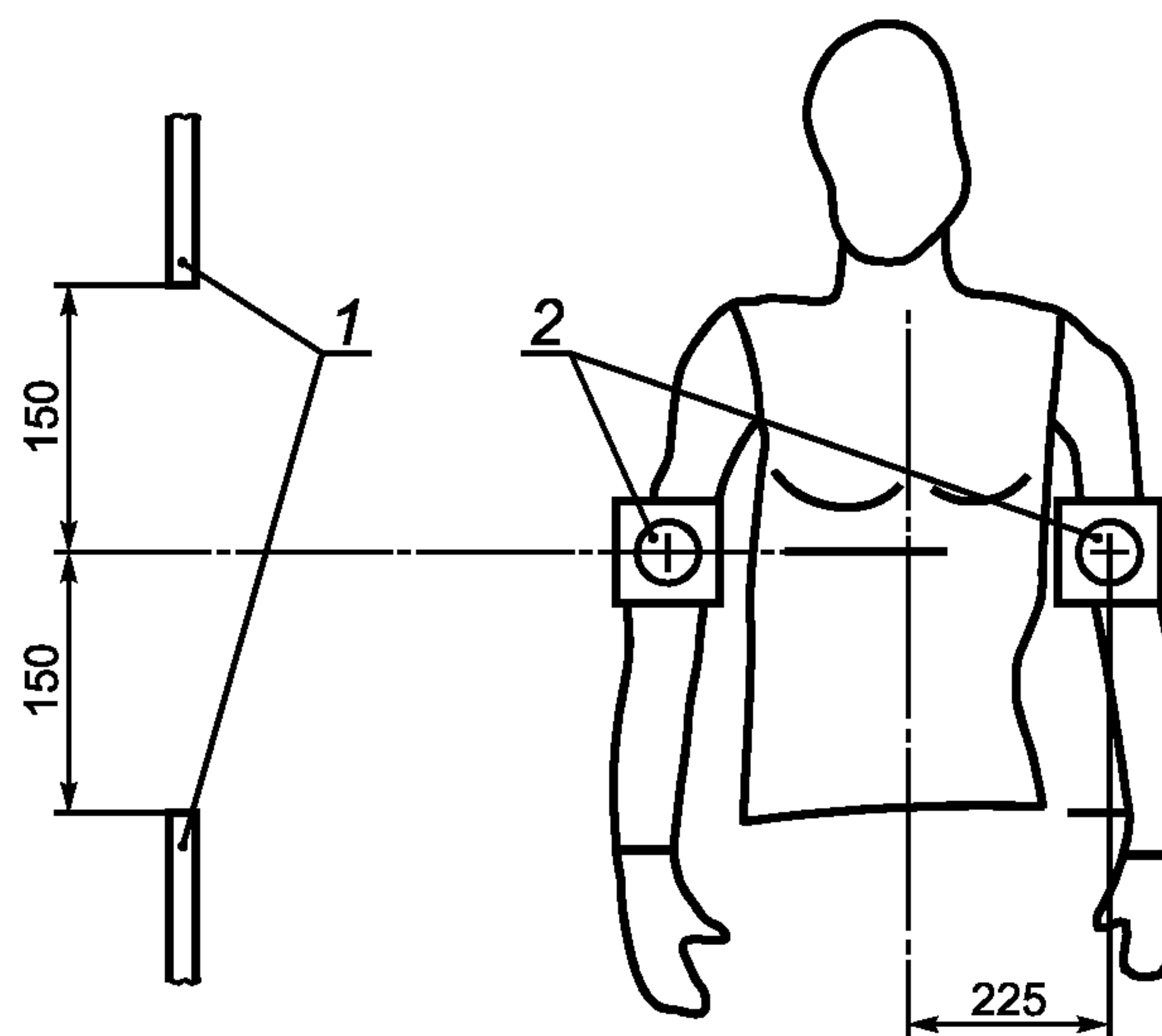
1 — электрод; 2 — контрольный датчик
