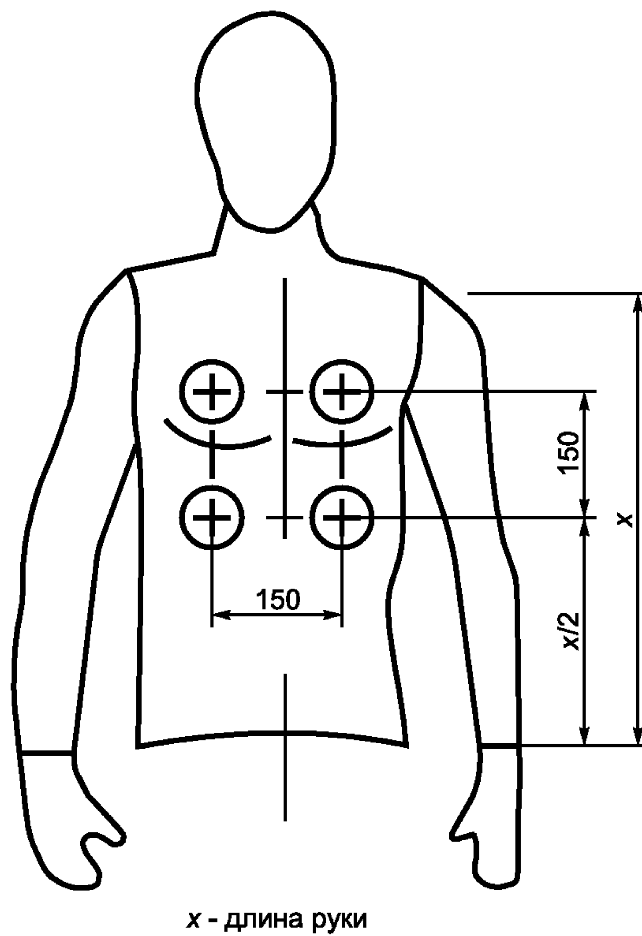
Рисунок 6 — Манекен с четырьмя датчиками
