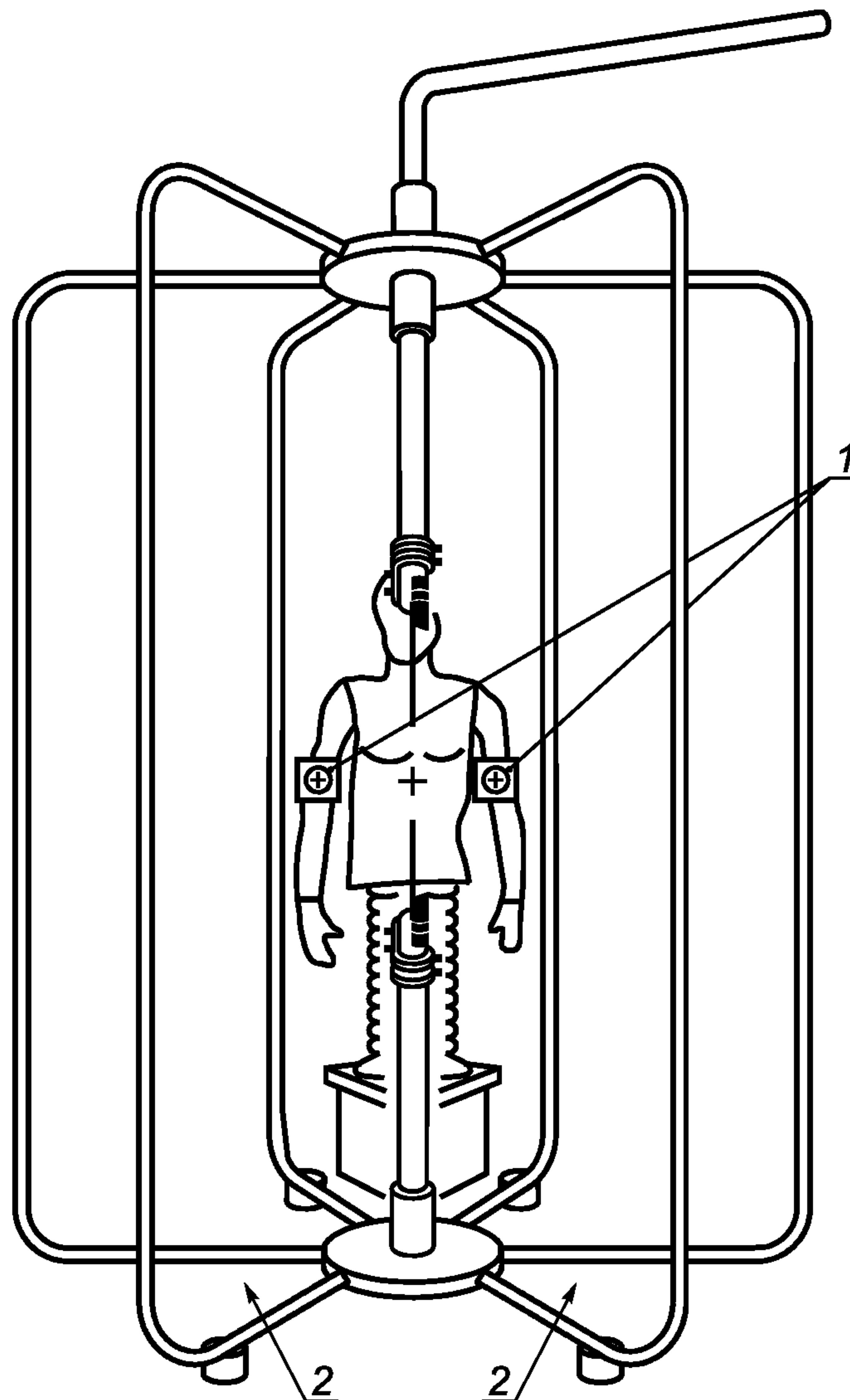
1 — контрольные датчики; 2 — дополнительные положения манекенов
