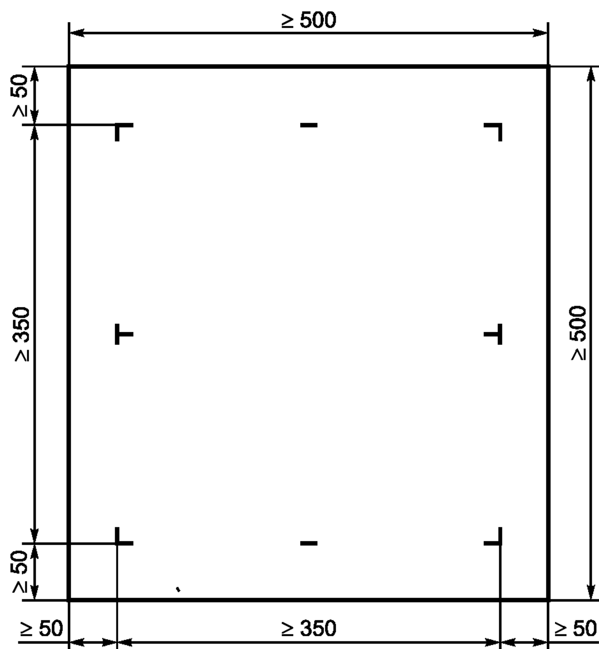
Рисунок 1 — Нанесение меток на образец ткани
