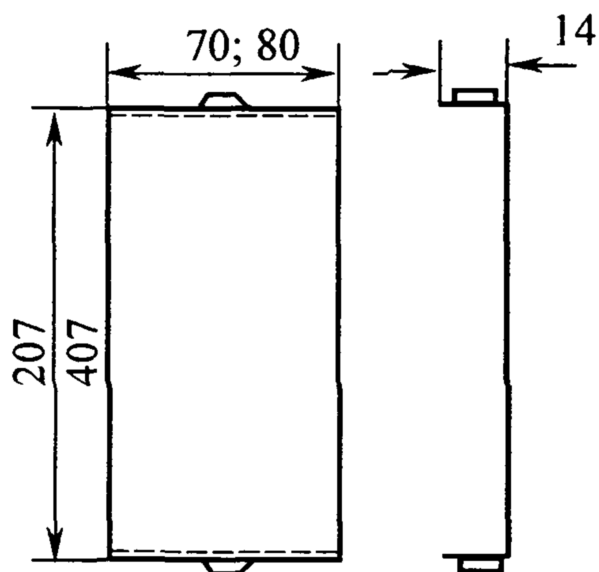
Рисунок А10 Накладка
