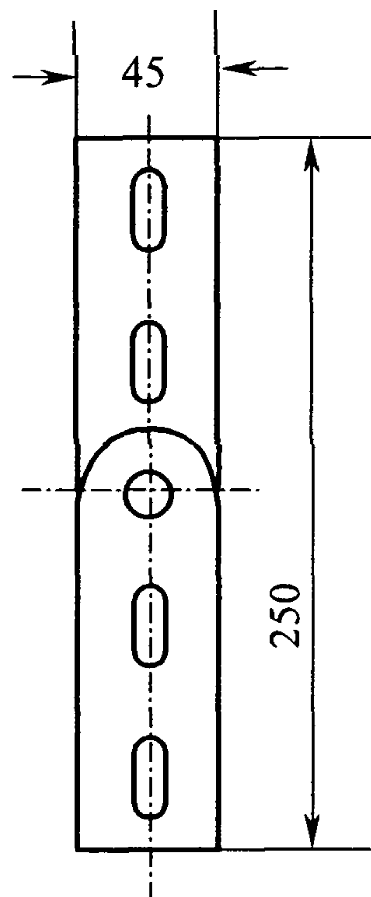
Рисунок А11 Шарнир
