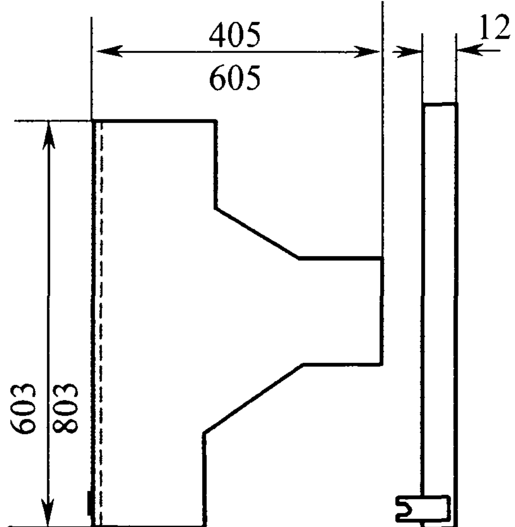
Рисунок А8 Крышка тройни- ковая КРТ
