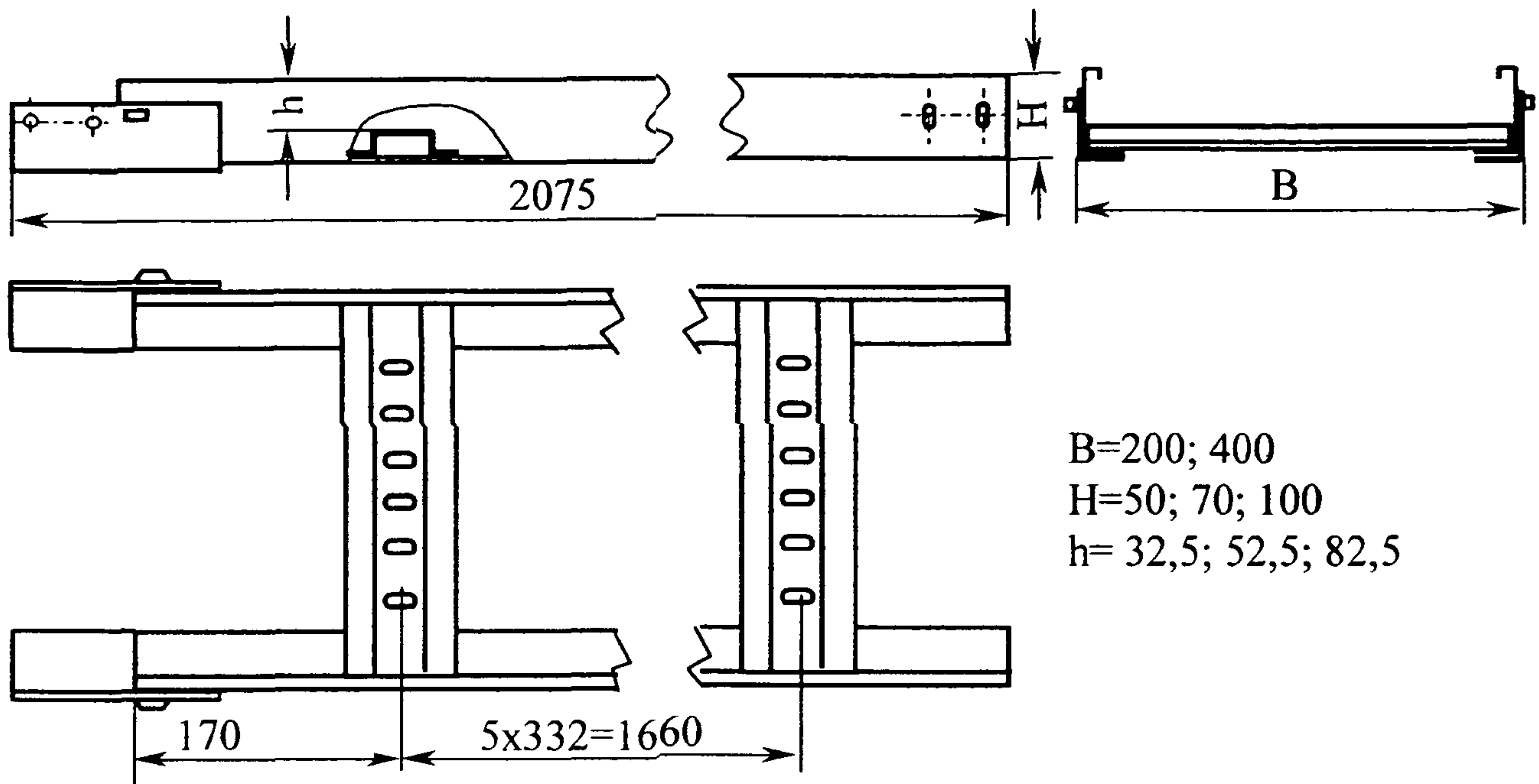
Рисунок А1 Секция прямая «ЛСП»
