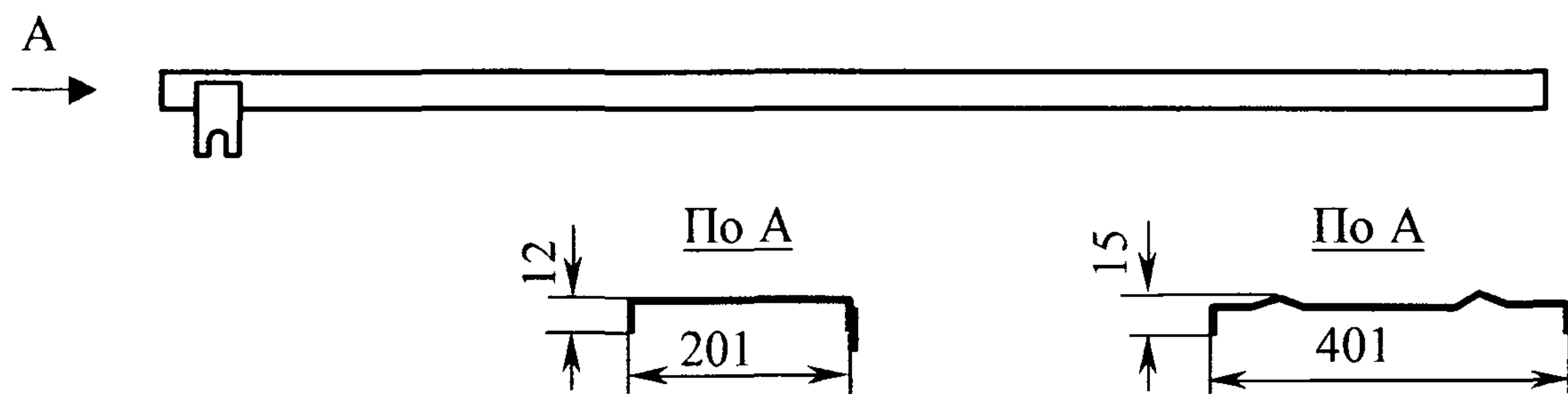
Рисунок А6 Крышка прямая КРП
