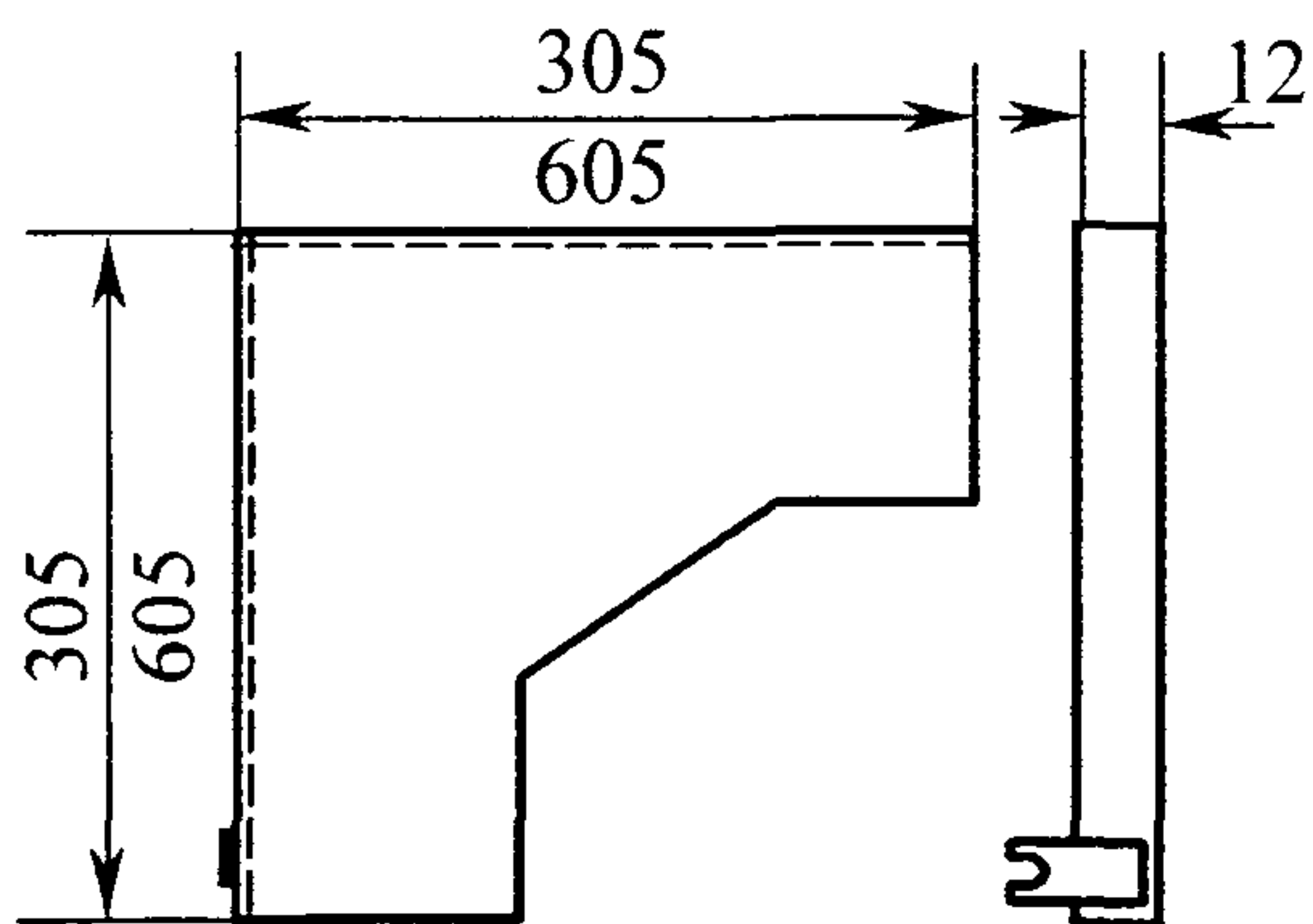
Рисунок А7 Крышка угловая КРУ
