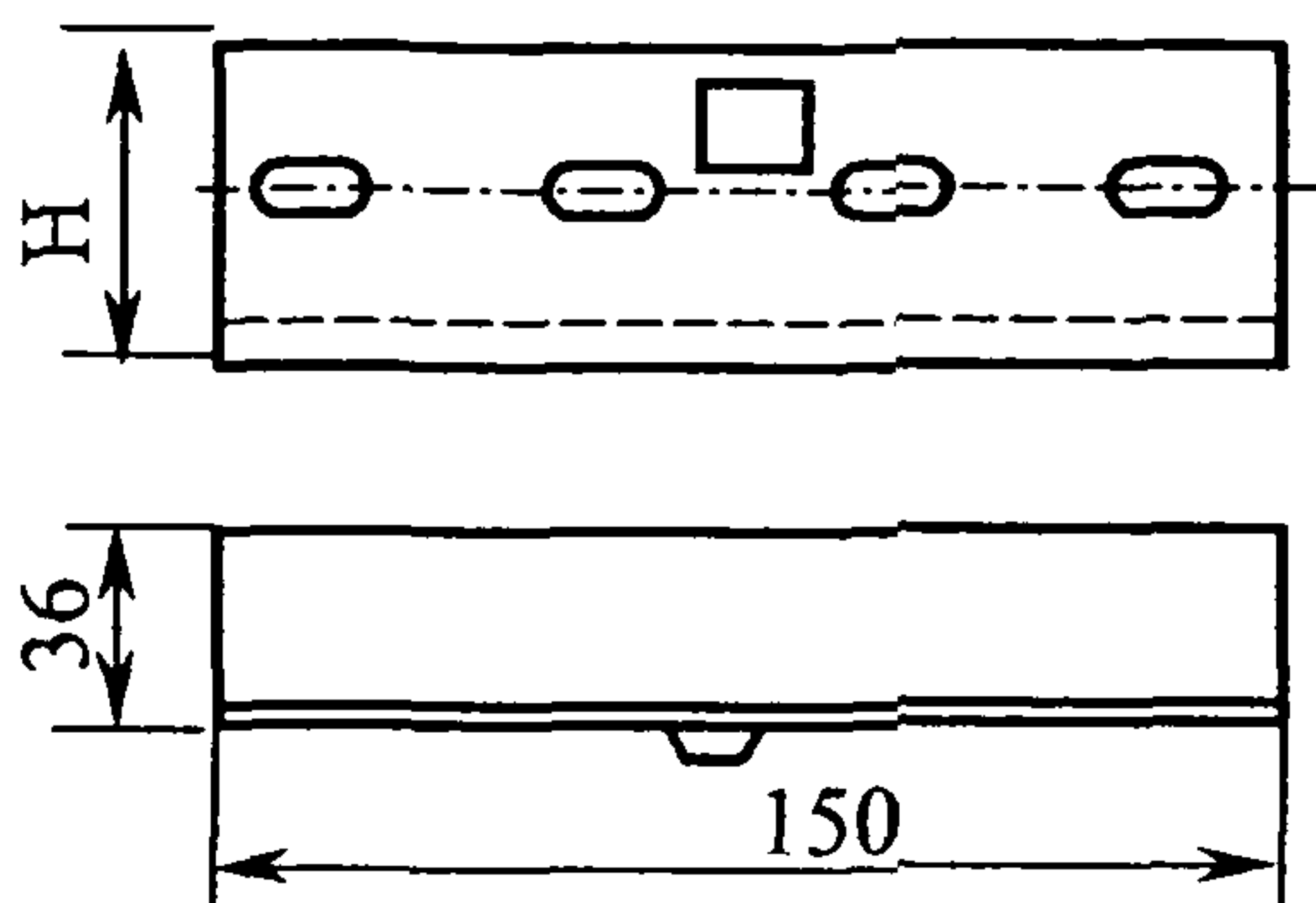
Рисунок А9 Угольник
