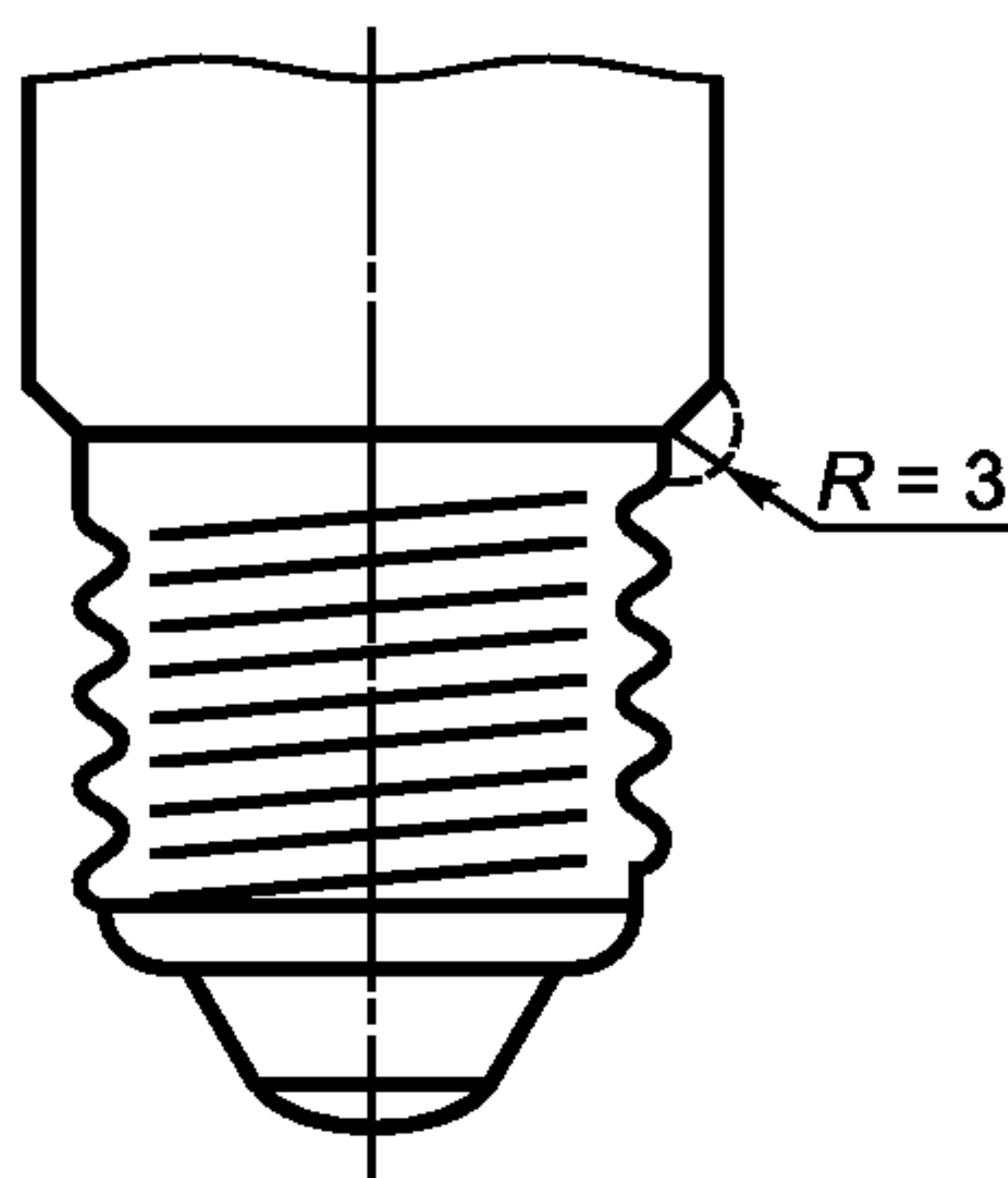
Рисунок 1 — Лампа с резьбовым цоколем
