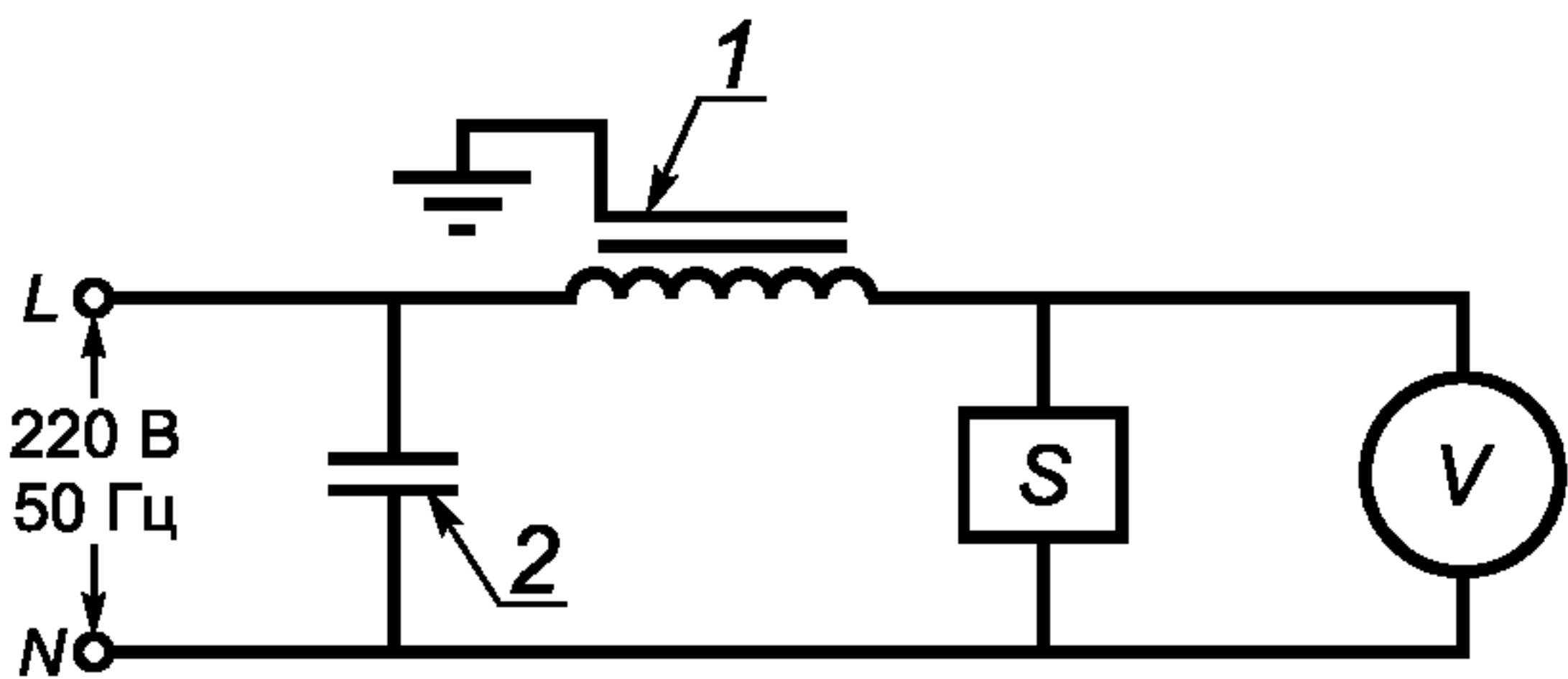
1 — пускорегулирующий аппарат; 2 — конденсатор для повышения коэффициента мощности
