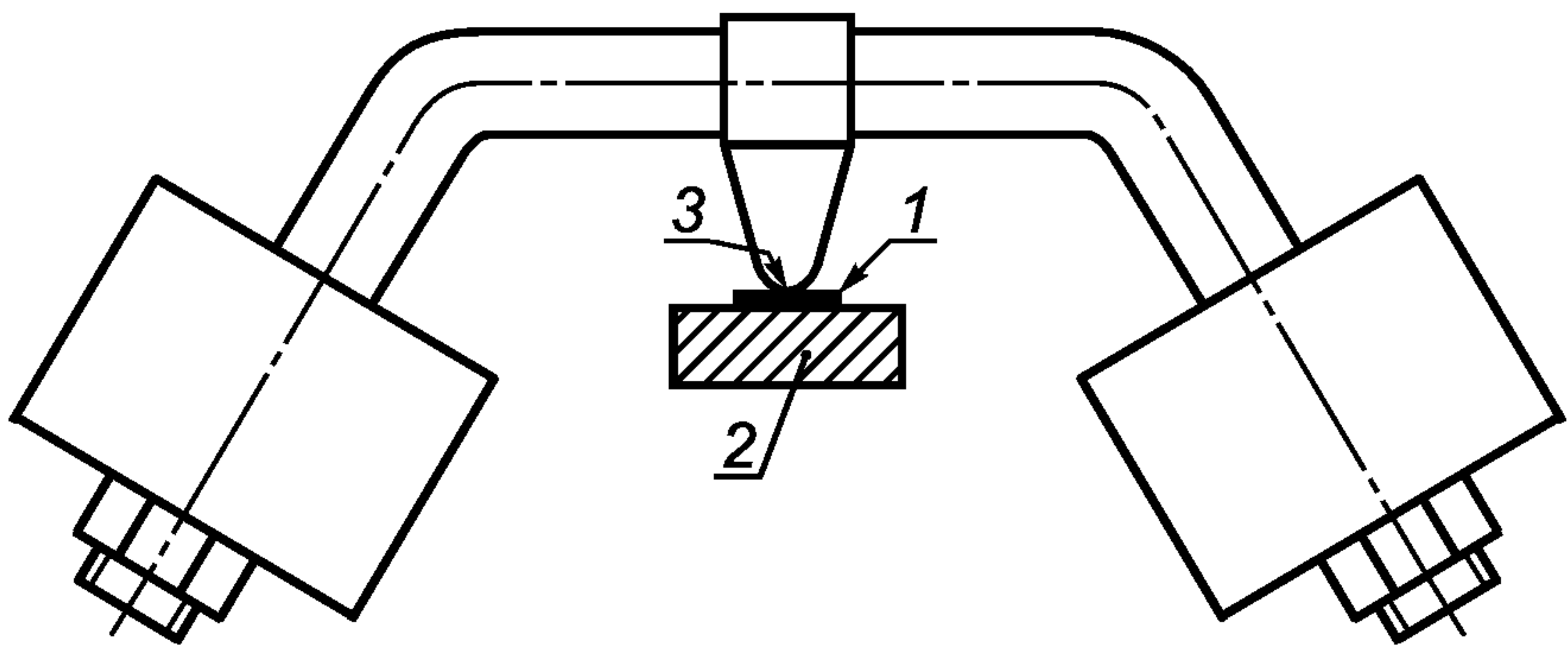
1 — образец; 2 — опора; 3 — сферический радиус R = 2,5\text{ мм}
