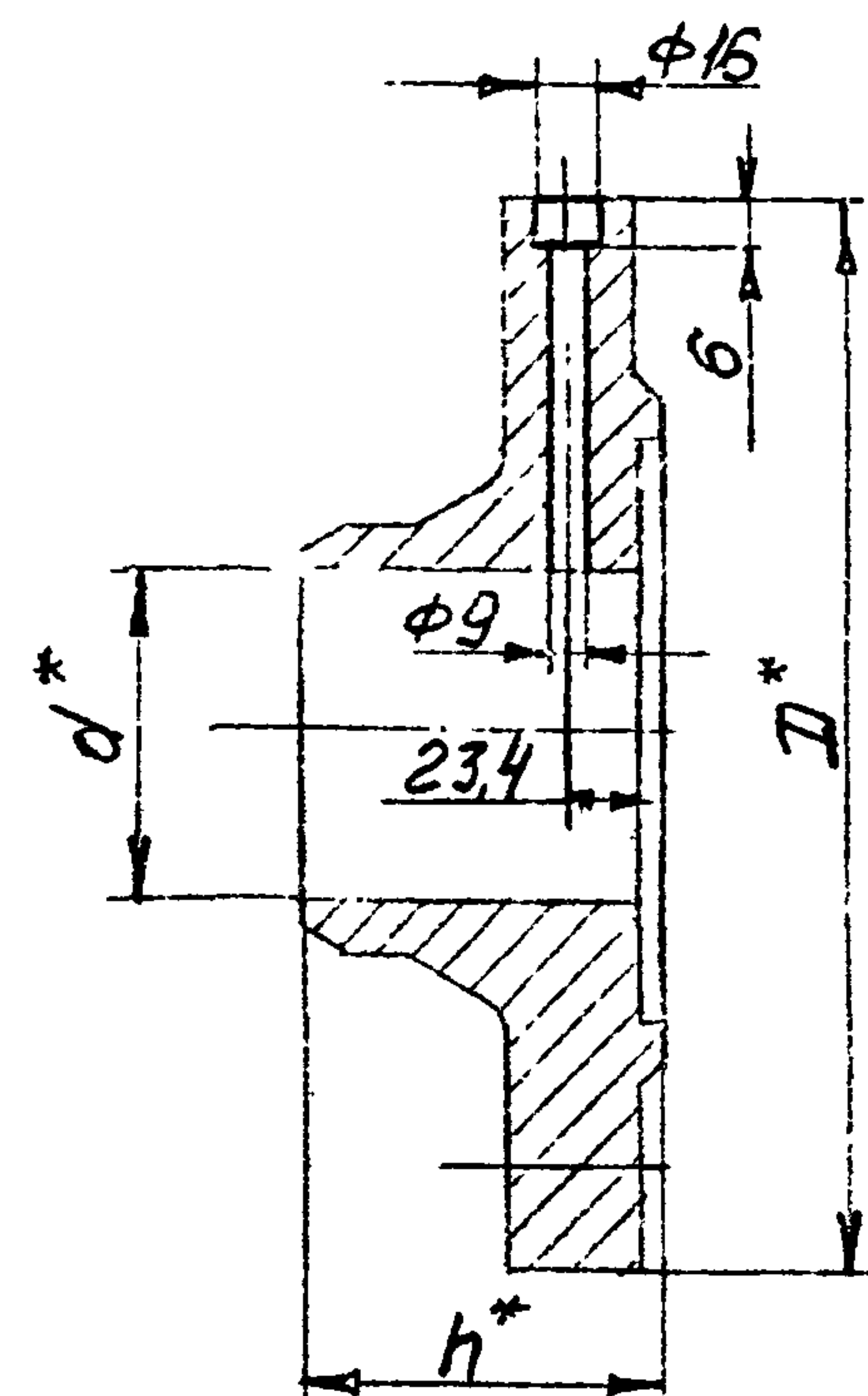
Поз.1 фланец
