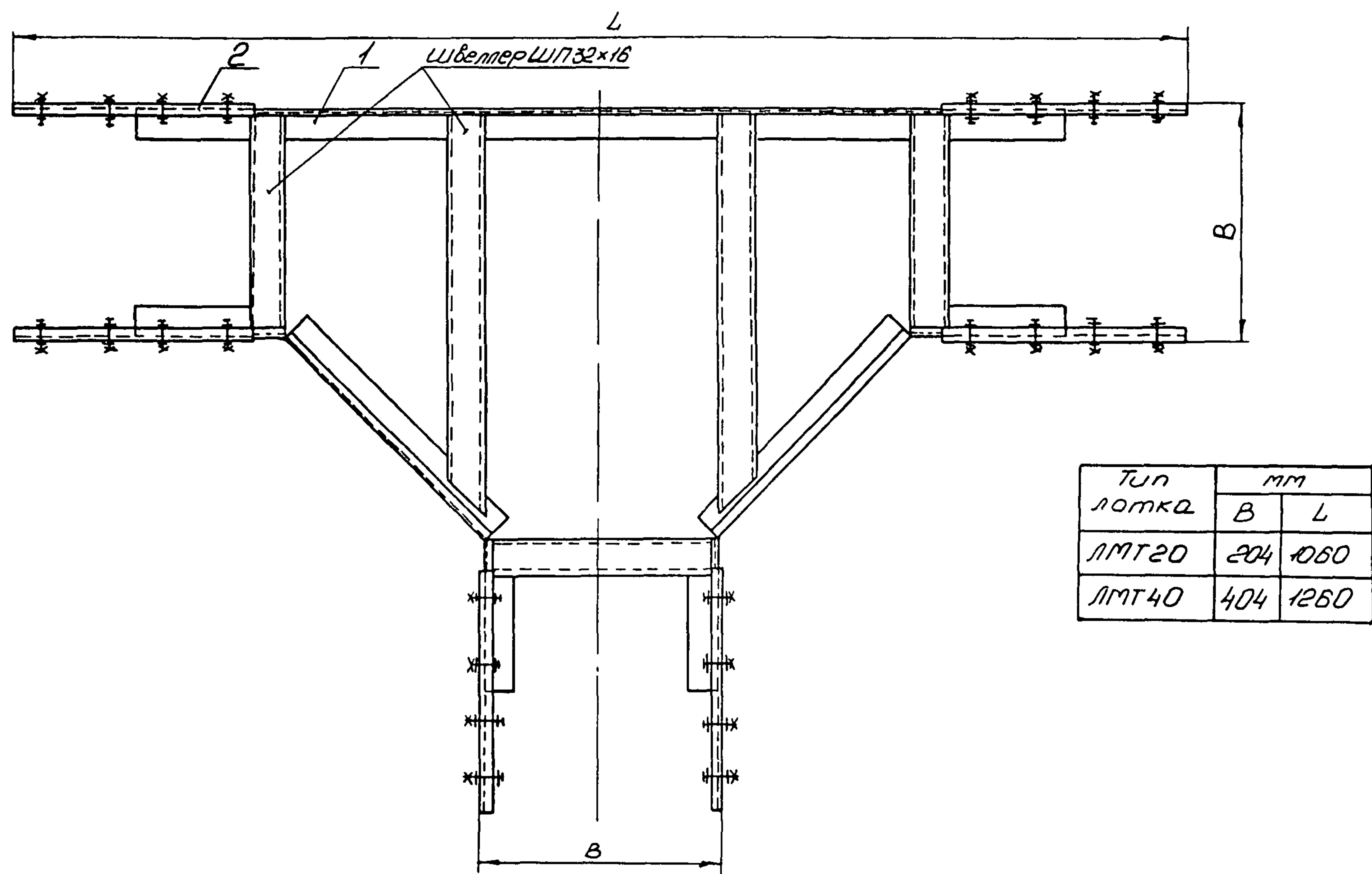
1 - корпус КСТ (ТК13-20-92); 2 - накладка ЛМТ Н ТУ36.22.21.001-86
