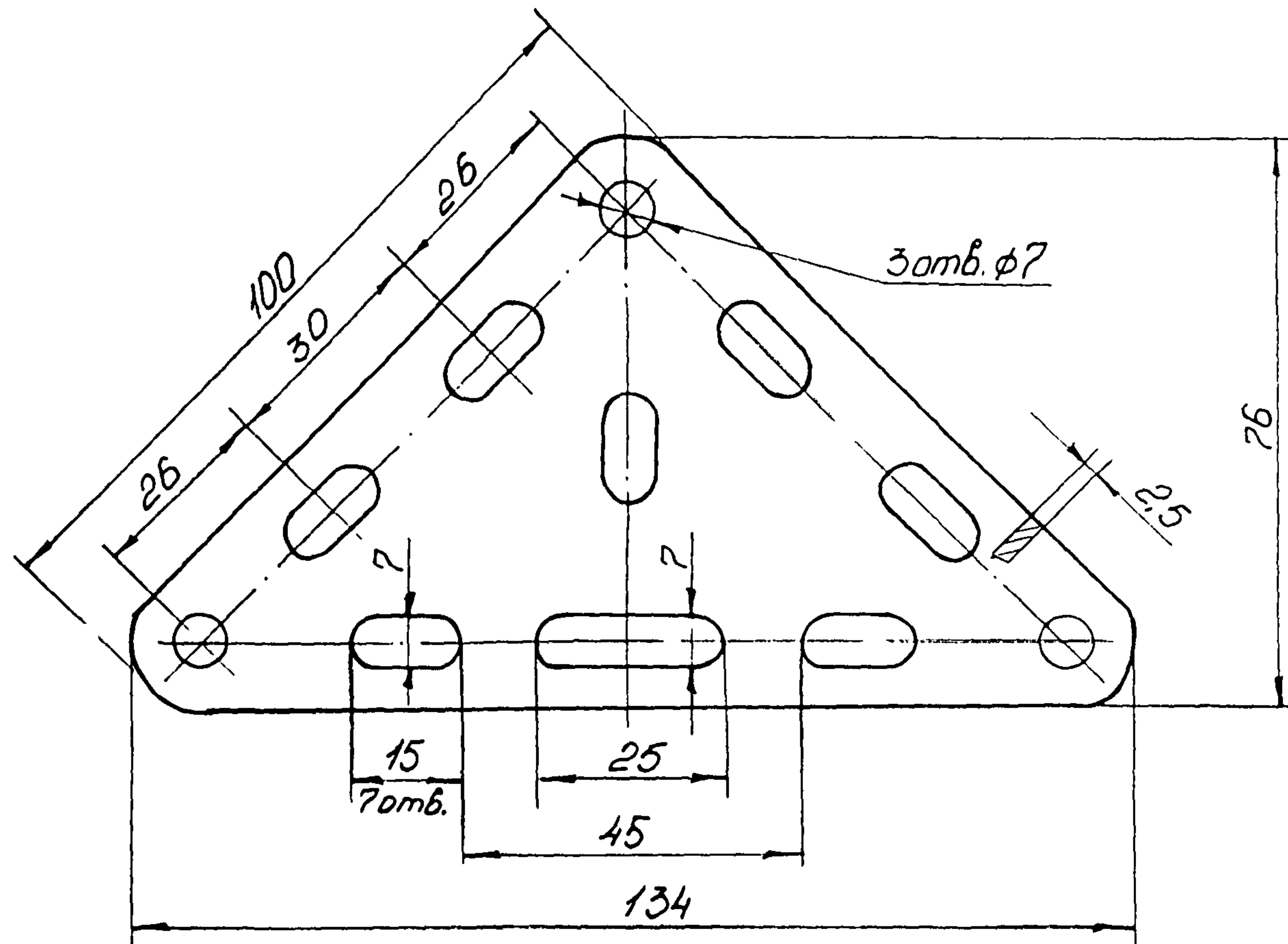
Косынка перфорированная КП 100
