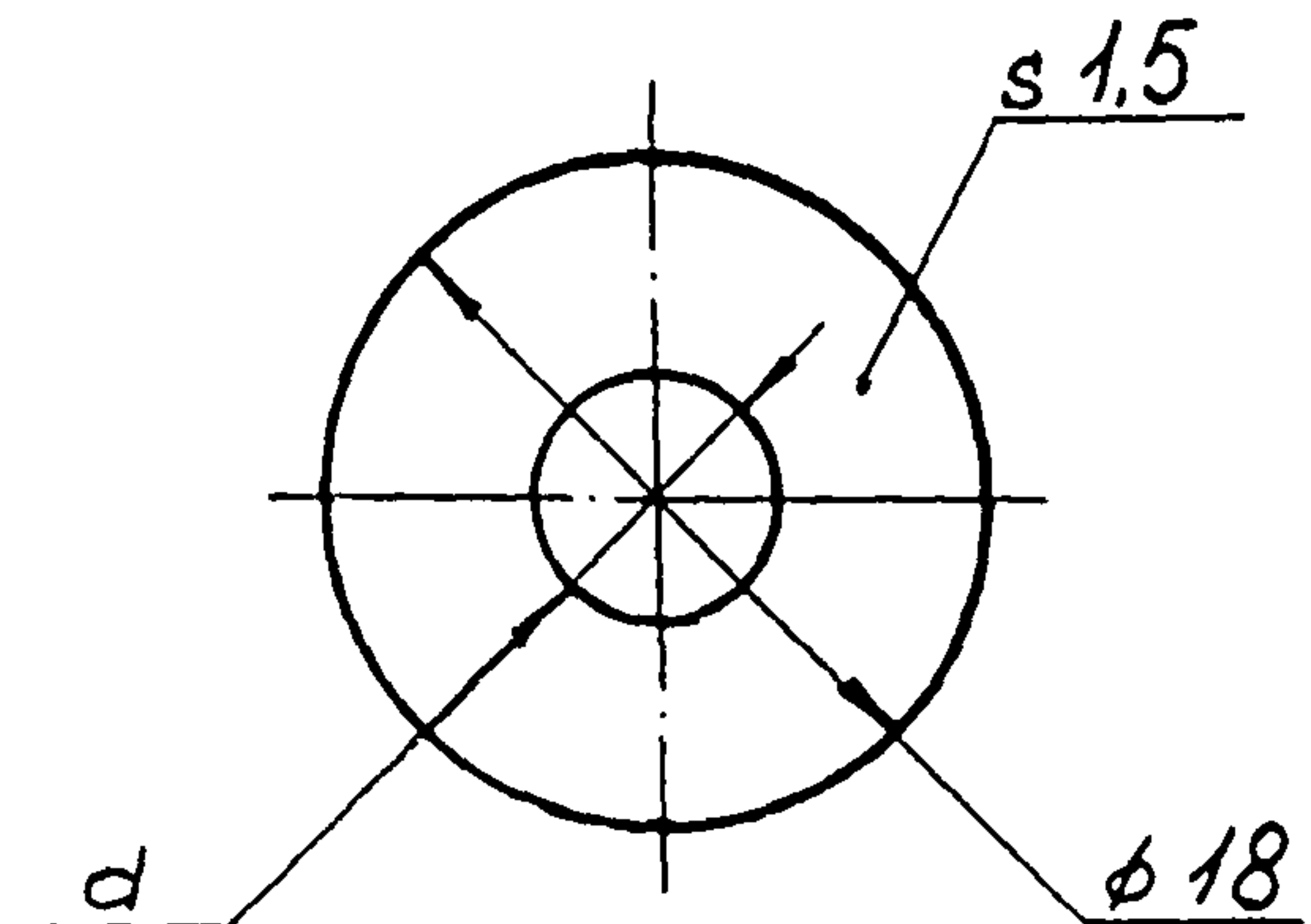
Шайба специальная ШС
