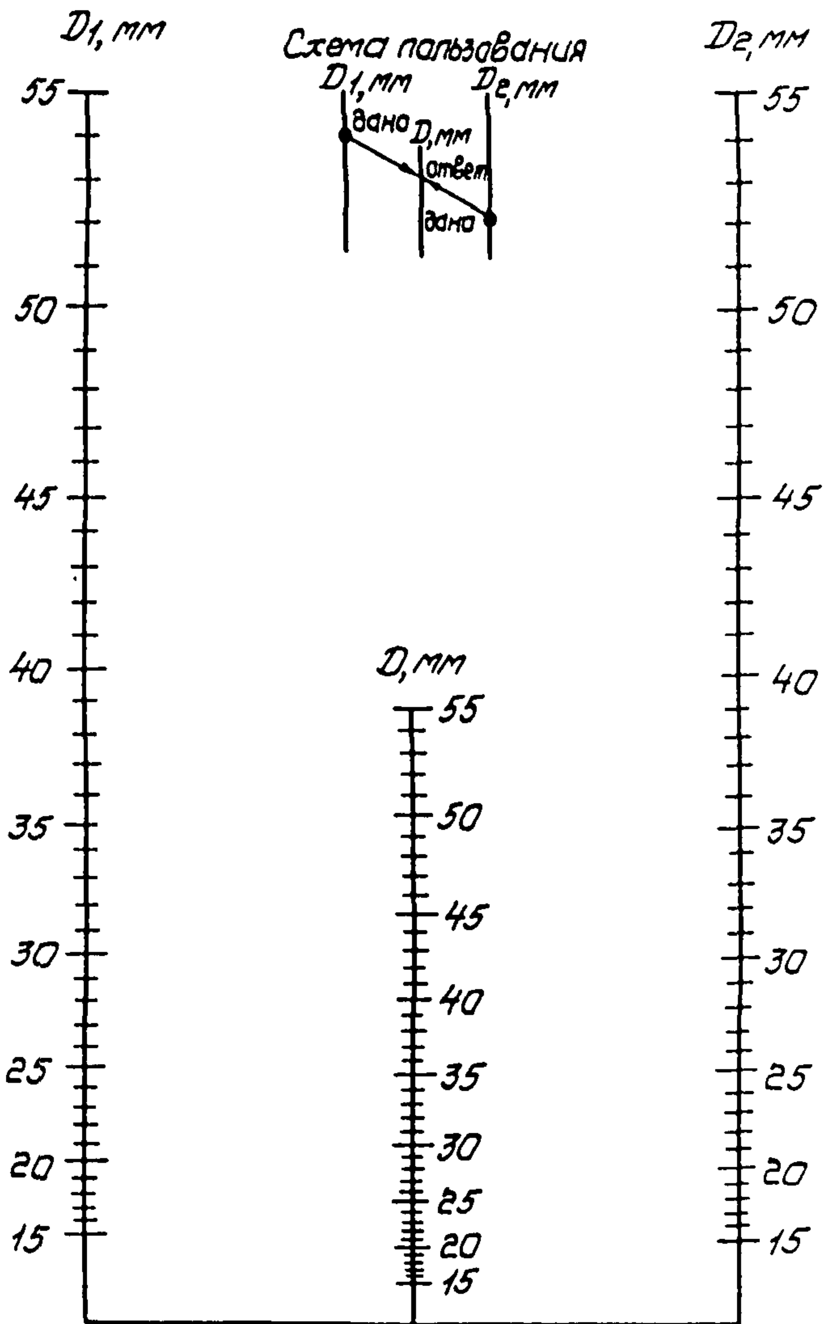
Рис.2. Номограмма определения внутреннего диаметра защитной трубы для прокладки проводников двух различных диаметров при общем числе их более двух.
