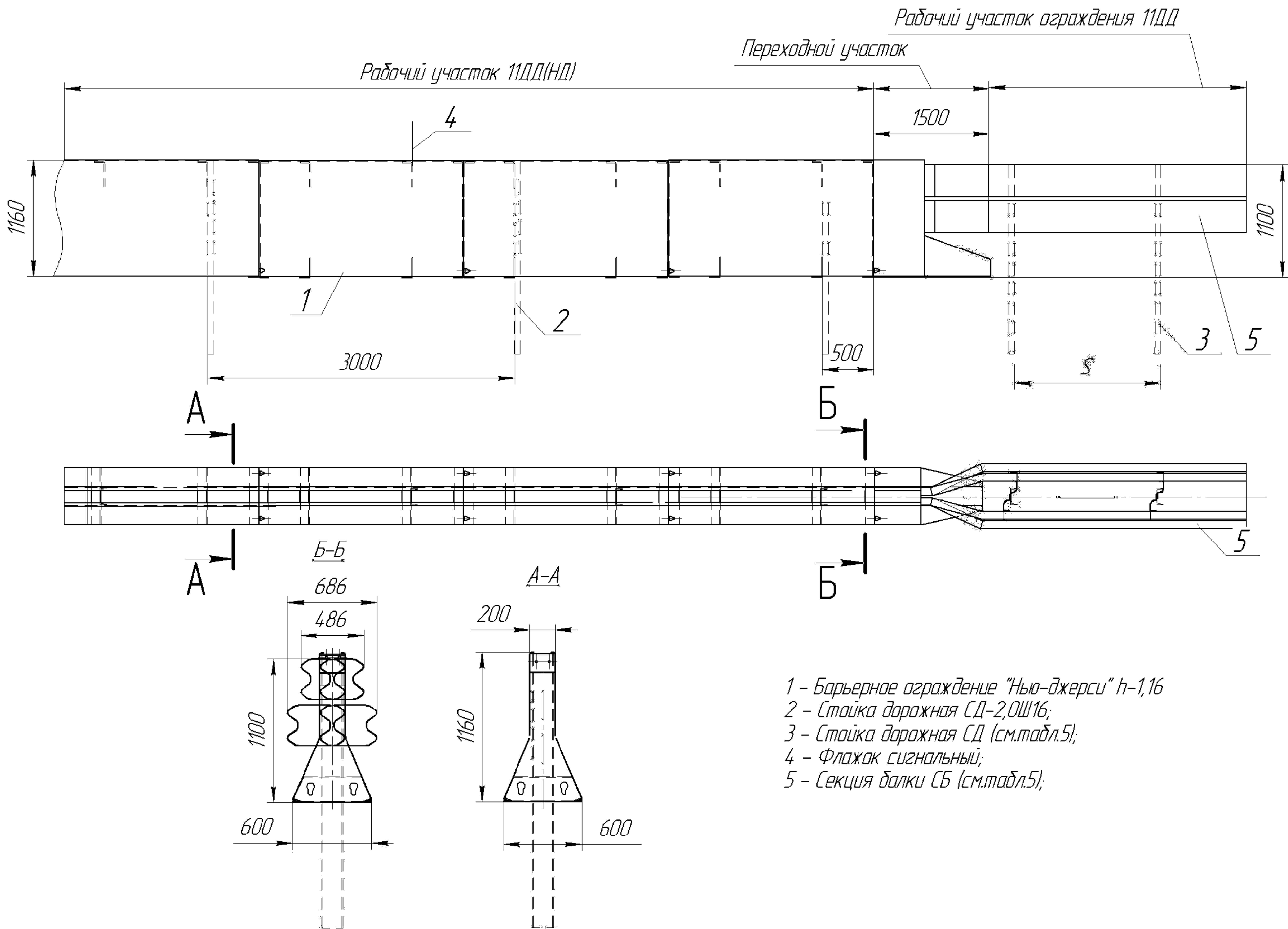
Рисунок 3.8 - Переходной участок 11ДД(НД)/1,16 на 11ДД/1,1
