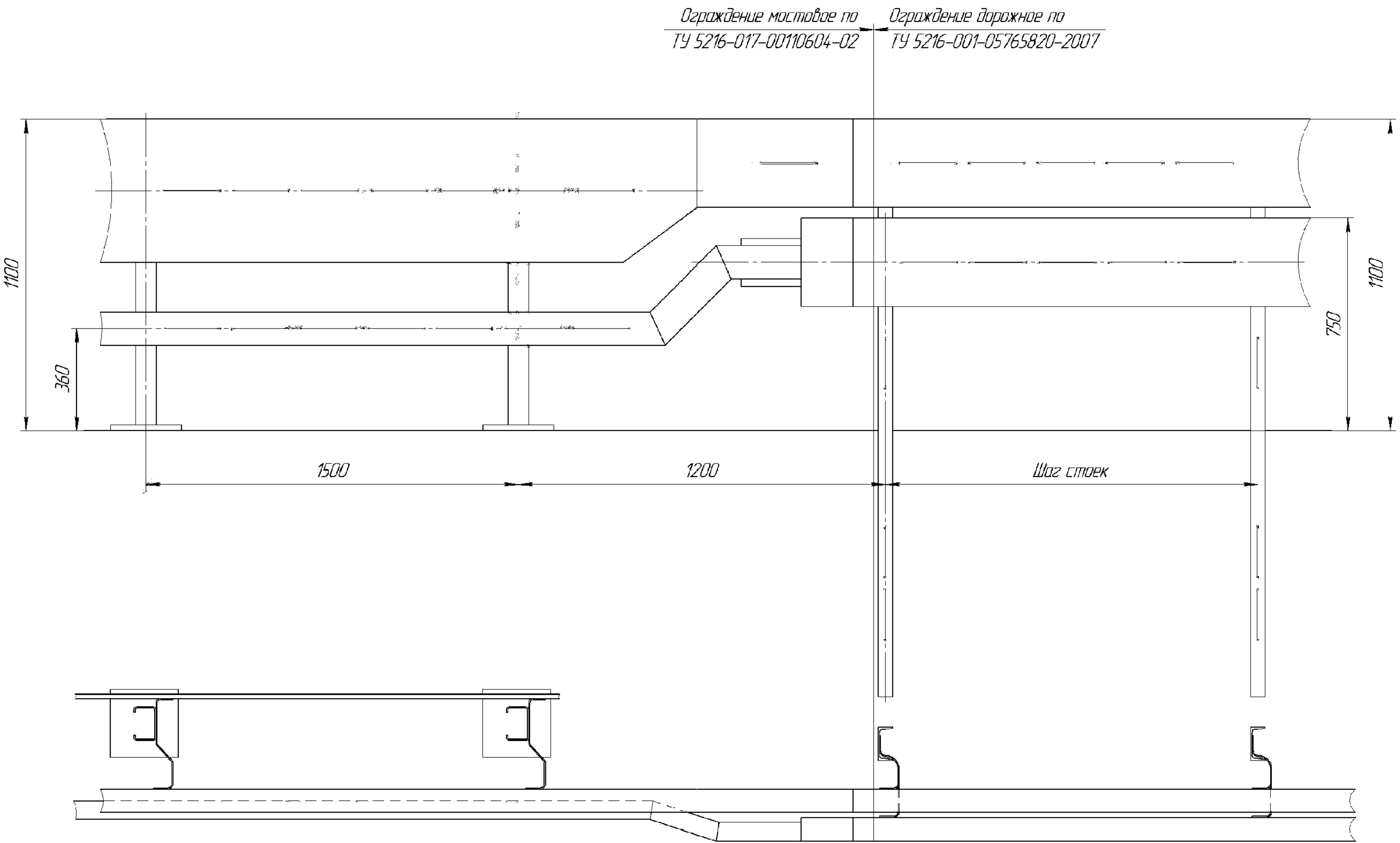
Рисунок В.16 Узел сопряжения огр. мостового (ТУ 5216-017-00110604-02) с огр. дорожным (ТУ 5216-001-05765820-2007)
