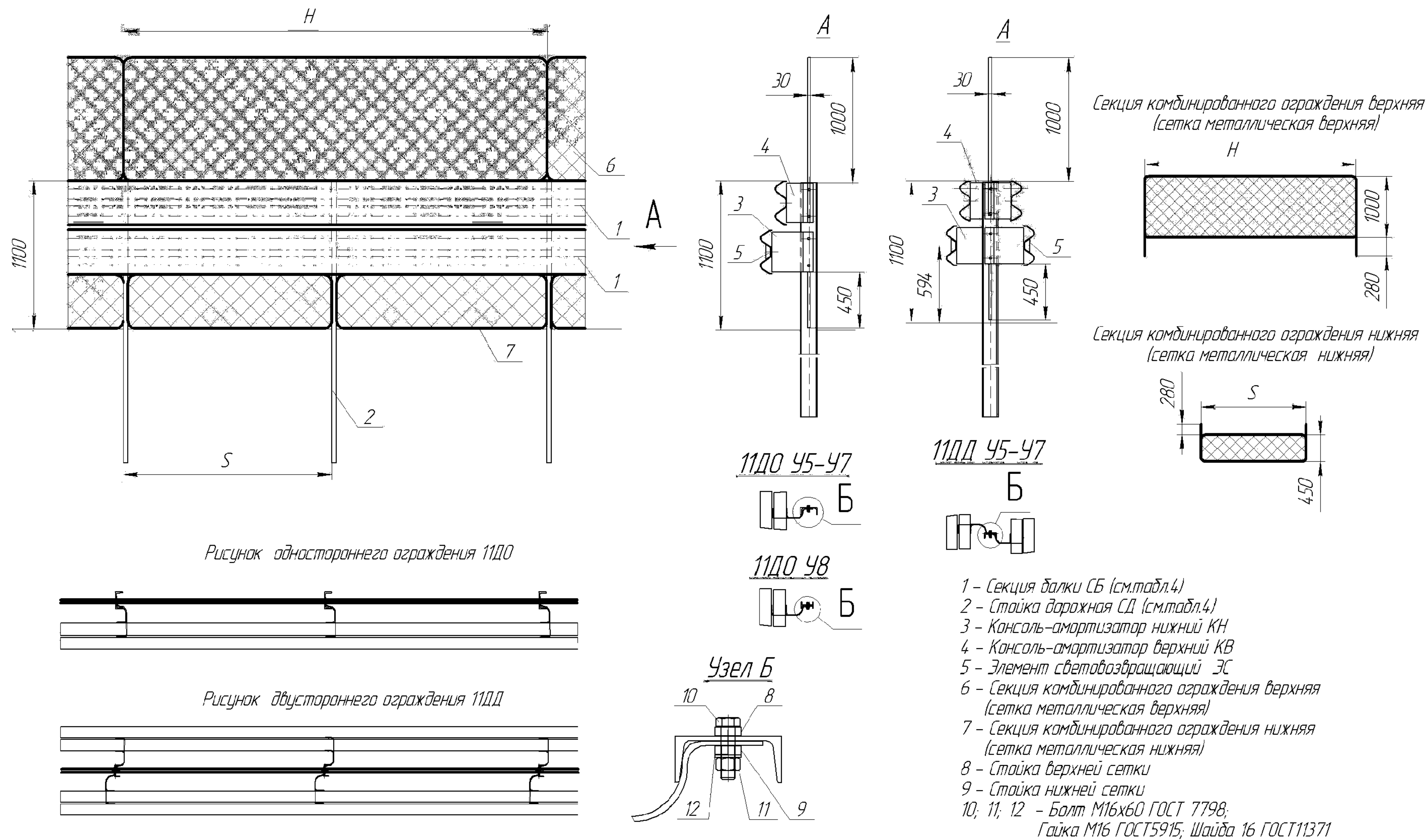
Рисунок Ж.6 Ограждение комбинированное 45-48
