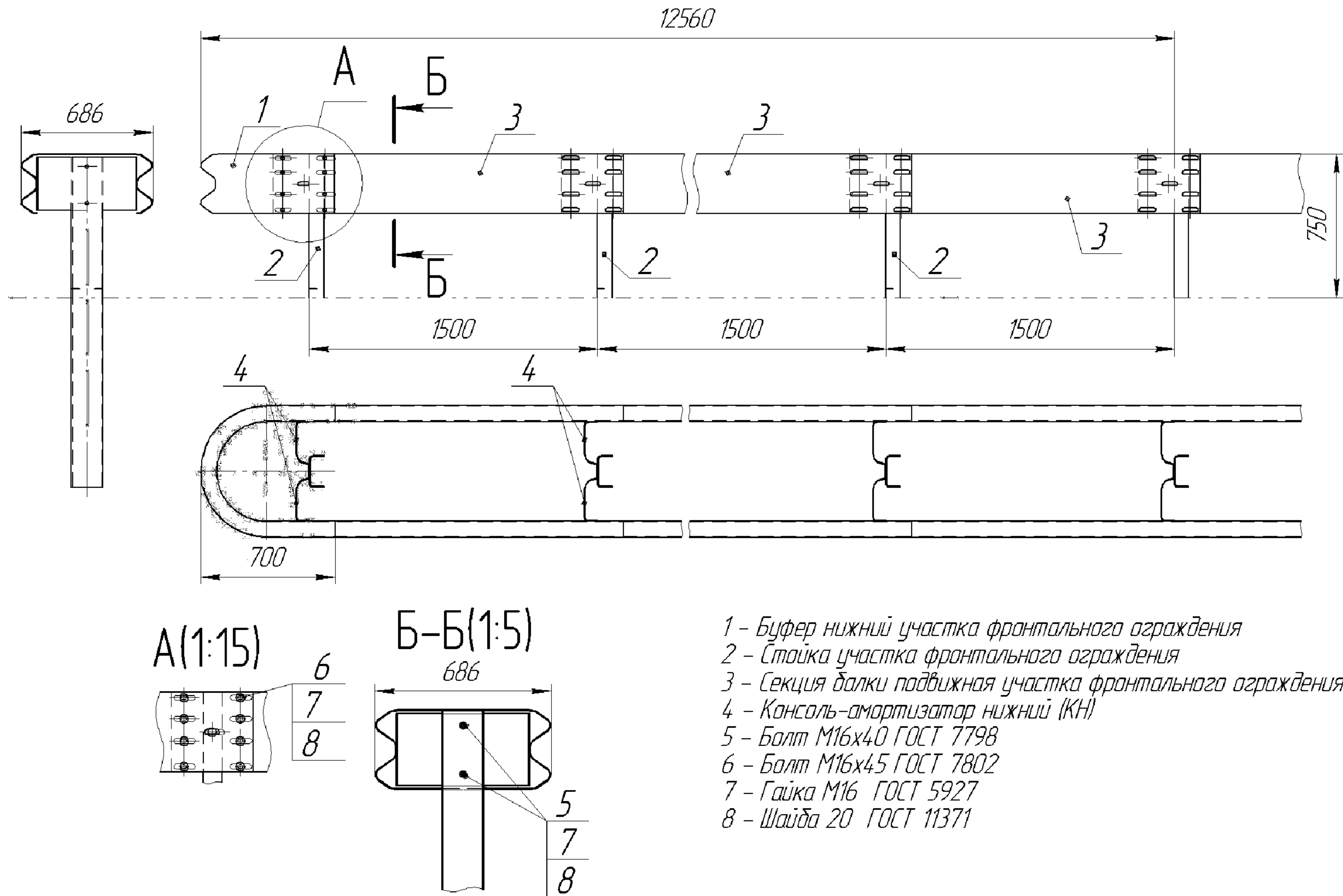
Рисунок И.1 Фронтальное ограждение
