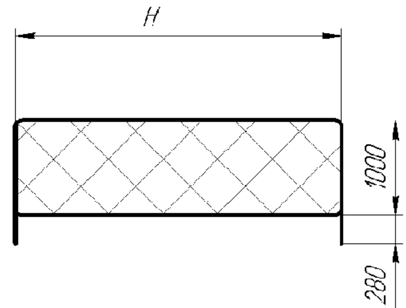
Секция комбинированного ограждения нижняя (сетка металлическая нижняя)
