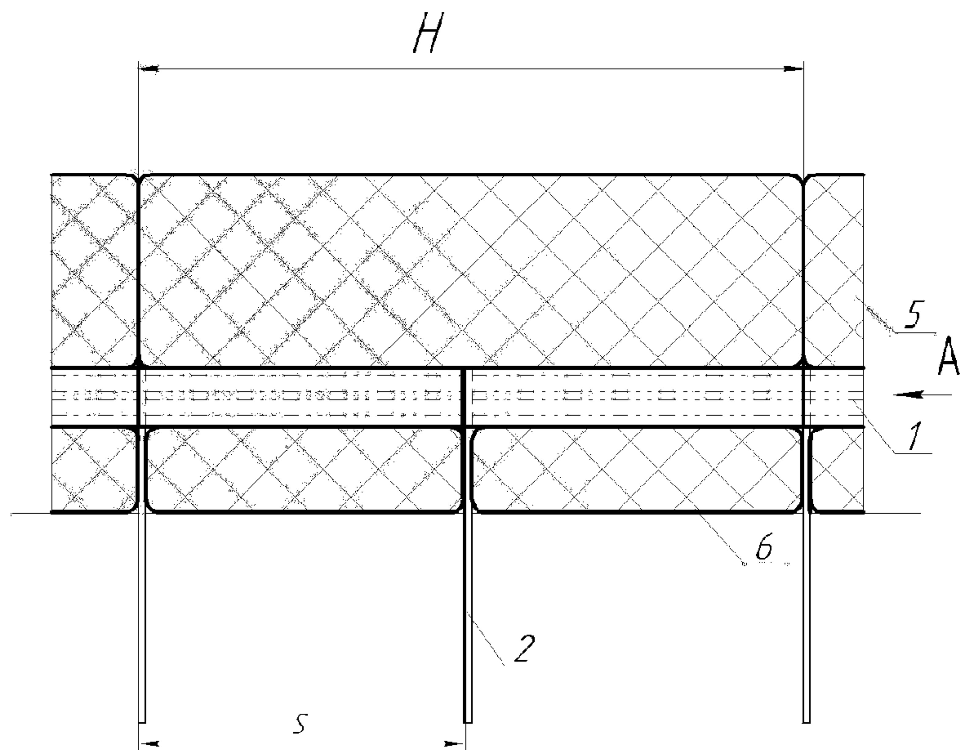
Рисунок одностороннего ограждения 11ДД У1-У4
