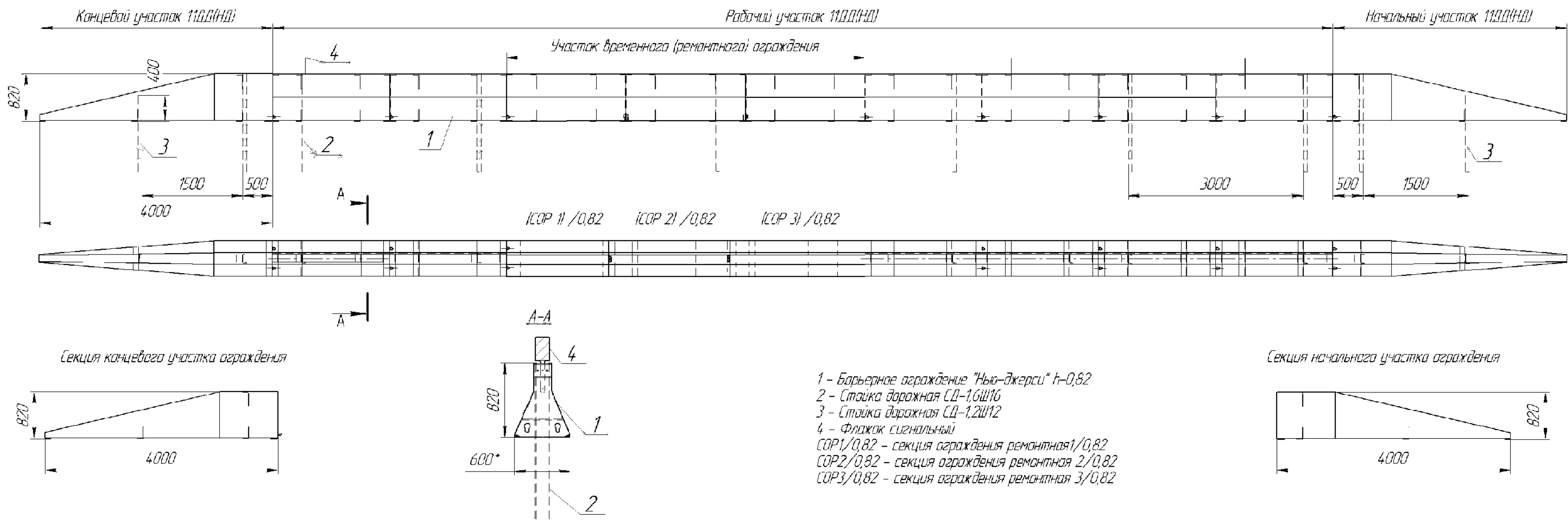
Рисунок 3.5 - Ограждение группы 11ДД(НД)-0,82
