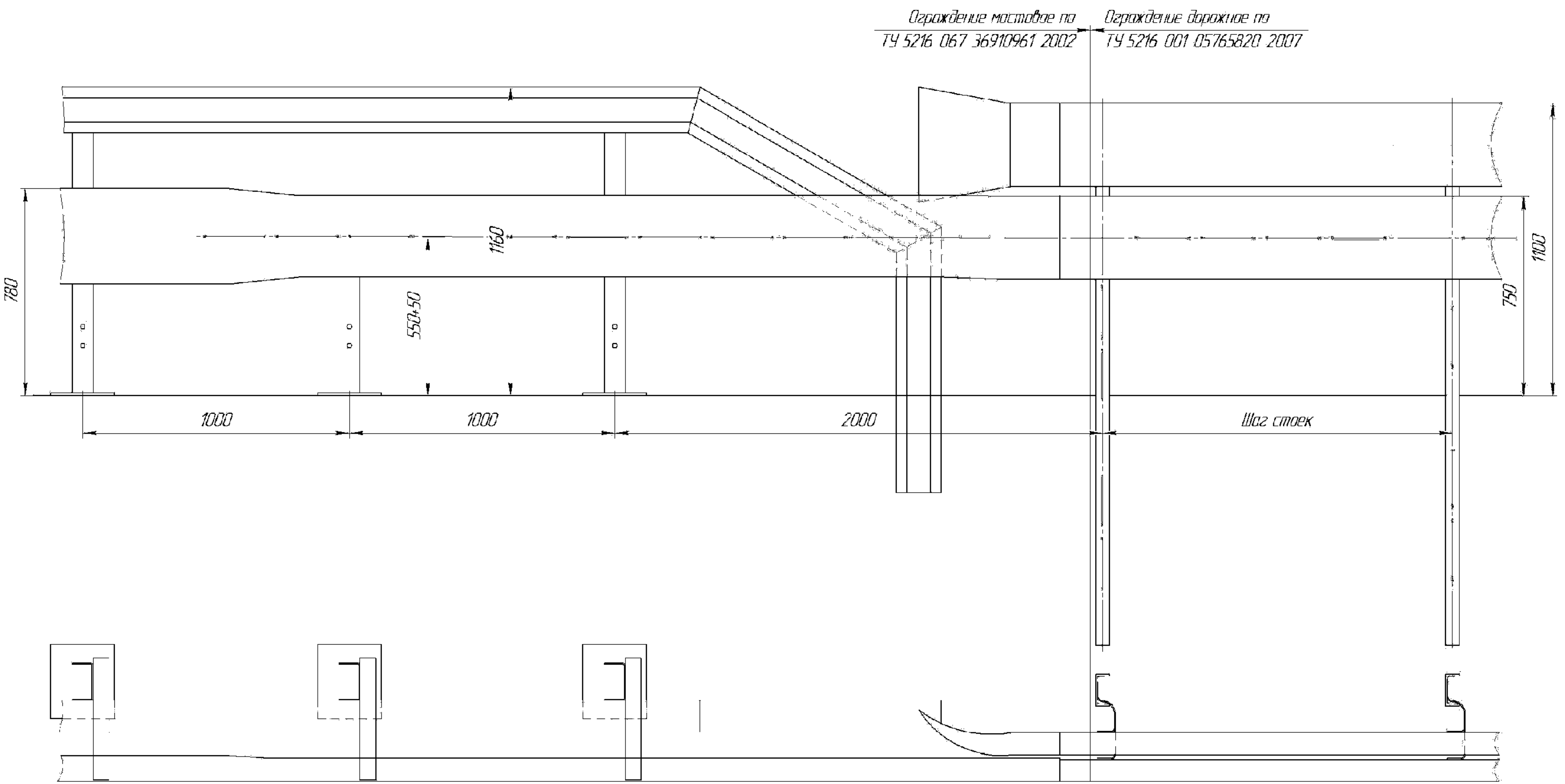
Рисунок В.2 Узел сопряжения отр. Мостового (ТУ 5216-067-36910961-2002)с отр. дорожным (ТУ 5216-001-05765820-2007)
