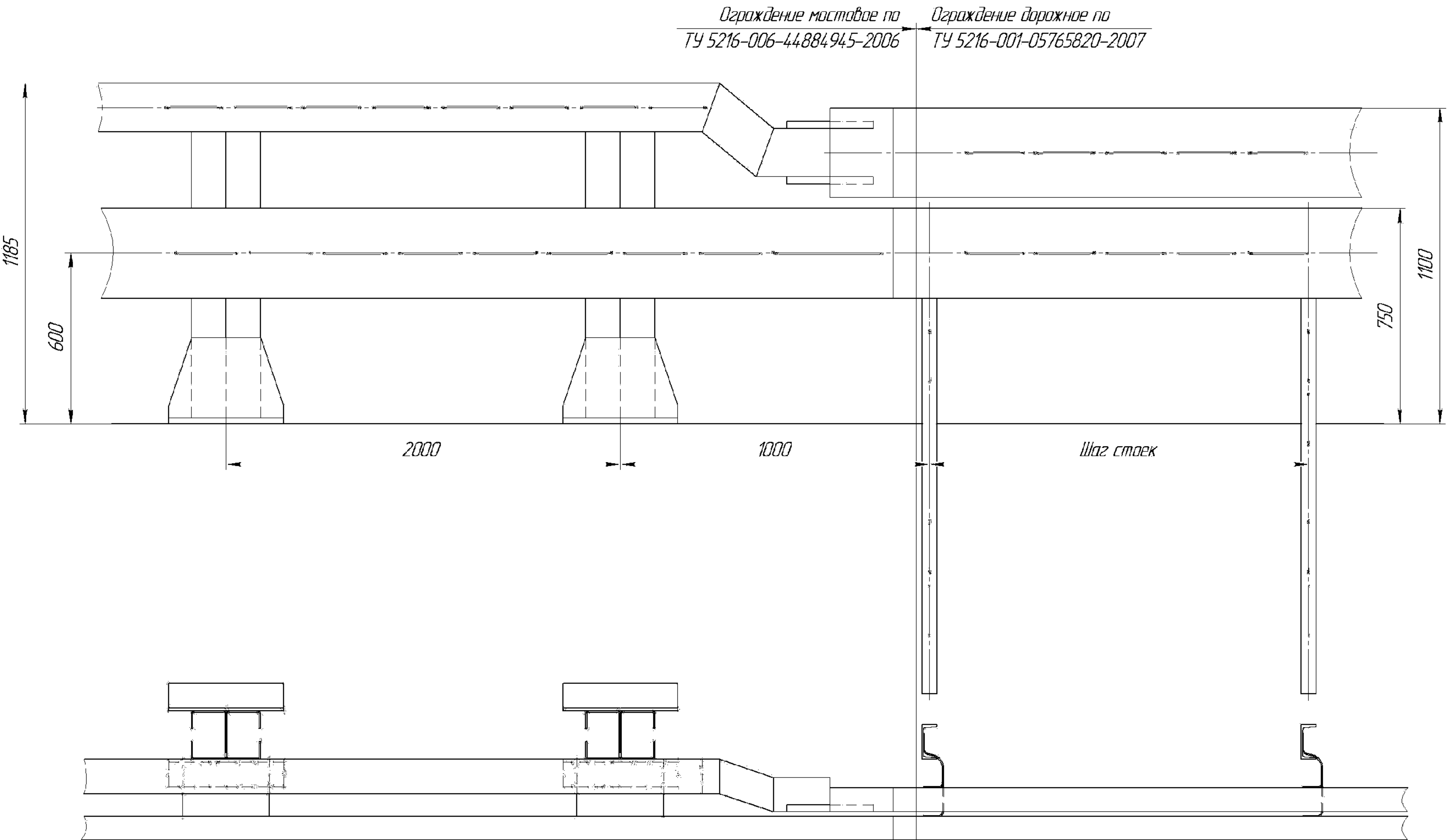
Рисунок В.6 Узел сопряжения отг. мостового (ТУ 5216-006-44884945-2006) с отг. дорожным (ТУ 5216-001-05765820-2007)
