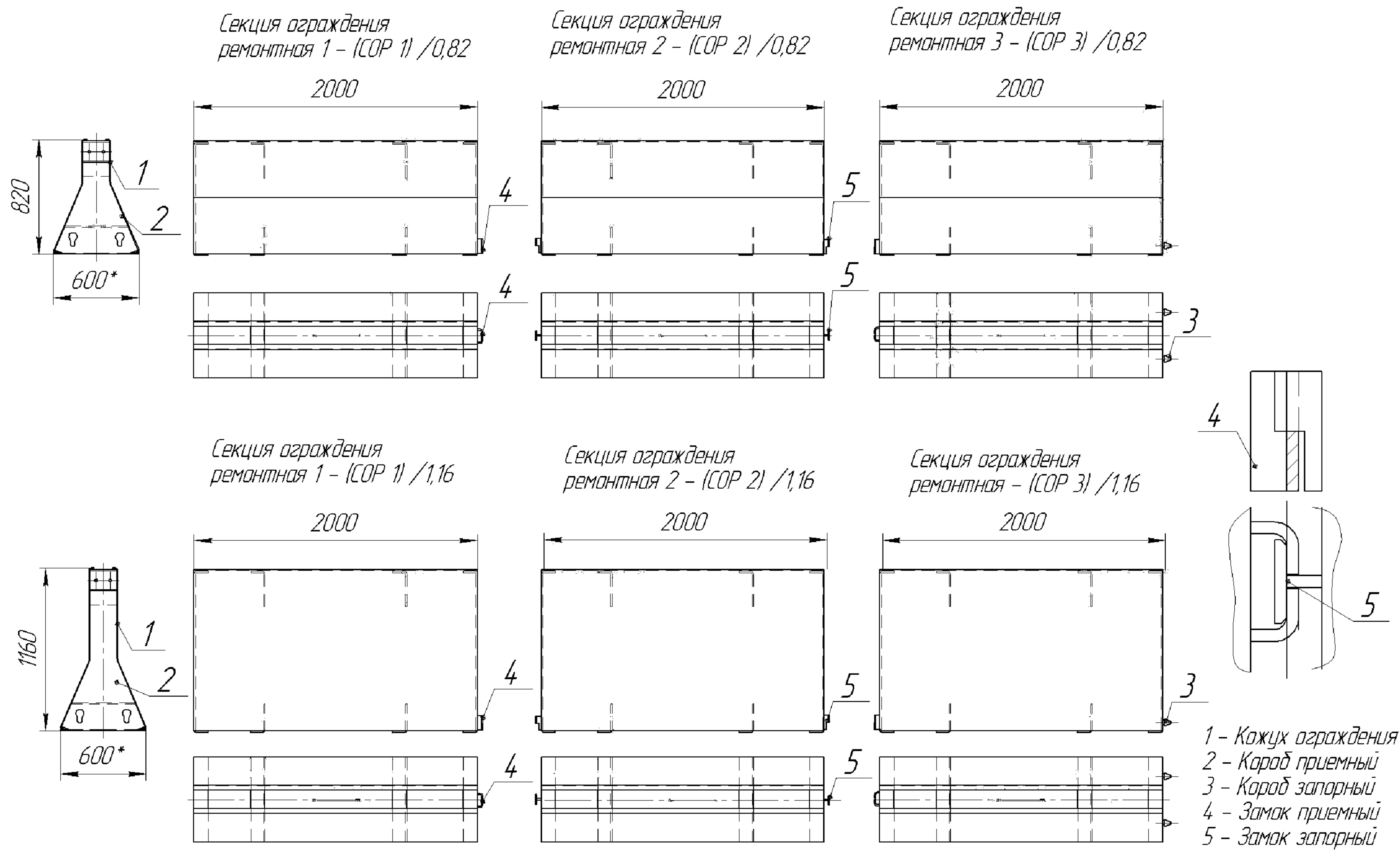
Рисунок 3.4 - Секции ограждения временного (ремонтного) 11ДД(НД)
