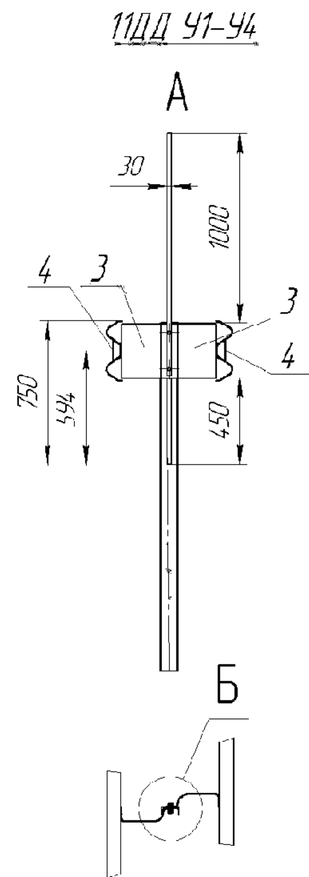
Секция комбинированного ограждения верхняя (сетка металлическая верхняя)
