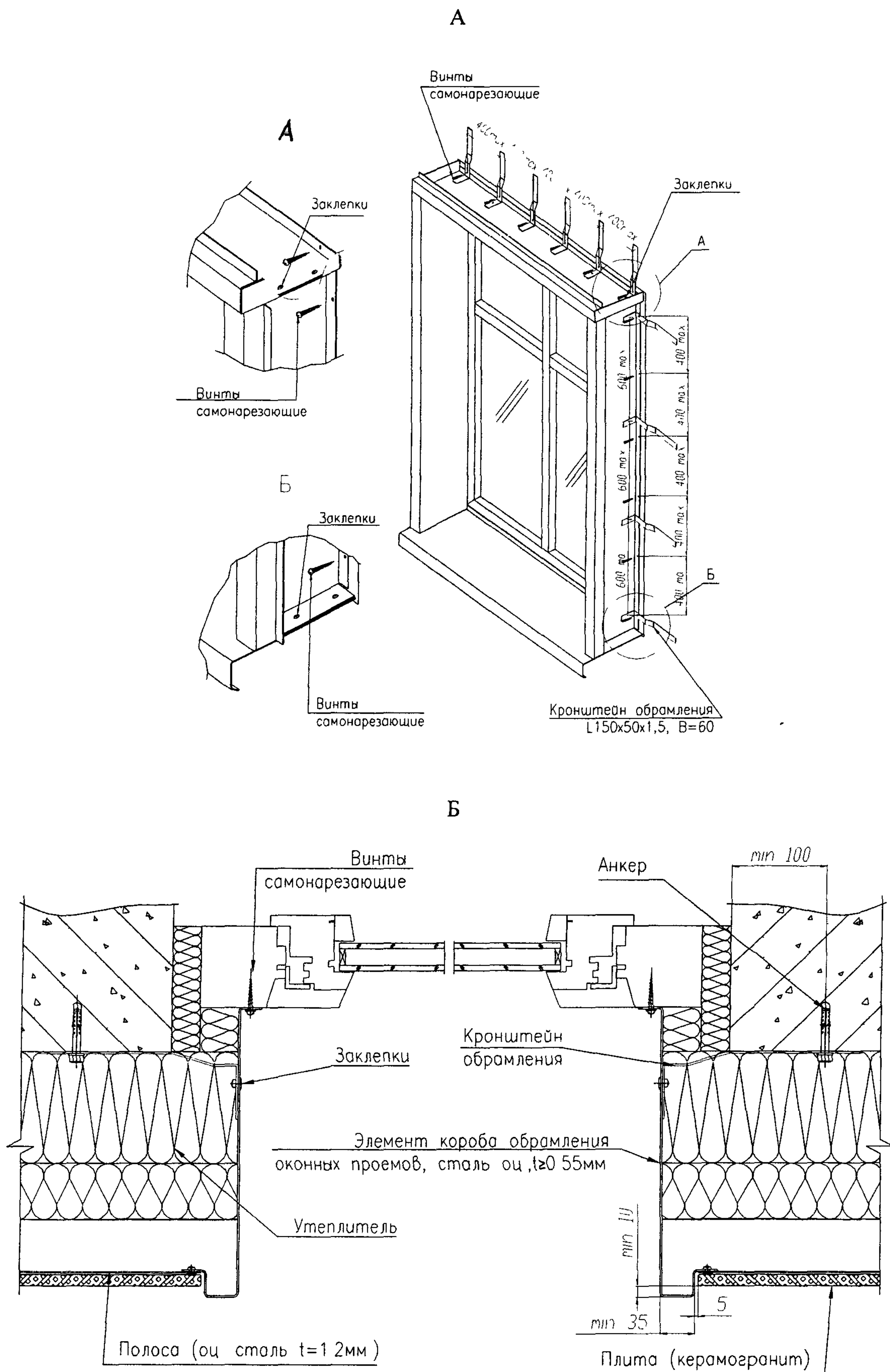
Рис.В.5. Схема установки оконного обрамления (А) и узел крепления бокового откоса (Б) в фасадной системе СО-01.
