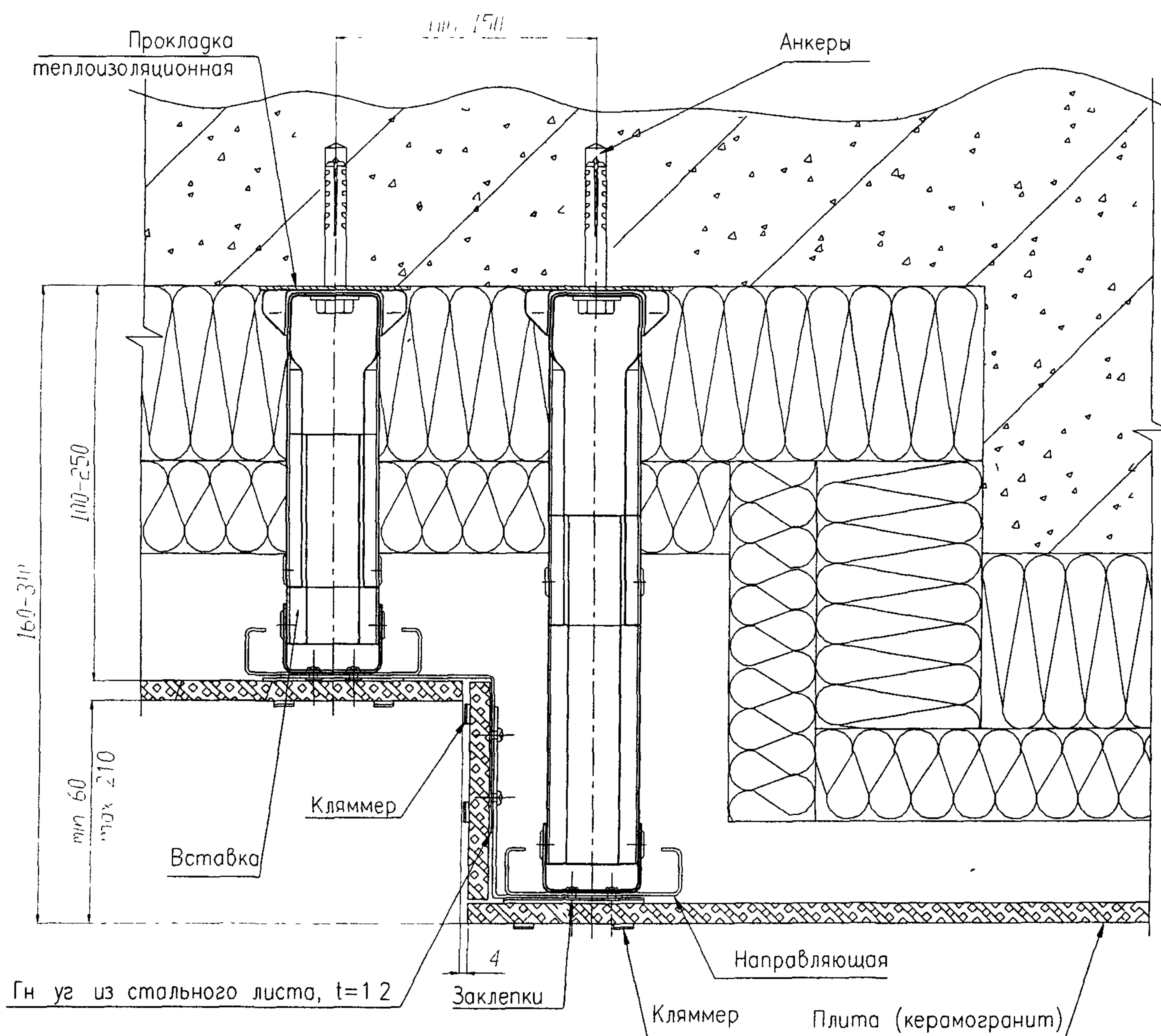
Рис.В.8. Узел облицовки стены с вертикальным уступом (СО-01).
