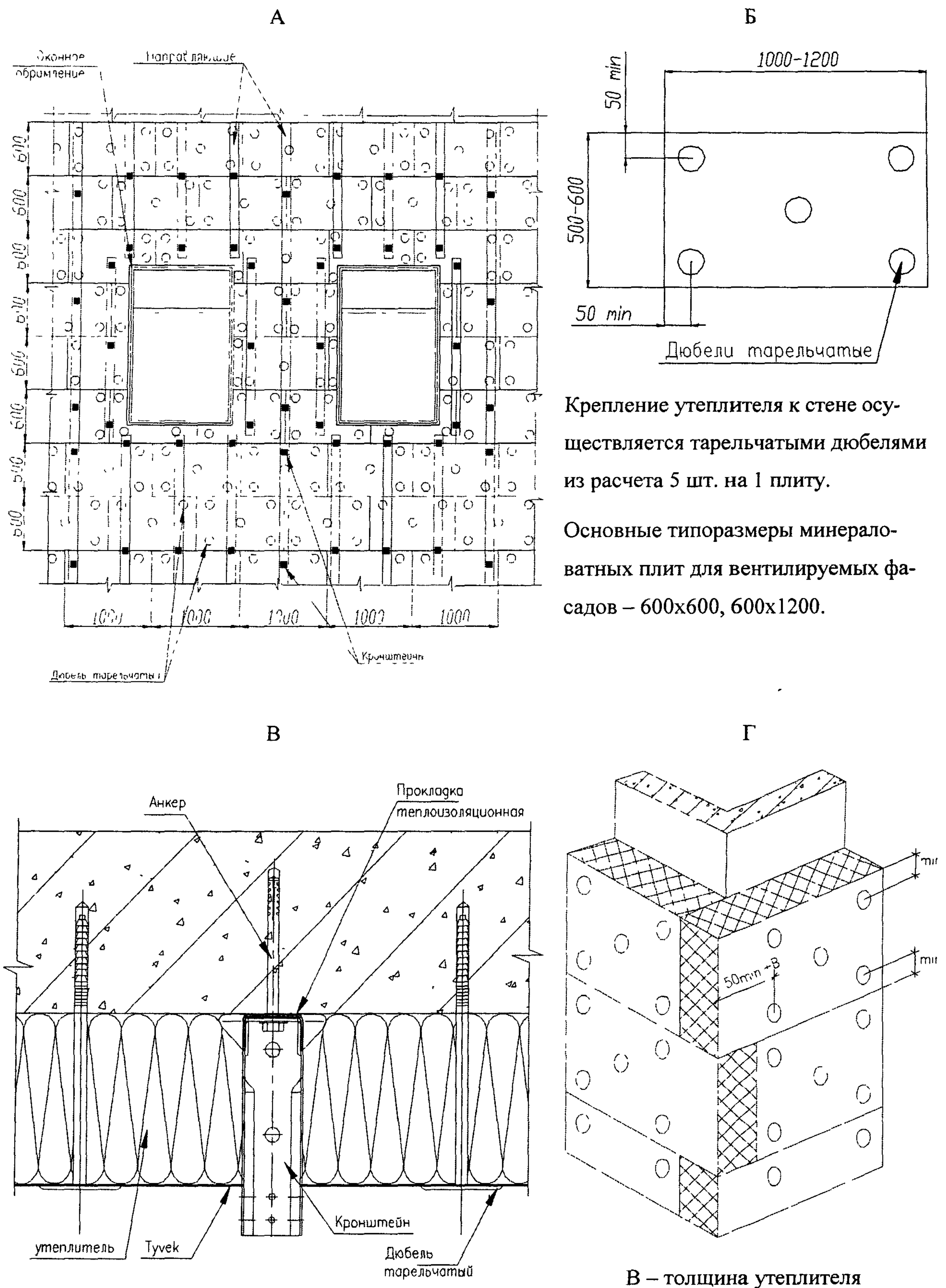
Рис.В.4. Принципиальная схема установки утеплителя (А); схема крепления утеплителя (минераловатные плиты) (Б); узел крепления утеплителя (В); схема крепления утеплителя на углу здания (Г).
