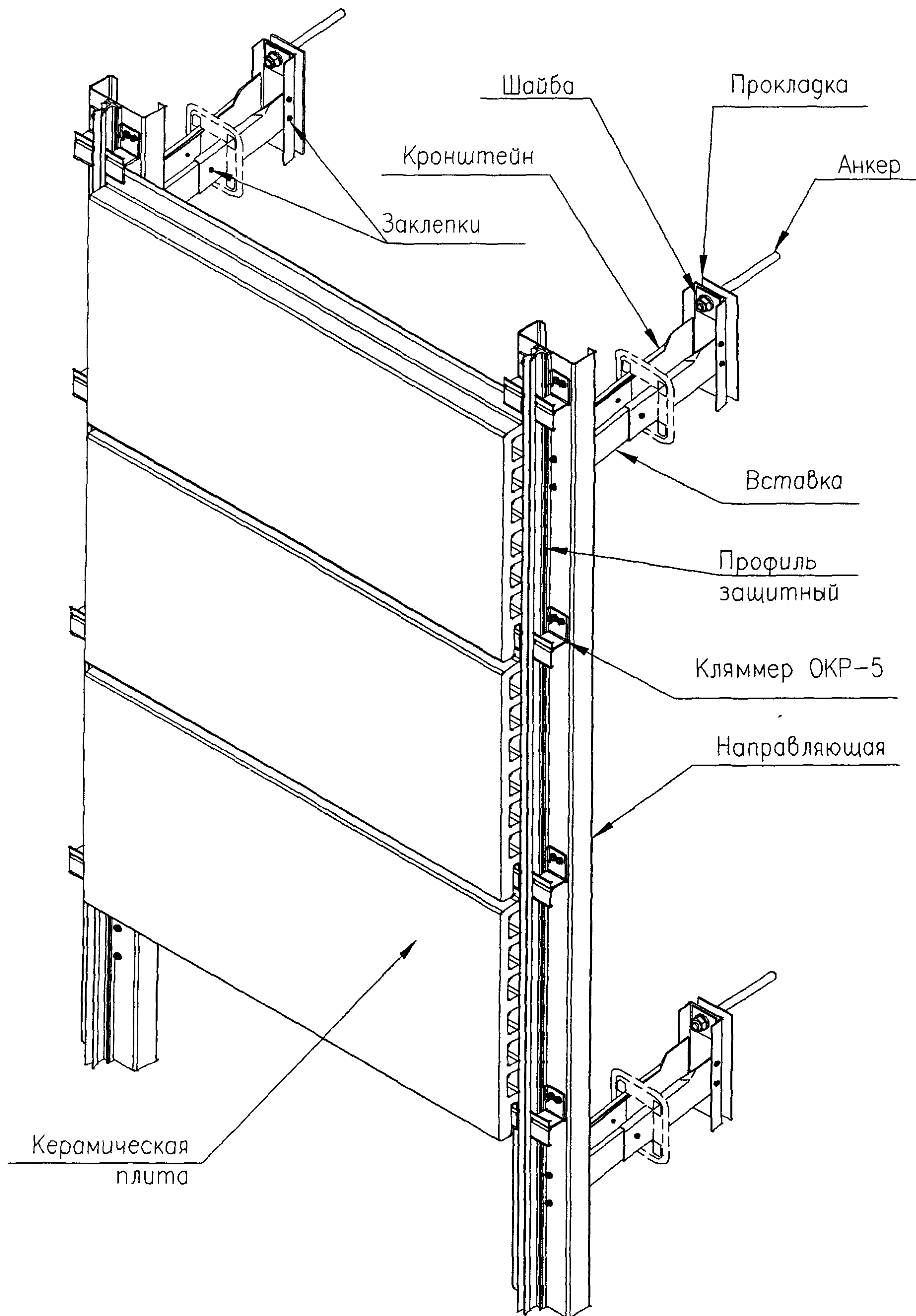
Рис.Б.10. Принципиальная схема фрагмента фасадной конструкции с облицовкой керамическими плитами (скрытое крепление с использованием кляммеров).
