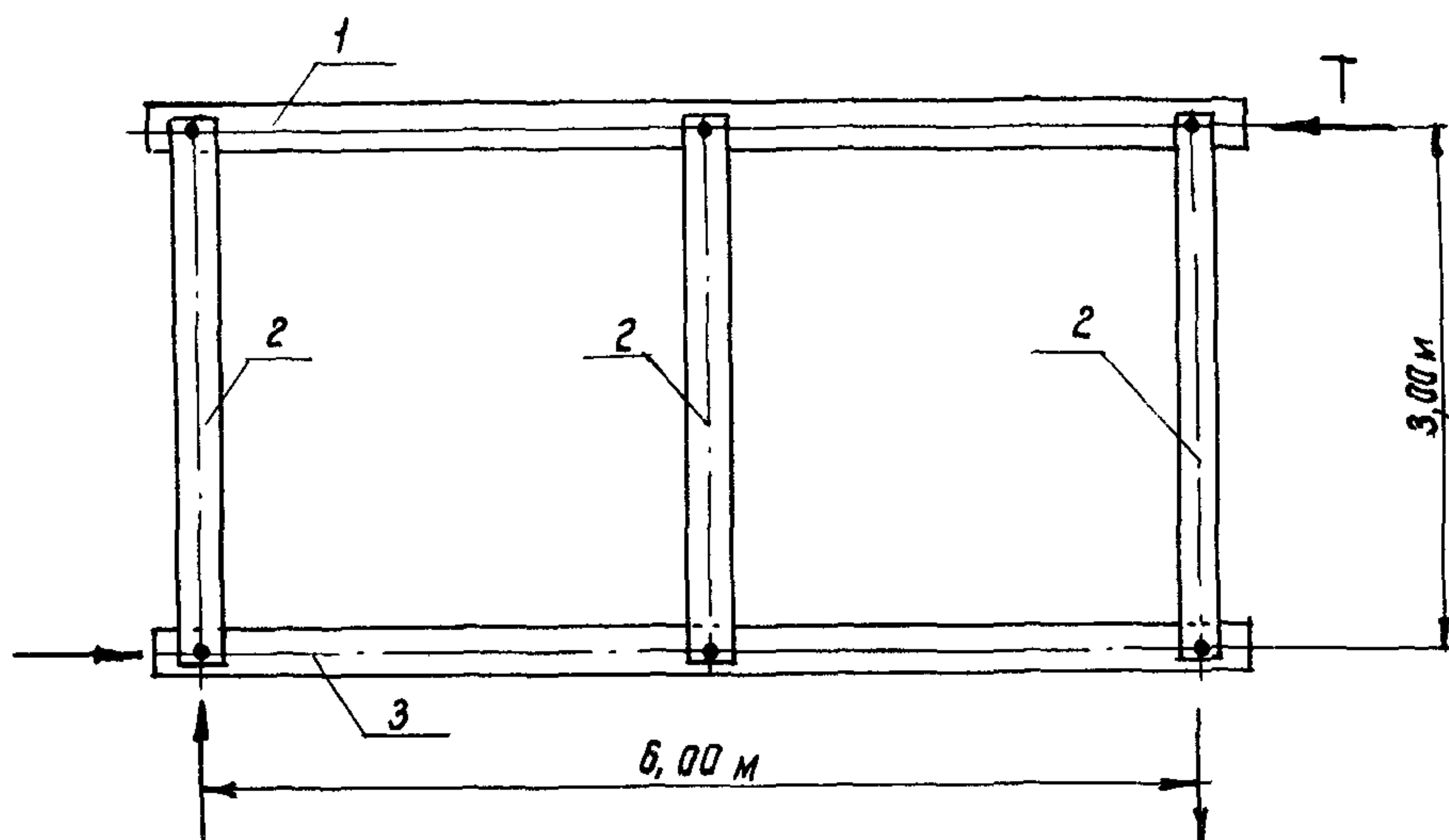
Рис. I. Схема силовой установки 1 – подвижная сторона 2 – поперечина 3 – неподвижная сторона
