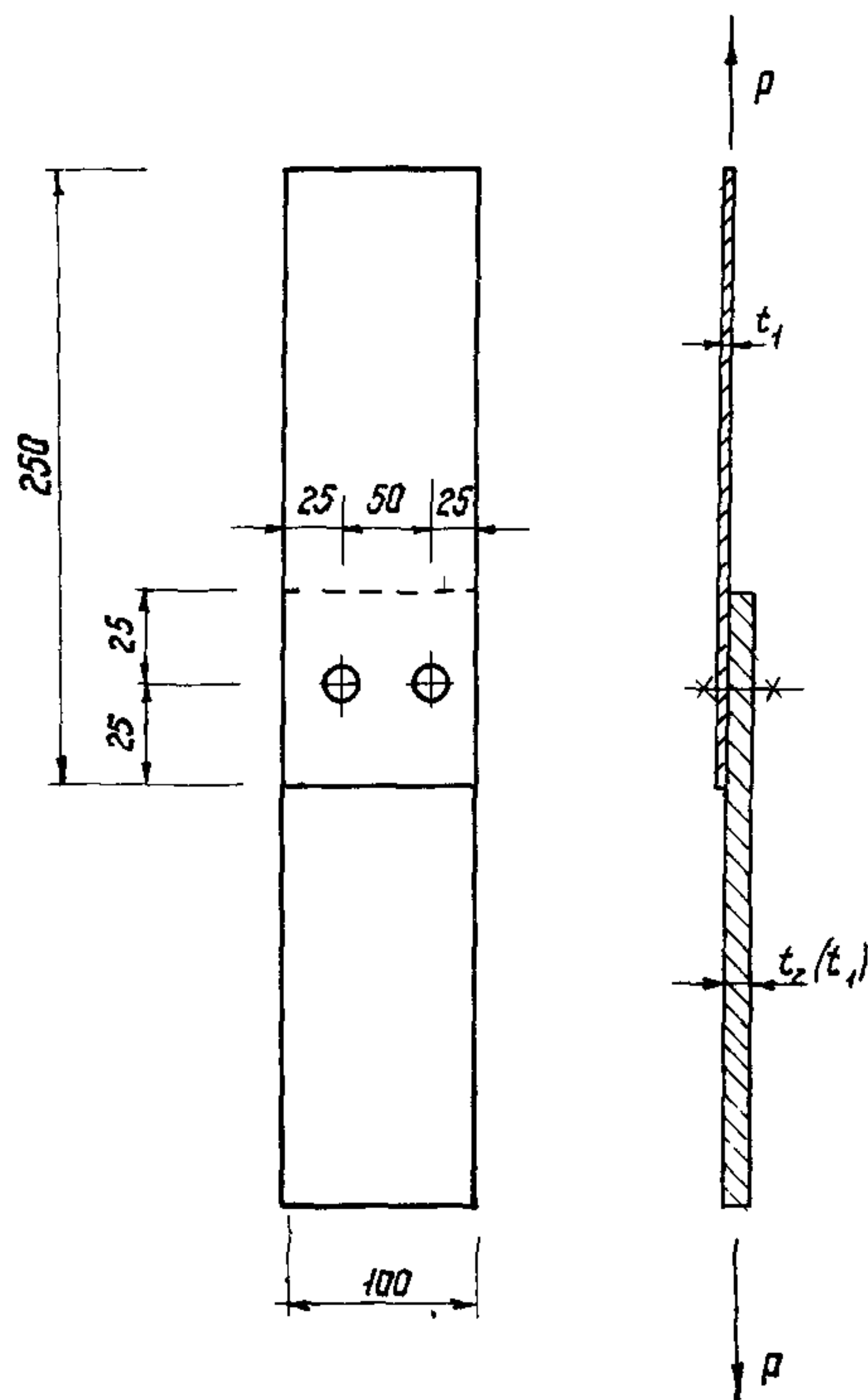
Рис.2. Образец для испытаний соединений настила
