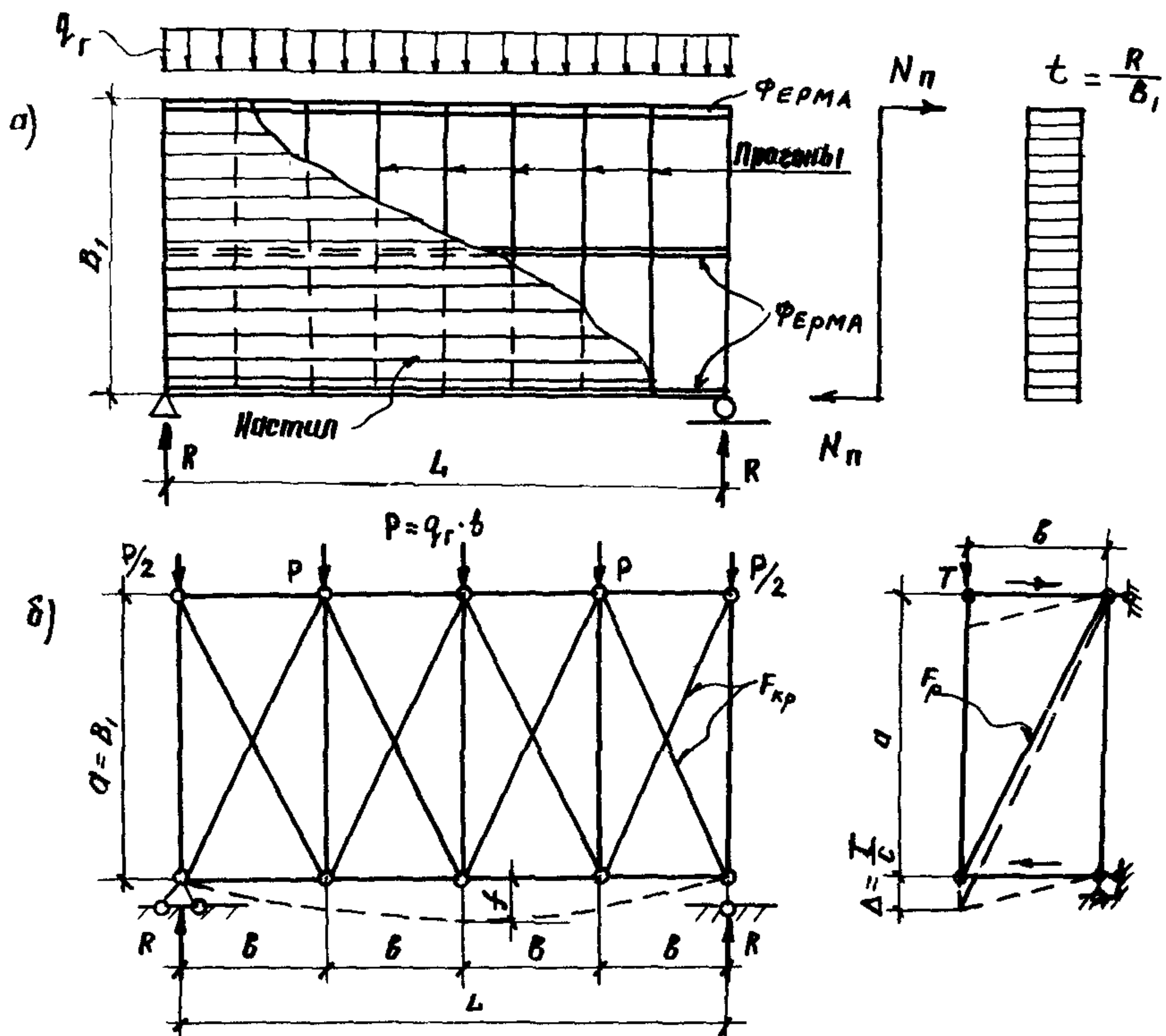
Рис. 4. Расчетная схема поперечной диафрагмы:
