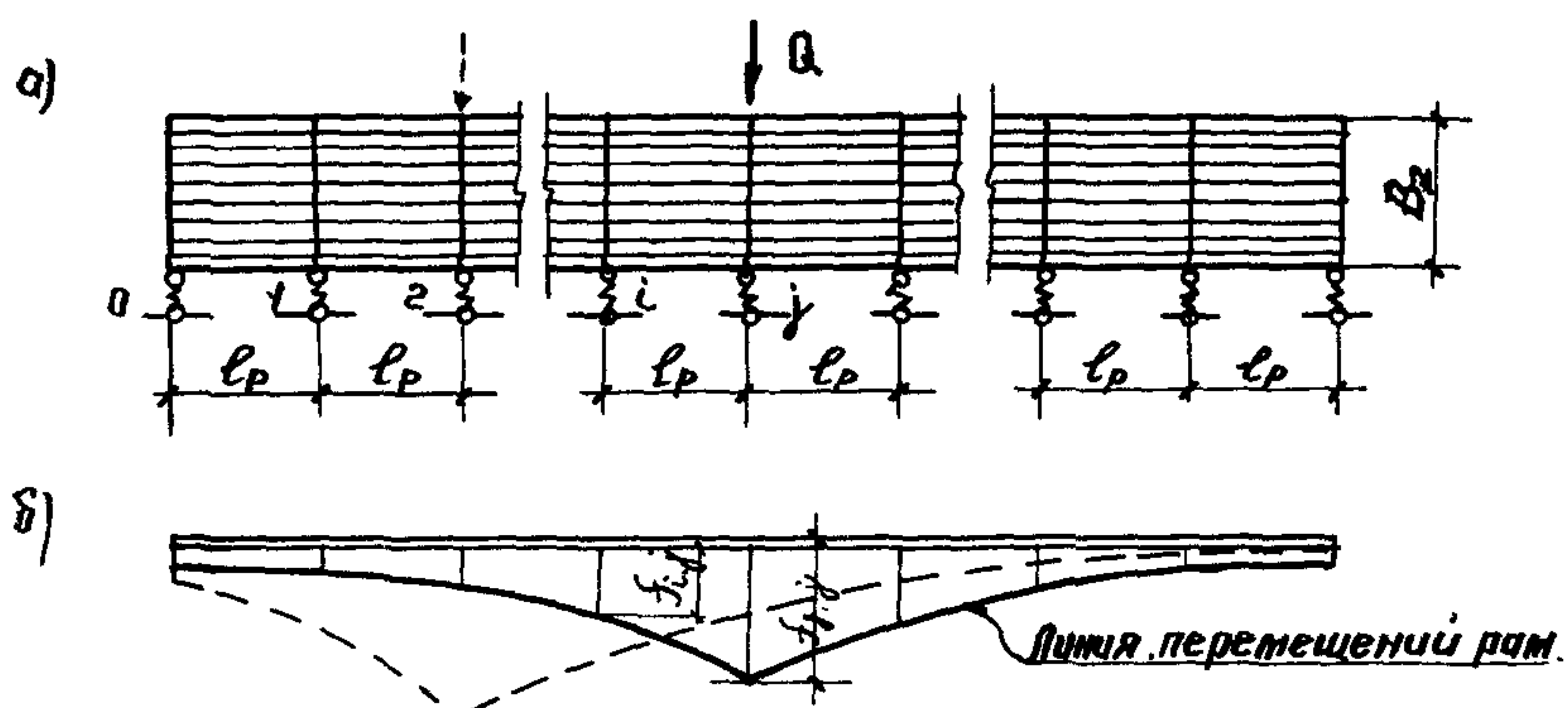
Рис. 5. Расчетная схема продольной диафрагмы:
