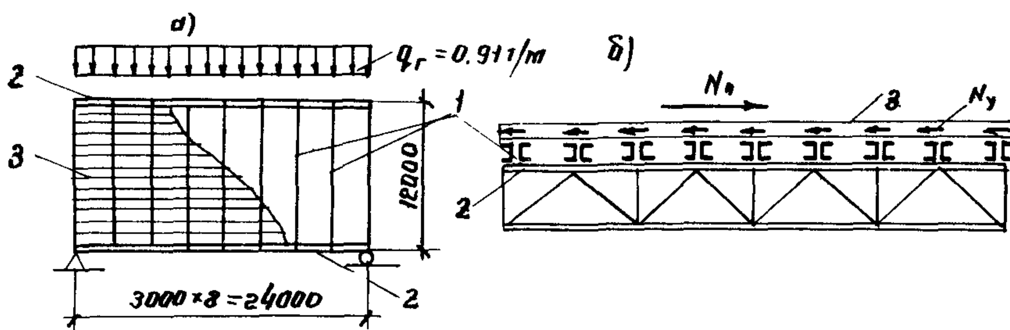
Рис. 2. Расчет поперечной диафрагмы:
