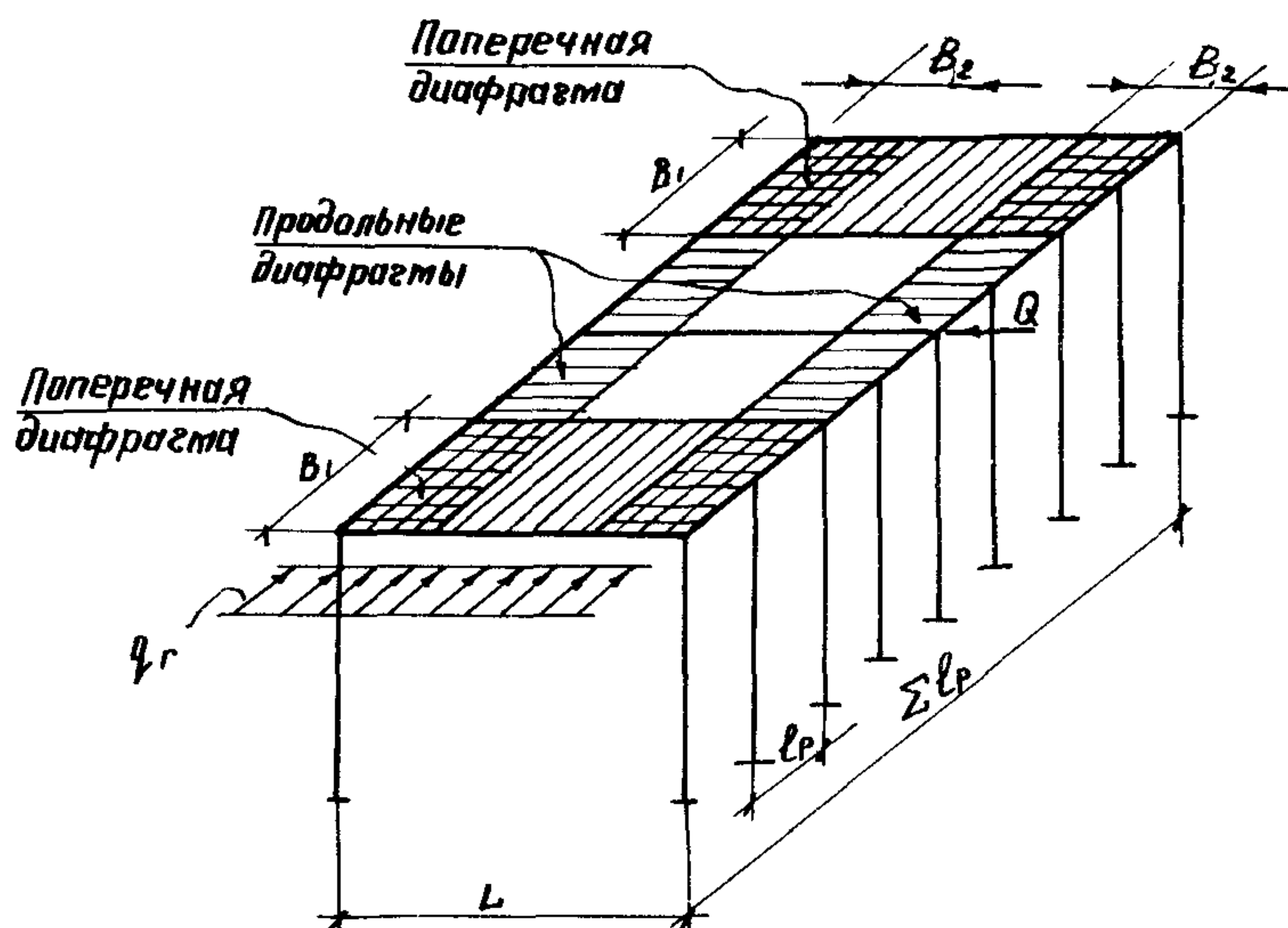
Рис. I. Расчетная схема здания (отсека) с продольными и поперечными диафрагмами.
