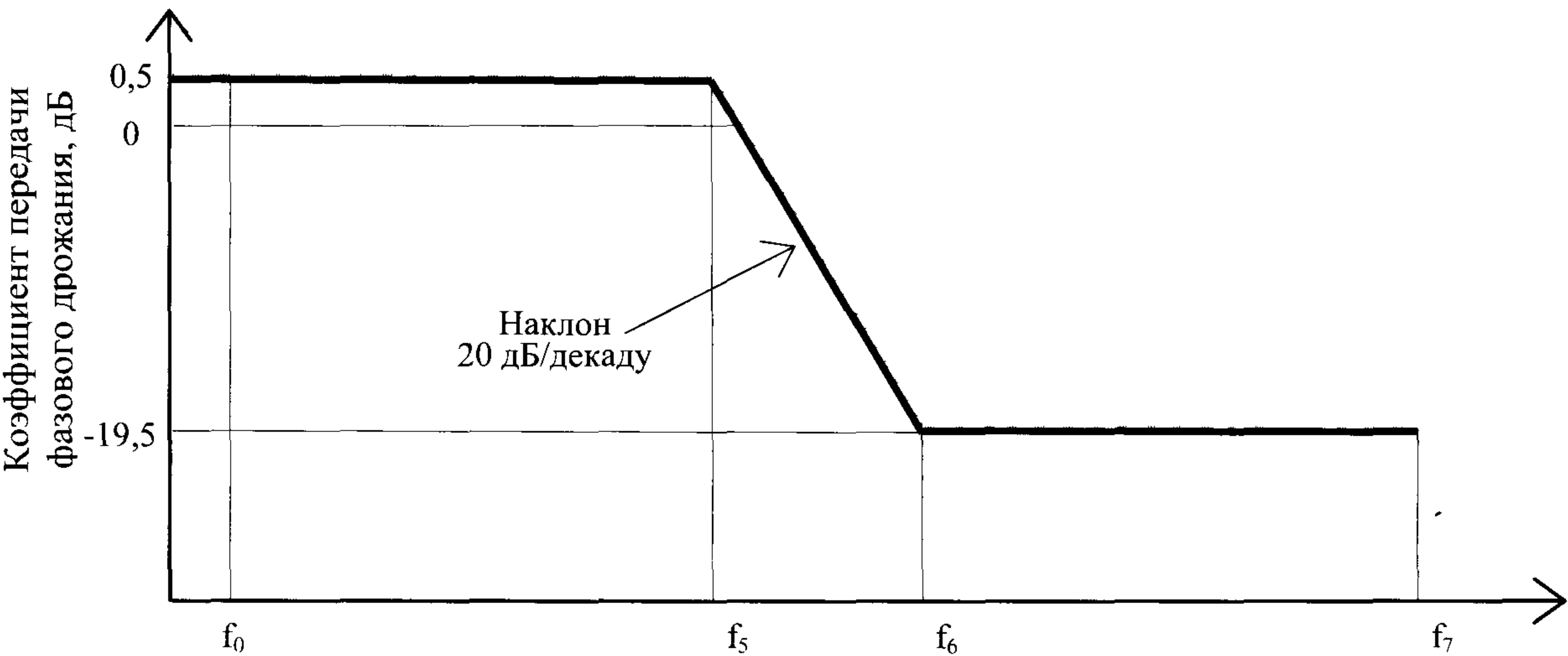
Рисунок 4. Частота фазового дрожания, логарифмическая шкала
