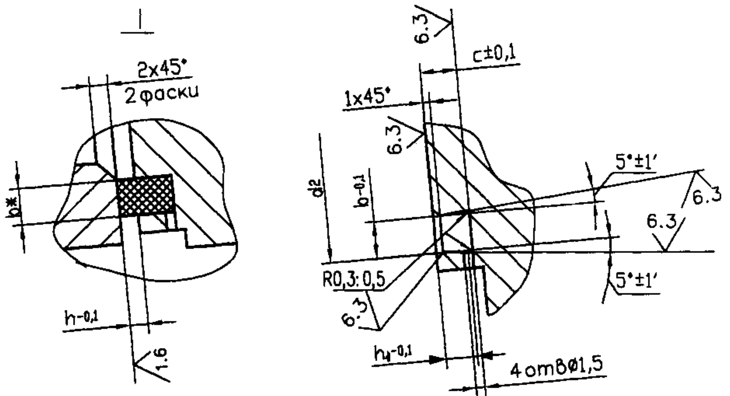
Разделка паза под кольцо
