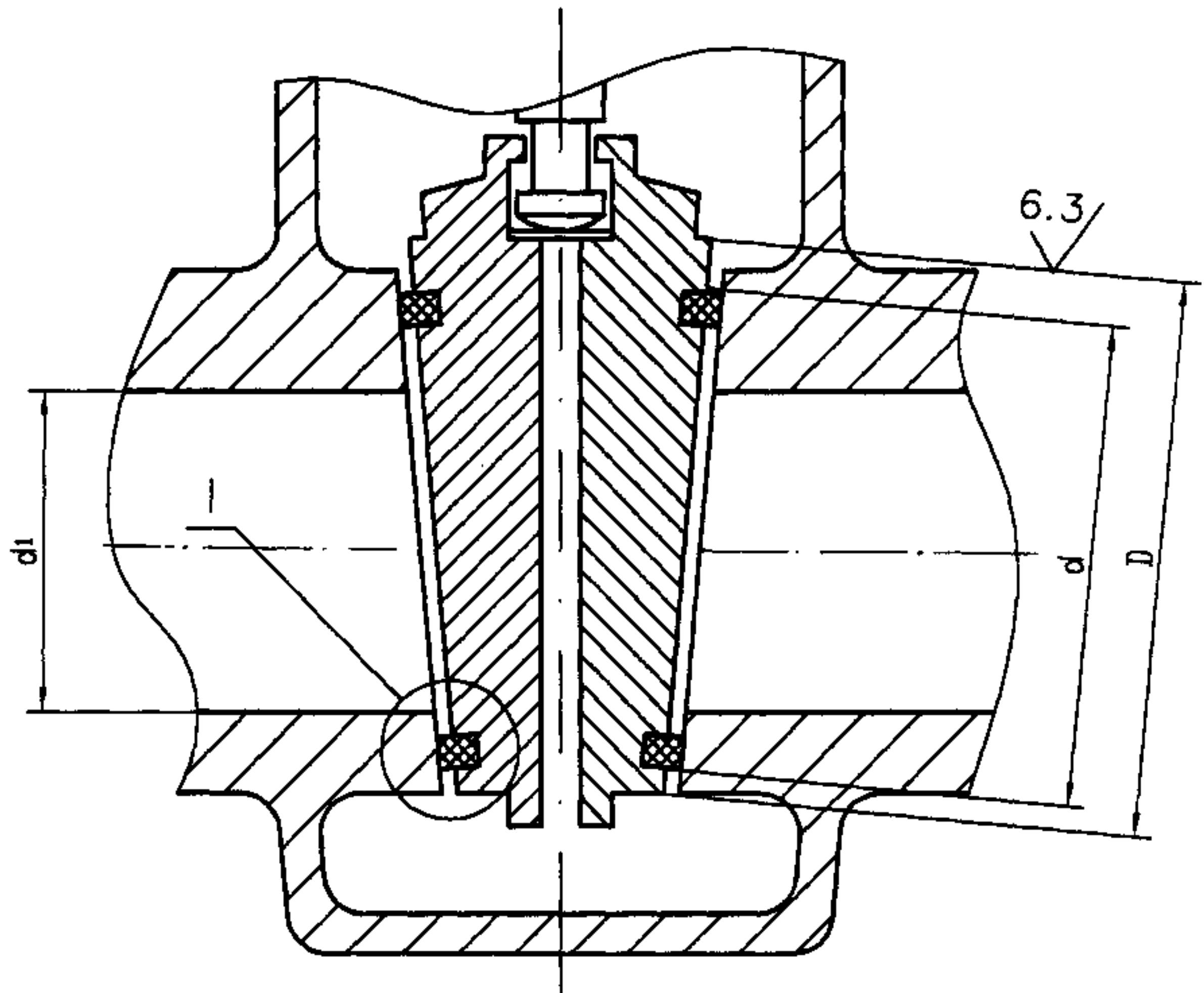
Разделка паза под кольцо
