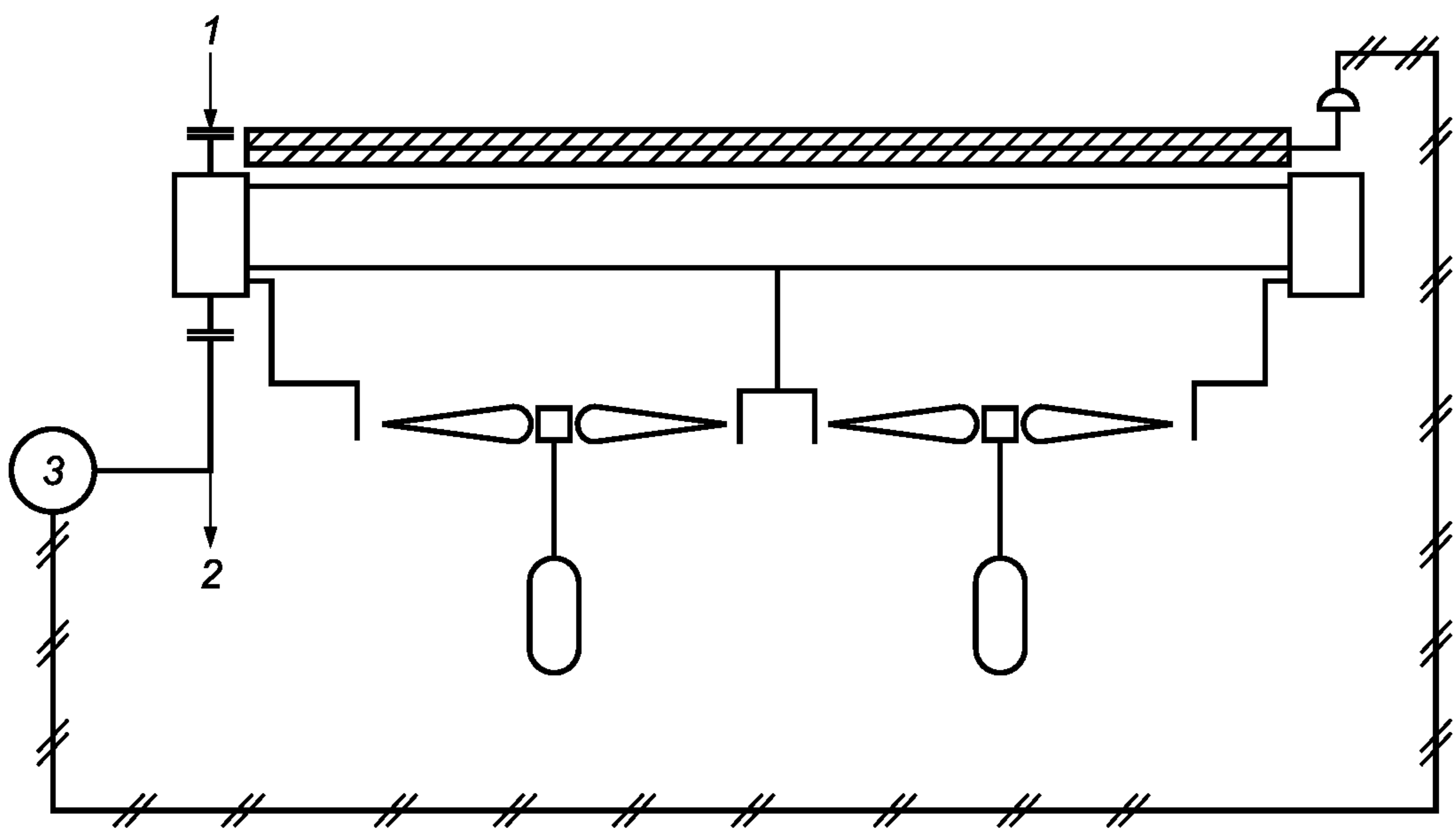
1 — вход технологической среды; 2 — выход технологической среды; 3 — контроллер с индикацией температуры Примечание — Воздухоохлаждаемый теплообменник может быть с нагнетательной или отсасывающей тягой.
