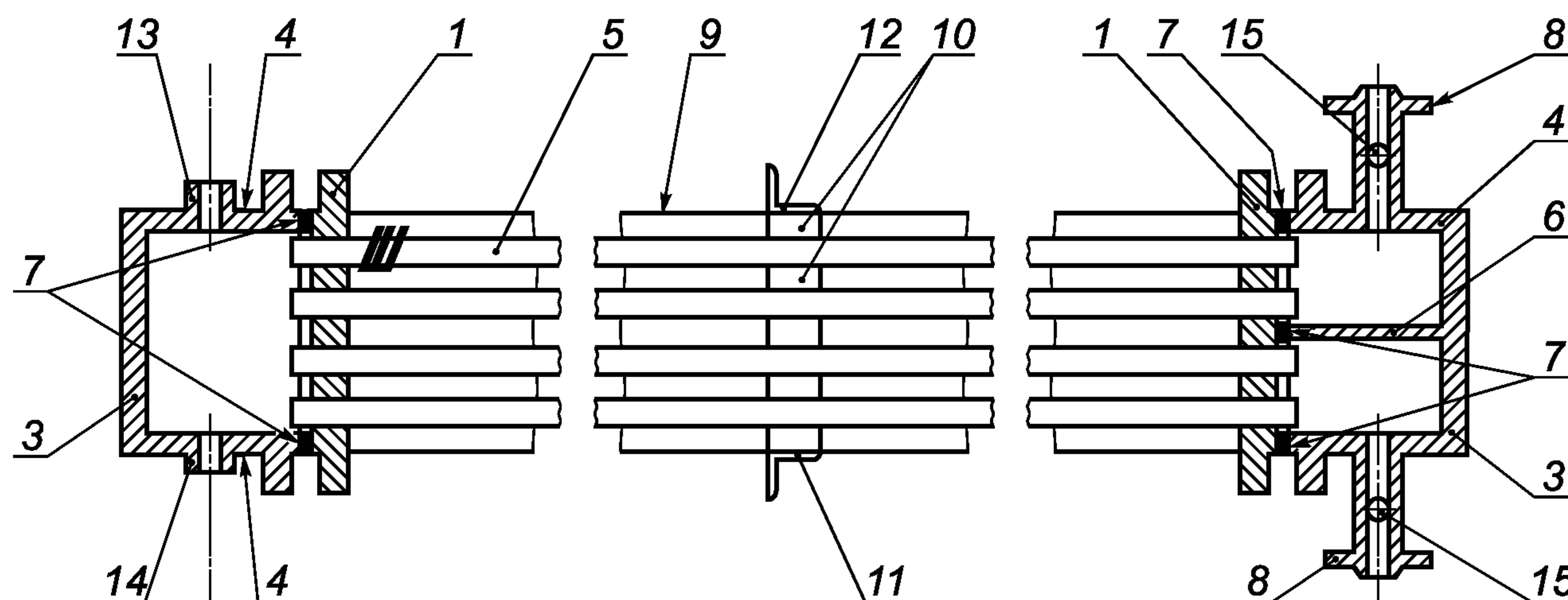
б — коллектор со съемным колпаком
