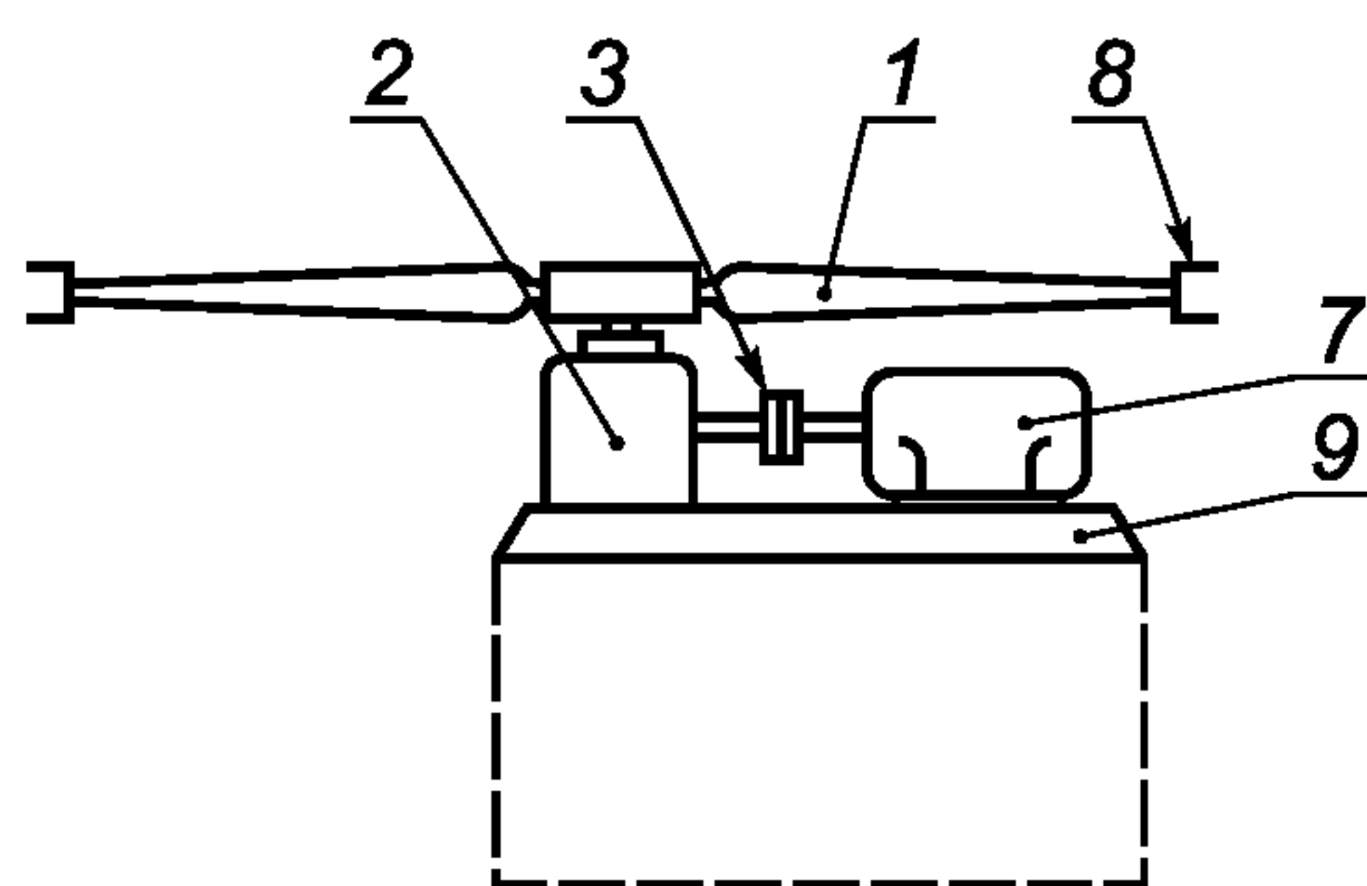
a - привод с прямой ортогональной зубчатой передачей
