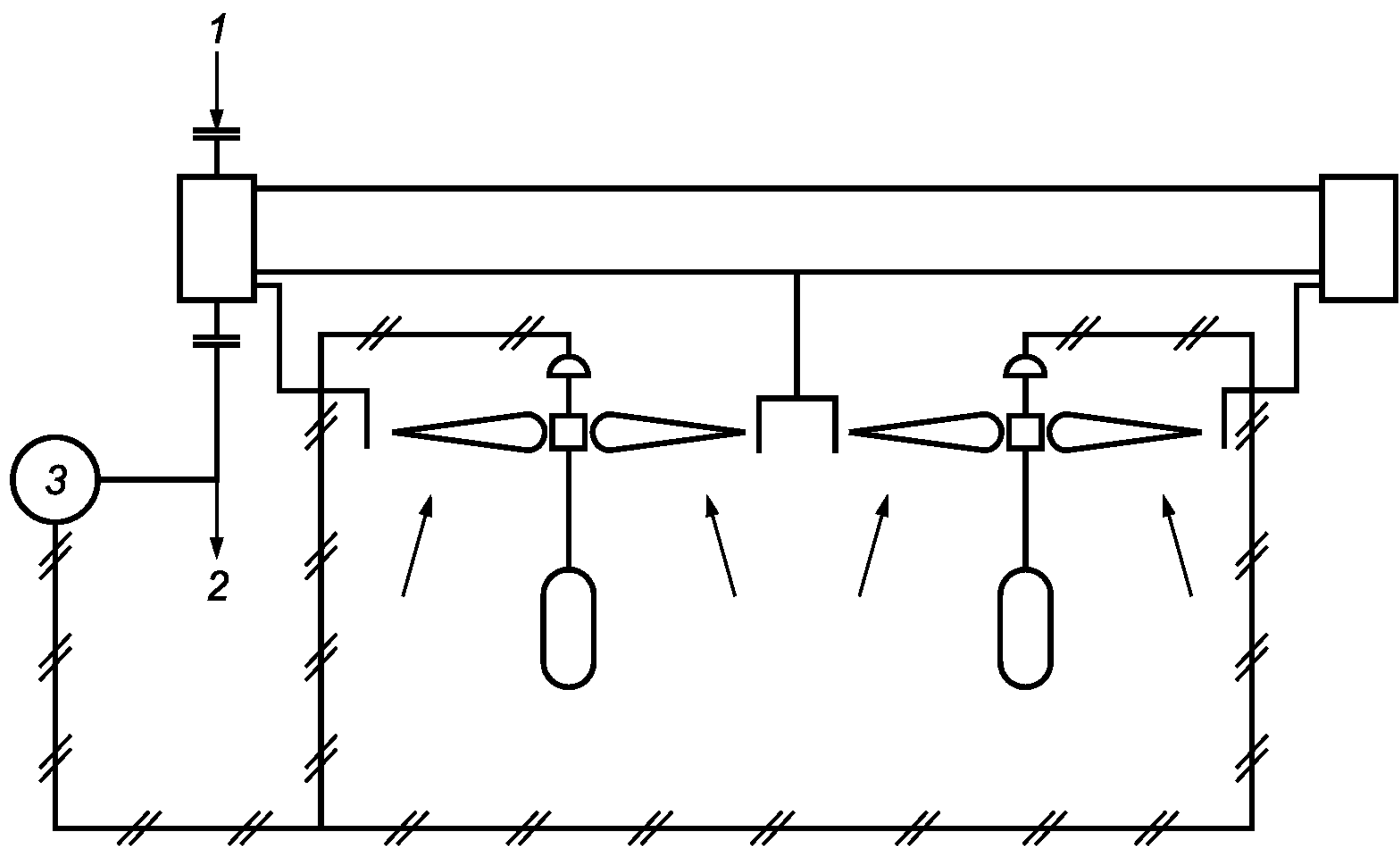
1 — вход технологической среды; 2 — выход технологической среды; 3 — контроллер с индикацией температуры Примечание — Воздухоохлаждаемый теплообменник может быть с нагнетательной или отсасывающей тягой.
