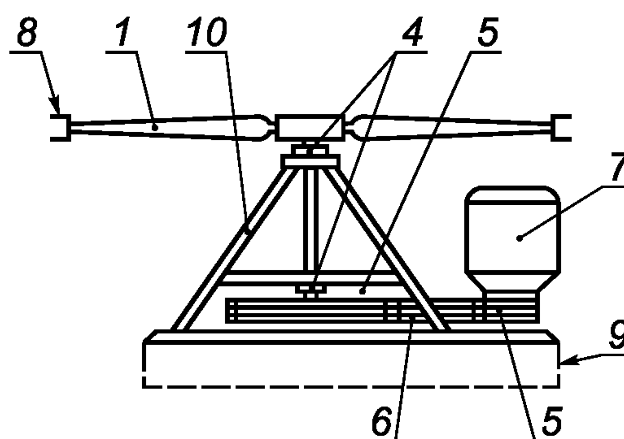
b - ременный привод
