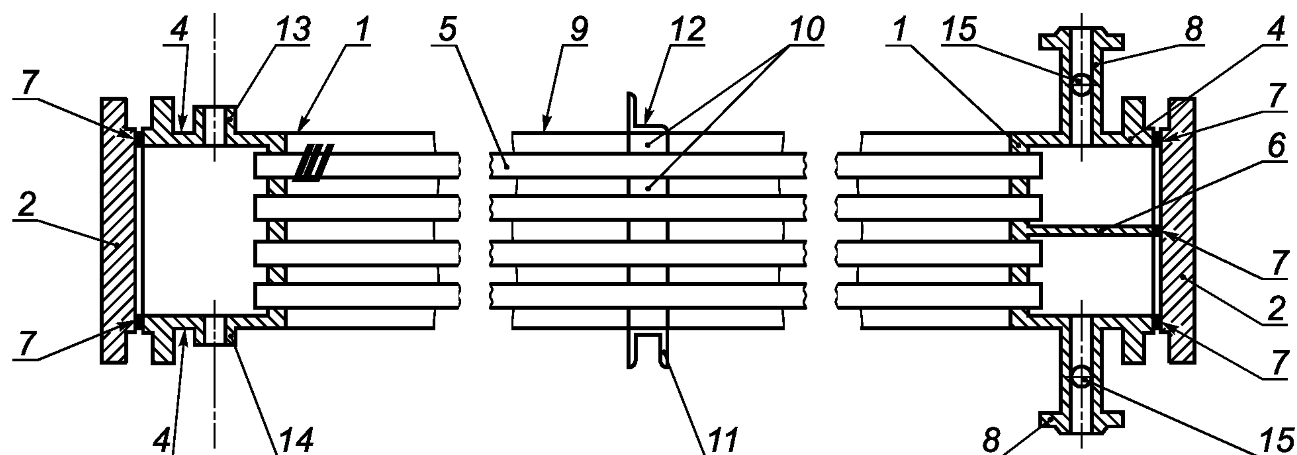
а — коллектор со съемной крышкой
