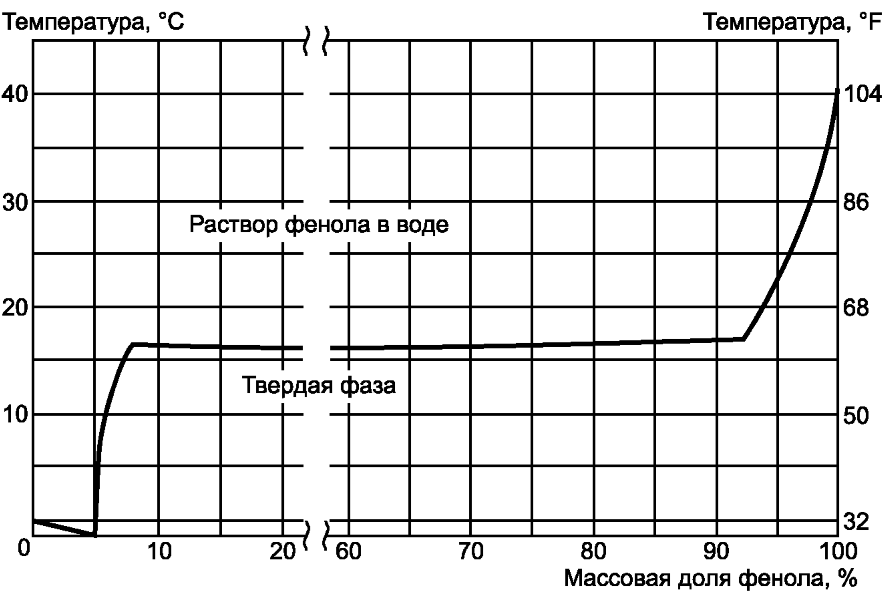
Рисунок С.7 — Точка замерзания водных растворов фенола
