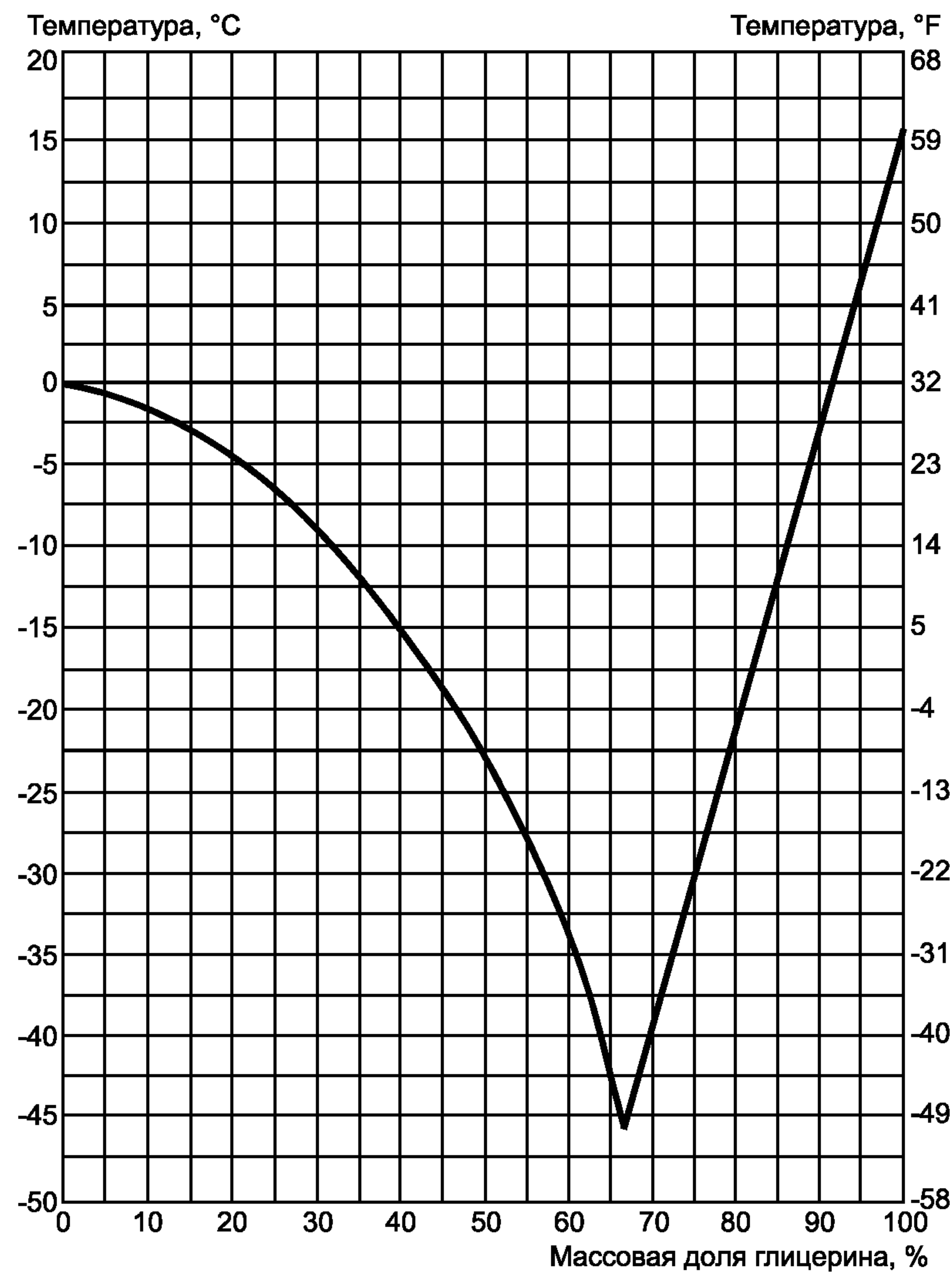
Рисунок С.9 — Точка замерзания водных растворов глицерина
