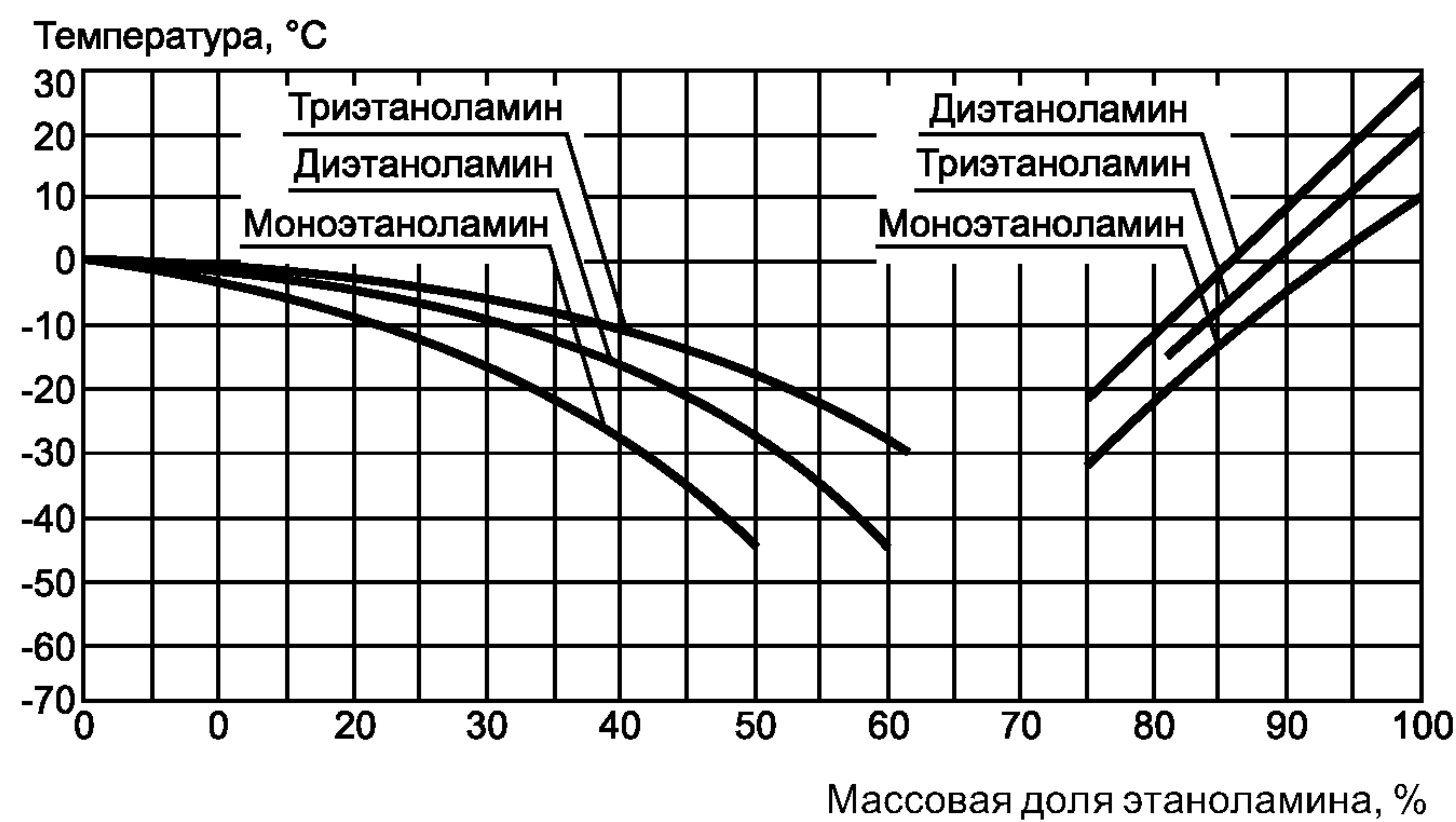
Рисунок С.8 — Точка замерзания водных растворов этаноламина
