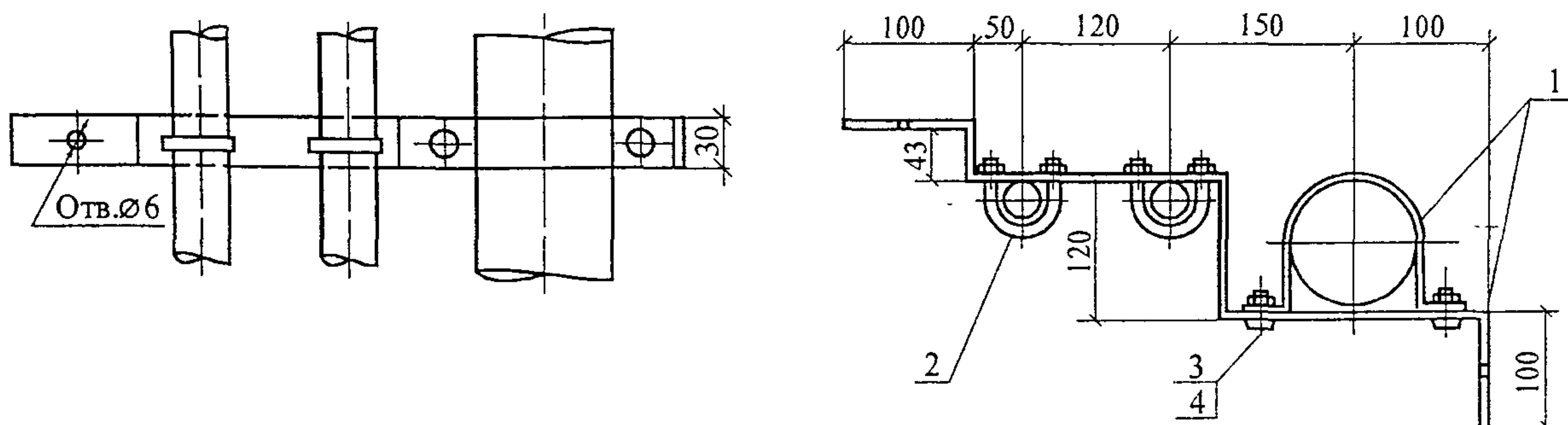
1 – полоса 4×38; 2 – хомут М6; 3 – гайка М6; 4 – болт М6×30
