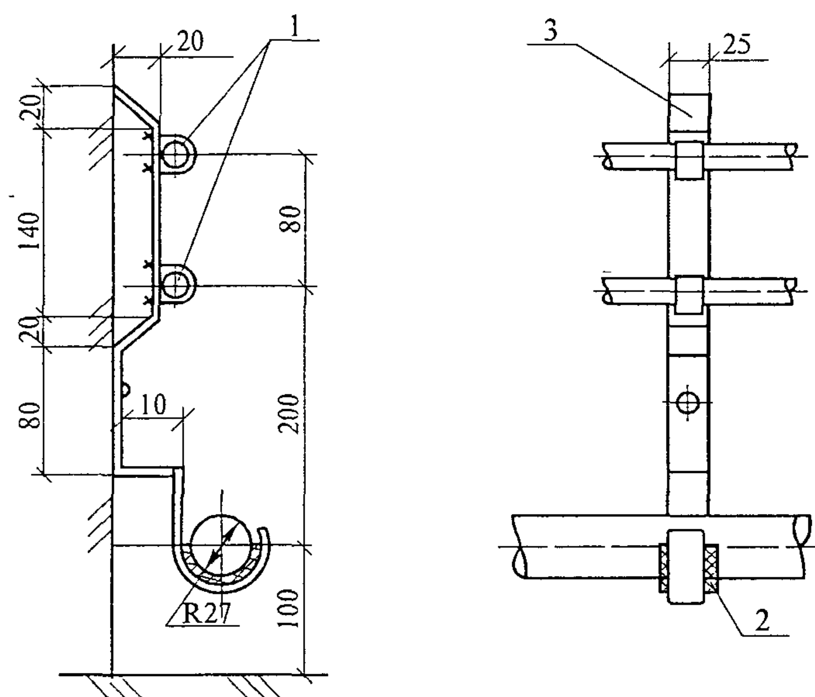
1 – хомут СТД 805; 2 – прокладка резиновая; 3 – лист 3
