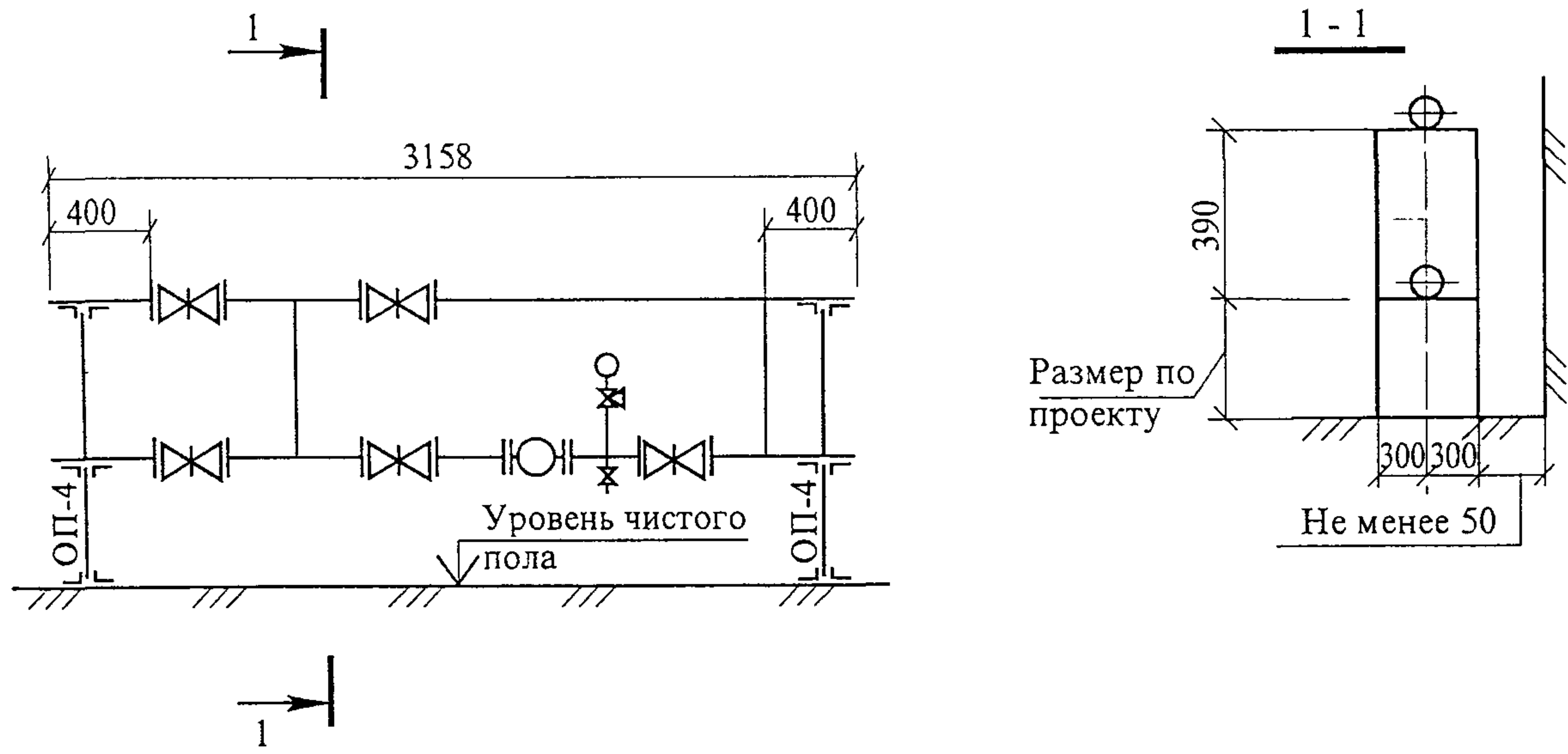
Рисунок 1 – Схема установки водомерного узла № 12
