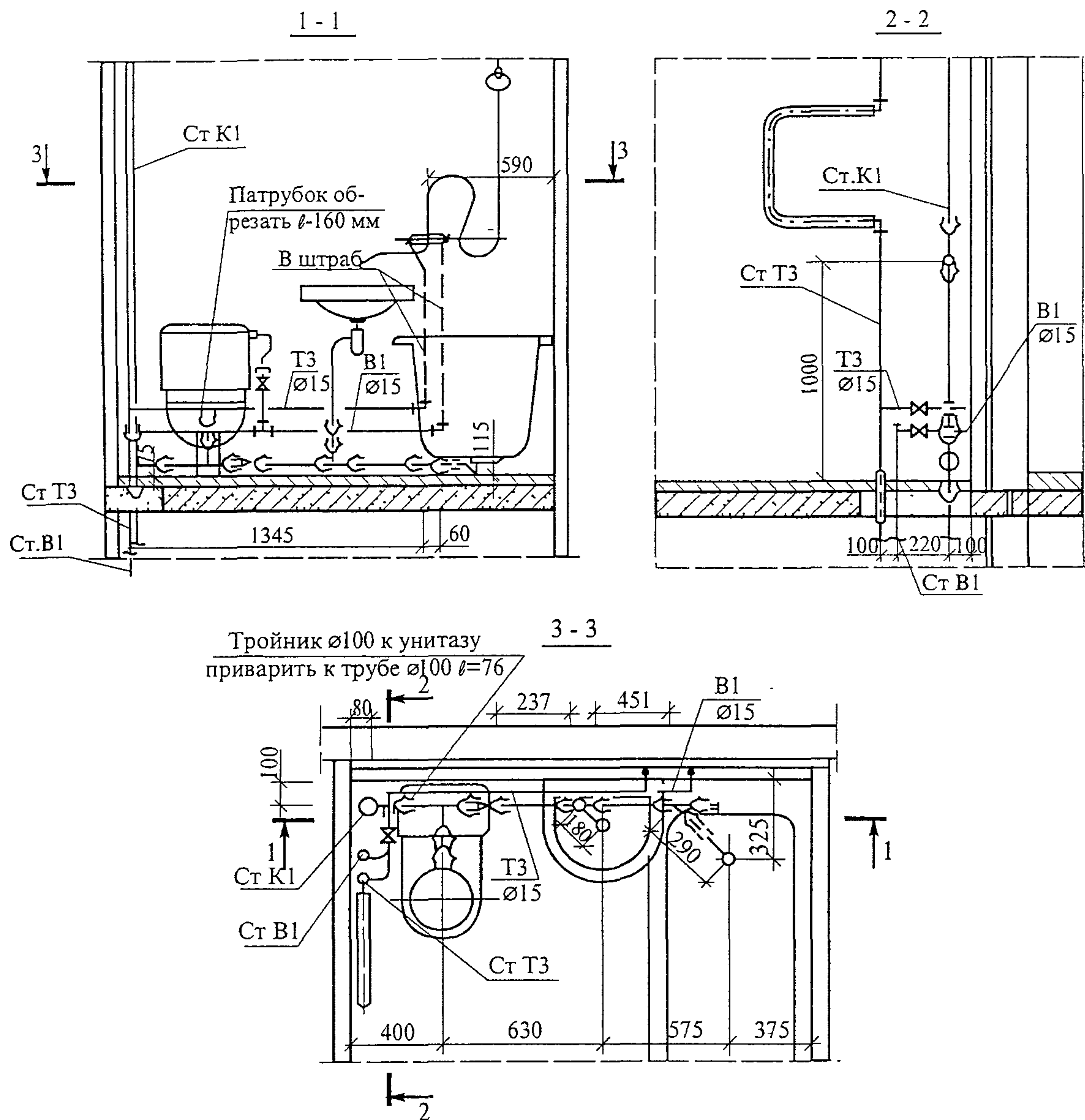
Рисунок 2 – Совмещенный санузел типа ЗСУ пр 02
