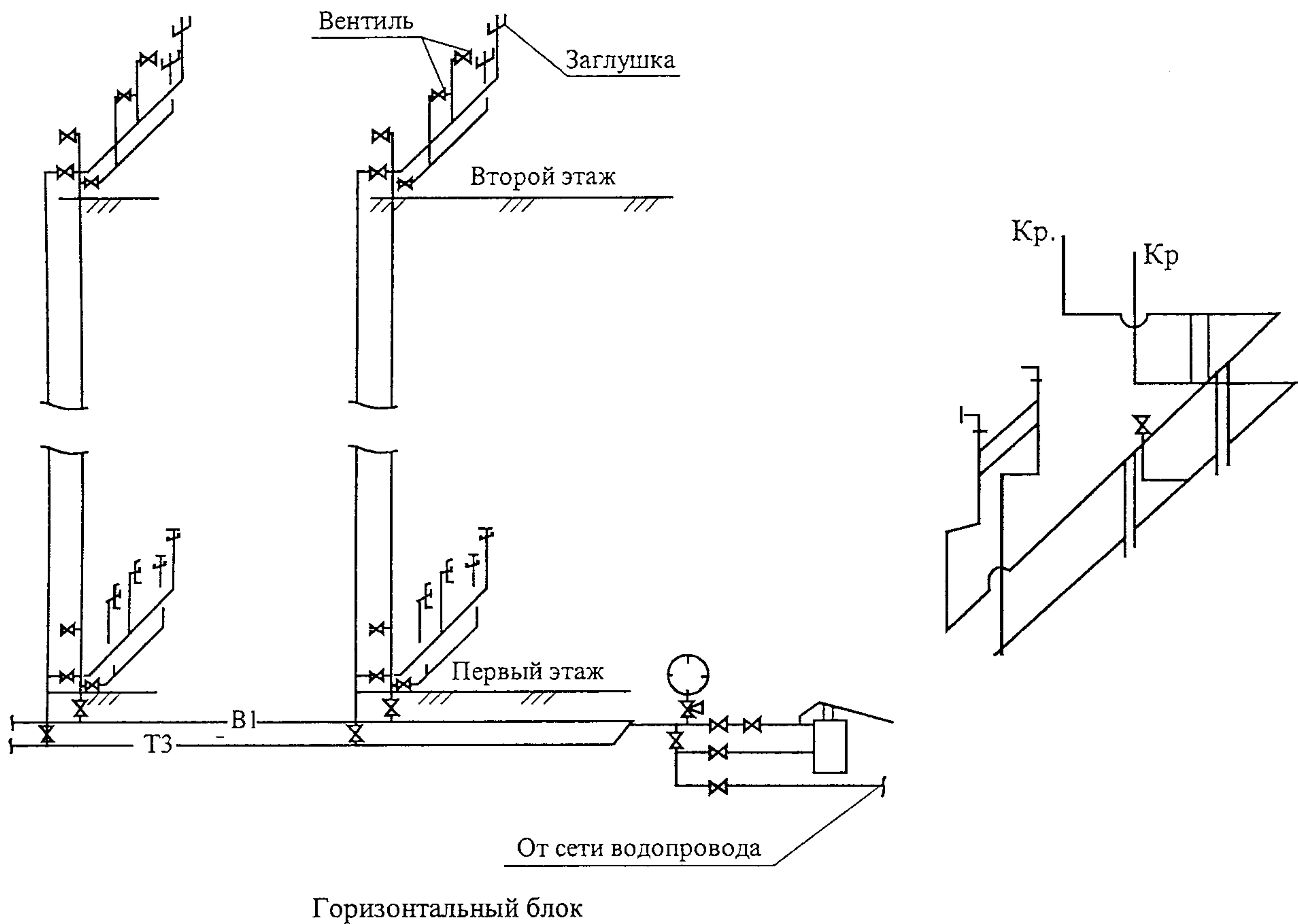
Рисунок 6 – Схема проведения гидростатического испытания
