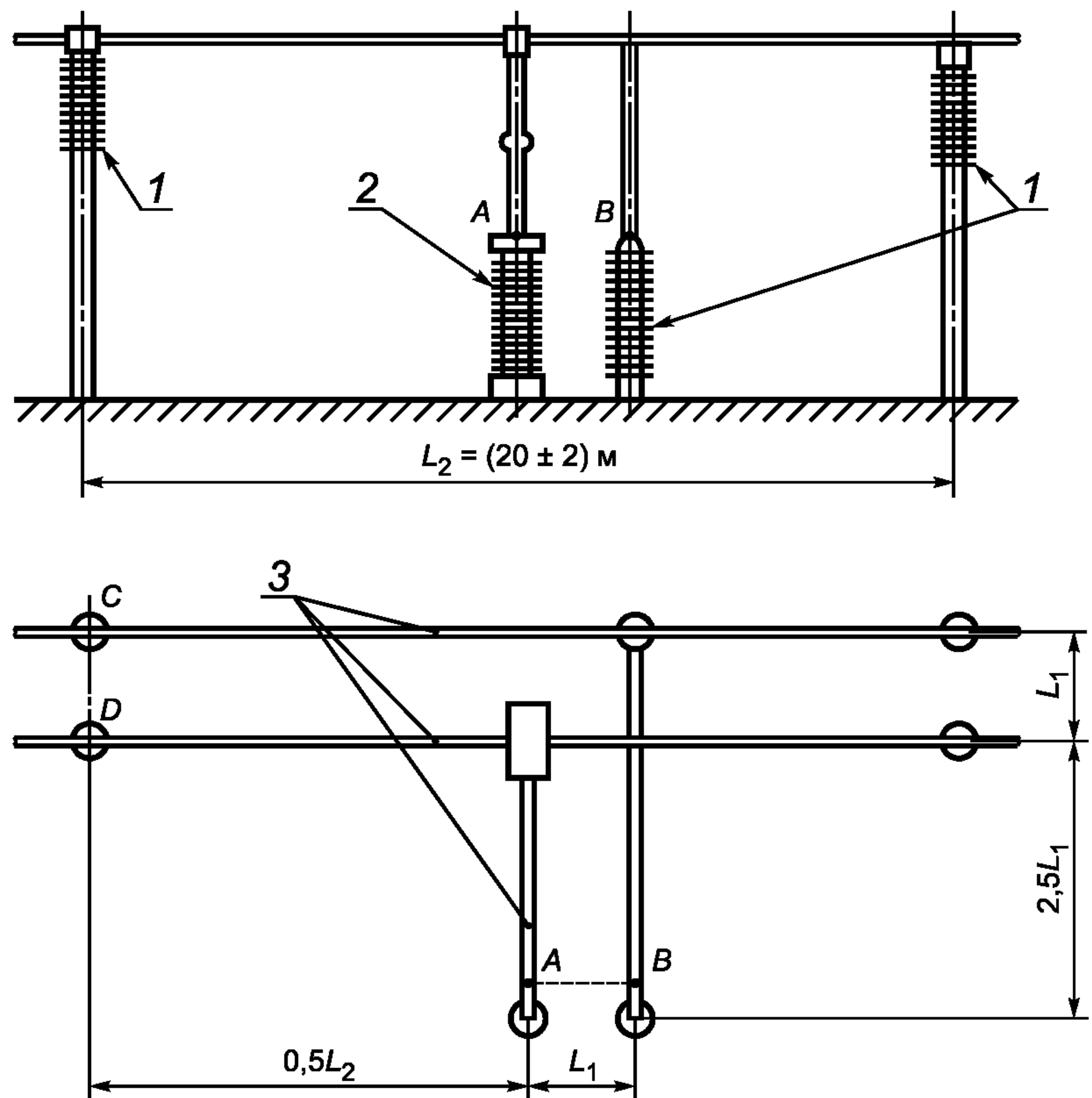
1 — изолирующие опоры; 2 — испытуемый аппарат; 3 — токопроводы; L_1 — минимальное межосевое расстояние между соседними полюсами A—B или C—D — соединение проводников накоротко или с источником жесткой ошиновкой
