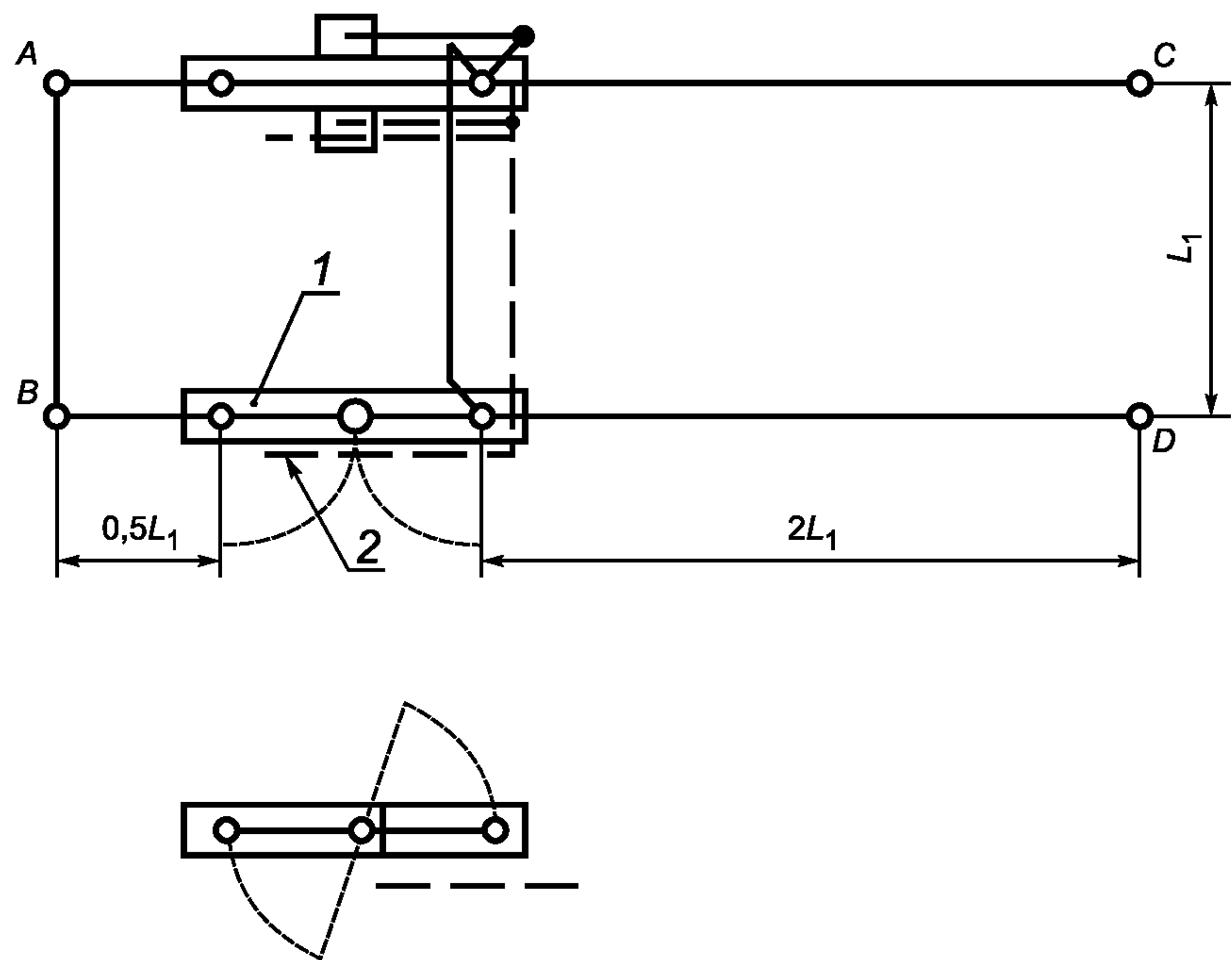
1 — испытуемый разъединитель; 2 — испытуемый заземлитель; A—B — короткозамкнутое соединение; C—D — источник питания; L_1 — минимальное расстояние между осями соседних полюсов
