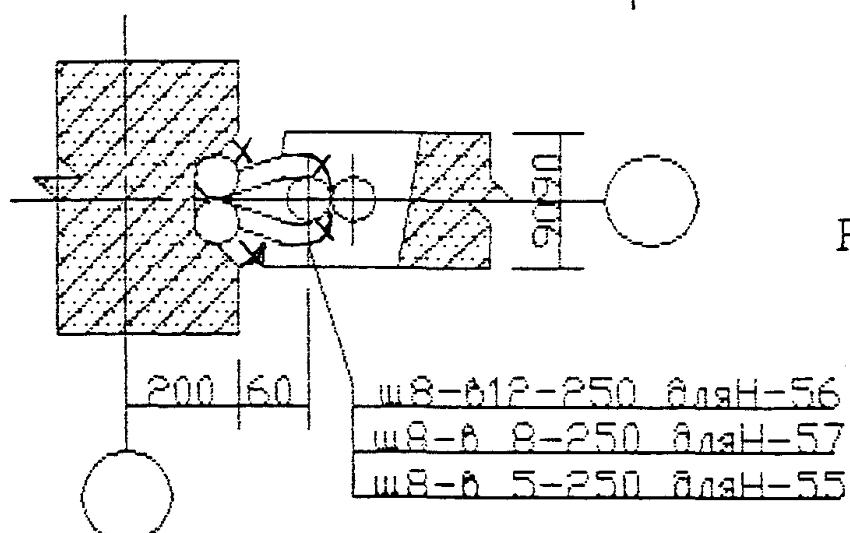
Вариант закладной детали колонн, "Бетипар-22"
