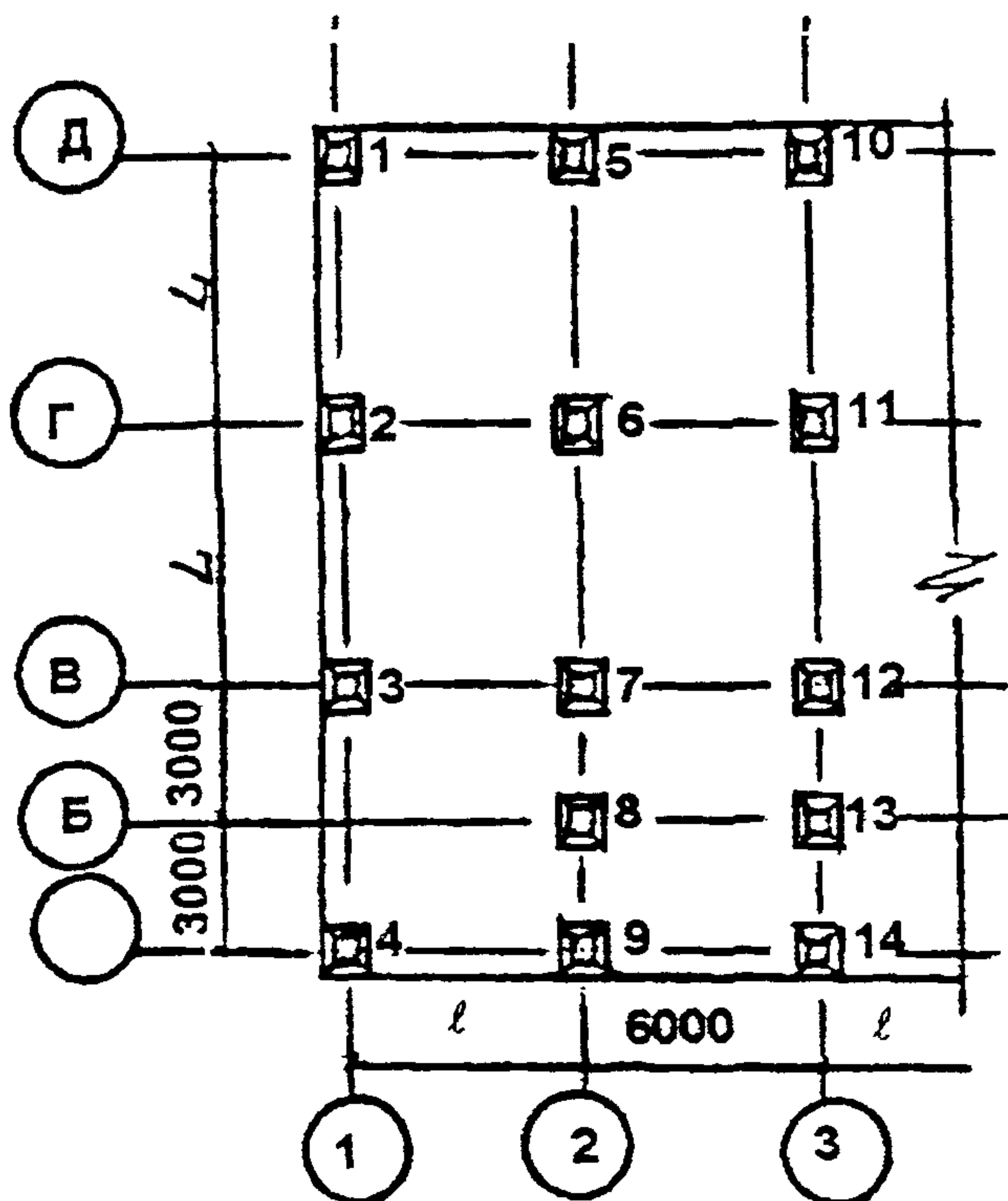
Схема 1 Установка кондукторов
