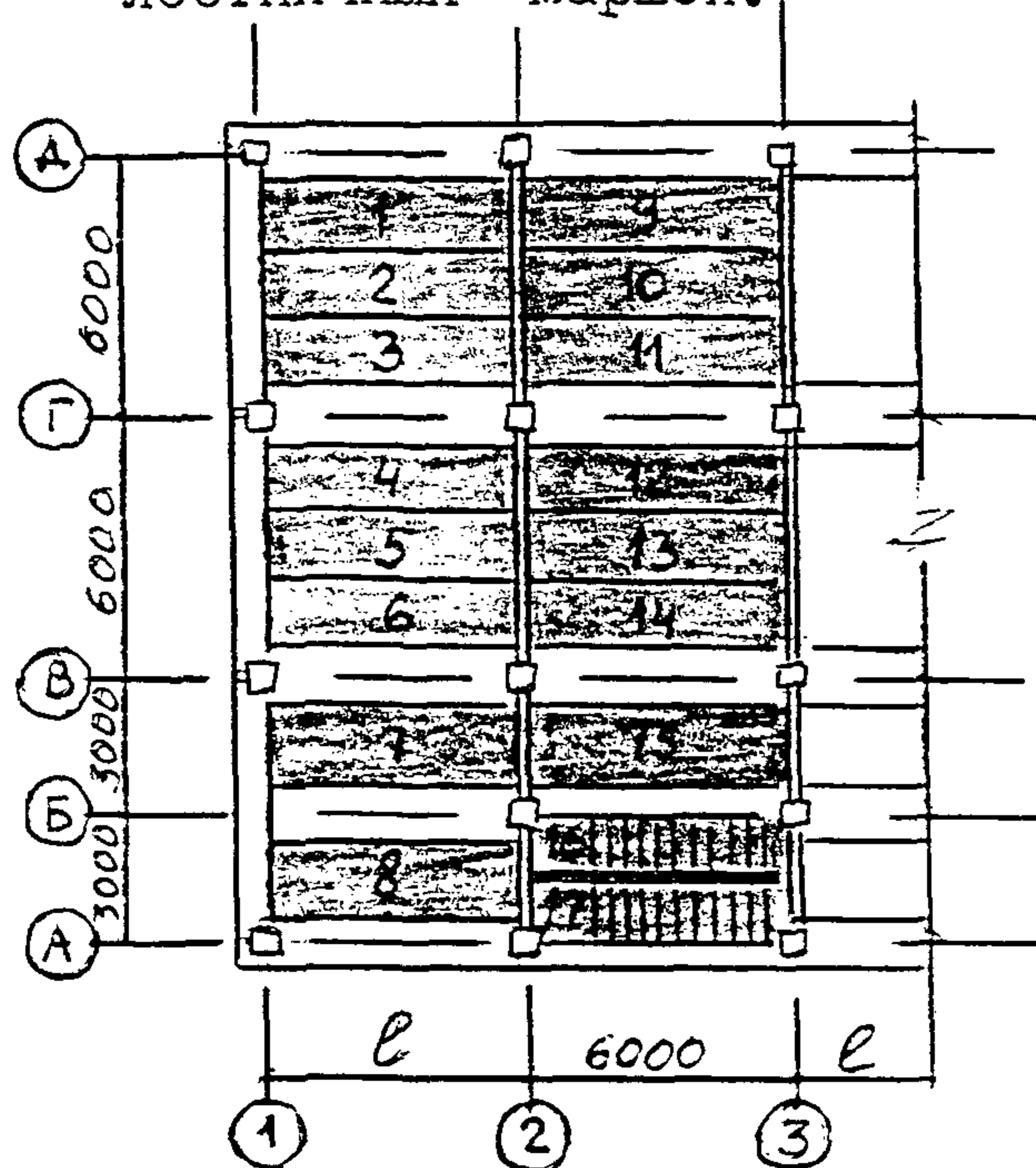
Схема 7. Укладка панелей перекрытия и лестничных маршей.
