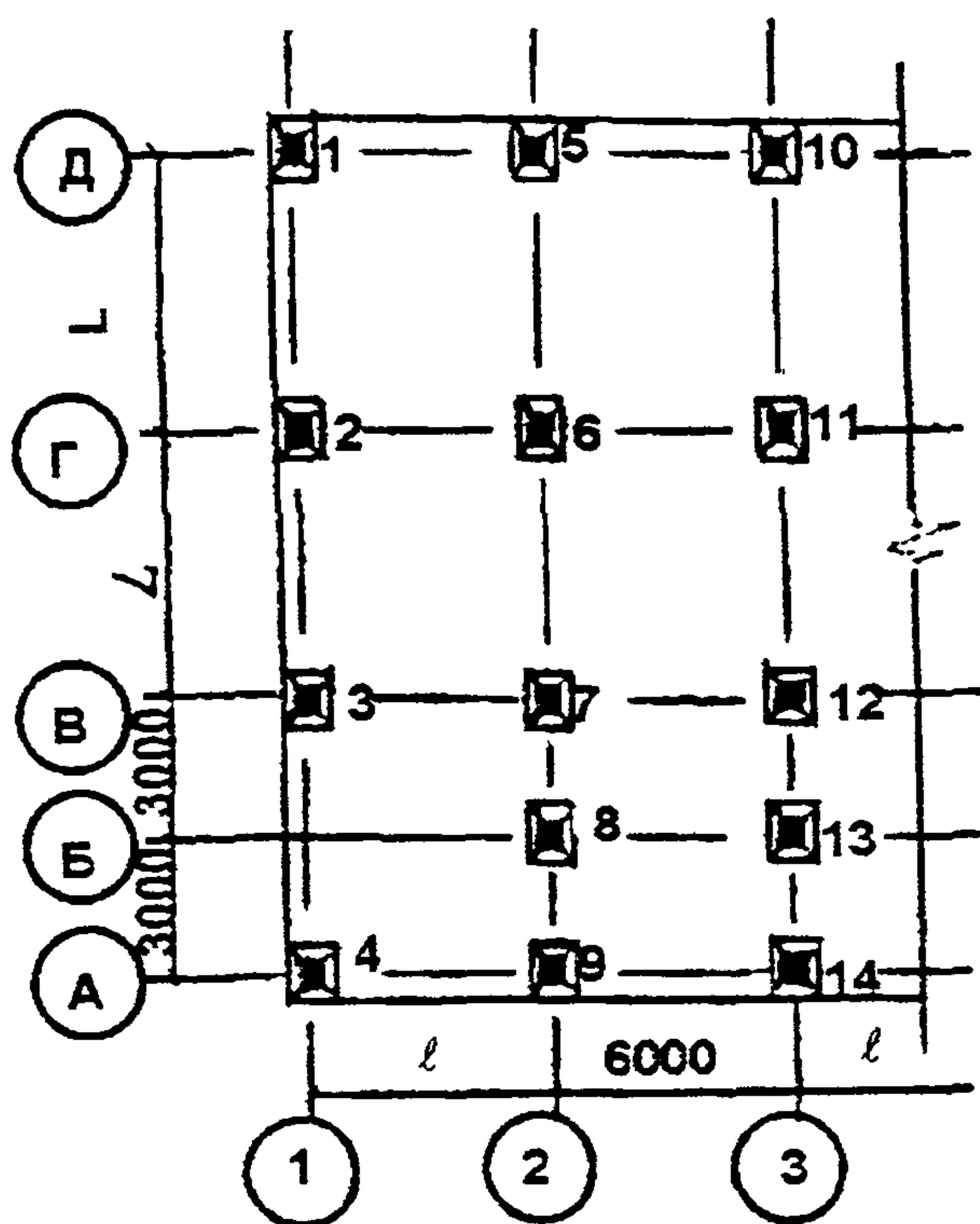
Схема 2 Монтаж колонн
