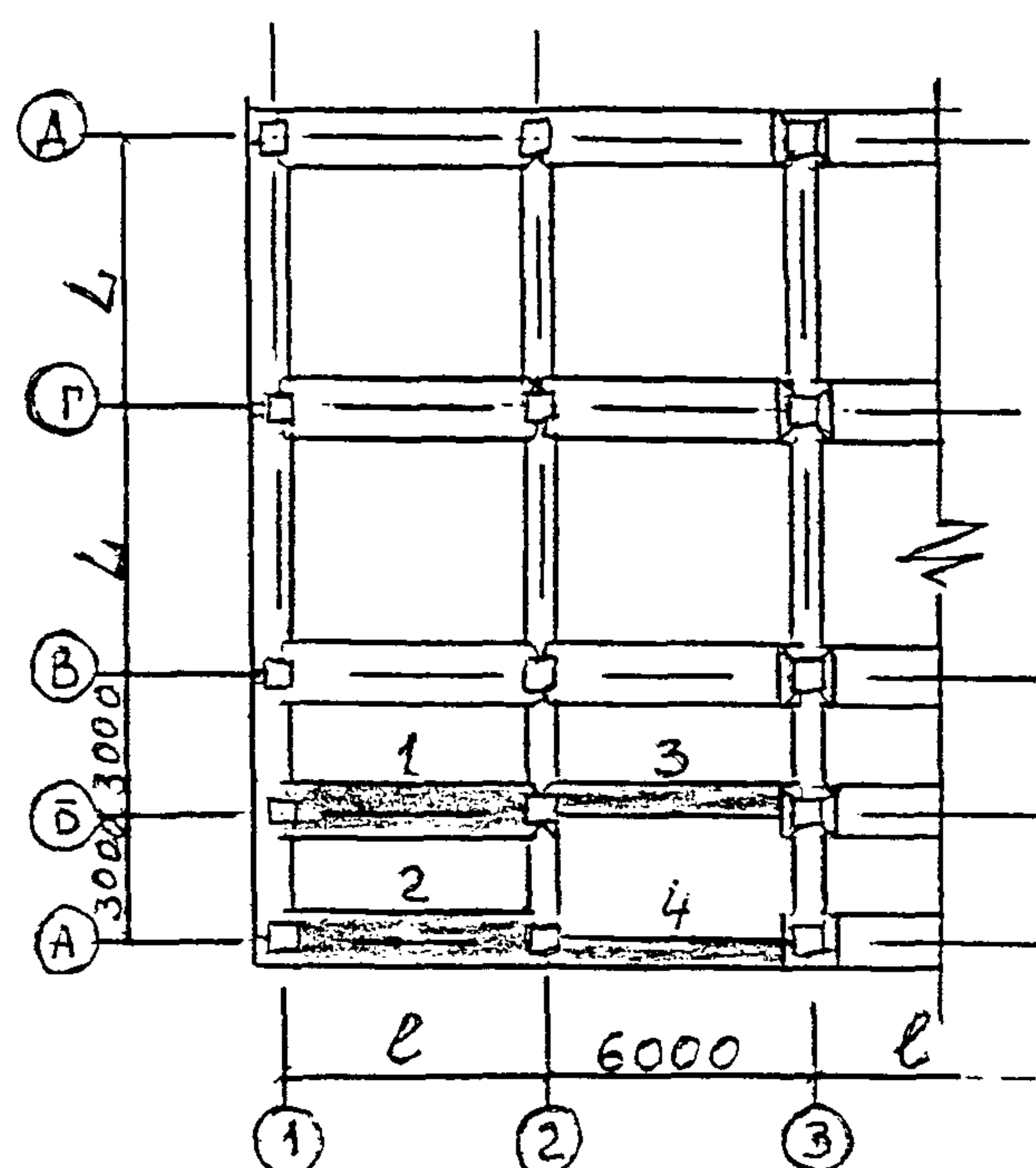
Схема 6. - 18 Снятие метал. распорок и укладка распорных плит.
