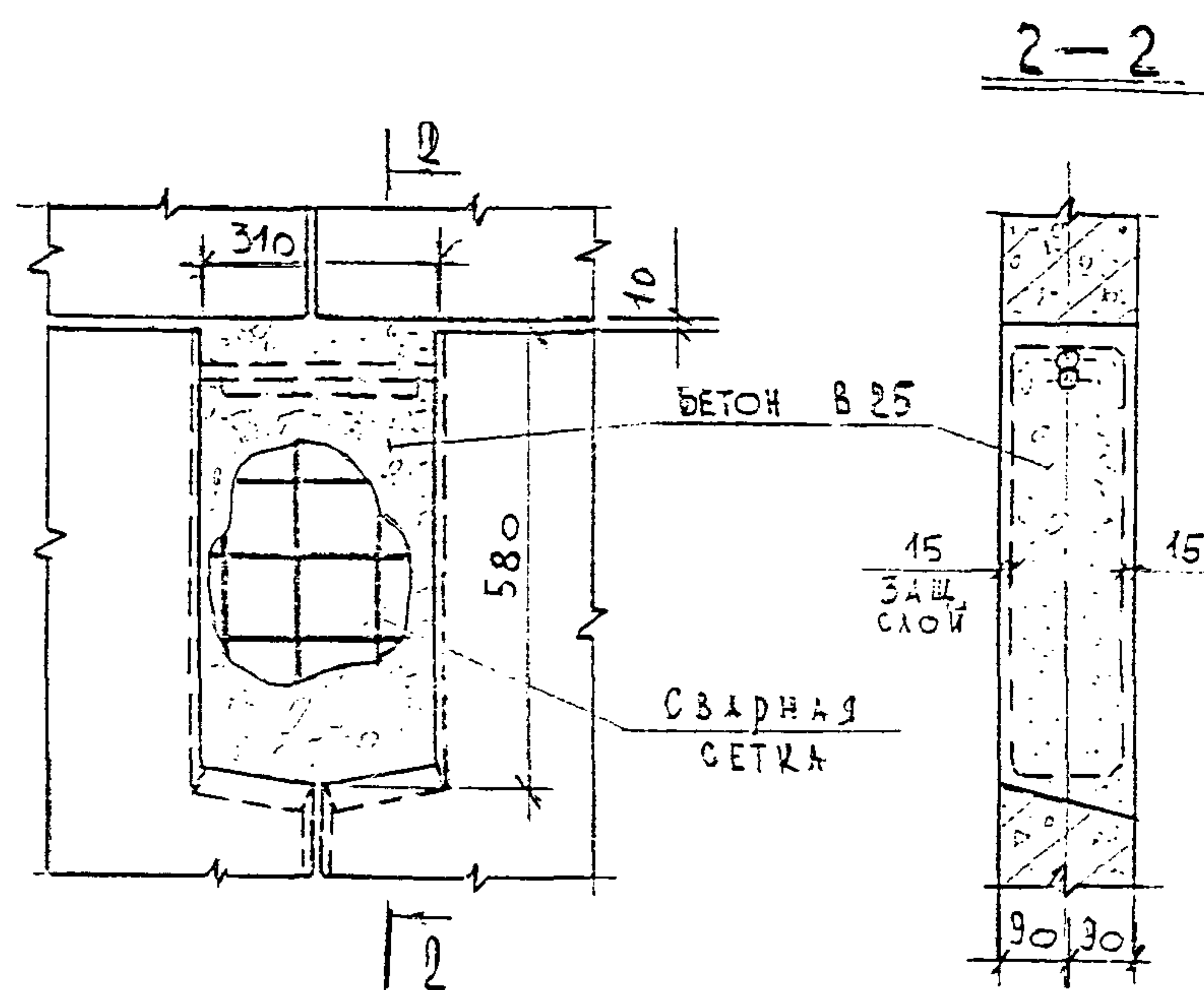
Деталь омоноличивания узла для консольных стен жесткости выполнять по сечению I - I
