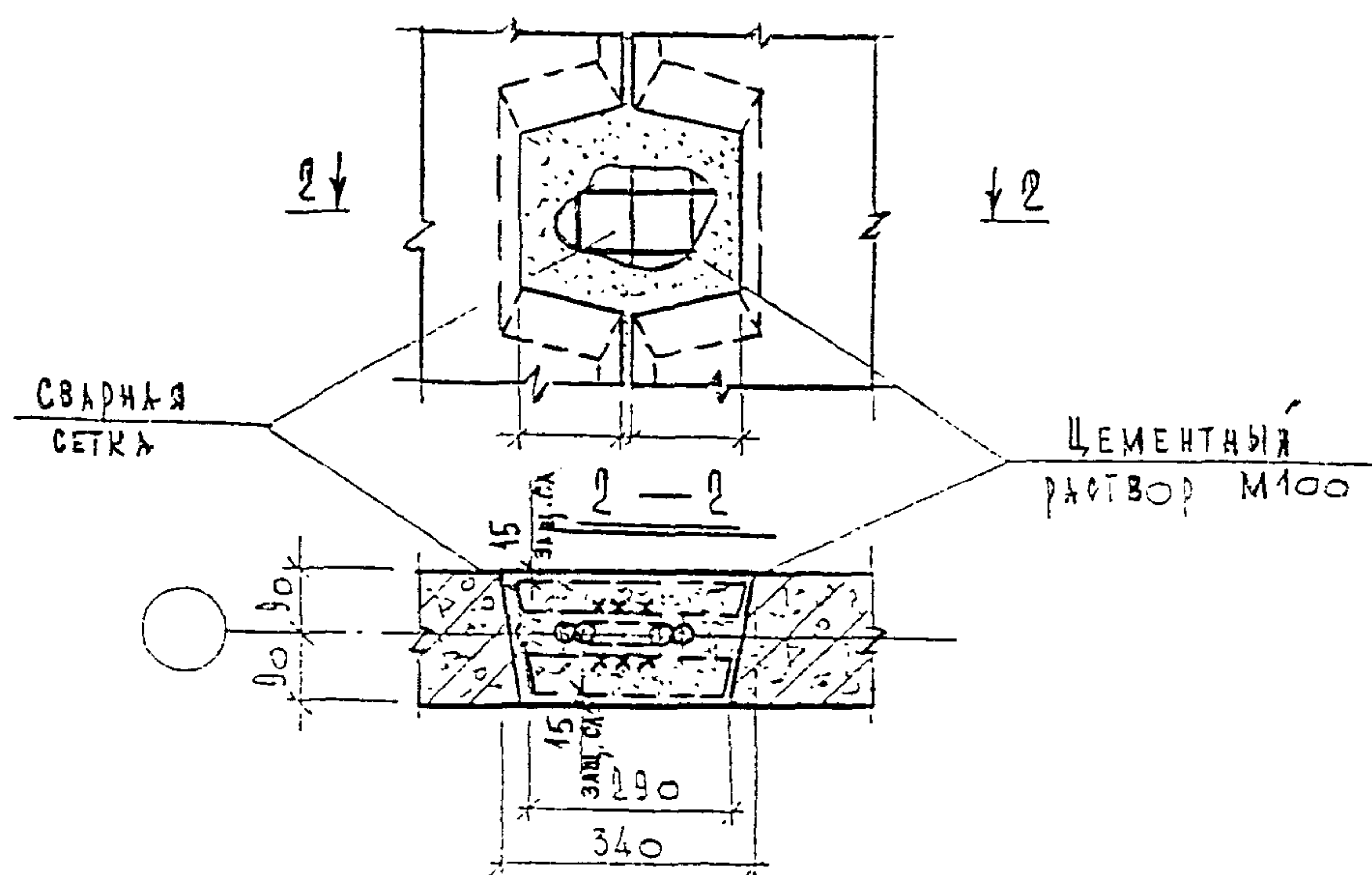
Деталь омоноличивания стыка
