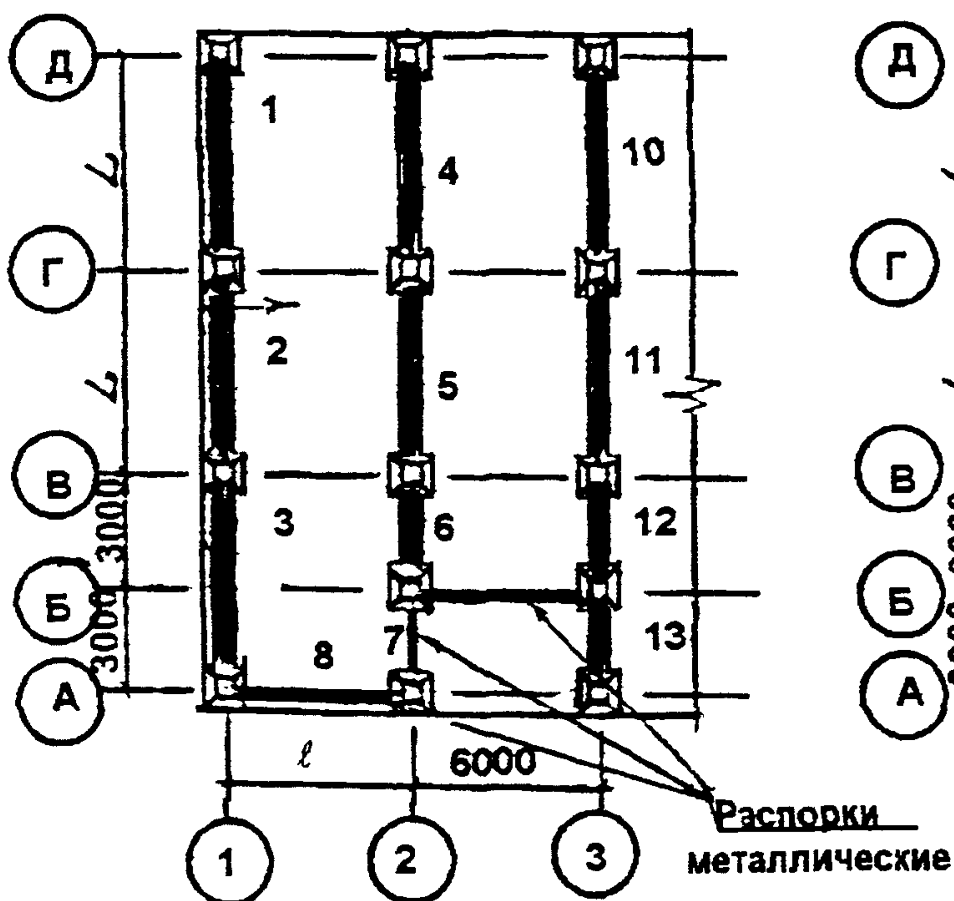
Схема 3 Укладка ригелей и установка временных метал.распорок
