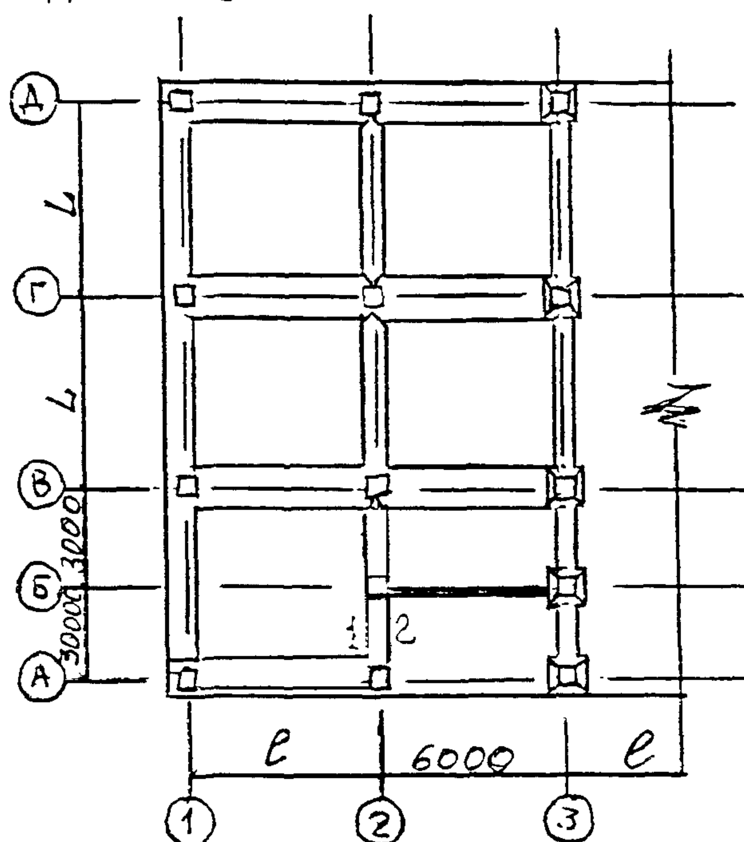
Схема 5. Укладка лестничного и рядового ригелей.
