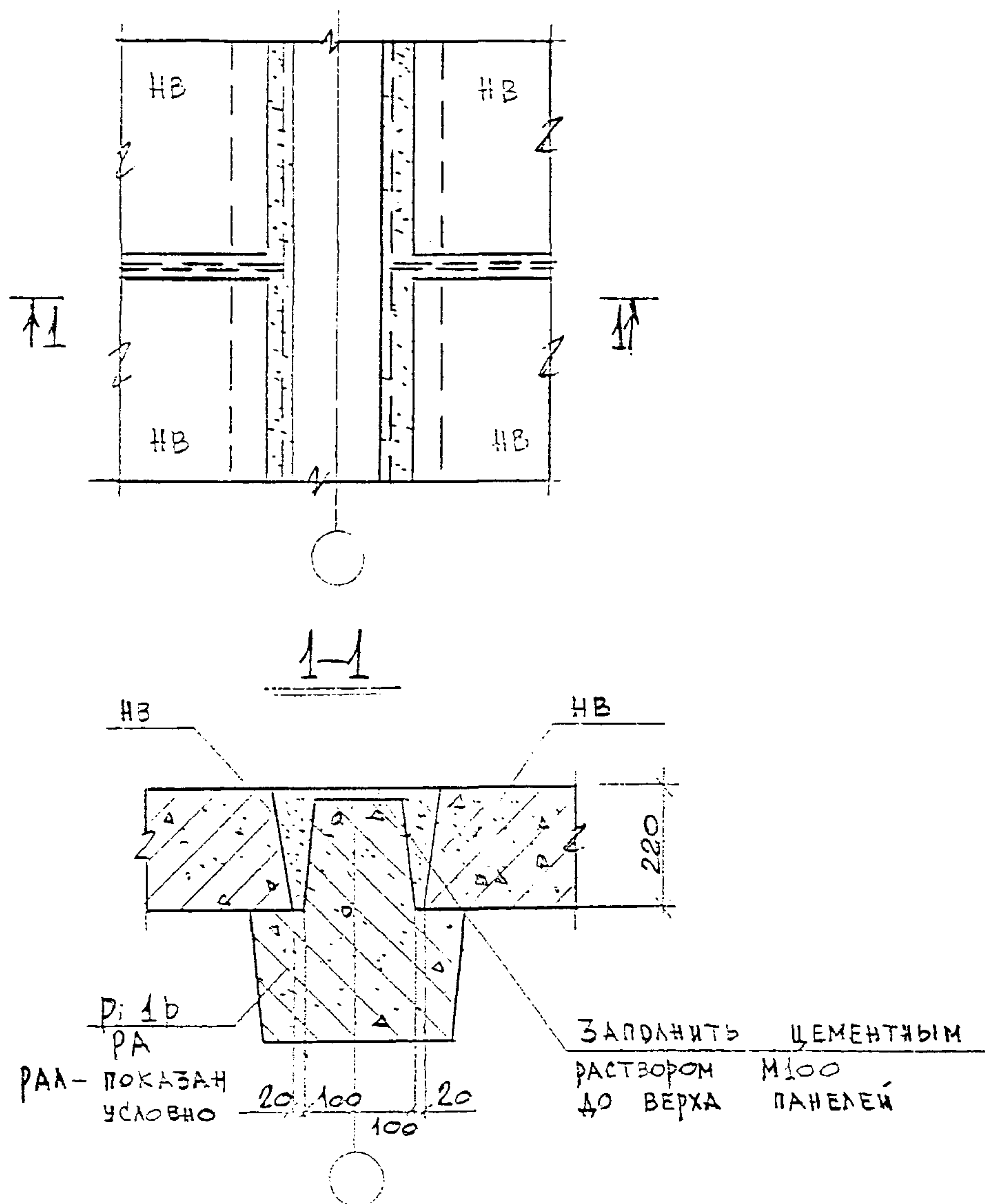
Рис.22 Опираение панелей перекрытия НВ на ригель
