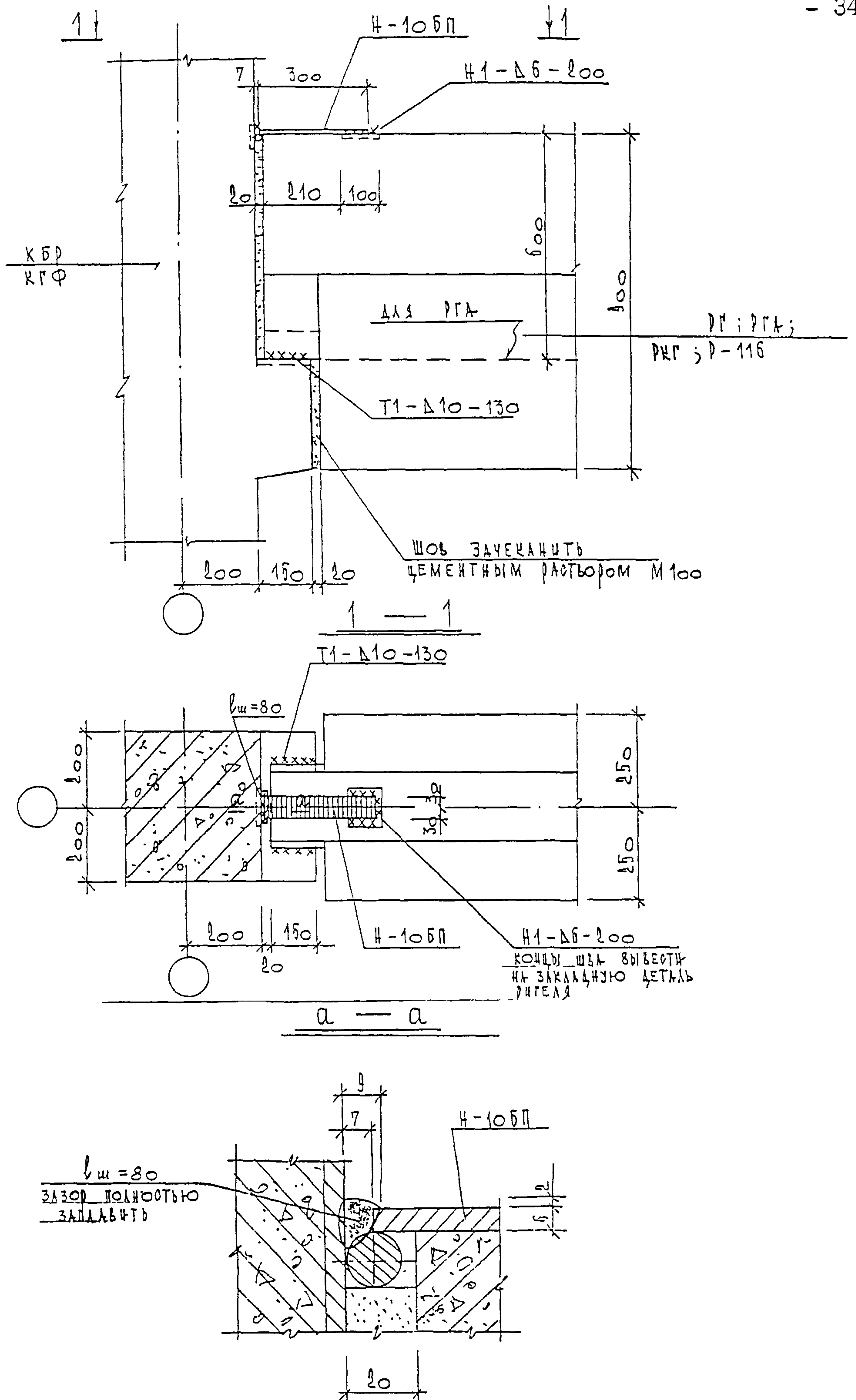
Рис. II Стык ригелей с колонной
