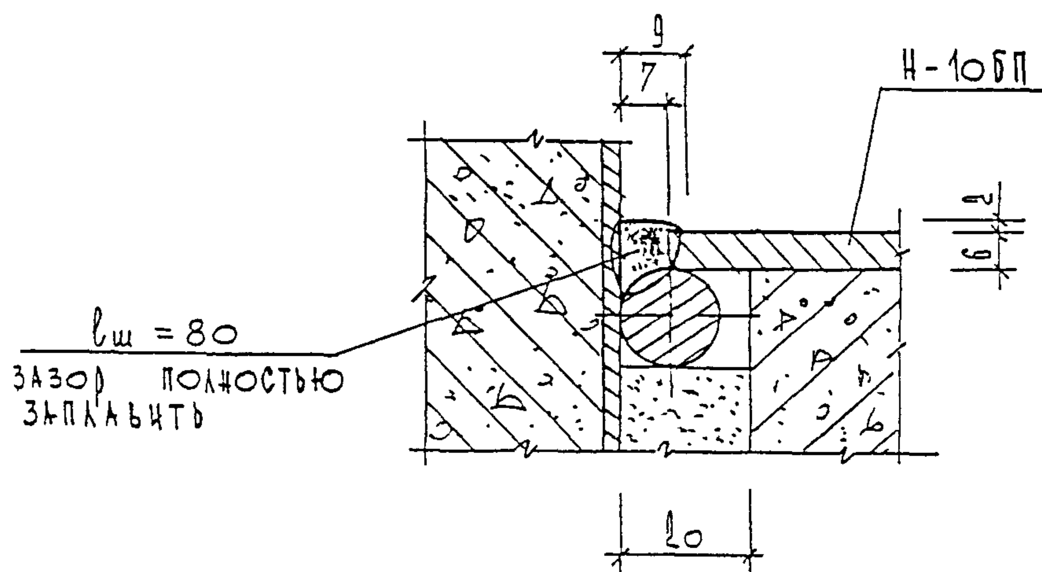
Рис. 12 Стык фасадного ригеля РГФ с колонной
