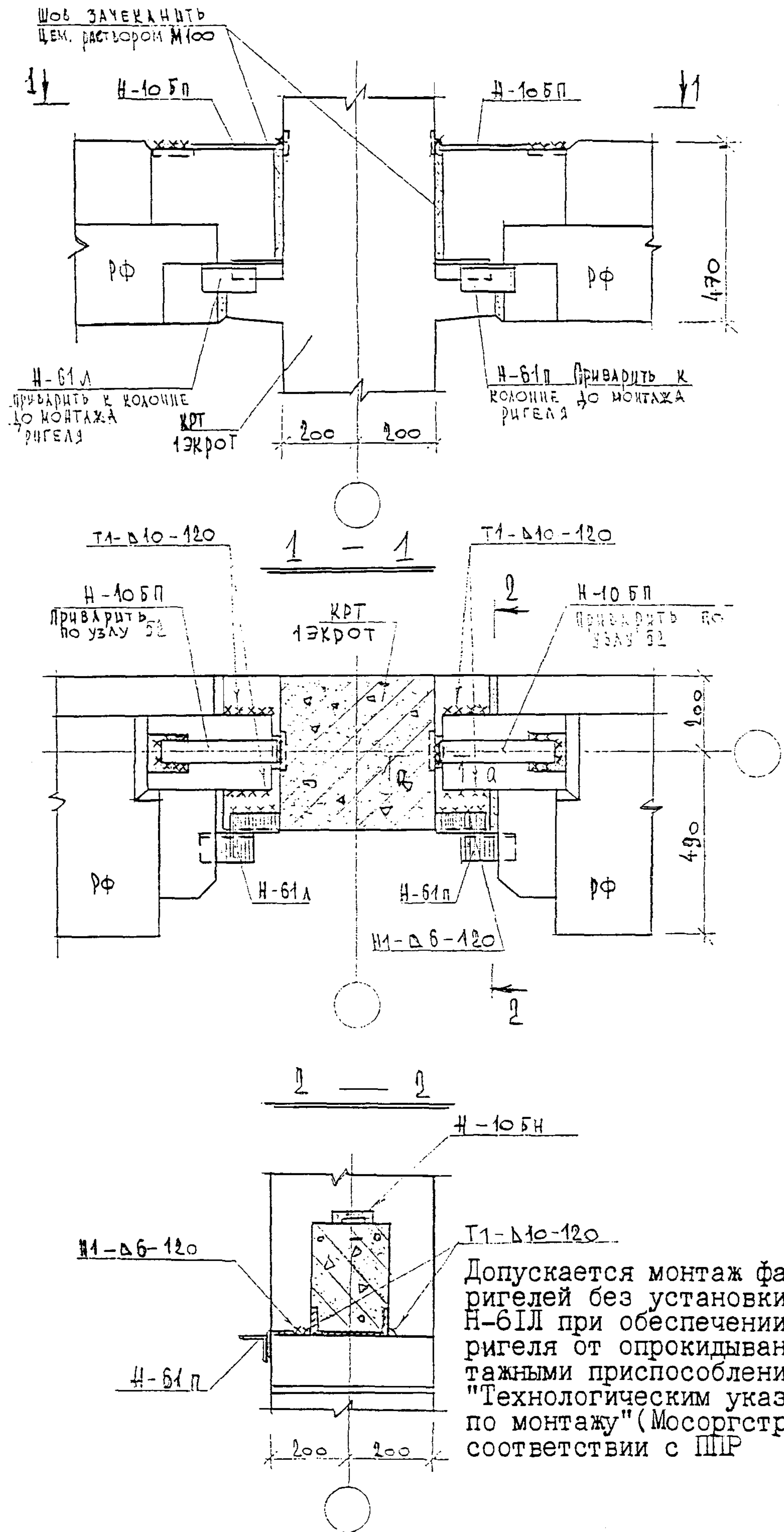
Рис. 21 Стык фасадного ригеля с колонной
