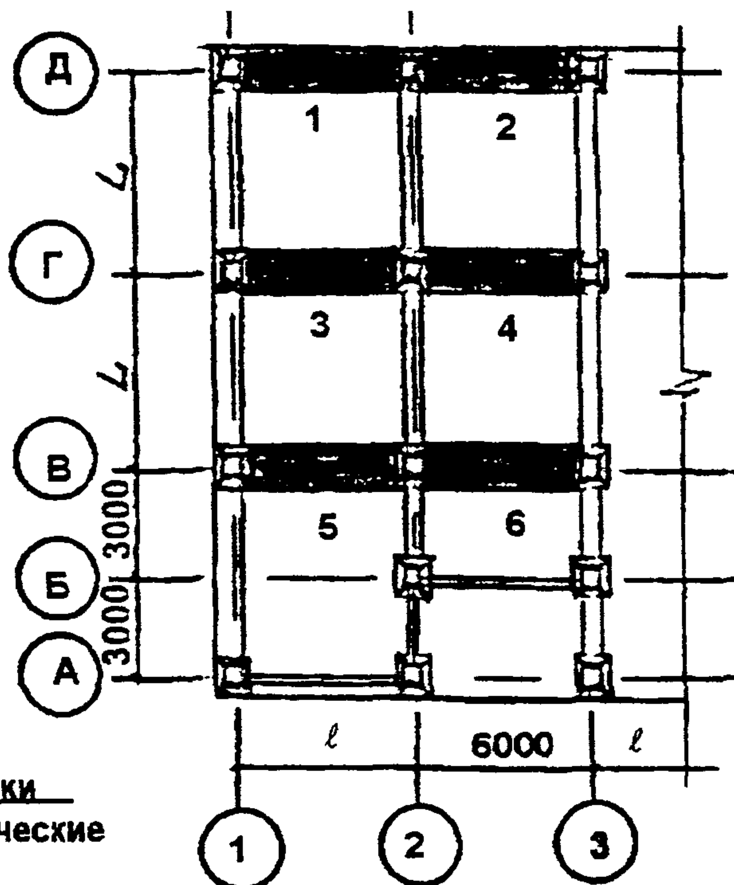
Схема 4 Укладка распорных плит
