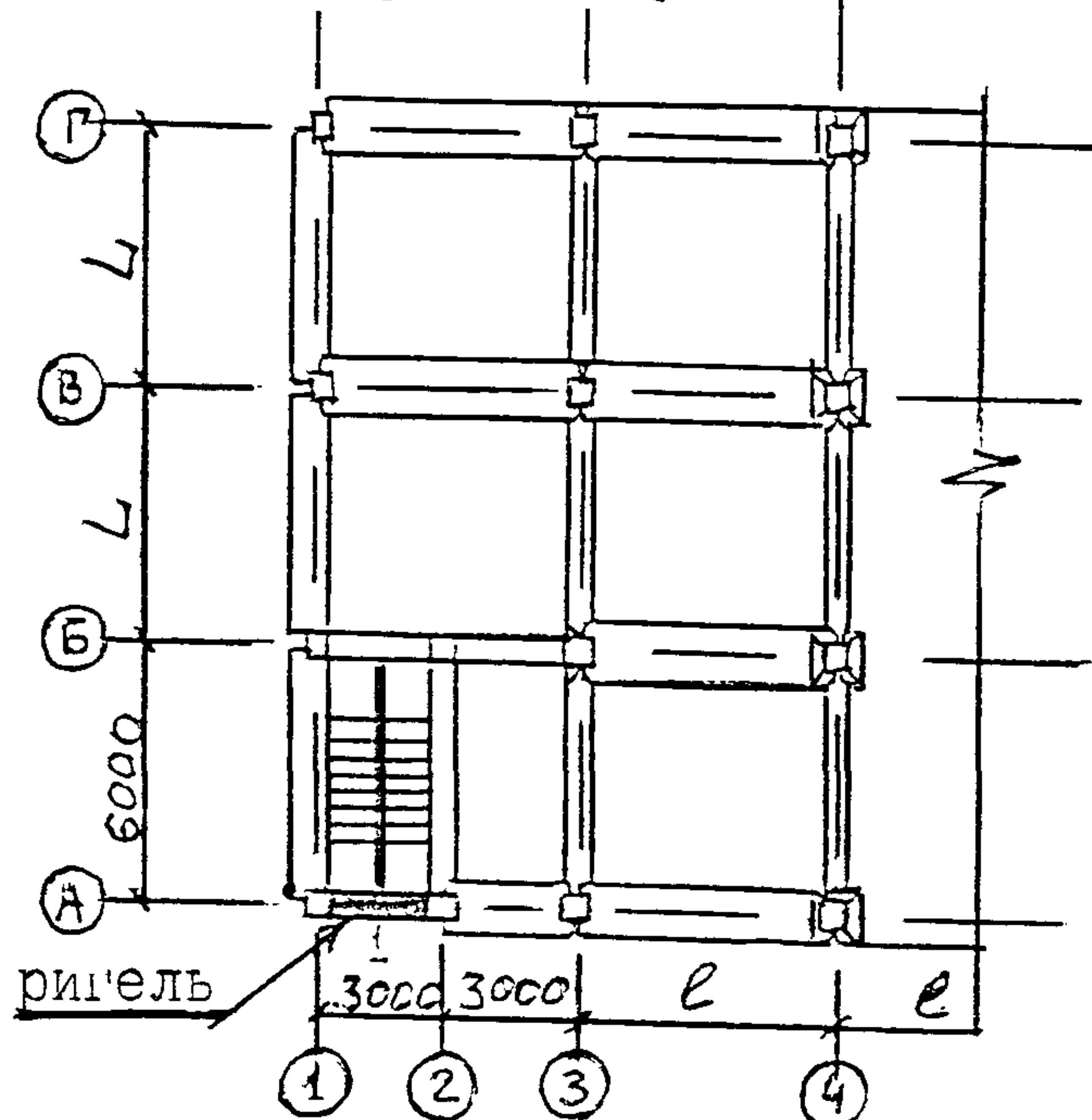
Схема 6. Снятие временной панели перекрытия и укладка ригеля.
