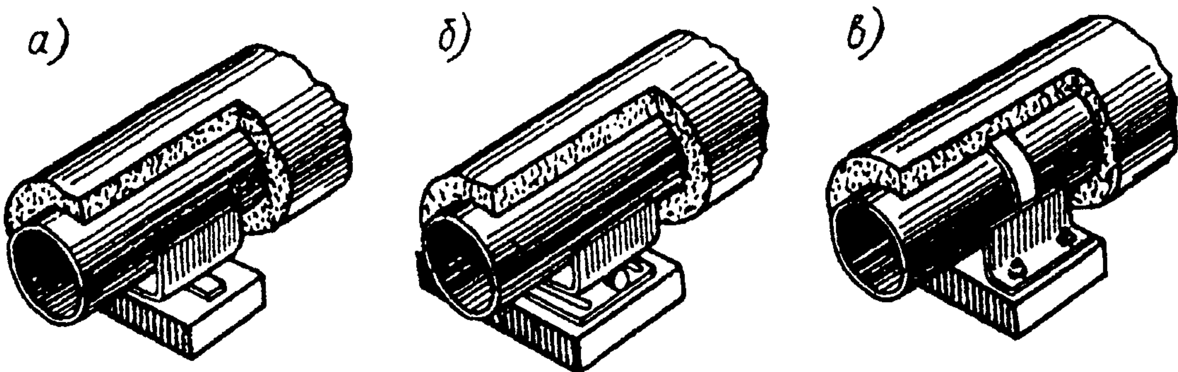
а — скользящая; б — катковая; в — неподвижная
