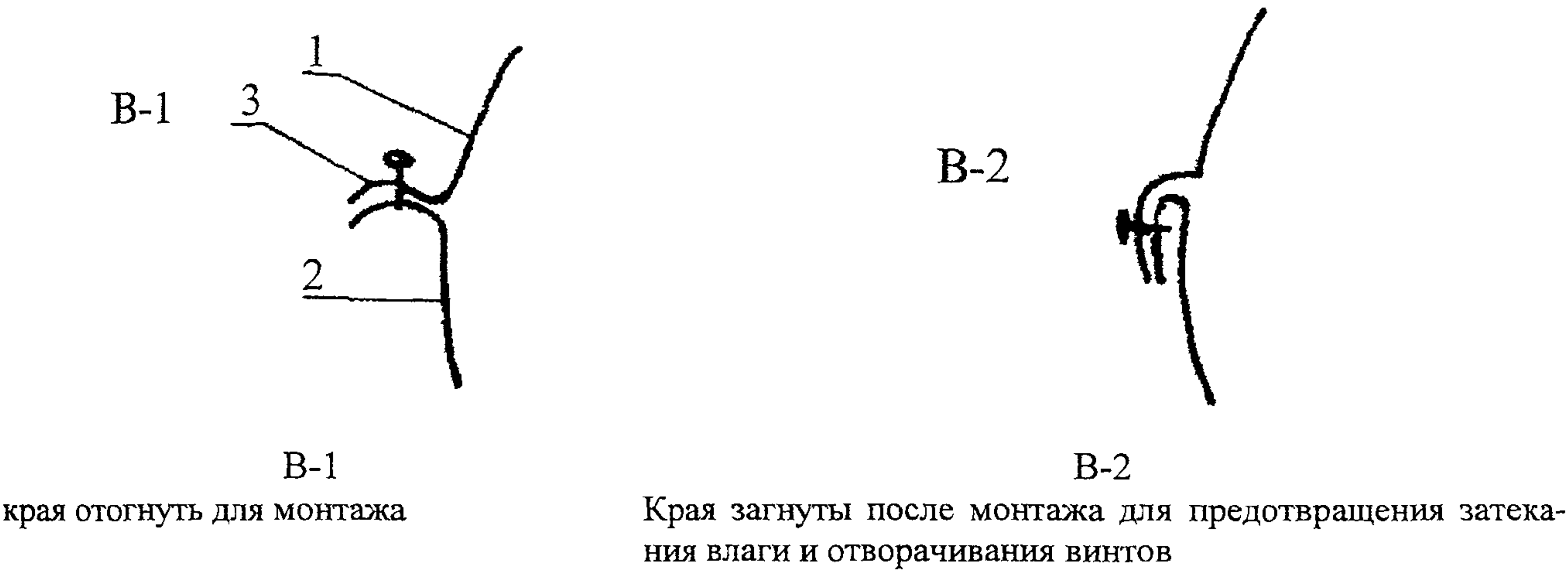
Рисунок 7 – Узел закрепления стяжек при установке скорлуп
