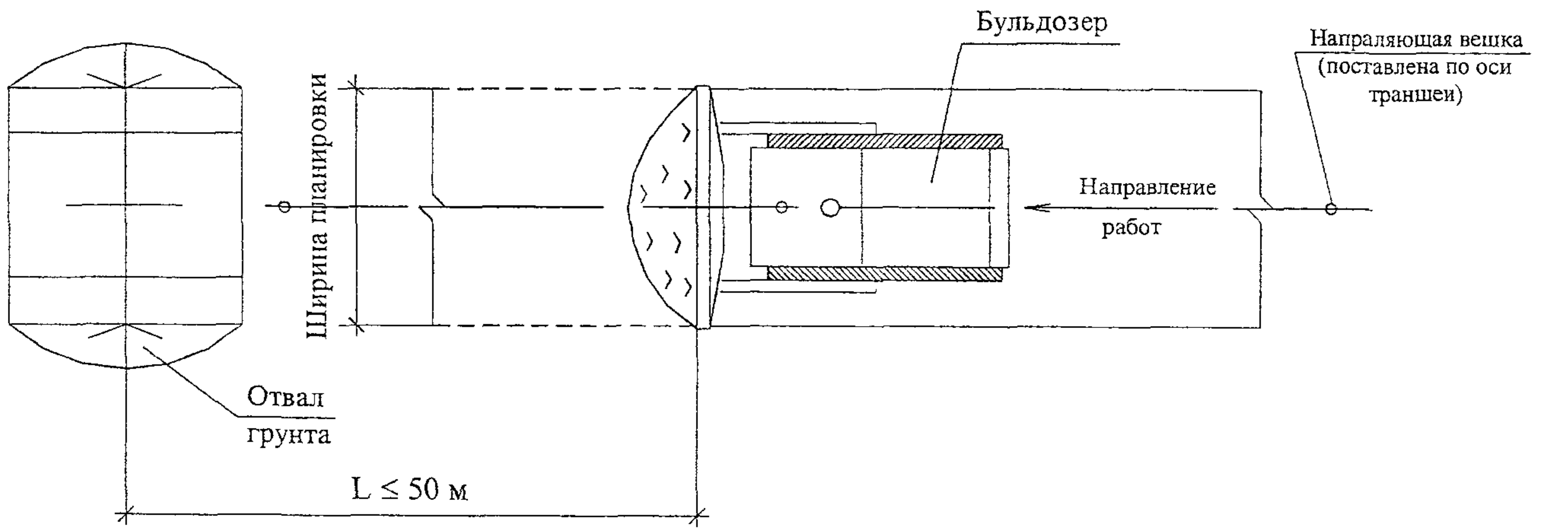
Рисунок 4 – Схема производства работ по планировке поверхности земли бульдозером
