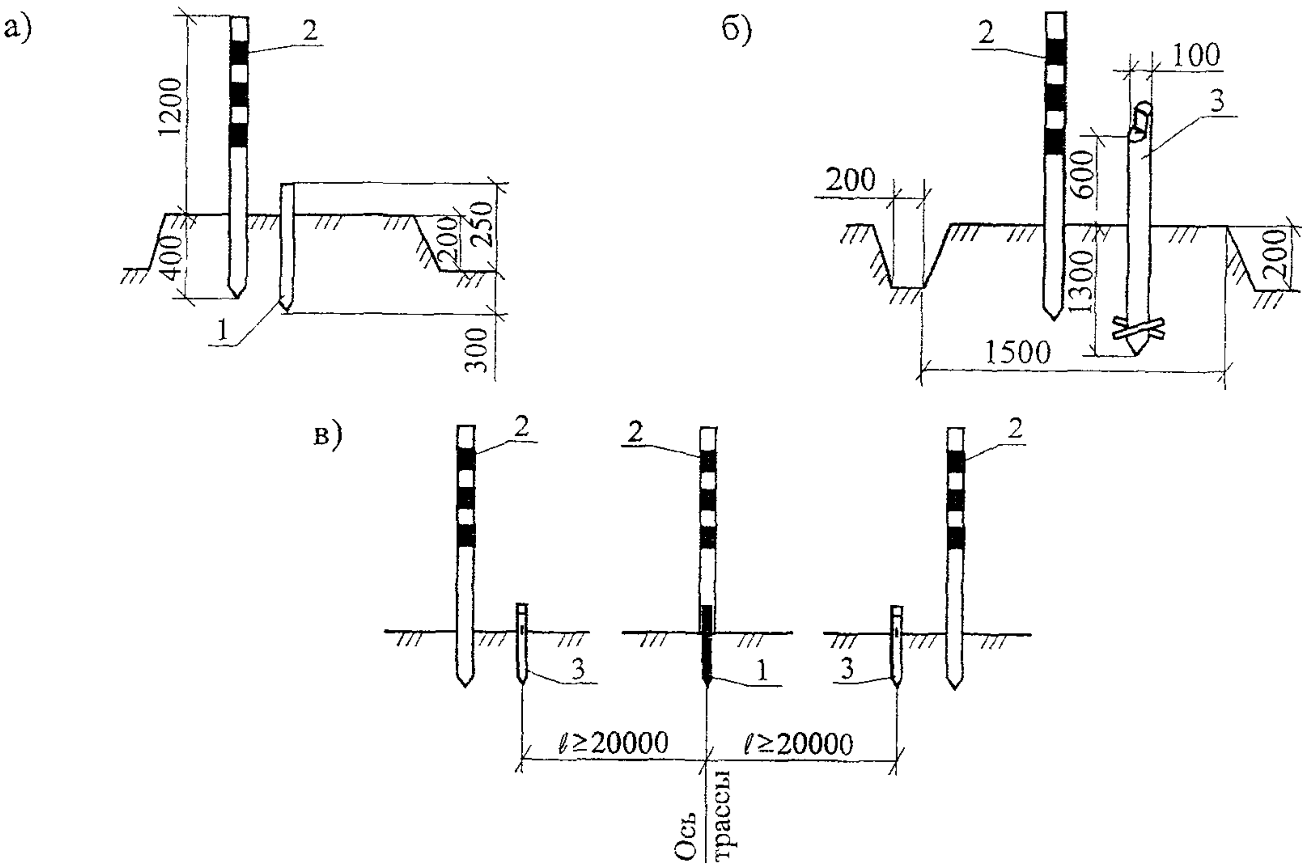
а, б – геодезические знаки; в – схема закрепления знаков разбивочных осей
