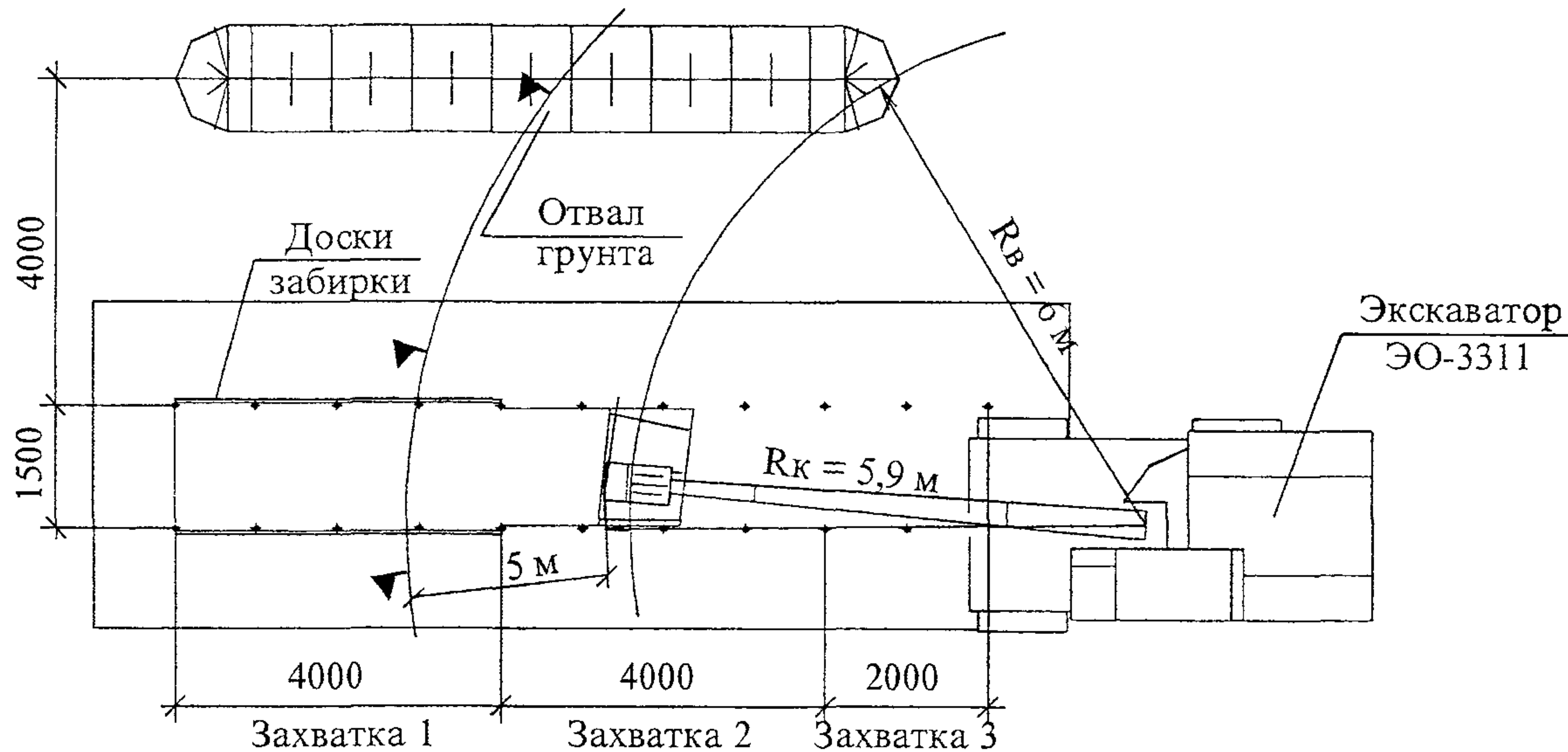
Рисунок 13 – Схемы производства работ по разработке грунта траншеи глубокого заложения с креплением стенок
