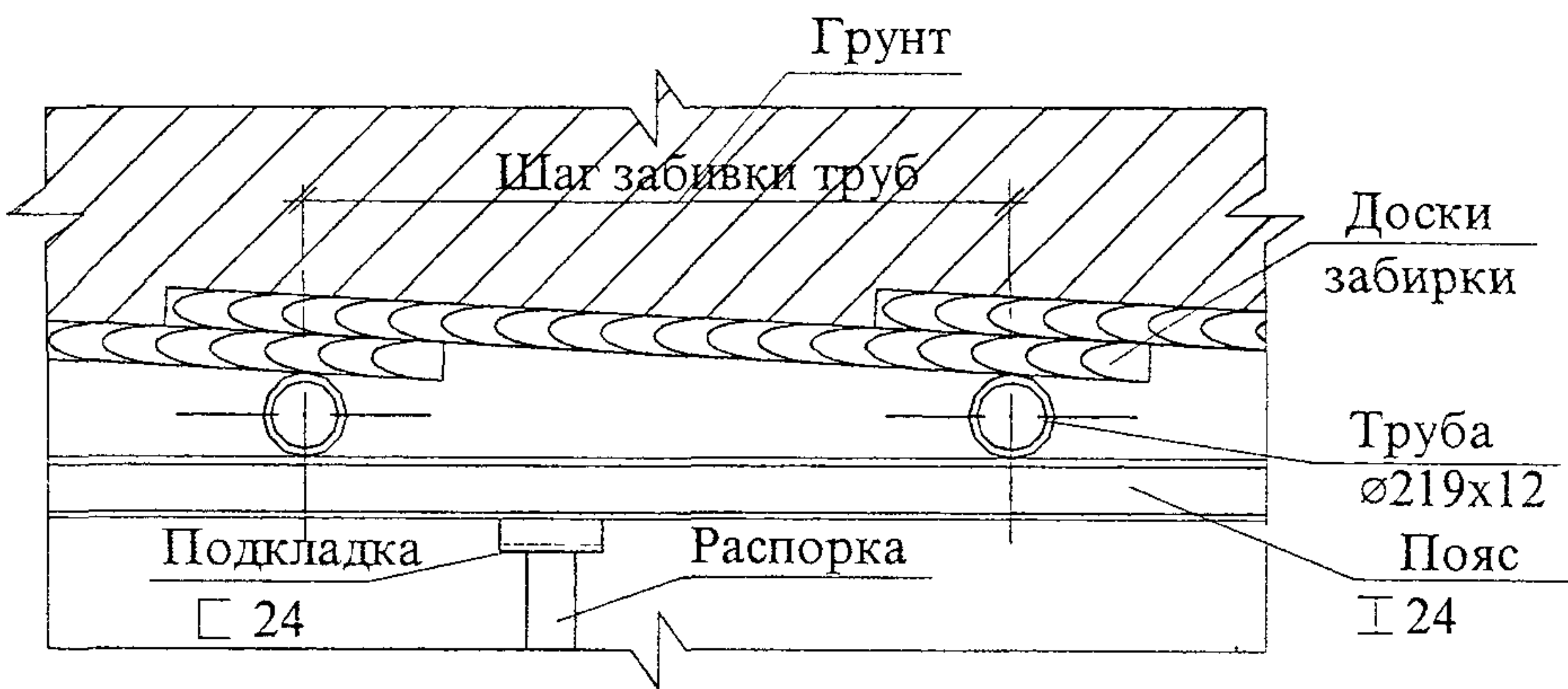
Рисунок 3 – Крепление стенок с применением стальных труб и распорок
