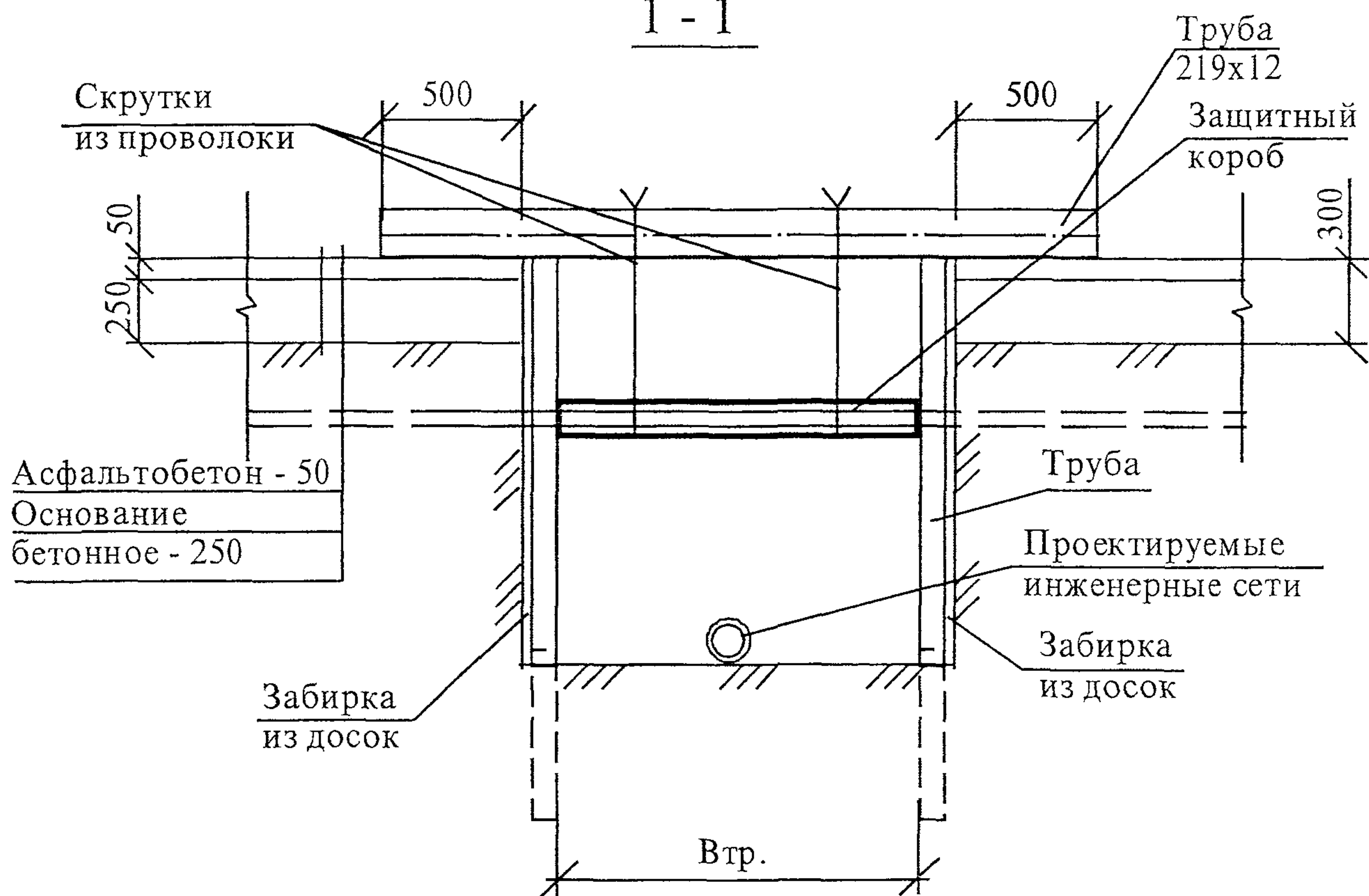
Рисунок 9 – Пример формирования траншеи при пересечении с действующими коммуникациями
