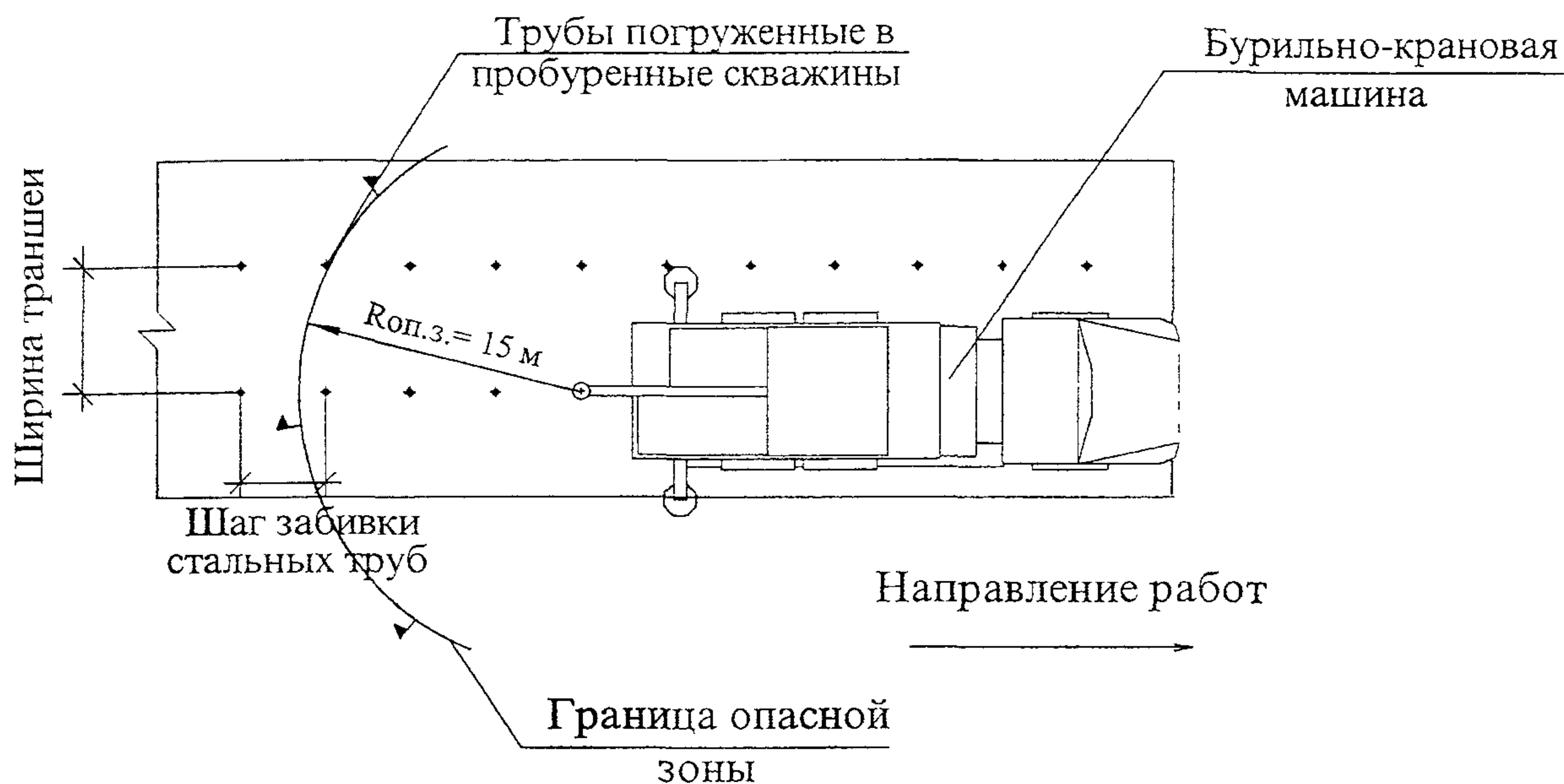
Рисунок 6 – Схема производства работ по бурению скважин и установке в них стальных труб
