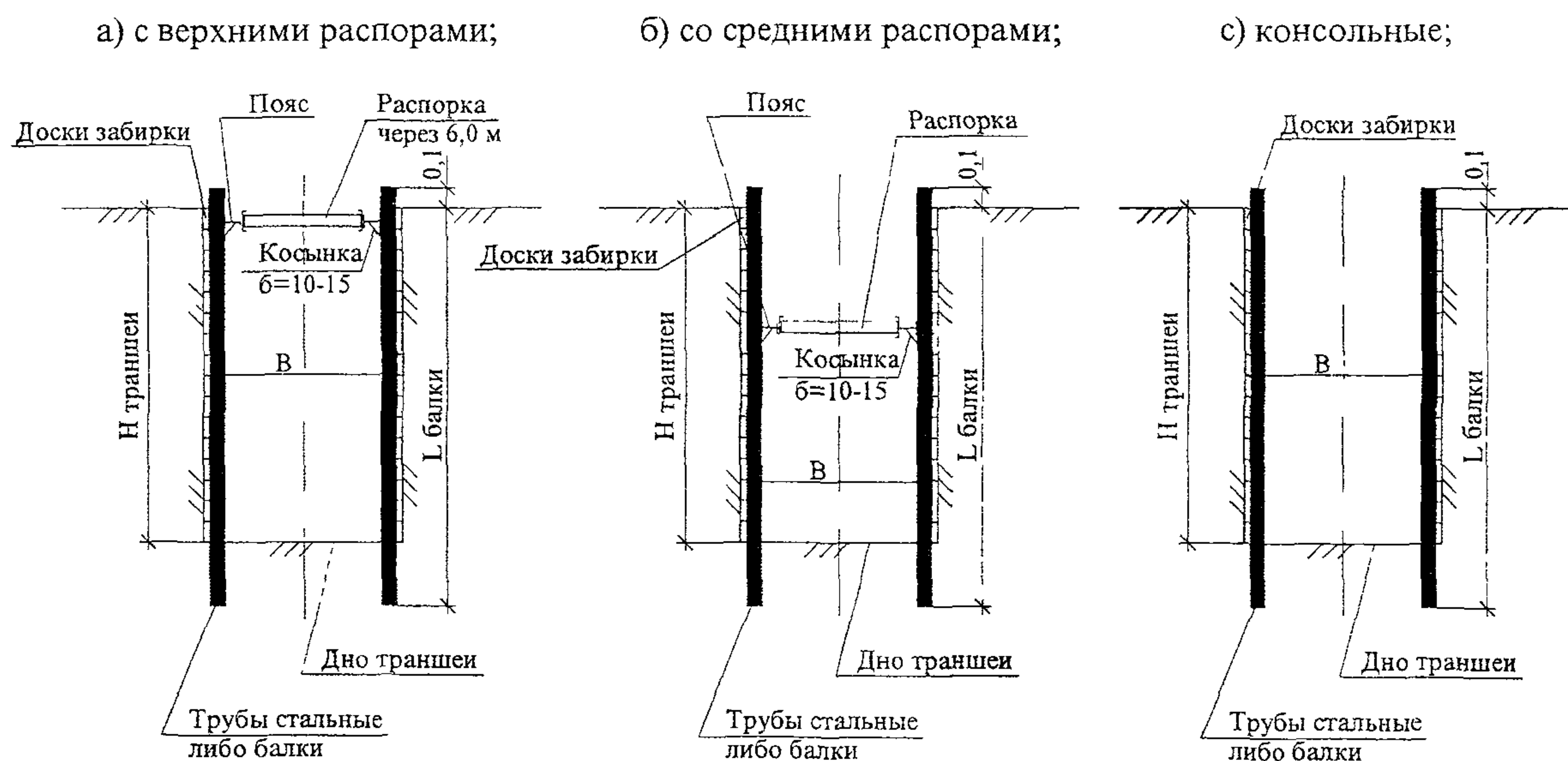
Рисунок 1 – Варианты крепления стенок траншей глубокого заложения
