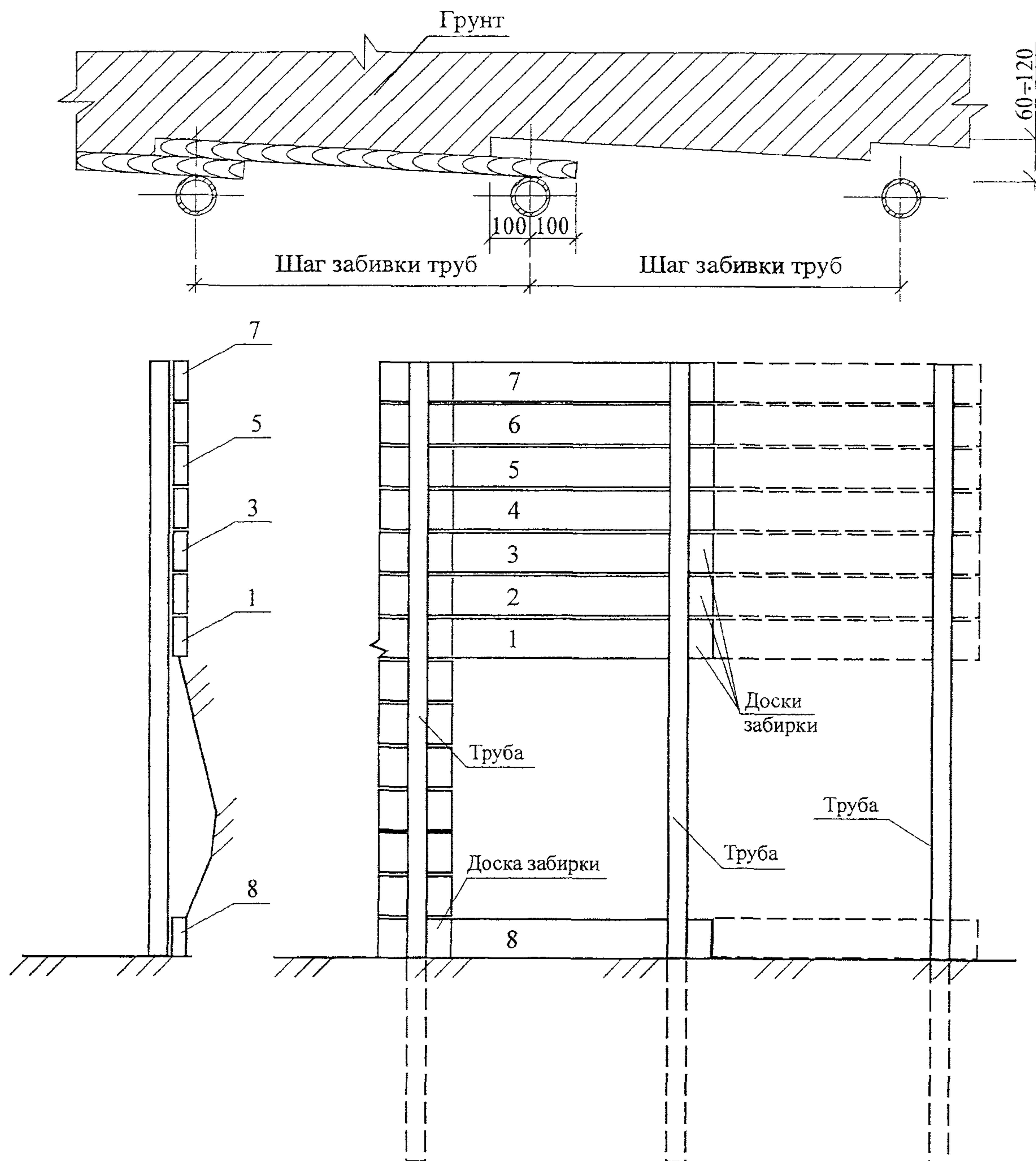
Рисунок 11 – Последовательность и схема устройства заборки
