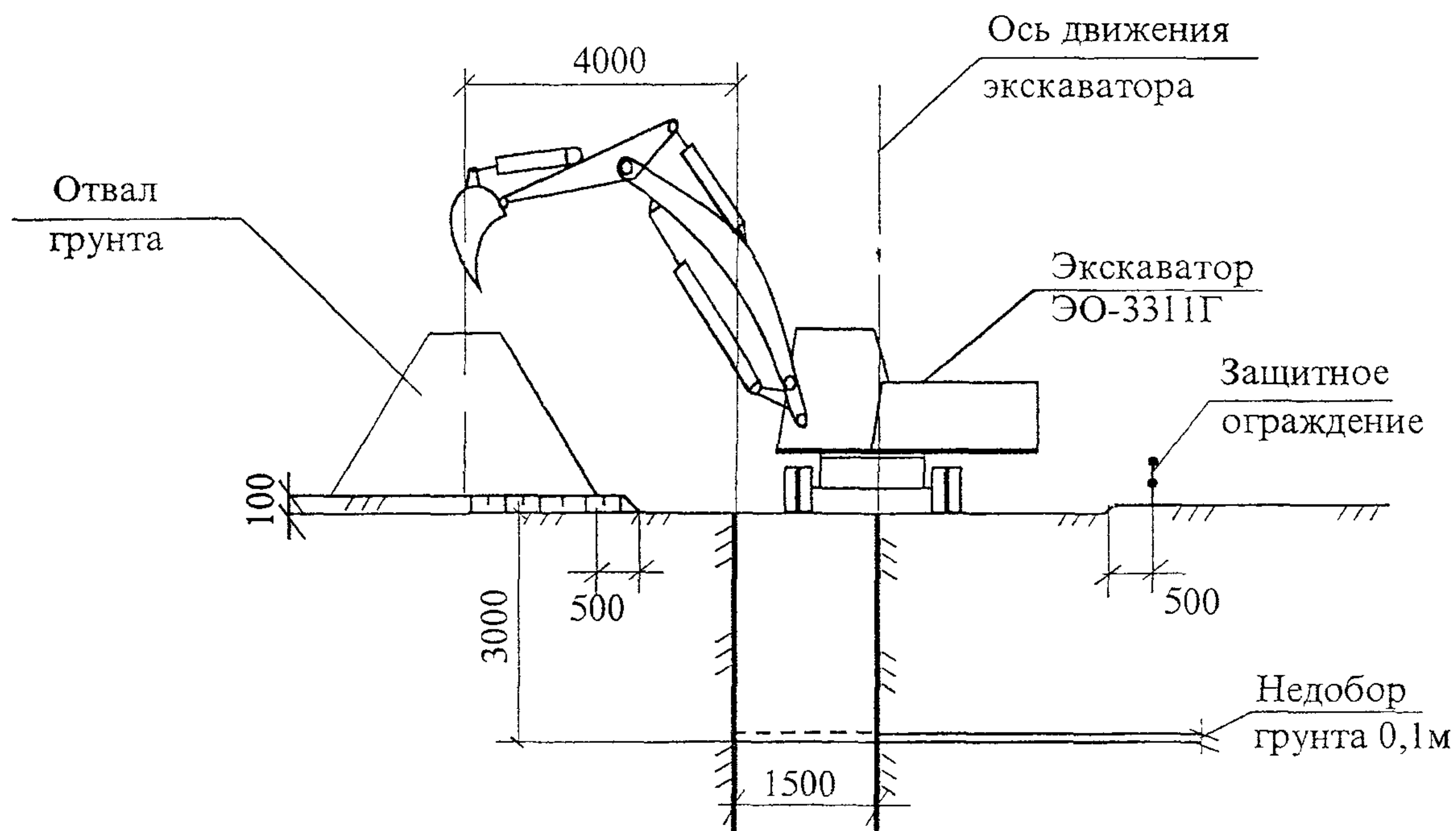
Рисунок 12 – Пример геометрии траншеи для цифровых расчетов
