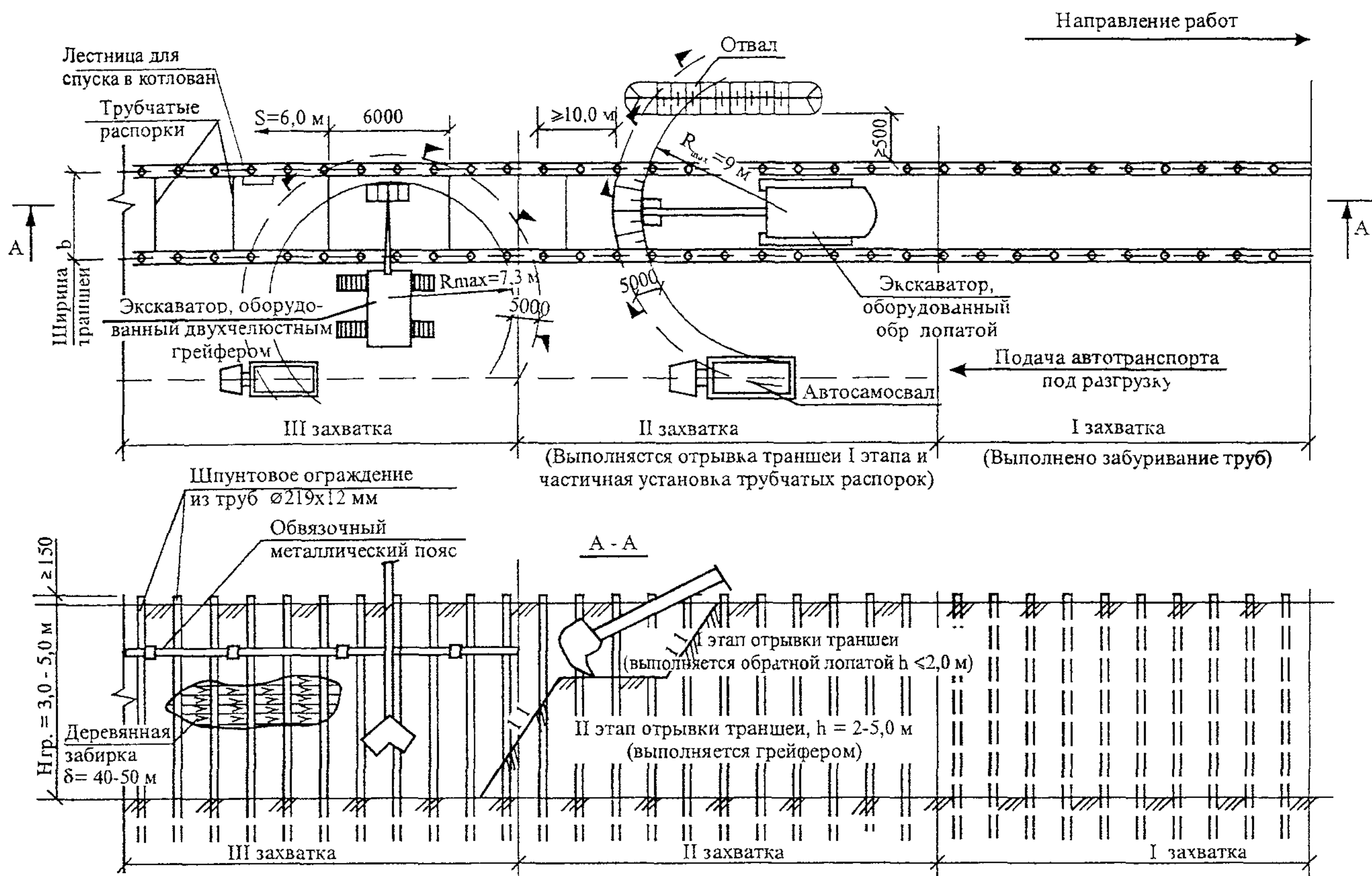
Рисунок 8 – Схема поэтапного производства работ при отрывке траншей экскаватором, оборудованным обратной лопатой и грейфером в траншеях с креплением распорками
