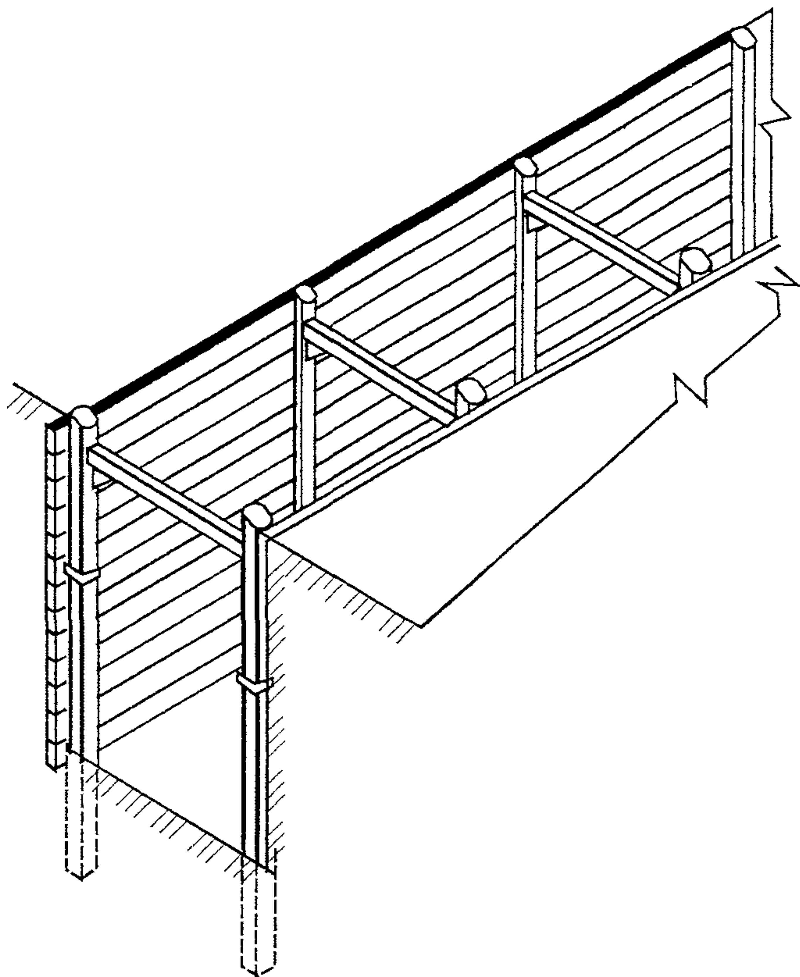
Рисунок 2 – Общая схема траншеи с верхним креплением
