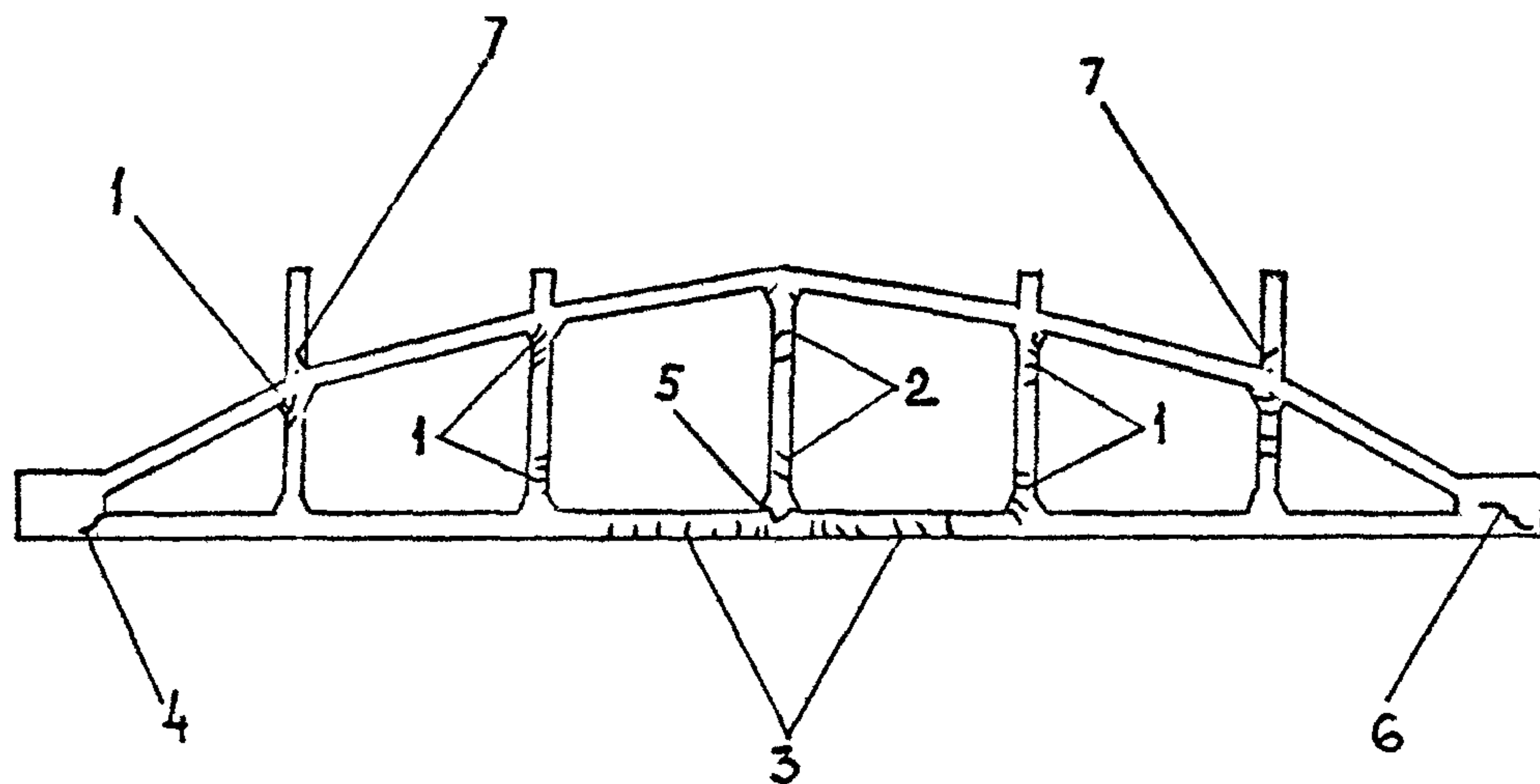
Рис.3.10. Характерные дефекты и повреждения железобетонных стропильных безраскосных ферм
