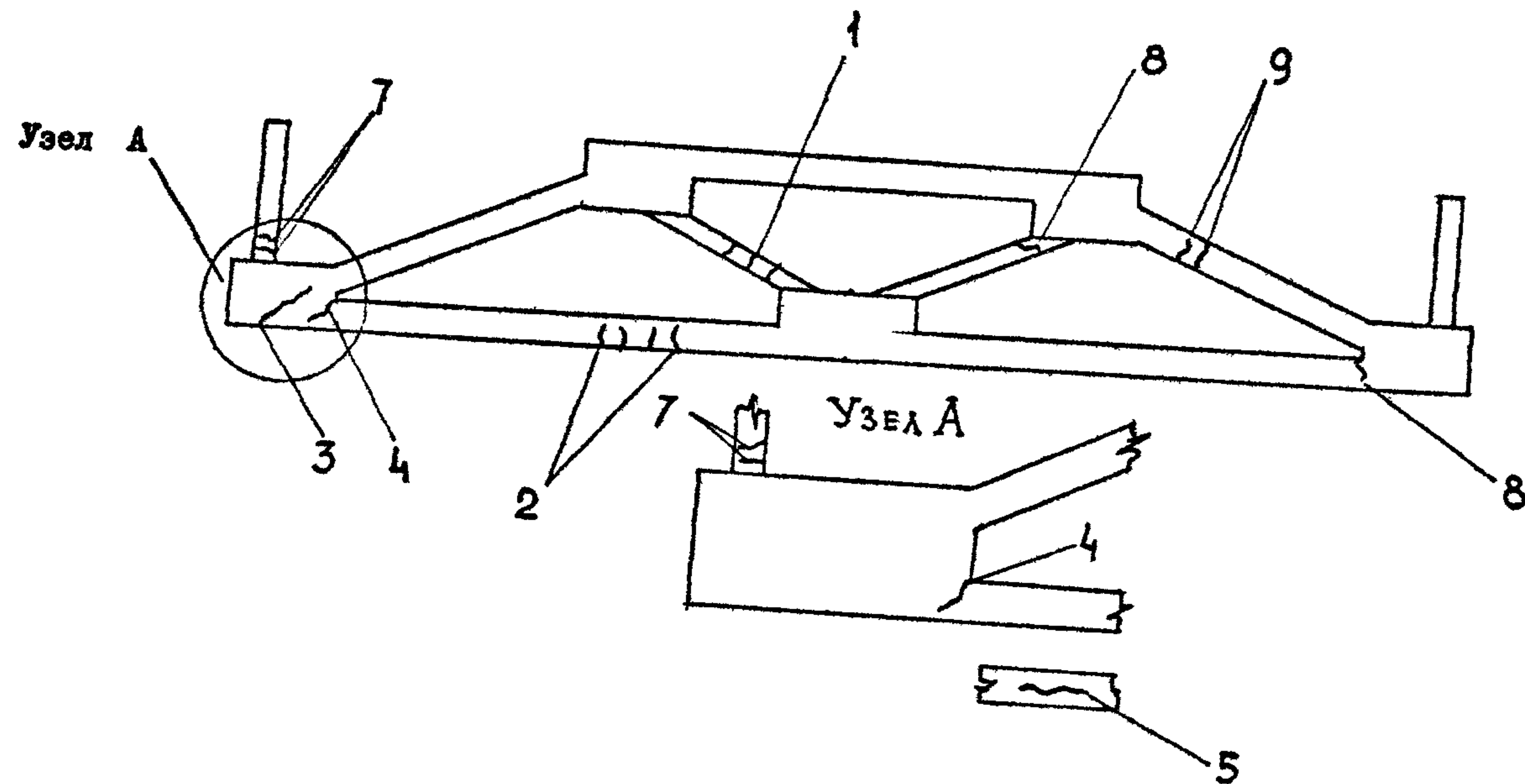
Рис. 3. II. Характерные дефекты и повреждения железобетонных подстропильных ферм с параллельными поясами
