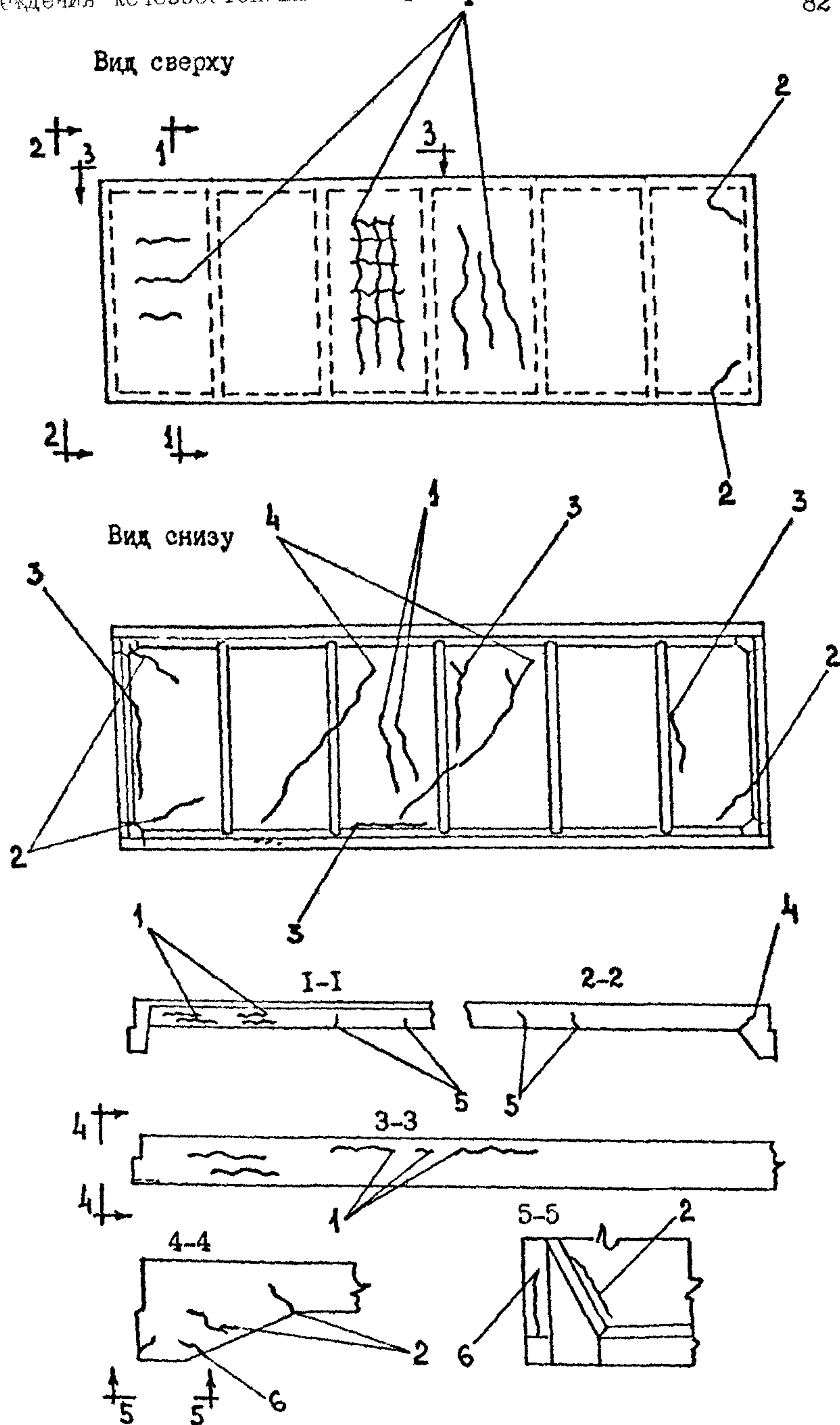
Характерные дефекты железобетонных ребристых плит Рис. 3.16. покрытий, появляющиеся на стадиях изготовления, транспор- тировки и монтажа
