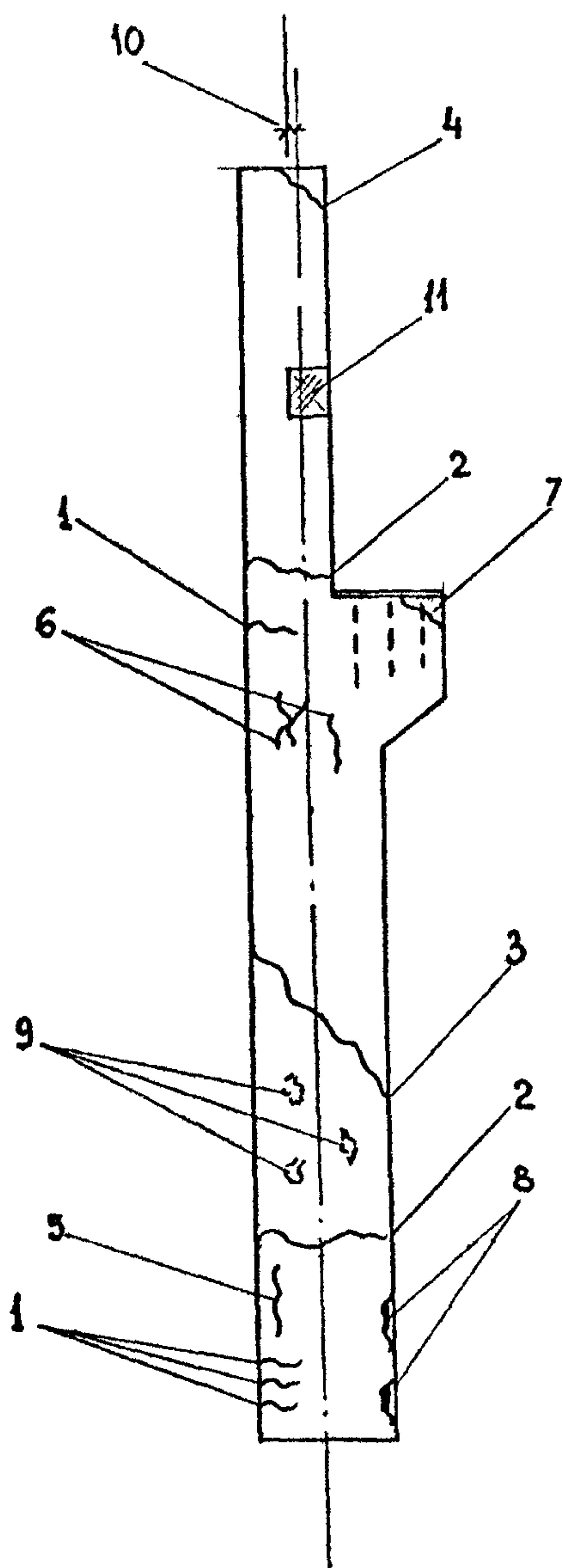
Рис. 3.1. Характерные дефекты и повреждения одноветвевых колонн
