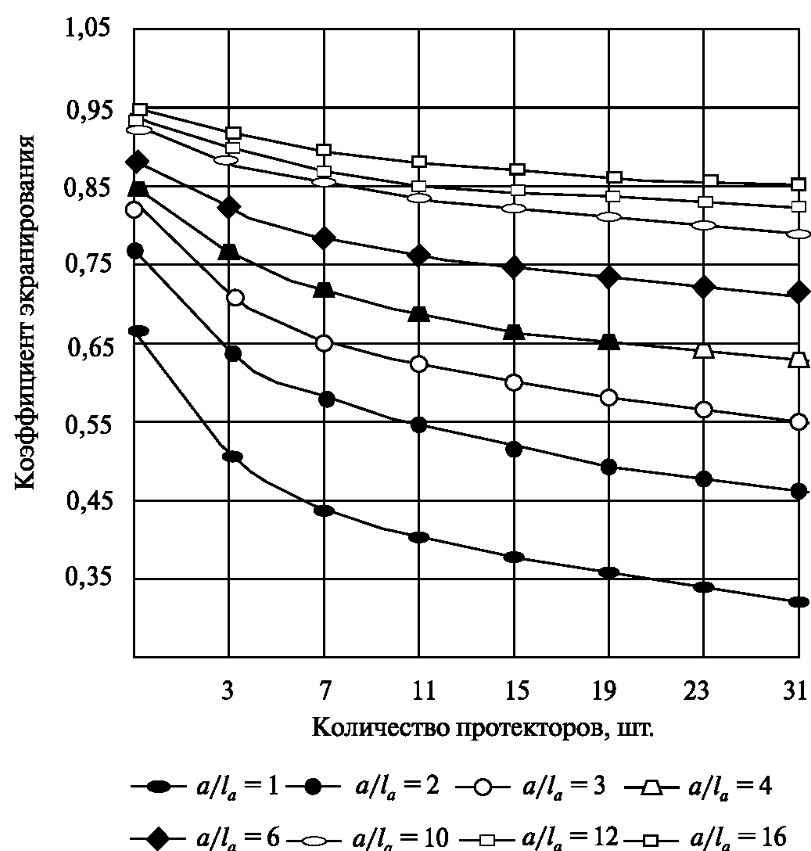
Рисунок 9.1 – Коэффициент экранирования протекторов в групповой протекторной установке в зависимости от отношения расстояния между ними и их длиной [a/l_a] (глубина установки протекторов в грунт 1,6 м)
