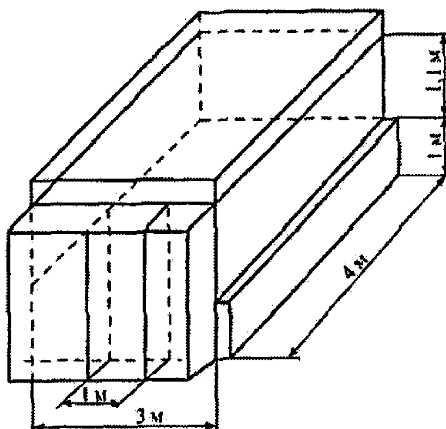
Рисунок 16 — Общий вид кабины наблюдения
