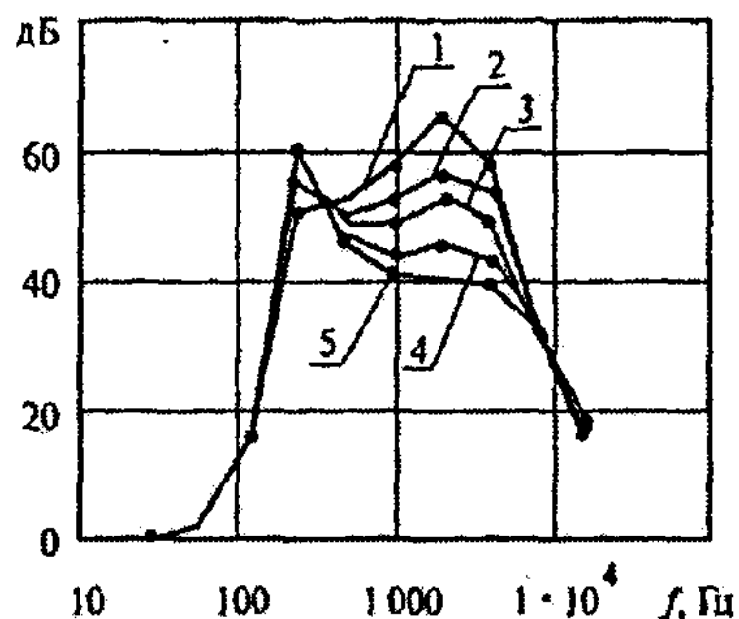
Базовая конструкция: ЗПМ — БСТВ-20; сопротивления продуванию: 1 - 180 Па·с/м; 2 - 250 Па·с/м; 3 - 300 Па·с/м; 4 - 400 Па·с/м; 5 - 500 Па·с/м Рисунок 19 — Влияние сопротивления продуванию защитной ткани на частотную характеристику глушителя
