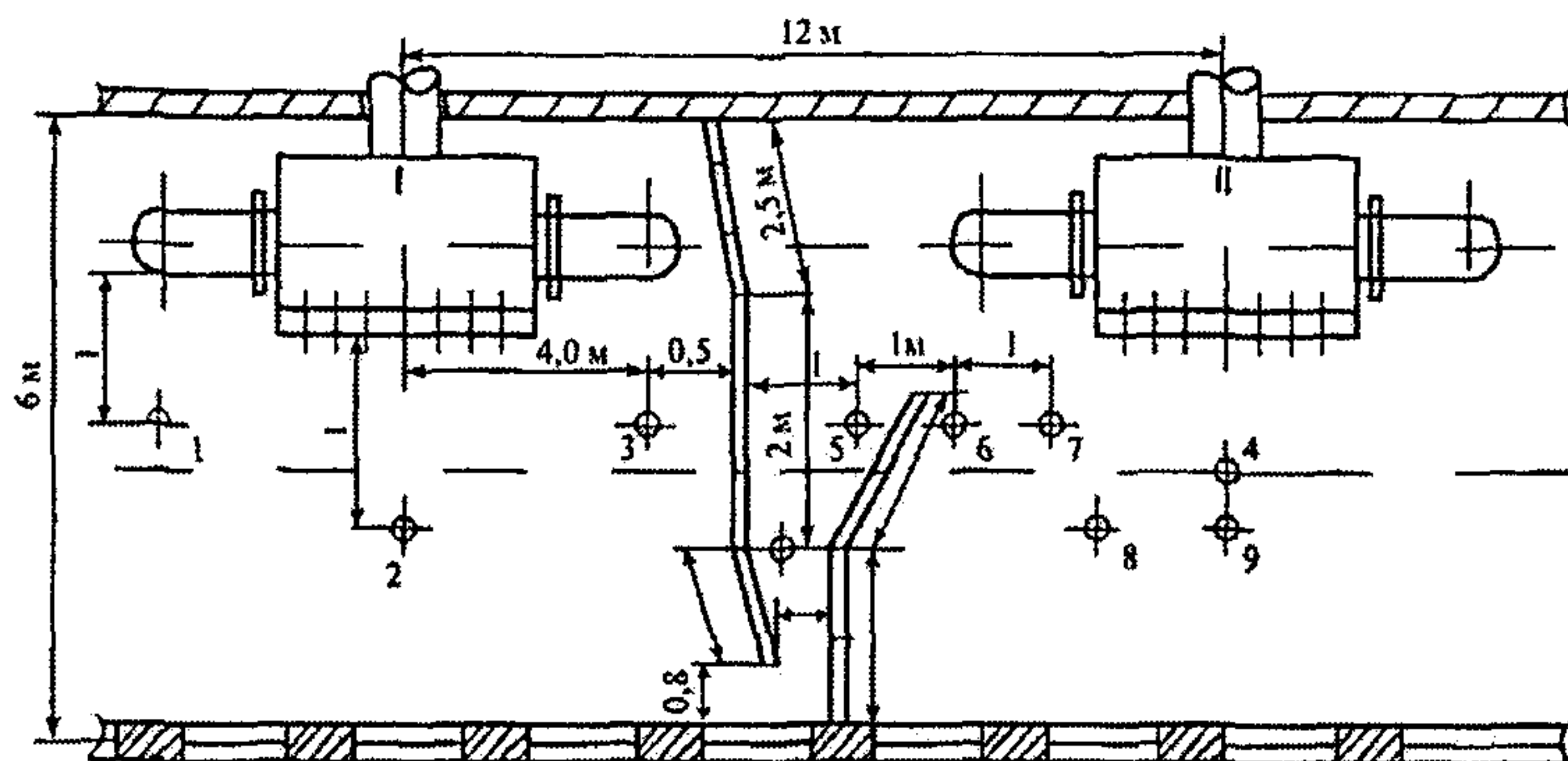
I - работающий агрегат; II - ремонтируемый агрегат; 1-9 - точки измерения Рисунок 11 — Схема размещения акустического экрана и точек измерения в галерее магнетателей
