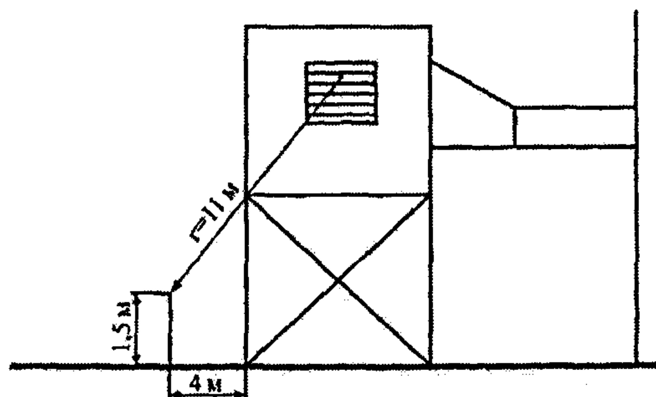
Рисунок 6 — Схема для акустического расчета глушителей шума всасывания
