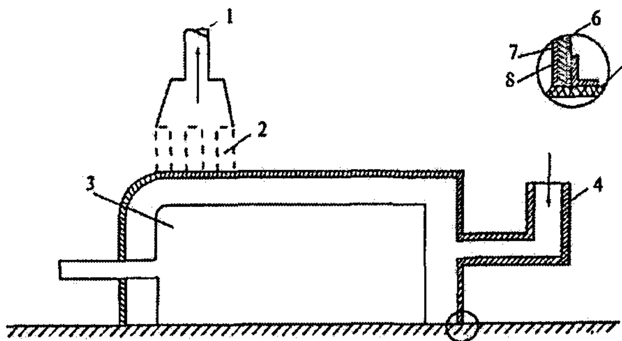
Рисунок 10 — Схема звукоизолирующего кожуха
