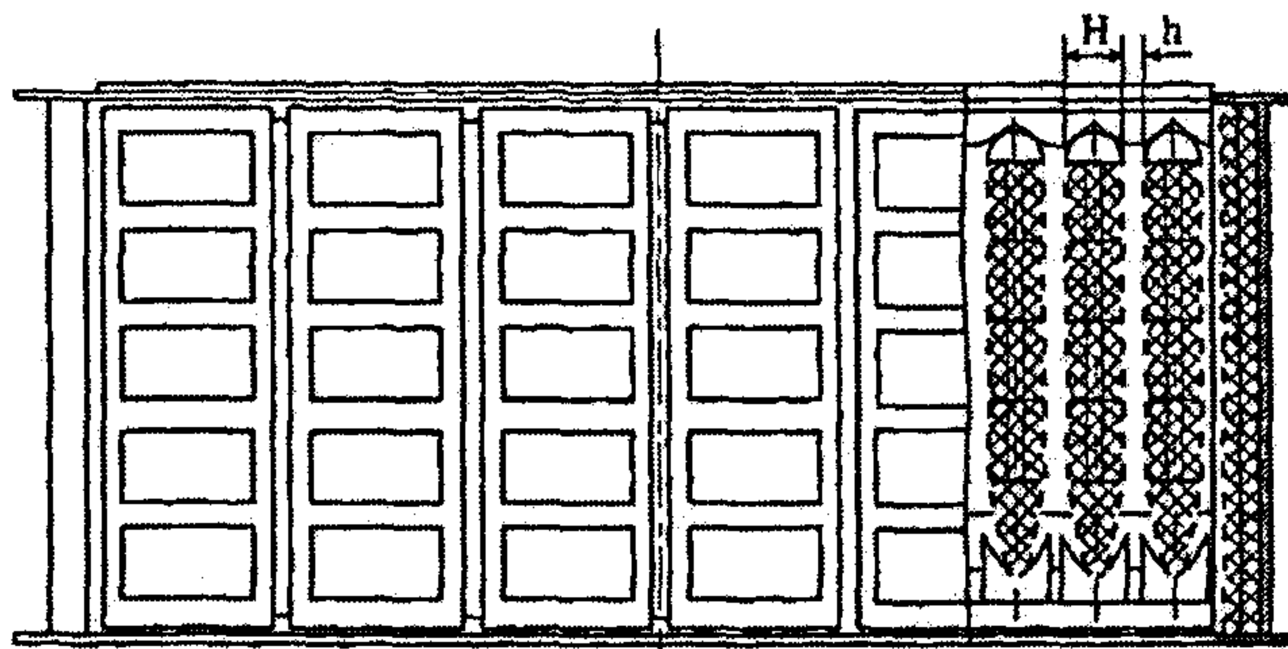
Рисунок 5 — Пластинчатый глушитель шума ГТУ
