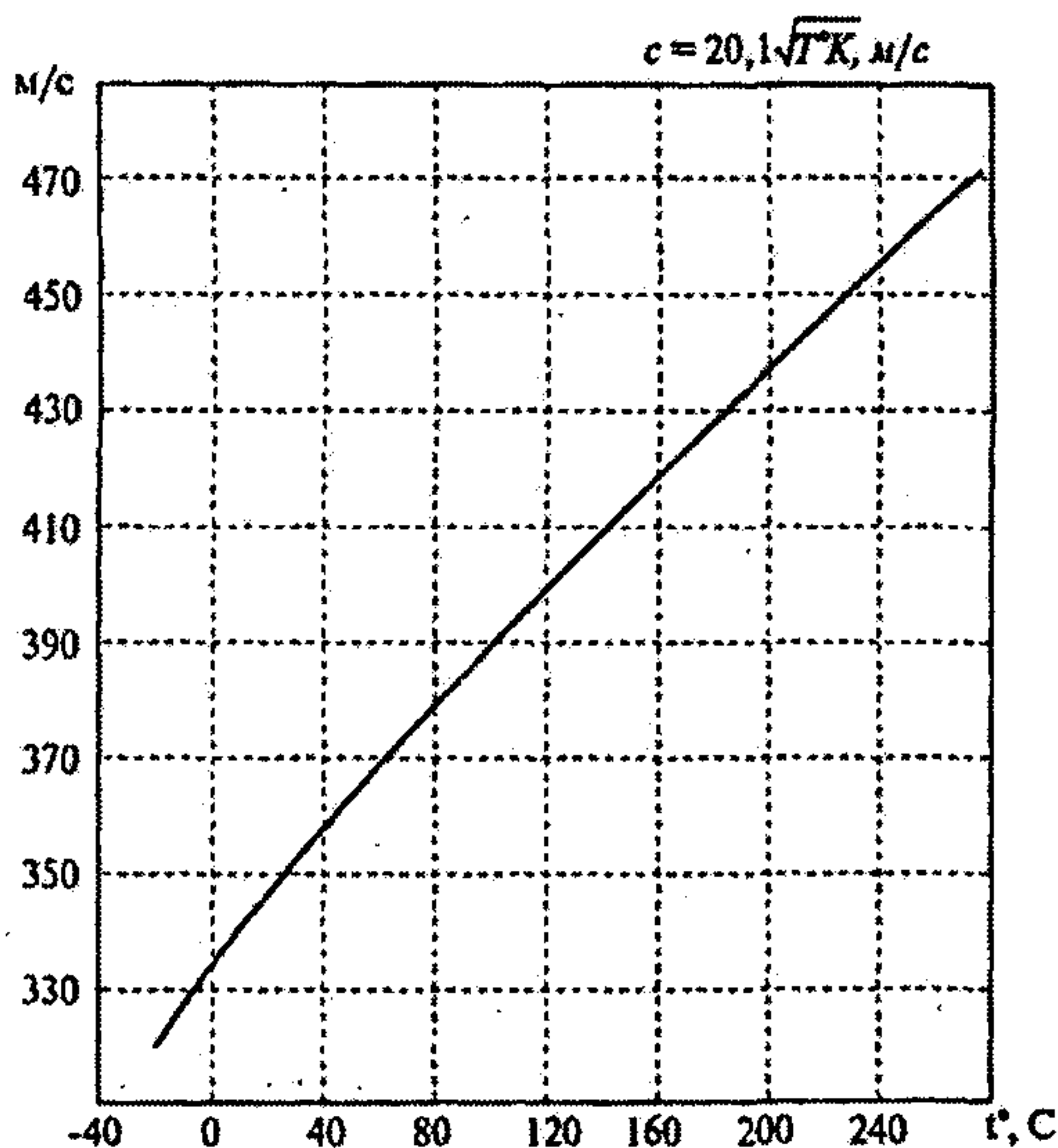
Рисунок 8 — Зависимость скорости звука от температуры газовой среды
