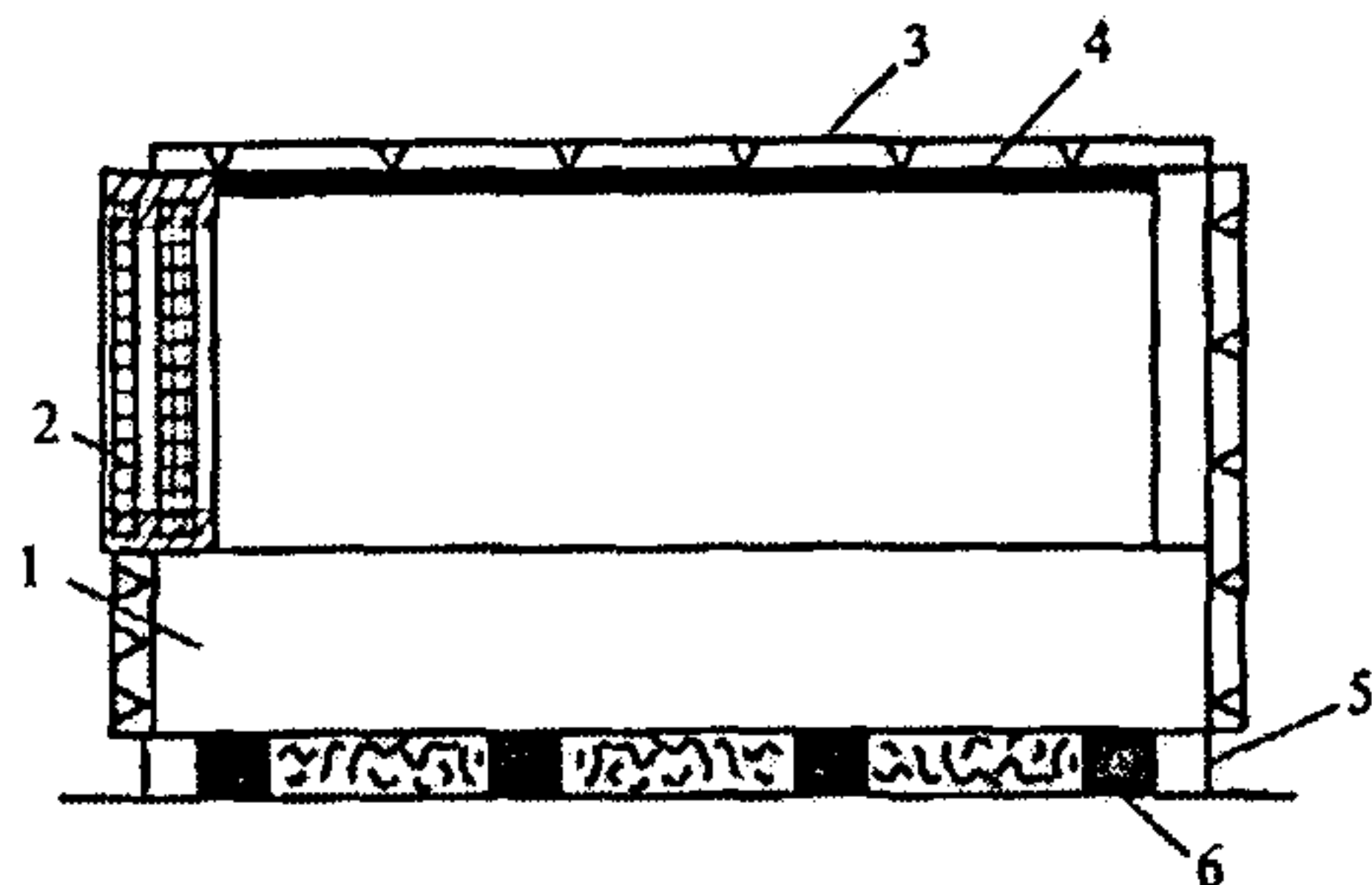
Рисунок 17 — Конструкция кабины наблюдения
