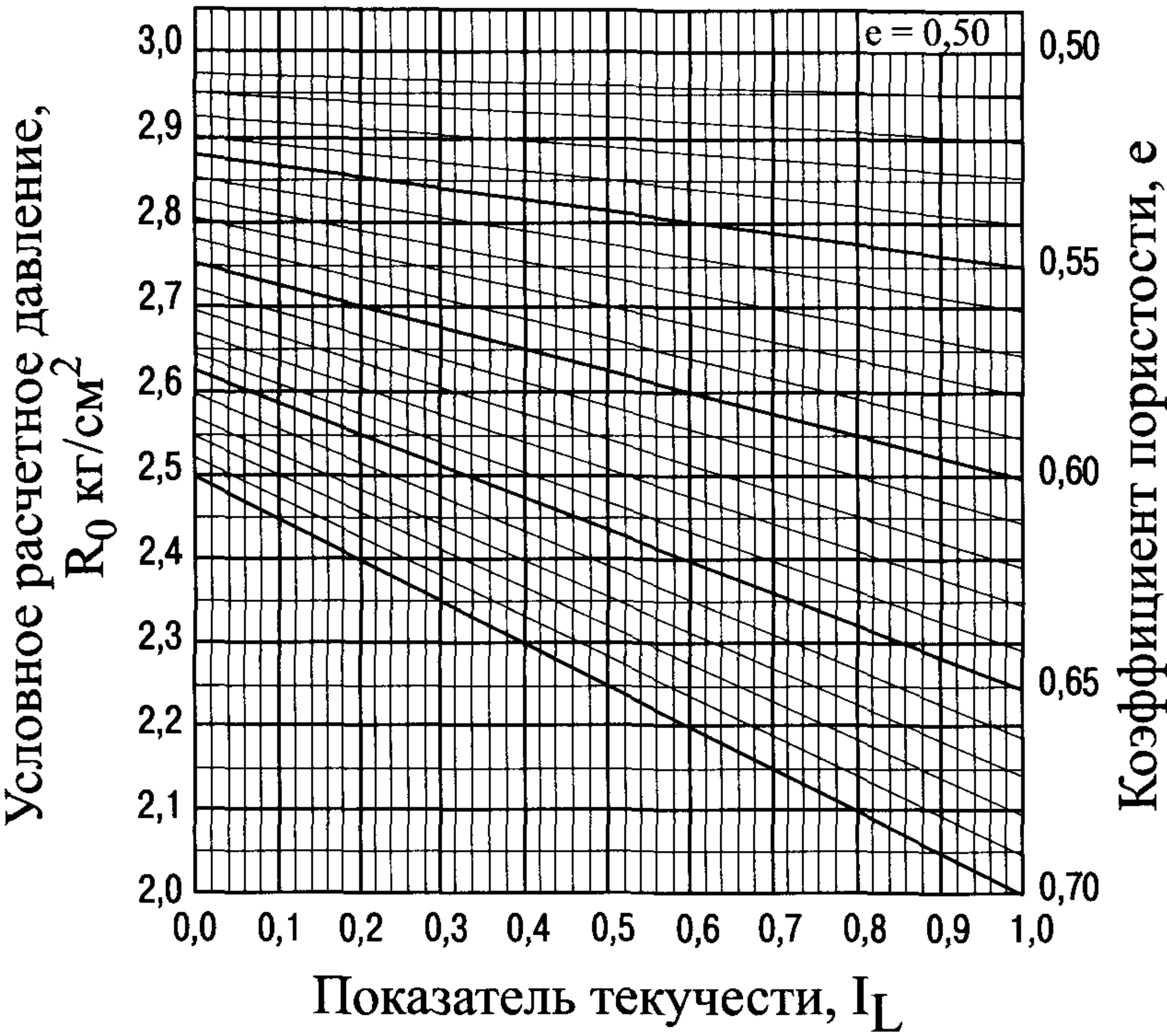
Номограмма для определения условного расчетного давления (расчетного сопротивления) R_0 на супеси [3]
