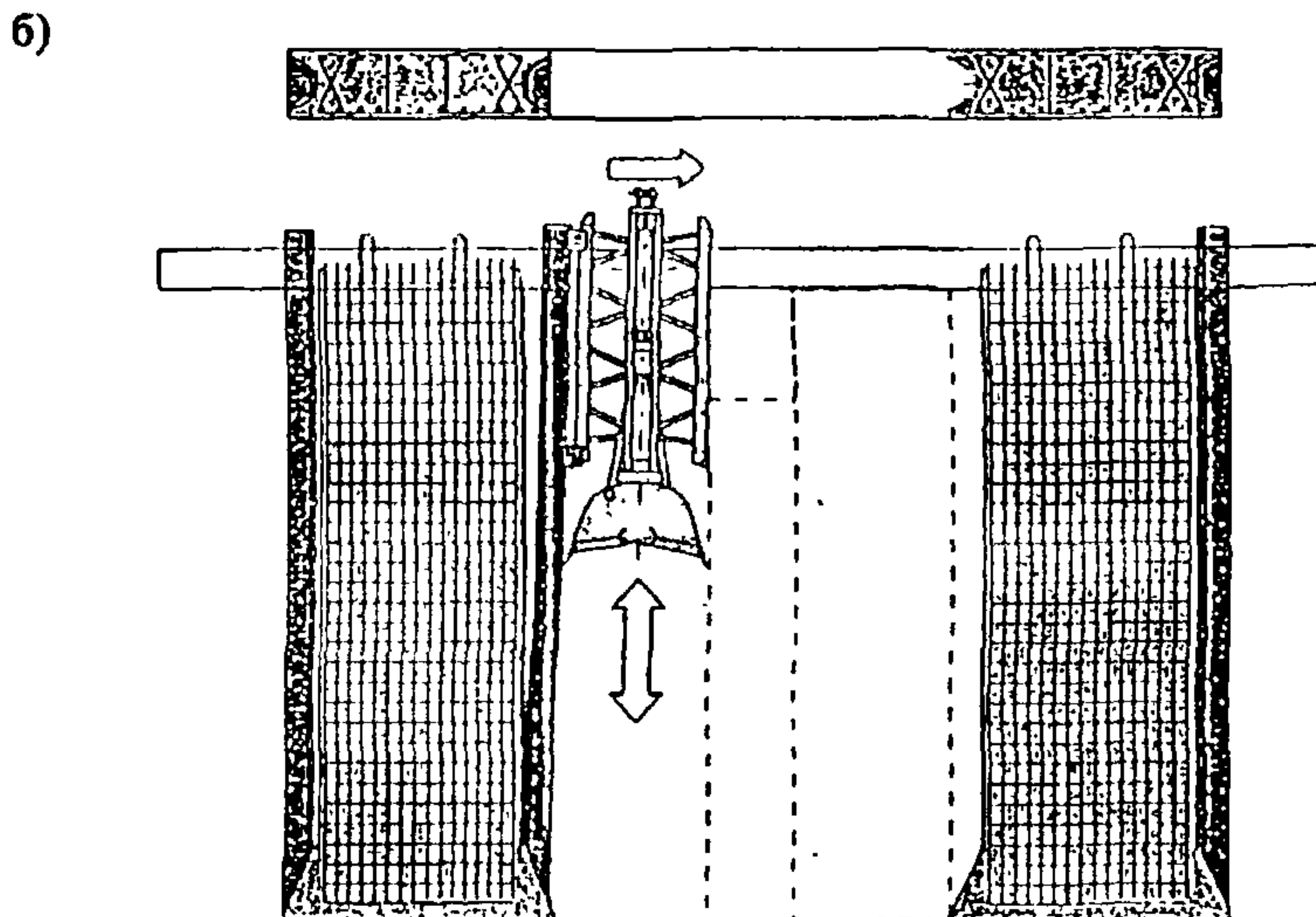
а – установка разделительных элементов с уплотнителями в захватках первой очереди, б – извлечение разделителей при проходе захваток второй очереди
