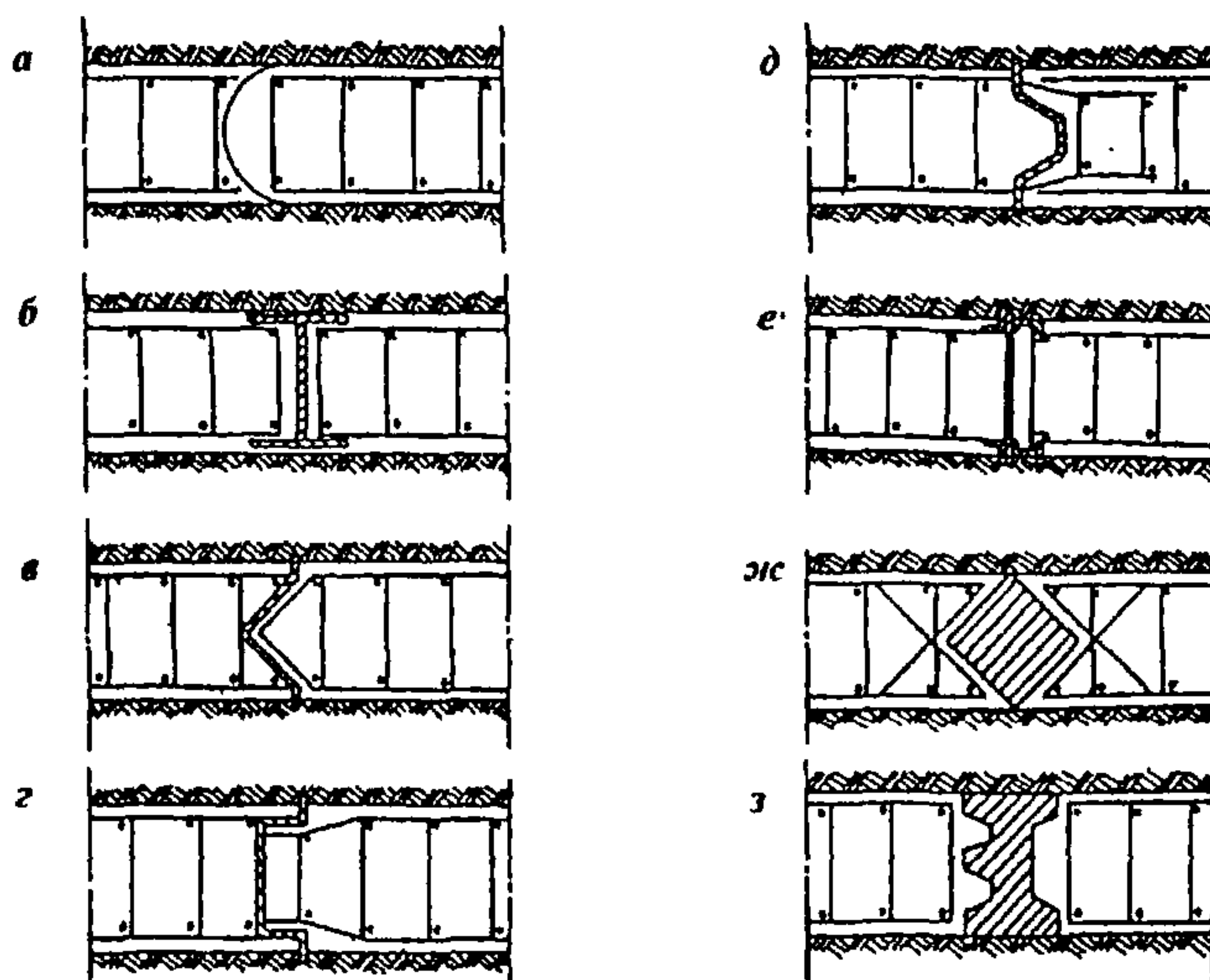
Рисунок 1 – Варианты контрфорсных стен в грунте
