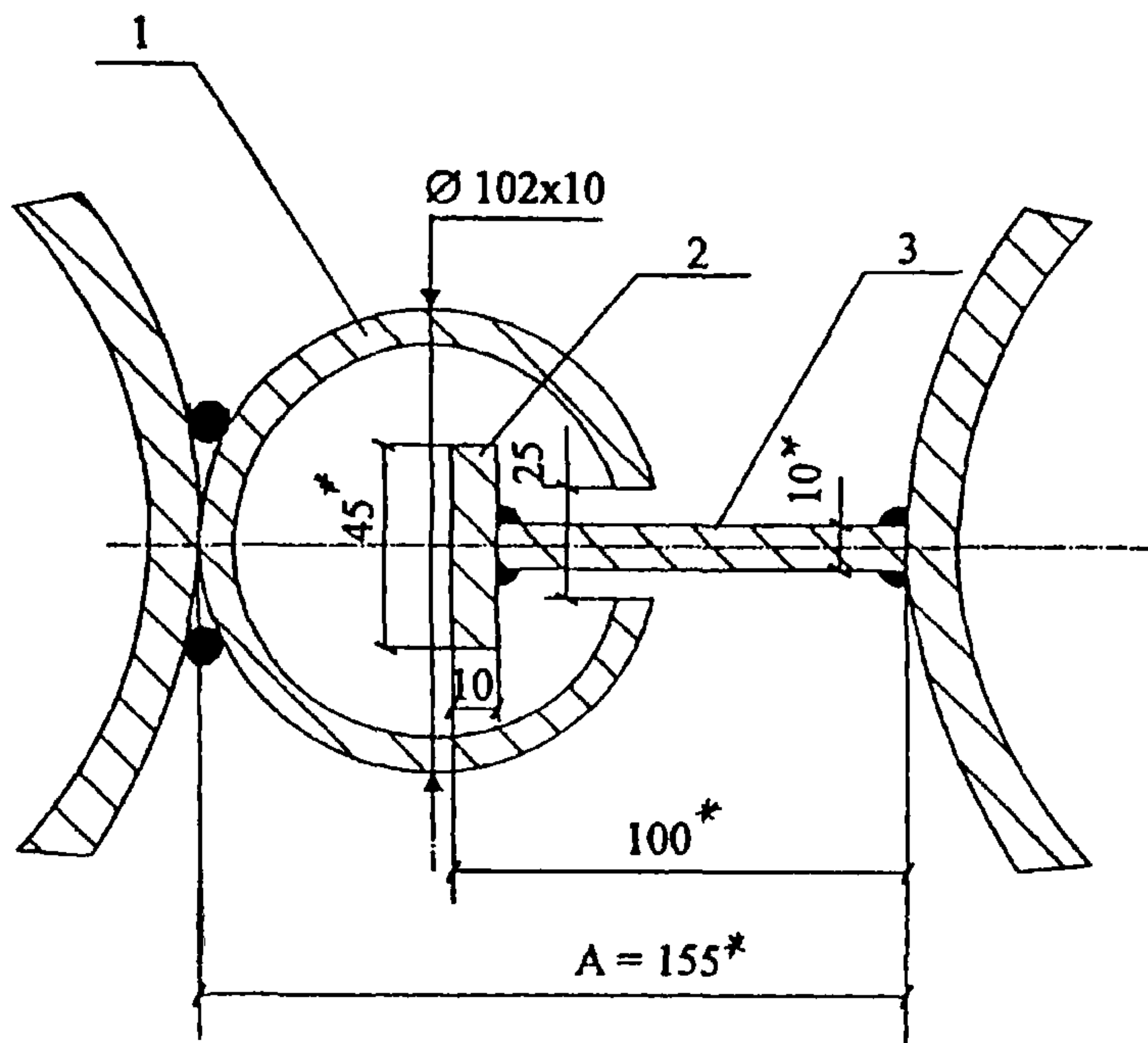
Рисунок 14 – Конструкция шпунтового замка (* – размеры приведены для справки)
